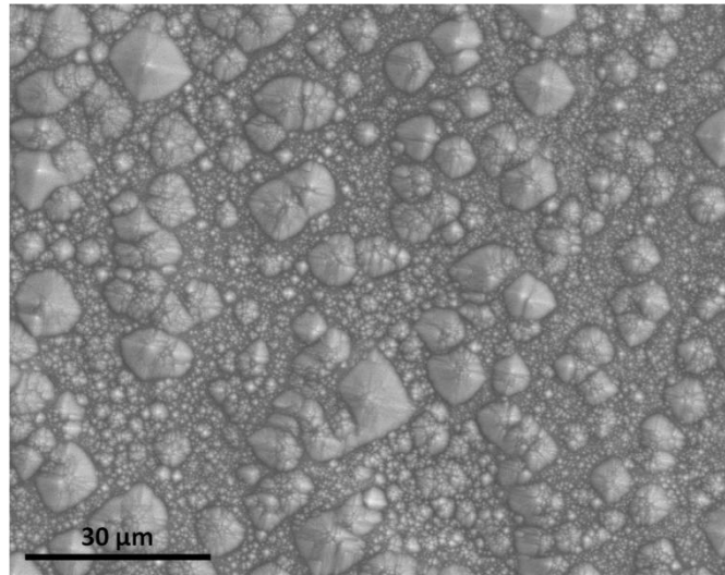
Figure IV.1 – Image MEB de la surface d'un échantillon de silicium (100) après immersion dans KOH (2mol/L) pendant 30 min
