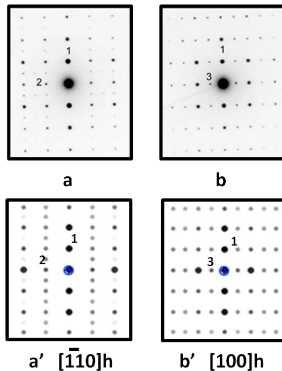
Figure III.15 – a et b) Clichés de diffraction électronique expérimentaux, sans tilt de l’échantillon, pour des nanobâtonnets fins, a’ et b’) simulations de clichés de diffraction avec la structure hexagonale de \text{WO}_3 avec d_1 = d_{(002)_h} = 0,374 nm, d_2 = d_{(110)_h} = 0,368 nm et d_3 = d_{(010)_h} = 0.638 nm
