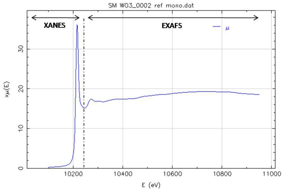
Figure II.8 – Spectre XAS au seuil L_{III} du tungstène d'une poudre de WO_3 monoclinique
