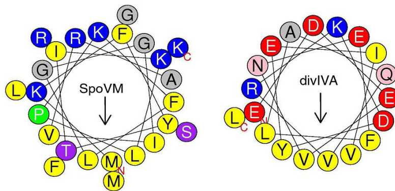
Figure 62. Représentation schématique des AAH des protéines SpoVM et divIVA de Bacillus subtilis . Codes cloueurs : en jaune, les résidus hydrophobes ; en violet, les sérines et les thréonines ; en bleu, les résidus basiques ; en rouge, les aa acides ; en rose, les asparagines et les glutamines ; en gris, les alanines. La flèche orientée vers le bas indique le moment hydrophobe. D'après (Drin and Antony, 2010).
