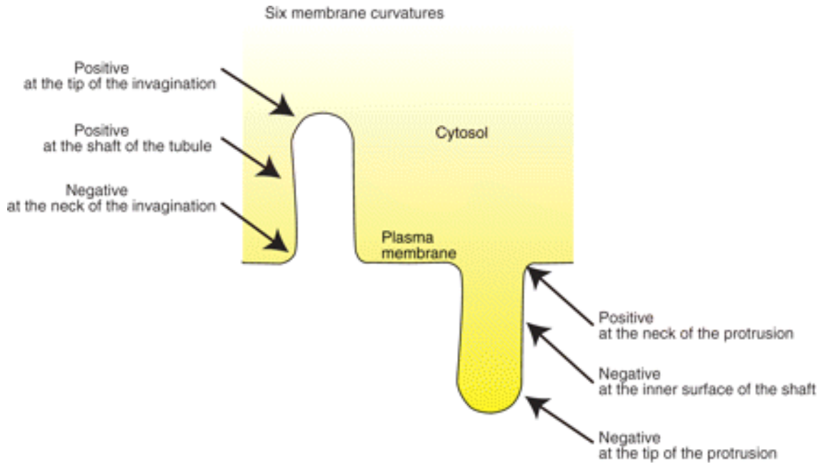
Figure 50. Courbures positives et négatives d'une membrane plasmique. D'après (Suetsugu et al. , 2010).
