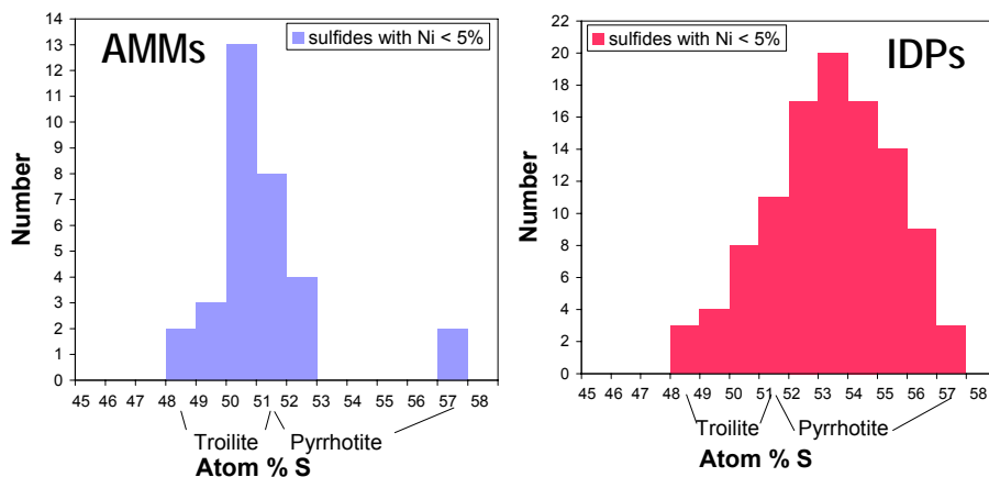
Figure 1-20 : Composition (le long de l'axe Fe-S) des sulfures de fer pauvres en Ni (< 5 at% Ni) dans les micrométéorites Concordia (AMMs, à gauche) et dans les interplanetary dust particles (IDPs, à droite). Adapté de Engrand et al. (2007b).
