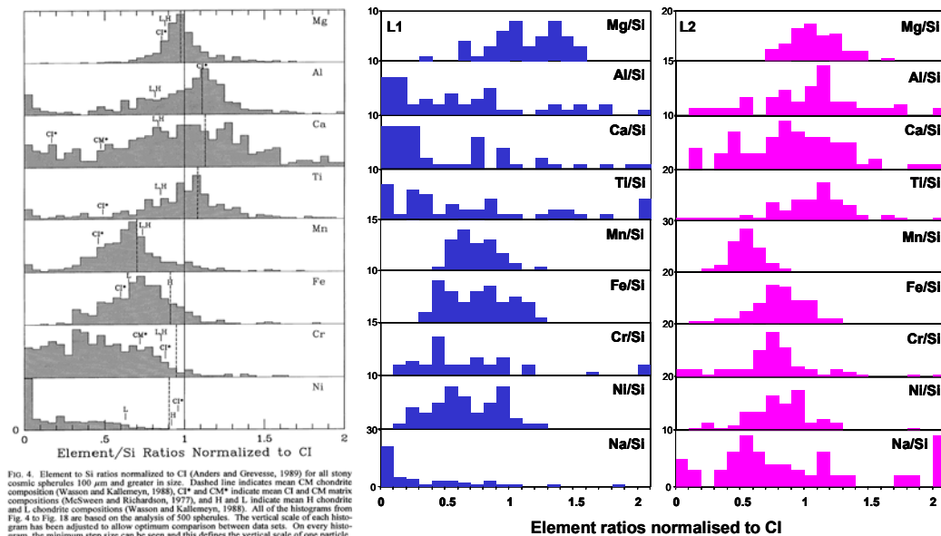
Figure 3-8 : Rapports élémentaires normalisés à Cl (Lodders 2003) et Si pour les sphérules cosmiques (Brownlee et al. 1997), et les particules des niveaux de poussières L1 (en bleu) et L2 (en rose) de la carotte de glace EPICA-Dôme C. D'après (Engrand et al. 2008a).
