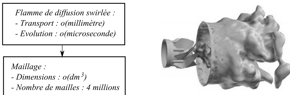
FIGURE 2.2 – LES d'une flamme de diffusion swirlée en chambre de combustion (TAC) (Selle, 2002, CERFACS, Toulouse)
