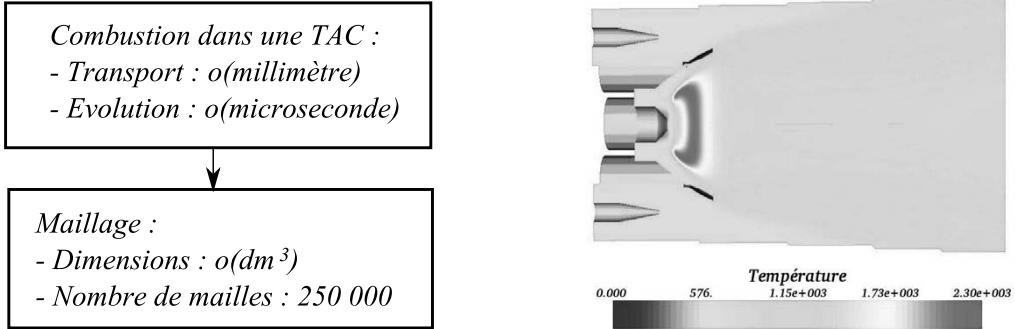
FIGURE 2.3 – Calcul RANS de combustion dans une TAC avec flamme non-prémélangée swirlée. (Fichet et al., 2007, EDF R&D, Chatou).
