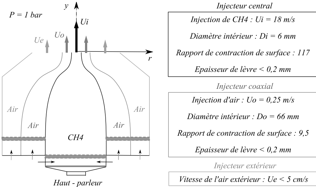
FIGURE 9.1 – Brûleur "Cocorico". Flamme méthane-air à jets coaxiaux
