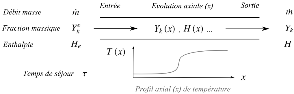
FIGURE 5.2 – Schéma descriptif d'un réacteur "piston" (PFR)
