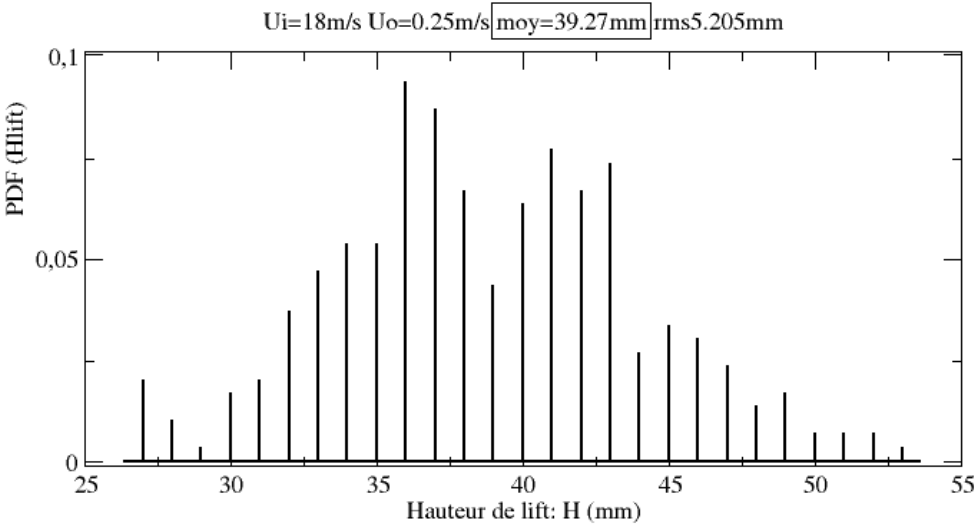
FIGURE 9.10 – Pdf de la hauteur de la flamme "Cocorico" (Wyzgolik, 2008)
