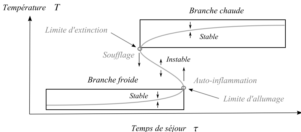
FIGURE 5.4 – Courbe hystérésis "Température - Temps de séjour" qui caractérise un réacteur parfaitement agité ( PSR )
