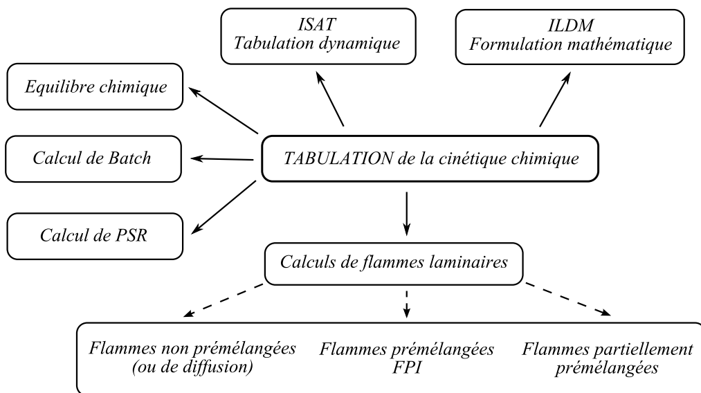
FIGURE 6.2 – Méthodes de tabulation de la cinétique chimique
