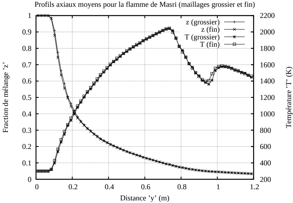
FIGURE 8.4 – Profil axiaux de fraction de mélange moyenne \tilde{z} et de température moyenne \tilde{T} pour les maillages grossier et raffiné.
