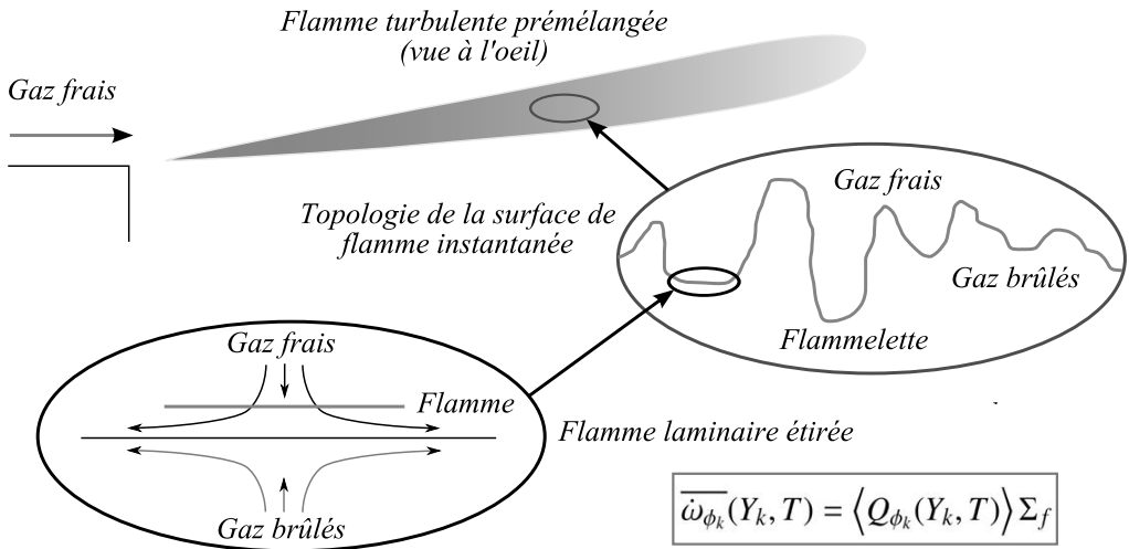
FIGURE 2.5 – Principe du modèle topologique de flammelettes étirées (de prémélange)
