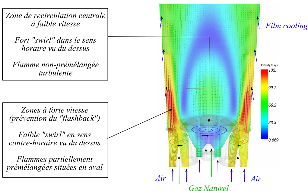
FIGURE 8.14 – Ecoulement turbulent réactif dans le tube à flamme industriel étudié.
