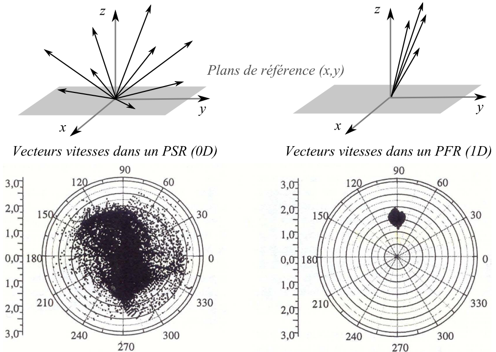
FIGURE 3.6 – Angles sagital et polaire des vecteurs vitesse dans un PSR et dans un PFR. Faravelli et al. (2001)
