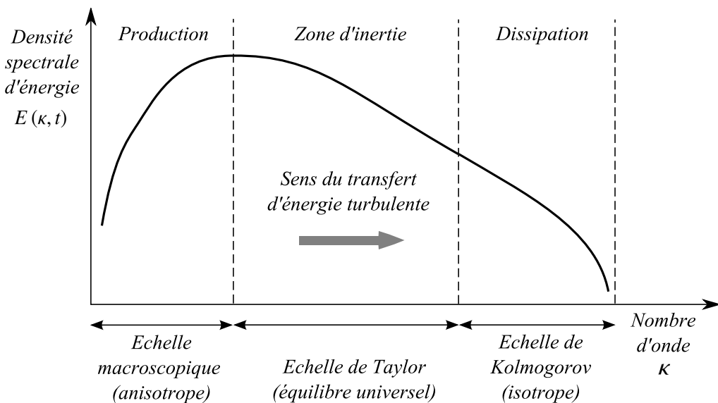
FIGURE 1.3 – Cascade d'énergie turbulente de Kolmogorov
