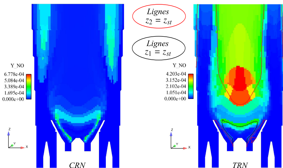
FIGURE 8.24 – Champs de Y_{NO} prédits par le CRN et le TRN dans le tube à flamme.
