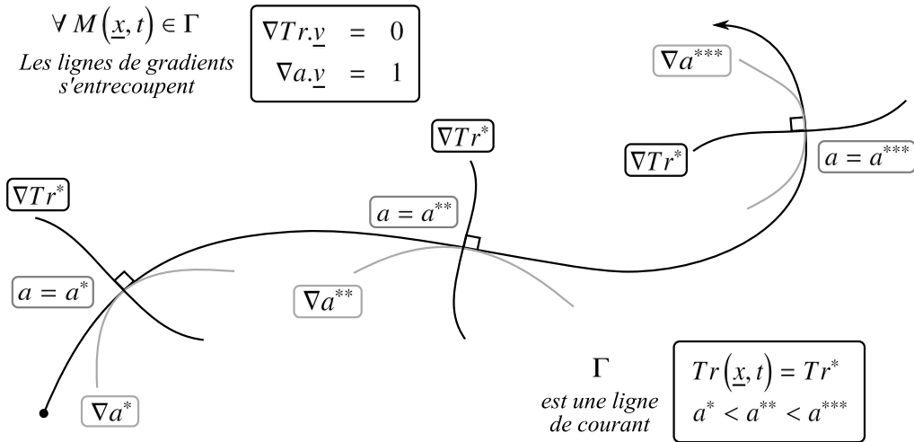
FIGURE 4.5 – Découpage de l'écoulement en zones homogènes basé sur les champs d'âge du fluide et de traceur
