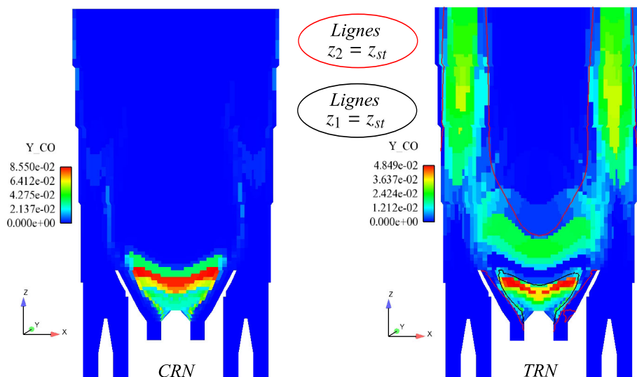
FIGURE 8.23 – Champs de Y_{CO} prédits par le CRN et le TRN dans le tube à flamme.
