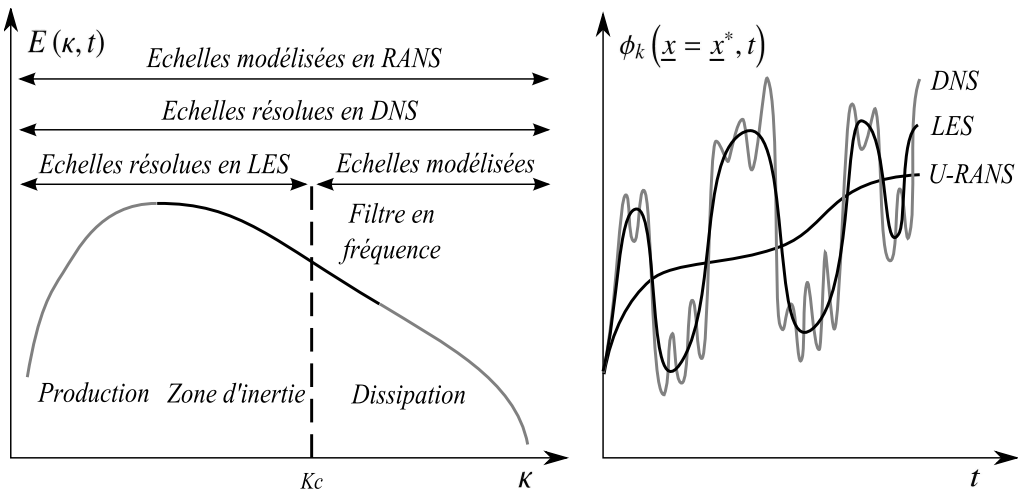
FIGURE 2.4 – Comparaison des approches DNS, LES et U-RANS dans l’espace spectral (à gauche) et temporel (à droite), inspirée de Poinot et Veynante (2005)
