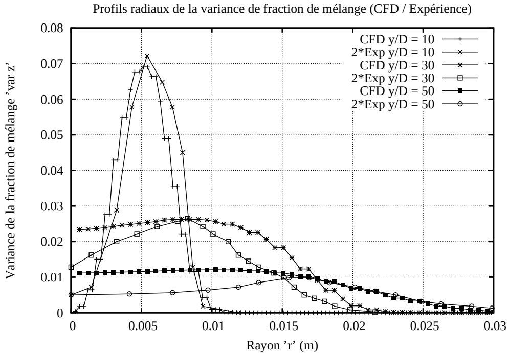
FIGURE 8.8 – Profils radiaux expérimentaux et numériques de \bar{z}''^2 .
