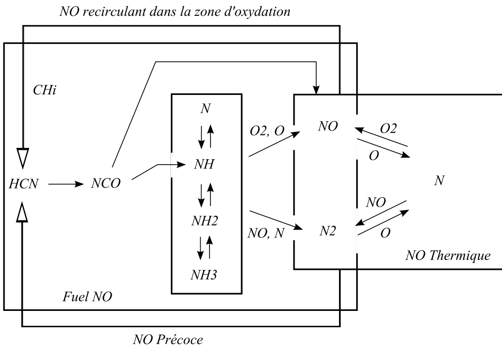
FIGURE 1.4 – Principaux mécanismes de formation du NO , inspiré de De Soete (1989)
