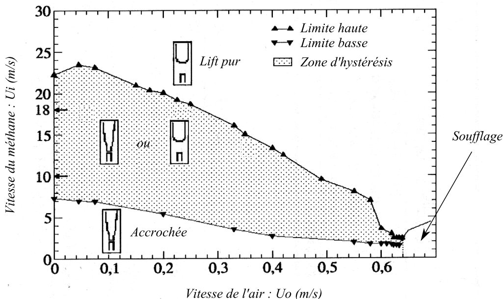
FIGURE 9.2 – Zone d'hystérésis de la flamme "accrochée - suspendue" (Wyzgolik, 2008)
