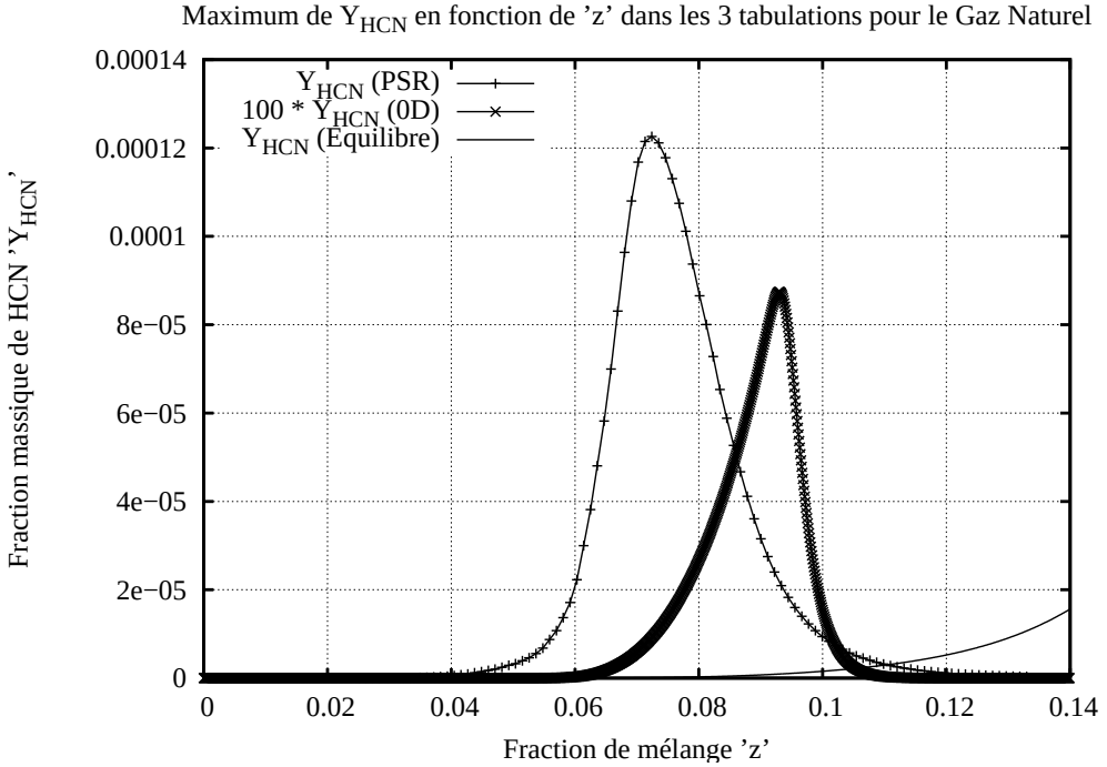
FIGURE 6.13 – Maximum de Y_{\text{HCN}} selon z dans les 3 tabulations pour le Gaz Naturel
