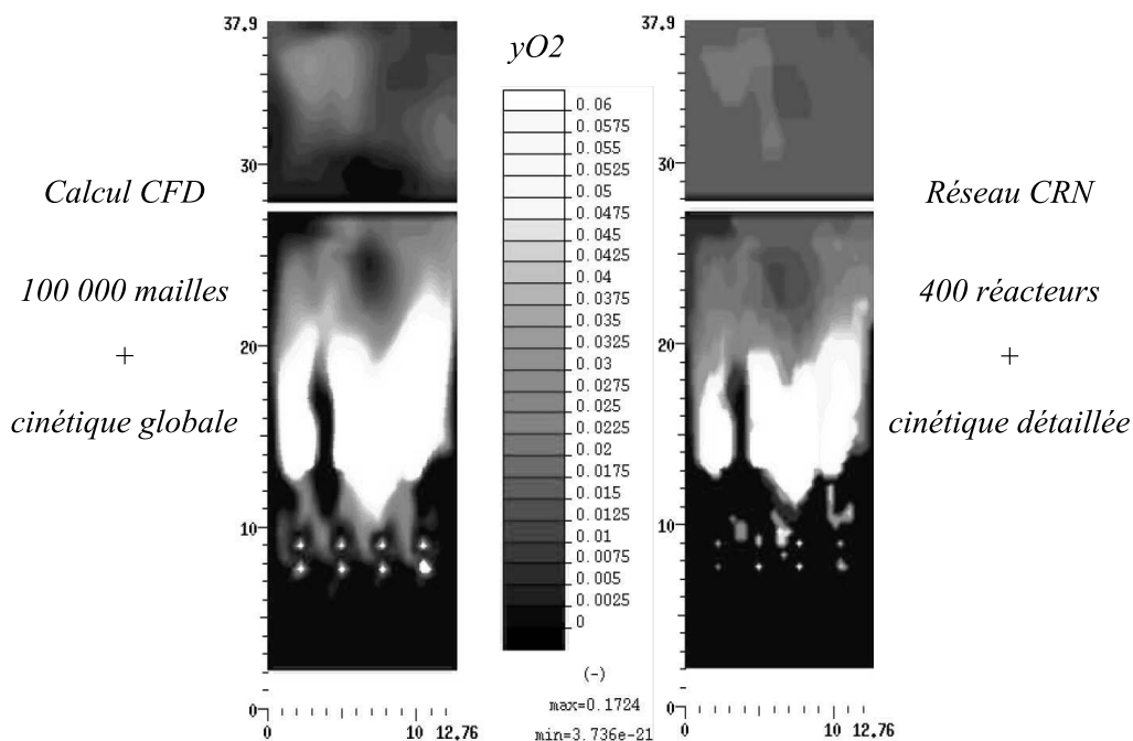
FIGURE 3.8 – Champs de fraction massique d' O_2 dans la chambre de combustion en coupe. Falcitelli et al. (2002c)
