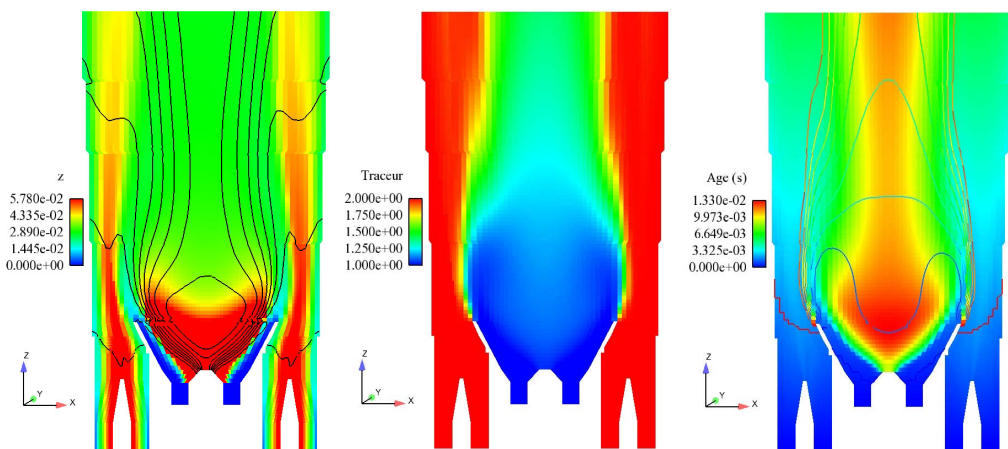
FIGURE 8.19 – Champs CFD moyens pour le tube à flamme industriel. De gauche à droite : L'interaction de z avec les iso-contours de l'âge a , le traceur Tr et son interaction avec l'âge ( quadrillage fluide ) par le biais de quelques iso-contours.
