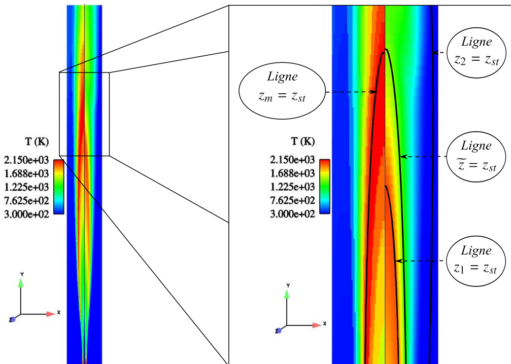
FIGURE 8.10 – Champs moyens de température T pour le CRN_212 (à gauche) et le calcul CFD (à droite). Dans le zoom, on rajoute les lignes stoechiométriques pour \tilde{z} ainsi que pour z_m , z_1 et z_2 de la pdf P(z, Y_f) du modèle LWP 4 pics (Robin et al., 2008).
