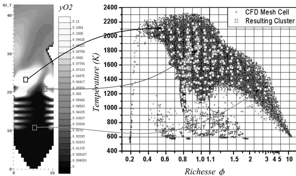
FIGURE 3.4 – Découpage dans l'espace chimique des champs CFD et réacteurs résultant de l'algorithme complet. Falcitelli et al. (2002c)
