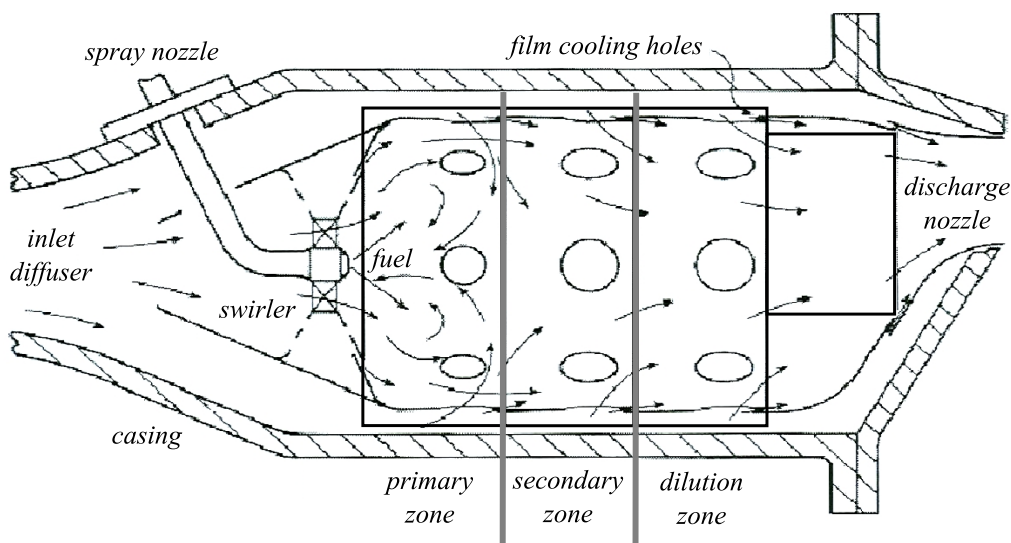
FIGURE 3.1 – Réseau de réacteurs grossier pour une chambre de combustion tubulaire
