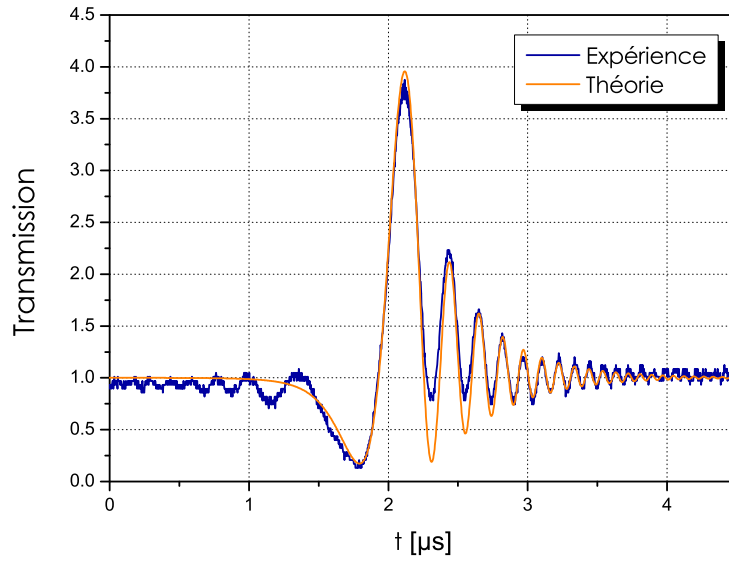
FIGURE 7.3 – Mesure en balayage rapide dans une microsphère \text{Er}^{3+} :ZBLALiP. L’ajustement du résultat dynamique permet d’identifier le régime d’amplification sélective \tau_0 = -1338 ns, \tau_e = 317 ns. La vitesse de balayage mesurée est de \tilde{V}_s = 5,6 MHz/ \mu\text{s} . Le signal à résonance présente un gain de T(0) = 4,2 dB et un retard de groupe \tau_g(0) = 1,35 \mu\text{s} .
