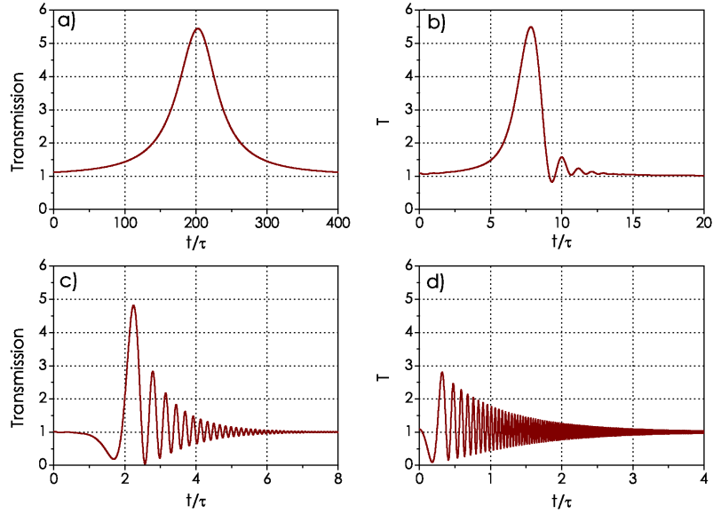
FIGURE 2.21 – Transmission en régime d'amplification pour différentes vitesses de balayage dans le cas \tau_0 = -2,5\tau_e . a) \tilde{V}_s = 0,0075 \tilde{V}_0 , b) \tilde{V}_s = 0,3 \tilde{V}_0 , c) \tilde{V}_s = 3 \tilde{V}_0 , d) \tilde{V}_s = 30 \tilde{V}_0 avec \tilde{V}_0 = 2/(\pi\tau^2) . L'axe des abscisses est normalisé par rapport au temps de vie global \tau .
