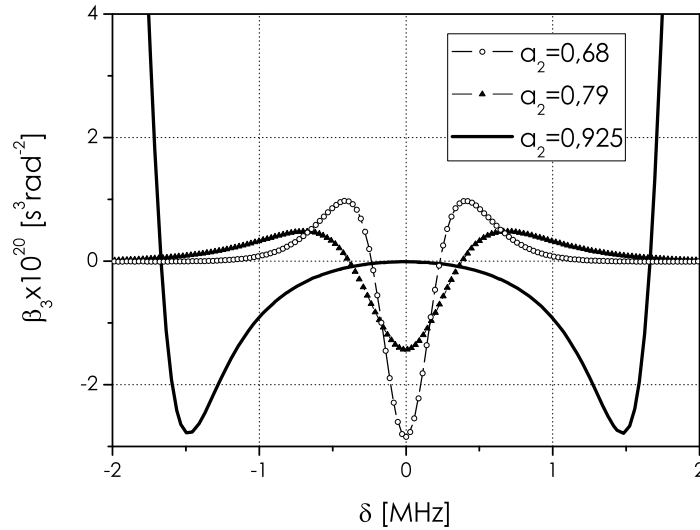
FIGURE 3.13 – Dispersion du troisième ordre pour 3 valeurs de a_2 obtenues expérimentalement. Pour a_2 = 0,925 la dispersion d’ordre 3 s’annule à résonance.
