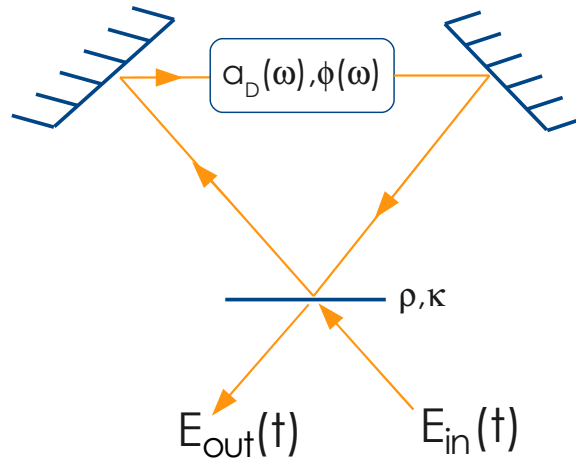
FIGURE 4.1 – Schéma d'une cavité en anneau contenant un milieu dispersif introduisant une phase supplémentaire \phi(\omega) et des pertes a_D(\omega) . Les coefficients de réflexion et de transmission du miroir d'entrée/sortie sont respectivement \rho et \kappa . Les deux autres miroirs sont totalement réfléchissants. Les champs d'entrée E_{in} et E_{out} sont reliés par la fonction de transfert en intensité T [Equ. (4.4)].
