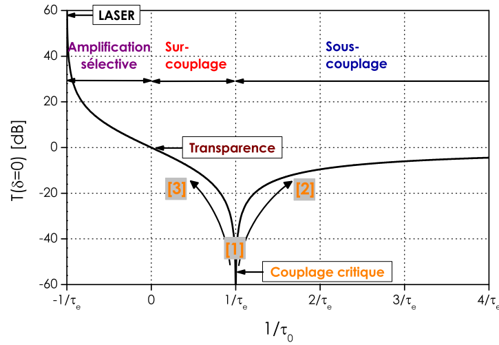
FIGURE 2.12 – Présentation des régimes de couplage étudiés dans le cadre de la validation expérimentale de la méthode de CRDM.
