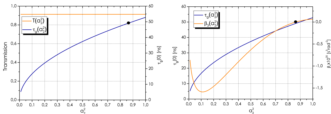
(a) Transmission et retard de groupe d'un CRIT en fonction des pertes intrinsèques a_2^2 . (b) Retard de groupe et dispersion d'ordre 3 d'un CRIT en fonction des pertes intrinsèques a_2^2 .
