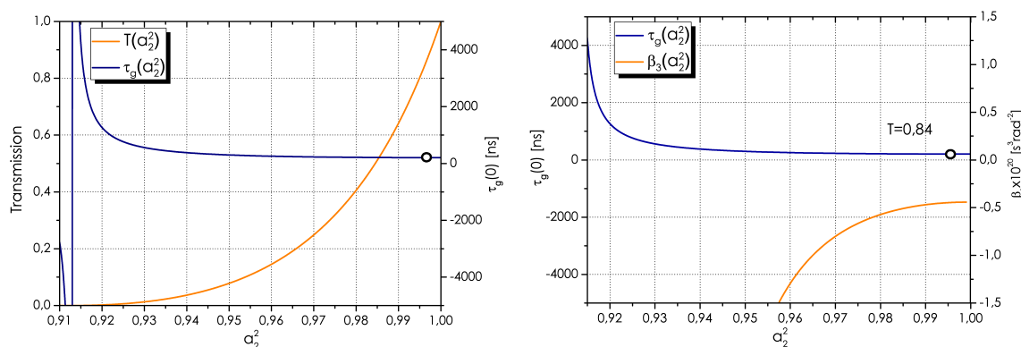
(c) Transmission et retard de groupe d'une cavité unique en fonction des pertes intrinsèques a_2^2 . (d) Retard de groupe et dispersion d'ordre 3 d'une cavité unique en fonction des pertes intrinsèques a_2^2 .
