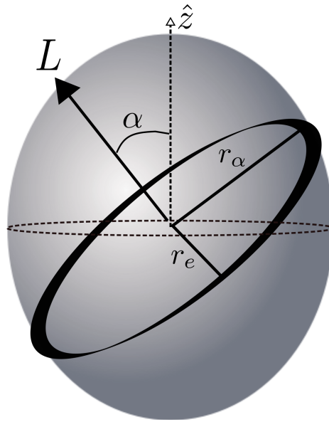
FIGURE 5.3 – Représentation d'un sphéroïde de type prolata. Un champ électromagnétique le parcourt en décrivant une ellipse caractérisée par ses axes r_\alpha et r_e et son angle d'inclinaison \alpha .
