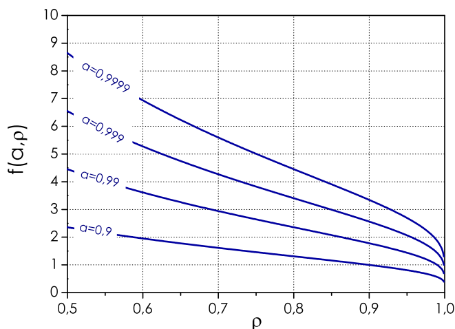
FIGURE 4.4 – Représentation de la fonction f(a, \rho) en fonction de \rho pour différentes valeurs du coefficient de perte a .
