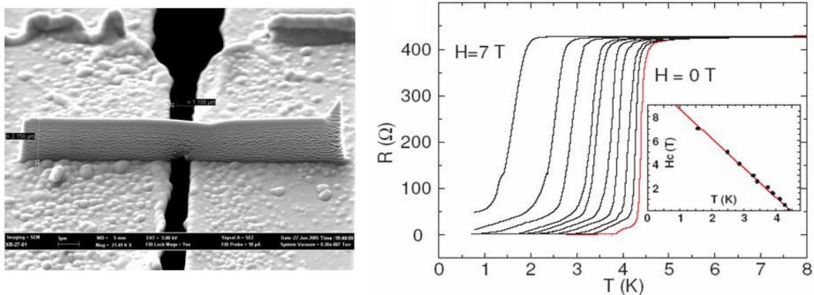
Figure 51 Propriétés d'un fil de W supraconducteur, en partie suspendu, réalisé au FIB (faisceau d'ions focalisés) (A. Kasumov et R. Deblock).
