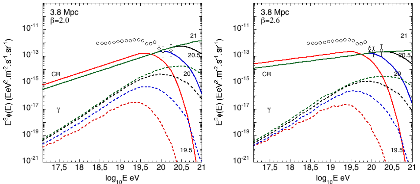
FIG. 5.16 – Influence d'une source proche sur les flux de photons secondaires : spectres propagés des RCUHEs et photons secondaires, depuis une source placée à 3.8 Mpc, avec une composition pur-proton et un indice spectral d'injection \beta = 2.6 . Quatre énergies maximales d'accélération aux sources sont considérées : 10^{21} eV (vert), 10^{20.5} eV (noir), 10^{20} eV (bleu), et 10^{19.5} eV (rouge). Les données d'Auger (RCUHEs) sont tracées (ronds noirs). On a redressé tous les spectres par E^3 pour une meilleure visibilité.
