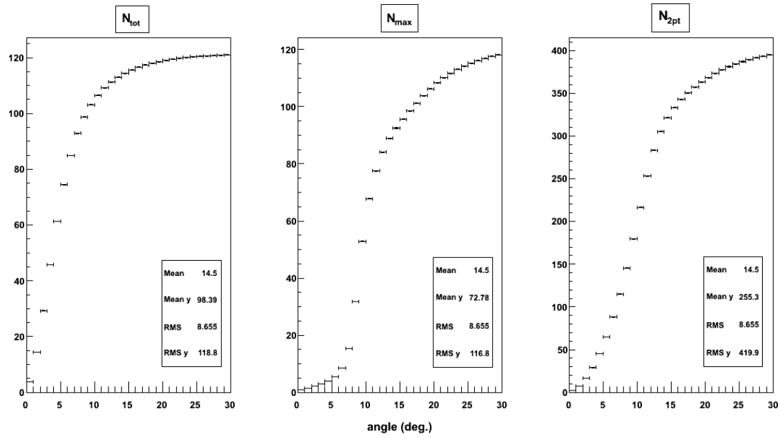
FIG. 8.10 – Valeurs moyennes de trois observables différentes en fonction de l'échelle angulaire considérée, pour tous les seuils en énergie et pour des réalisations isotropes.
