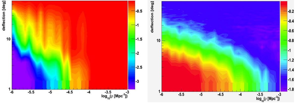
FIG. 7.4 – Pouvoir de rejet des deux tests pris individuellement, et utilisés pour construire le double-test. On a tracé \mathcal{P}_{\pm}^0 pour chaque modèle (n_s, \delta) testé ( n_s \equiv \rho ). Gauche : on a cherché pour chaque modèle (n_s, \delta) , la fraction minimum \mathcal{P}_{\pm, \min}^0 des simulations dudit modèle ayant moins de paires que les données d’Auger. Les données étant assez peu clusterisées, il est difficile pour un modèle à peu de sources et petites déflexions d’avoir encore moins de paires que les données. C’est pourquoi la zone (violette) concentrée en bas à gauche donne des petites fractions et donc des petites \mathcal{P}_{\pm}^0 (cf. figure 6.10). Droite : on a cherché pour chaque modèle (n_s, \delta) , la fraction minimum \mathcal{P}_{\pm, \min}^0 des simulations dudit modèle ayant plus de paires que les données d’Auger. Les données étant assez peu clusterisées, il est aisé pour un modèle à peu de sources et petites déflexions d’avoir plus de paires que les données, car ce sont des modèles fortement anisotropes, qui donnent aisément un fort clustering, tout du moins plus que les données. C’est pourquoi la zone (rouge) concentrée en bas à gauche donne des grandes fractions et donc des grandes \mathcal{P}_{\pm}^0 (cf. figure 6.10). A l’inverse, les modèles peu clusterisés (densité et déflexions fortes) donnent rarement un clustering plus important que les données, et les fractions observées, tout comme leur \mathcal{P}_{\pm}^0 associée, sont faibles : c’est une zone où les modèles sont rejetés avec une significativité supérieure à 98%.
