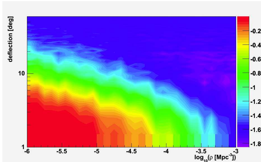
FIG. 7.3 – Log. de \mathcal{P}_+ pour le test des données sur les modèles de sources homogènes.
