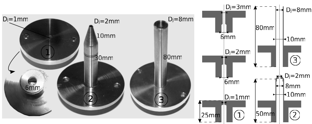
FIGURE 6.3 – Photographies des buses plates (1) et sur-élevées (2) et (3)
