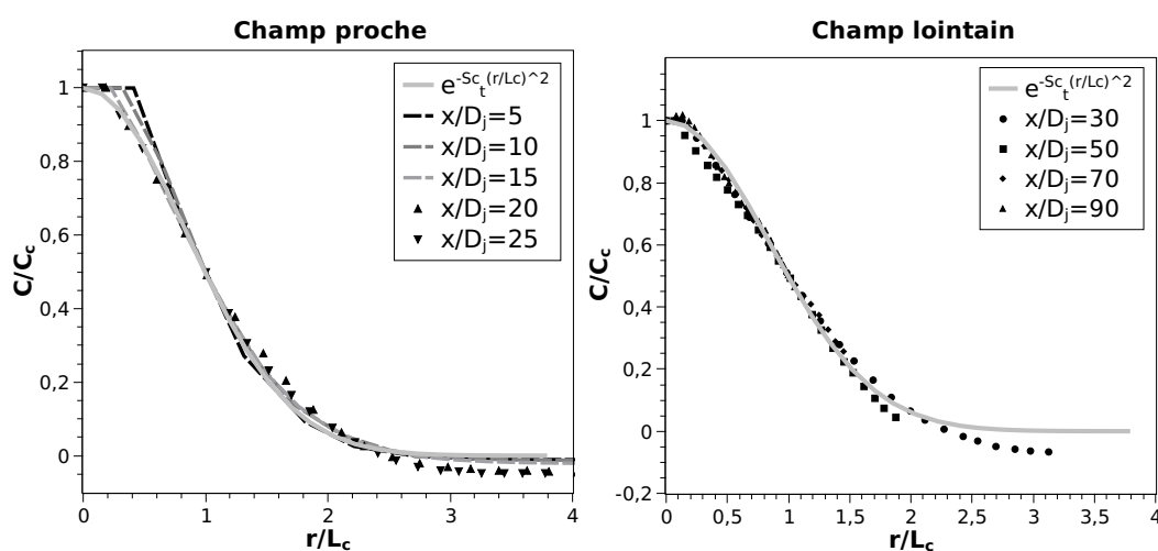
FIGURE 9.2 – Superposition des profils radiaux de la concentration moyenne, normalisés par la valeur maximale sur l'axe et par la demi-largeur de profil moyen pour un jet d'hélium de D_j = 2 mm et Re_j = 3000 (BOS101, annexe E.8)
