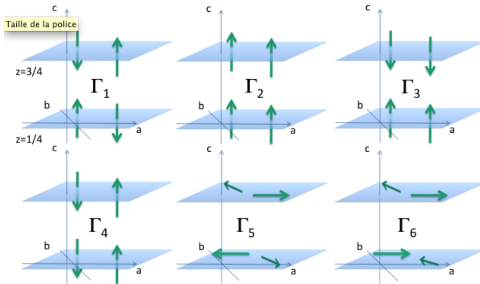
FIGURE 4.3 – Configurations magnétiques accessibles aux ions de terre rare sur le site cristallographique 4b. Les représentations \Gamma_1^R à \Gamma_4^R correspondent à des moments alignés le long de l'axe c , les configurations \Gamma_5^R et \Gamma_6^R à des moments alignés le long des axes a et b .
