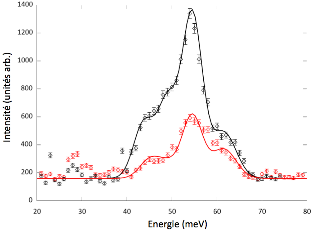
FIGURE 7.28 – Evolution de l'intensité diffusée à haute énergie pour Q=(0\ 0\ 6) (noir) et Q=(0\ 0\ 12) (rouge). La diminution d'intensité des excitations entre 40 et 65 meV est due au facteur de forme magnétique.
