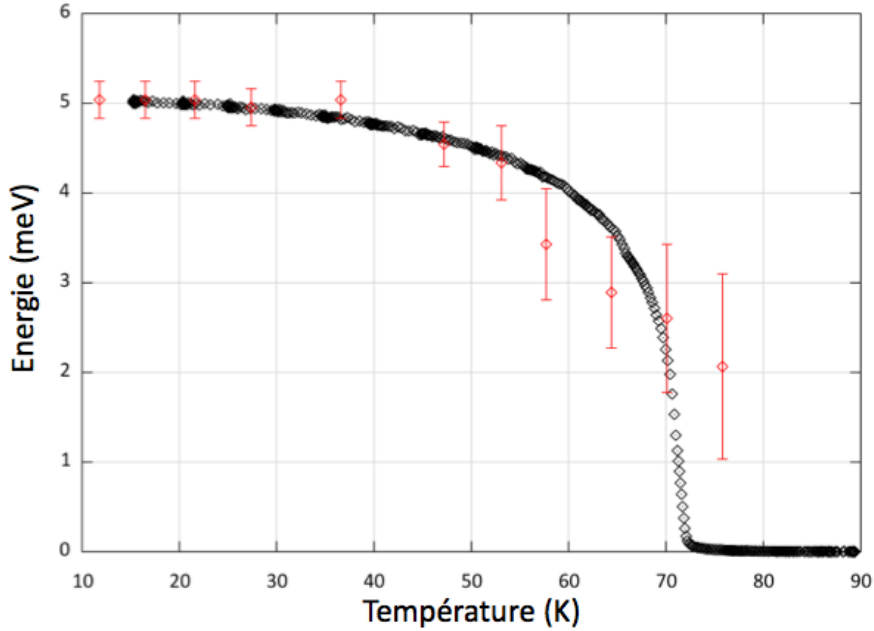
FIGURE 7.16 – Evolution du gap d'anisotropie planaire (rouge) et de S_i (noir) en fonction de la température dans le composé \text{YMnO}_3 .
