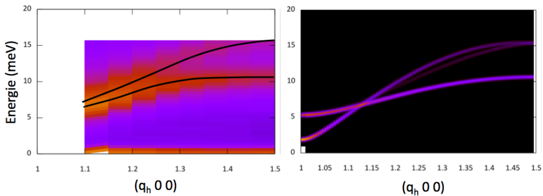
FIGURE 7.11 – Gauche : carte en fausses couleurs de l'intensité diffusée par le composé \text{YMnO}_3 dans la directions Q = (q_h\ 0\ 0) ; les lignes noires sont des guides pour l'oeil. Droite : carte en fausses couleurs du facteur de structure dynamique calculé pour des valeurs de J_{plan} = 2.55\ \text{meV} et D = 0.55\ \text{meV} .
