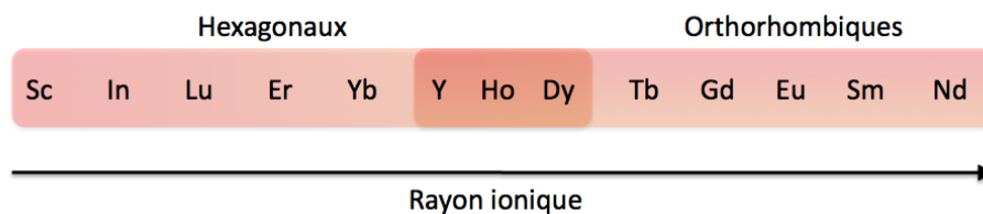
FIGURE 1.9 – Evolution de la structure stabilisée par les composés \text{RMnO}_3 en fonction du rayon de la terre rare. La structure des composés intermédiaires est dépendante des conditions de synthèse.
