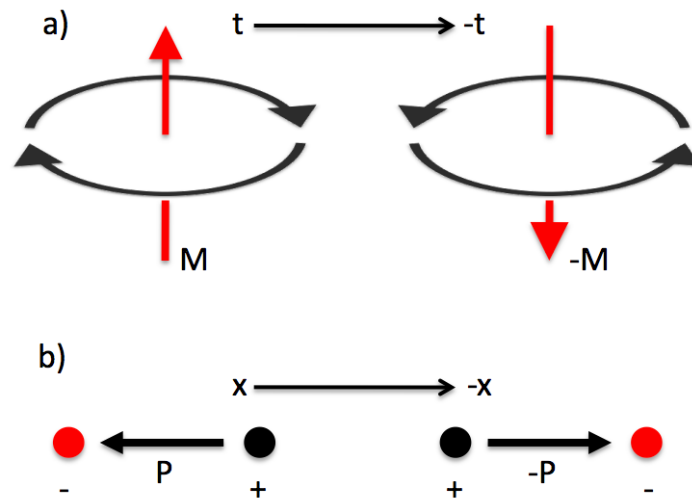
FIGURE 1.4 – a) Comportement de l'aimantation par application du renversement du temps. L'aimantation générée par le courant circulant dans la spire est renversée, l'inversion du temps inversant le sens de circulation du courant. b) Comportement de la polarisation par application du renversement de l'espace. L'échange des positions des charges + et - induit une inversion de la polarisation.
