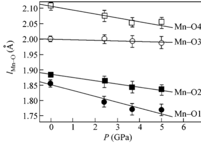
FIGURE 5.8 – Evolution des distances MnO 3 et MnO 4 en fonction de la pression appliquée sur l'échantillon. On observe une symétrisation progressive des chemins d'échange [Koz08].
