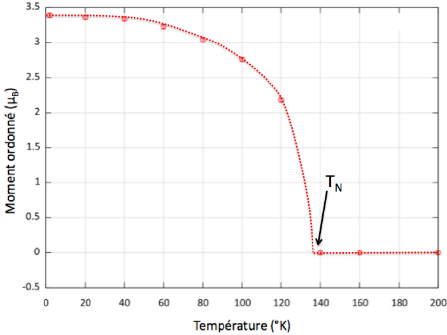
FIGURE 4.10 – Evolution du moment ordonné des Mn en fonction de la température. La T_N est marquée par l'apparition d'un moment ordonné à T = 137 \text{ K} .
