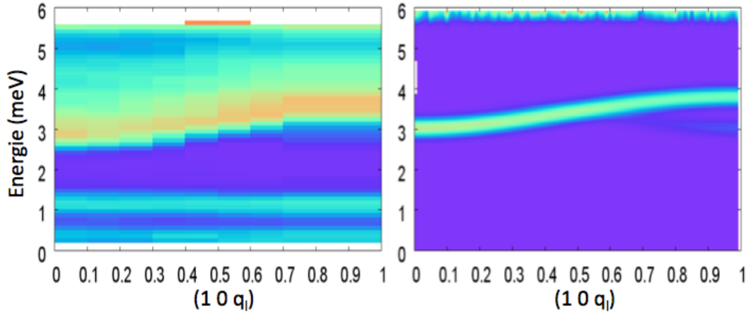
FIGURE 7.20 – Gauche : carte en fausses couleurs de l'intensité diffusée par le composé YbMnO 3 dans la direction (1 0 q_l ). Droite : Droite : carte en fausses couleurs du facteur de structure dynamique calculé pour des valeurs de J_{z_{eff}} = -0.012(2) \text{ meV} , D = 0.75 \text{ meV} et h = 0.2 \text{ meV} .
