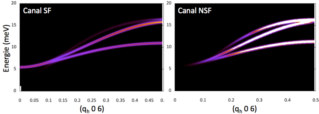
FIGURE 8.11 – Carte en fausses couleurs de l’intensité diffusée calculée dans le canal SF (gauche) et dans le canal NSF (droite) pour les \text{RMnO}_3 hexagonaux. L’existence d’intensité diffusée dans le canal NSF en bord de zone traduit l’existence d’une excitation de réseau de même énergie que les ondes de spin observées dans le canal SF. L’hybridation se produit donc en bord de zone à l’inverse de nos observations expérimentales.
