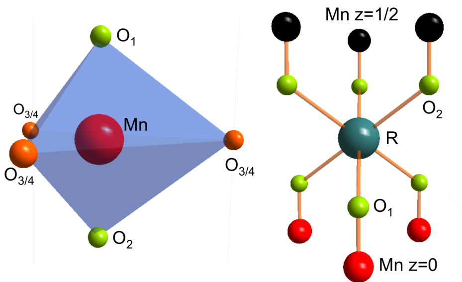
FIGURE 3.3 – Bipyramide \text{MnO}_5 et liaisons \text{R-O-Mn} .
