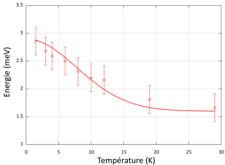
FIGURE 7.22 – Evolution du gap d’anisotropie uniaxiale dans le composé \text{YbMnO}_3 en fonction de la température. La ligne est un guide pour l’œil.
