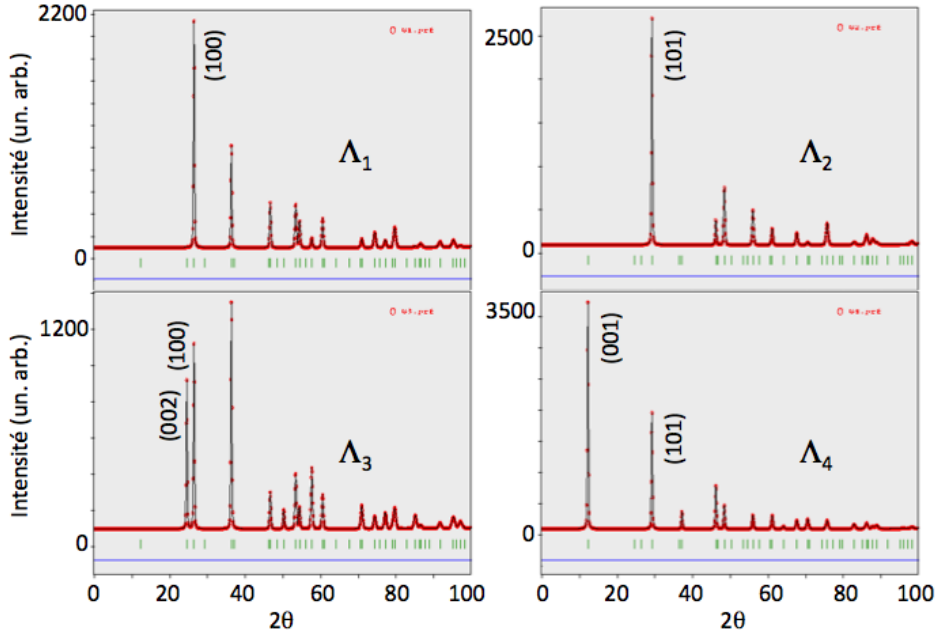
FIGURE 4.7 – Diffractogrammes magnétiques calculés pour les configurations \Lambda_1 à \Lambda_4 des ions \text{R}(2a) . Seule la contribution magnétique des ions de terre rare \text{R}(2a) est représentée. Chacune des configurations est facilement identifiable.
