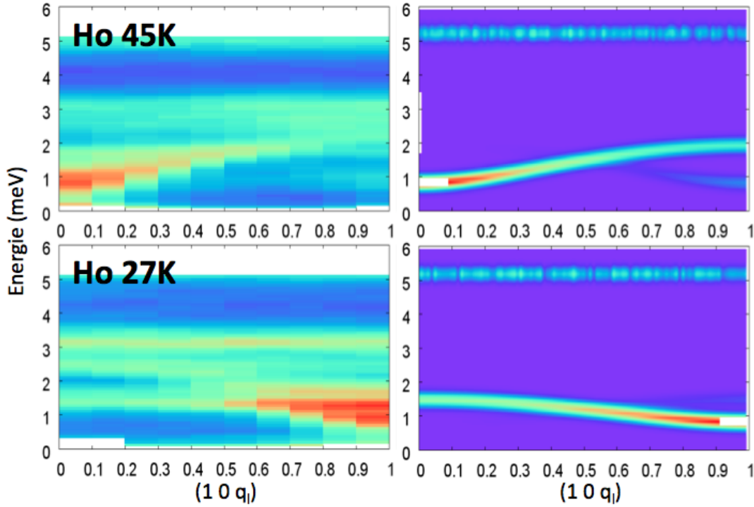
FIGURE 7.27 – Gauche : carte en fausses couleurs de l’intensité diffusée par le composé \text{HoMnO}_3 dans la direction (1\ 0\ q_{||}) . Droite : carte en fausses couleurs du facteur de structure dynamique calculé pour des valeurs de J_{z_{eff}}(45K) = -0.0038(5)\text{ meV} , D = 0.65\text{ meV} et h = 0.1\text{ meV} et J_{z_{eff}}(27K) = 0.0018(5)\text{ meV} , D = 0.65\text{ meV} et h = 0.1\text{ meV} .
