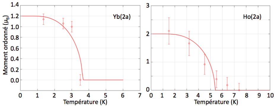
FIGURE 4.27 – Evolution du moment ordonné des ions \text{R}(2a) en fonction de la température et ajustement par une fonction de Brillouin dans \text{YbMnO}_3 (gauche) et \text{HoMnO}_3 (droite).
