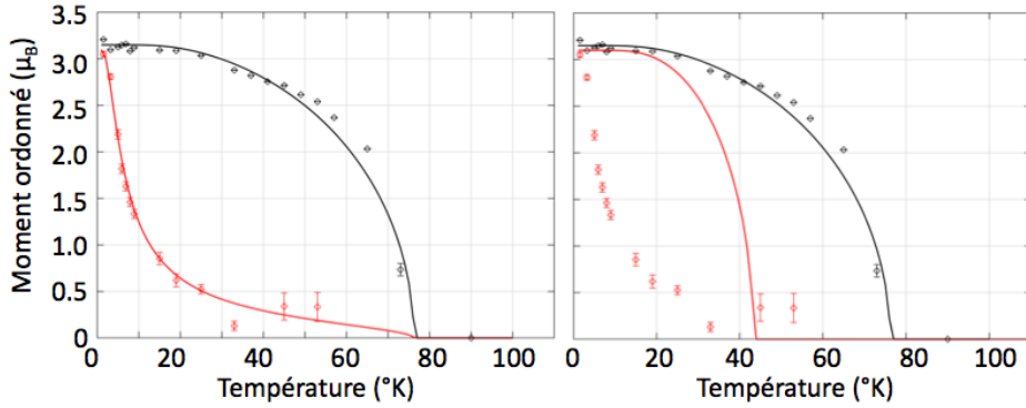
FIGURE 4.26 – \text{HoMnO}_3 : ajustement du moment ordonné des ions \text{Ho}(4b) (rouge) et \text{Mn} (noir) par une fonction de Brillouin. Gauche : prise en compte des interactions \text{Ho}/\text{Mn} uniquement. Droite : prise en compte des interactions \text{Ho}/\text{Ho} uniquement.
