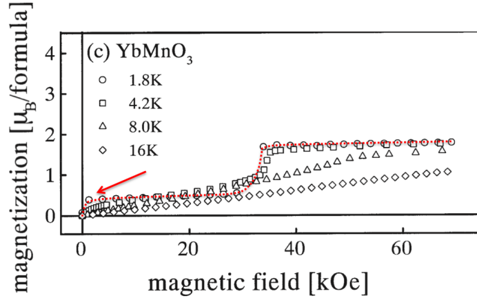
FIGURE 4.18 – Courbe d’aimantation du composé \text{YbMnO}_3 en fonction du champ extérieur appliqué. La courbe à T = 1.8\text{ K} (pointillés rouges) est caractérisée par un saut dans l’aimantation à de très faibles valeurs de champ (flèche rouge) [Sug02].
