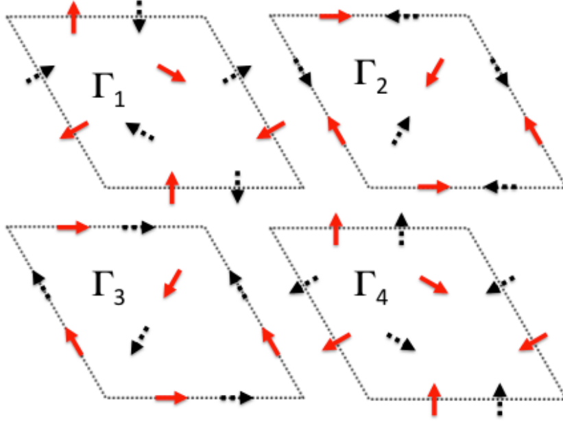
FIGURE 6.5 – Tableau des quatre représentations irréductibles de dimension 1 du groupe d'espace P6_3cm pour un vecteur de propagation k = (0 \ 0 \ 1/2) . Les flèches rouges représentent les composantes de Fourier de l'aimantation réelles, les flèches noires pointillées les composantes imaginaires. Les plans z entier ont un moment magnétique ordonné, les plans demi-entier restent paramagnétiques.
