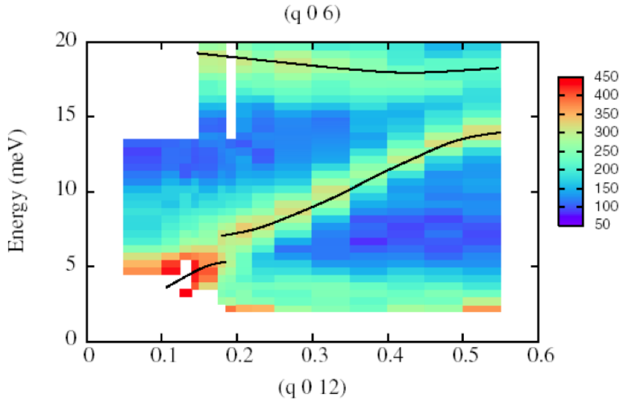
FIGURE 1.18 – Carte en fausses couleurs de la dispersion du phonon acoustique dans la direction Q = (0 0 6) pour le composé YMnO_3 . L'hybridation avec les excitations de spins est marquée par l'ouverture d'un gap dans la dispersion du phonon acoustique en dessous de T_N . Les lignes noires correspondent à l'affinement de la position des excitations à partir des spectres obtenus sur spectromètre 3-axes.
