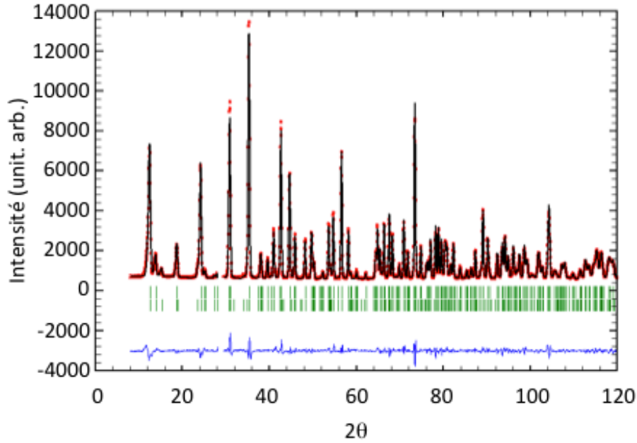
FIGURE 4.8 – Diffractogramme neutron expérimental (rouge) et calculé (noir) du composé \text{ScMnO}_3 à T = 2\text{K} .
