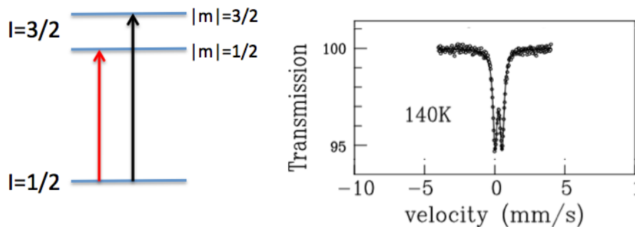
FIGURE 2.10 – Exemple de mesure Mössbauer sur un atome de ^{57}\text{Fe} . Deux pics d'absorption sont observés caractéristiques de la levée de dégénérescence des états l = 3/2 par interaction quadrupolaire électrique.
