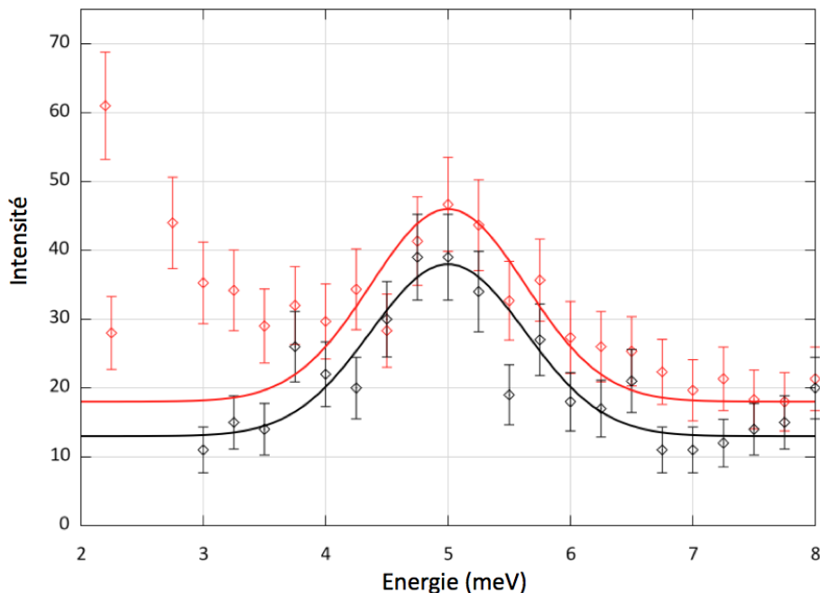
FIGURE 8.5 – Mesure de l'intensité diffusée dans le canal NSF en Q = (0\ 0\ 6) pour k_f = 2.662\ \text{\AA}^{-1} (rouge) et k_f = 1.97\ \text{\AA}^{-1} (noir). Le changement de longueur d'onde n'affecte pas la position en énergie de l'excitation observée éliminant une origine due à des processus harmoniques.
