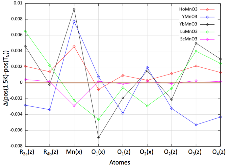
FIGURE 5.3 – Déplacements atomiques observés dans les différents composés entre T_N et T = 1.5 - 3 K . En abscisse les différents atomes sont repertoriés, en ordonné est reporté la valeur \text{pos}(1.5 K) - \text{pos}(T_N) .
