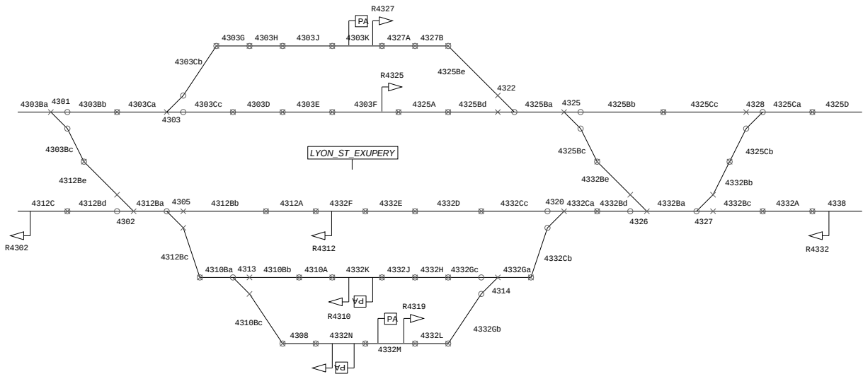
FIGURE 5.1 – Représentation métier de la gare TGV Lyon St Exupéry
