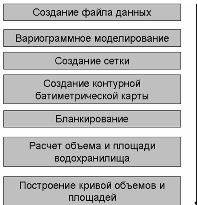
Рис.4.6. Этапы расчета объемов в программе SURFER Figure 4.6. Steps for calculation of reservoir volumes by SURFER
