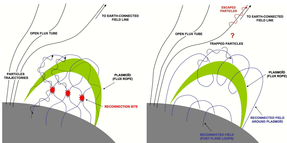
FIG. 2.4: Gauche : Suite à la montée du plasmöïde, les arcades magnétiques le surplombant se "pincent" en dessous, entraînant la reconnexion des lignes de champ ; Droite : Après avoir reconnecté, les lignes de champ forment deux types différents de boucles : les boucles post-éruptives et les boucles enveloppant le plasmöïde.
