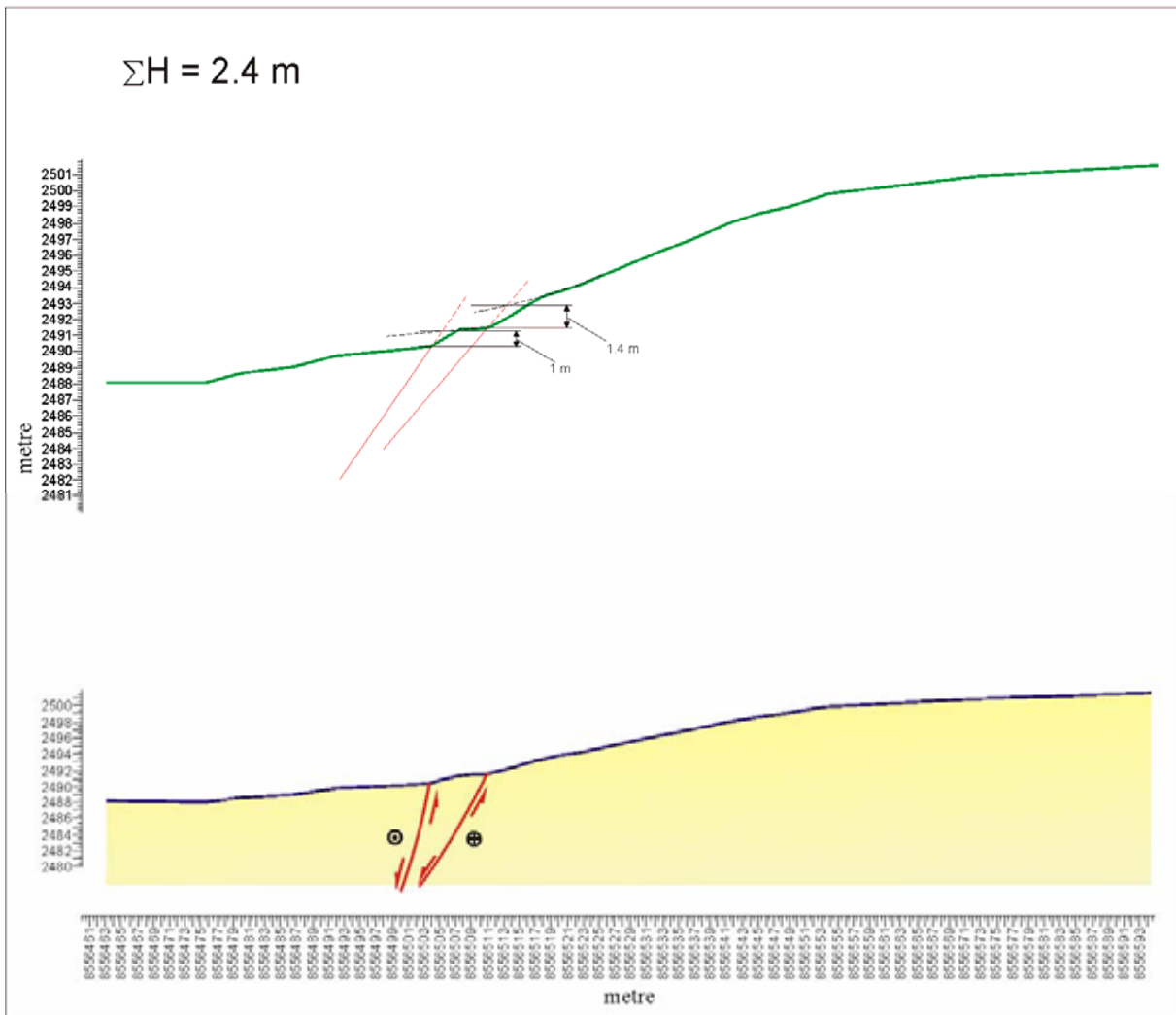
Profil 29-29'
