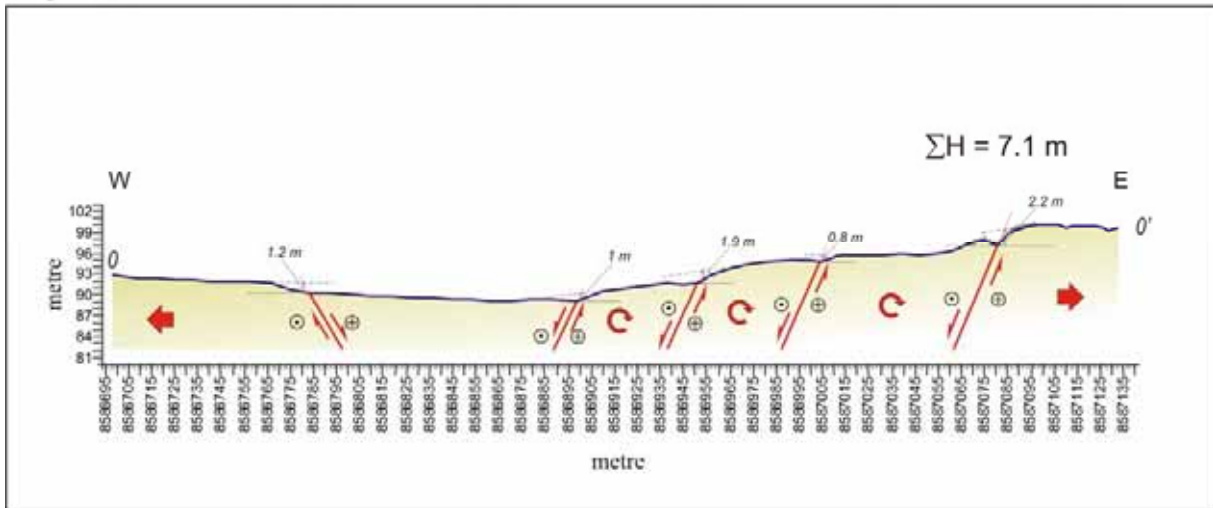
Profil 0-0'
