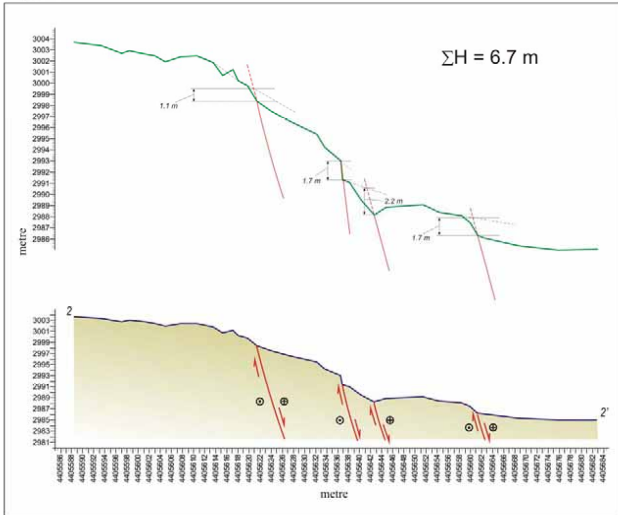
Profil 2-2'
