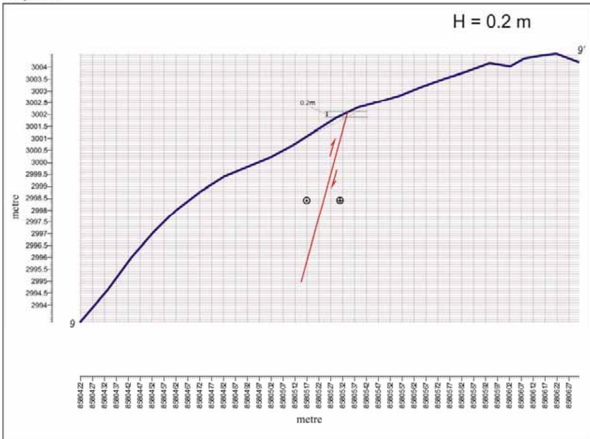
Profil 9-9'
