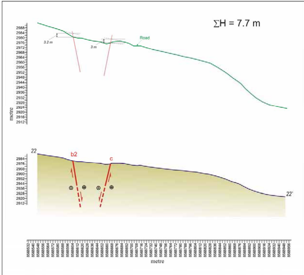
Profil 22-22'
