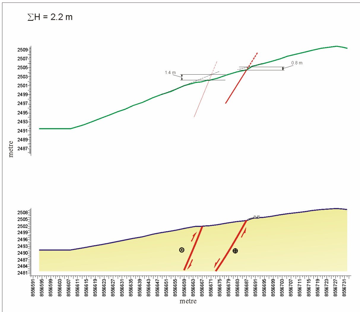
Profil 28-28'
