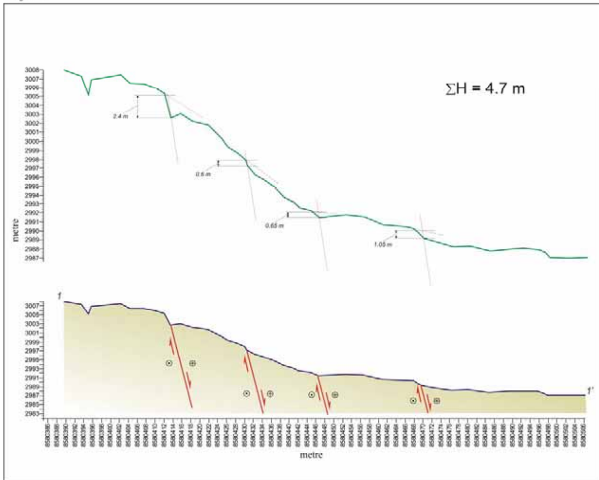
Profil 1-1'
