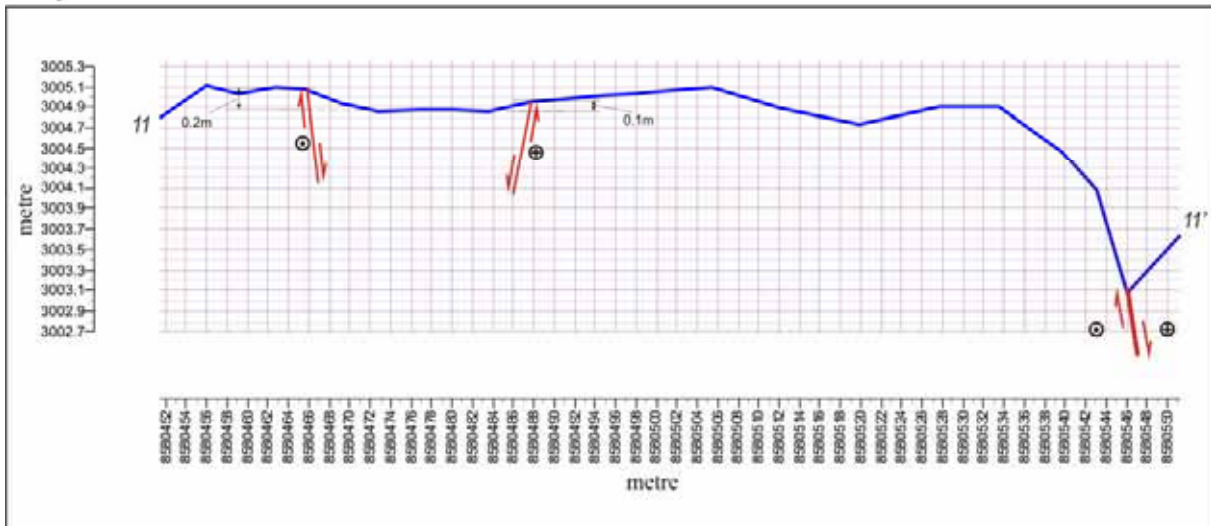
Profil 11-11'
