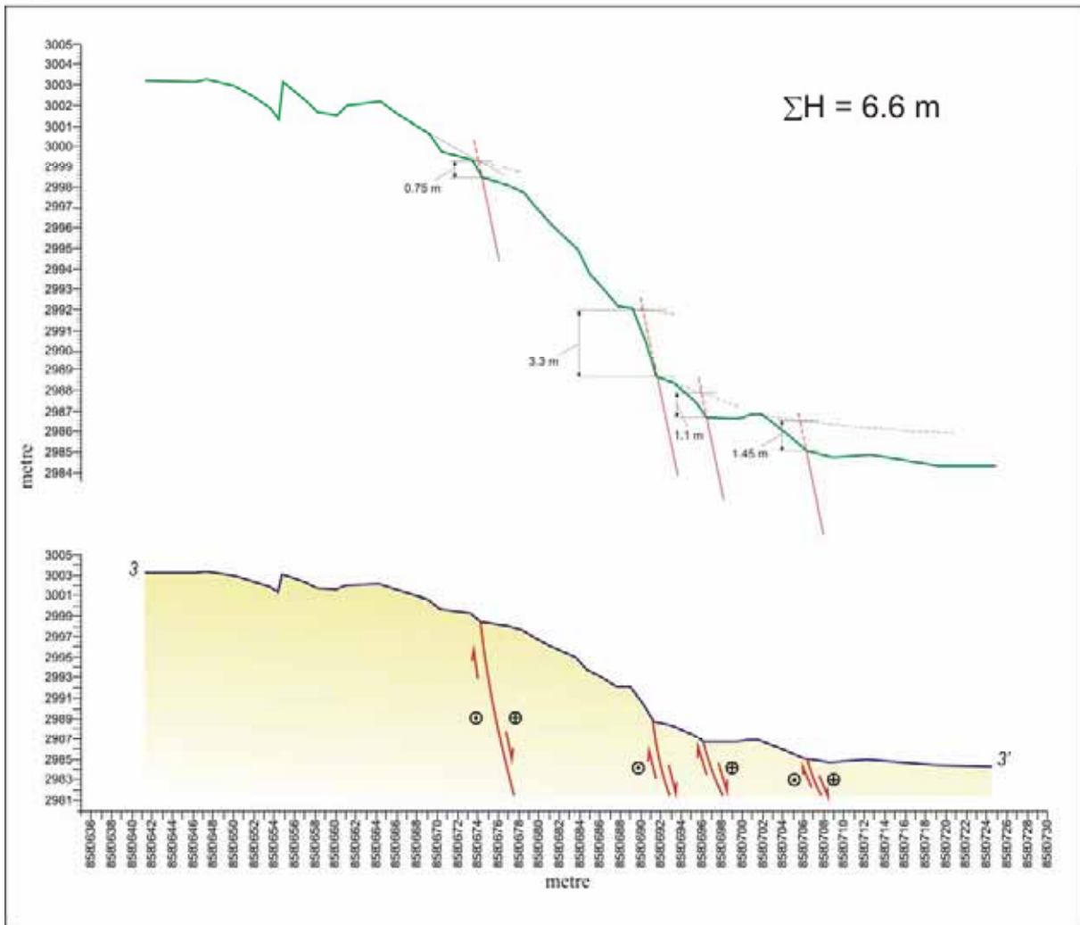
Profil 3-3'
