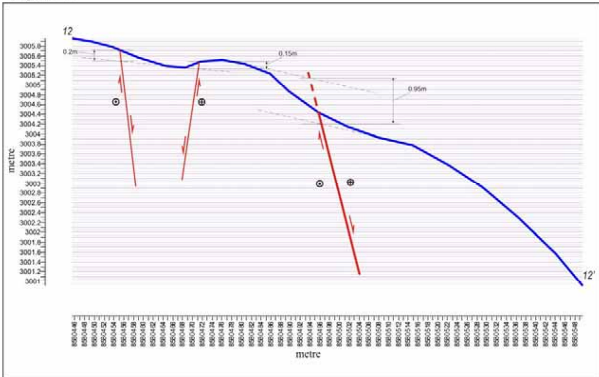
Profil 12-12'
