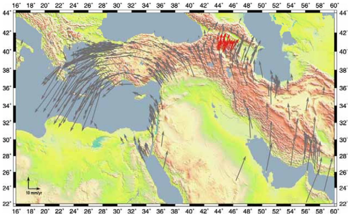
Figure II - 16 : Champ de vitesse dans le référentiel Eurasie de la zone de collision entre les plaques Arabe et Eurasienne. Les vecteurs gris sont de McClusky et al. (2000) et de Vernant, (2003). Les vecteurs rouges sont les résultats de cette étude.
