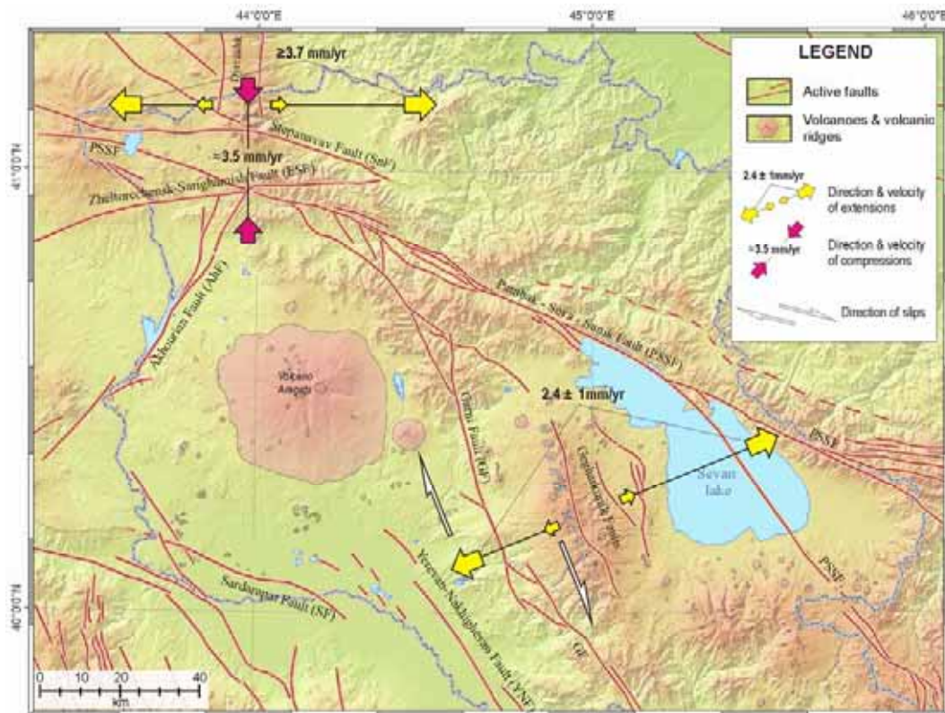
Figure II - 24 : Déformations horizontales estimés dans résultat de l'analyse de champ de vitesses de GPS le long des profils A1–A2, B1–B2 et C1–C2.
