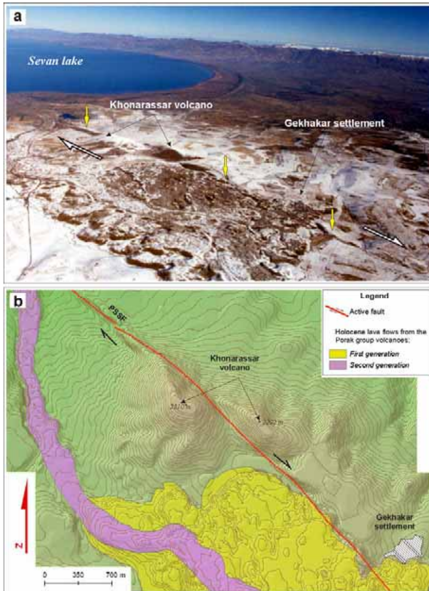
Figure III - 6 : Le volcan de Khonarassar coupé par la faille de Pambak-Sevan-Suynik (PSSF) est décalé en dextre: a- la photo fait de l'hélicoptère par A. Avanesyan. Les flèches jaunes indiquent la trace de la faille PSSF; b- le MNT (Modèle Numérique de Terrain) du territoire de la partie de Khonarassar-Porak de la faille PSSF avec une résolution de 5 mètre/pixel.
