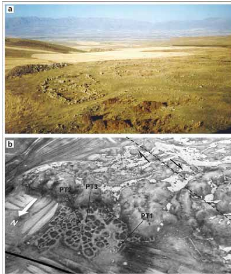
Figure III - 8 : La cité de Gekhakar: a- la photo d'une partie de cité (Philip, H. & Karakhanyan, A., 1999); b- la combinaison du modèle numérique tridimensionnel de la cité de Gekhakar avec une image aérienne. Les flèches montrent l'emplacement des fouilles.
