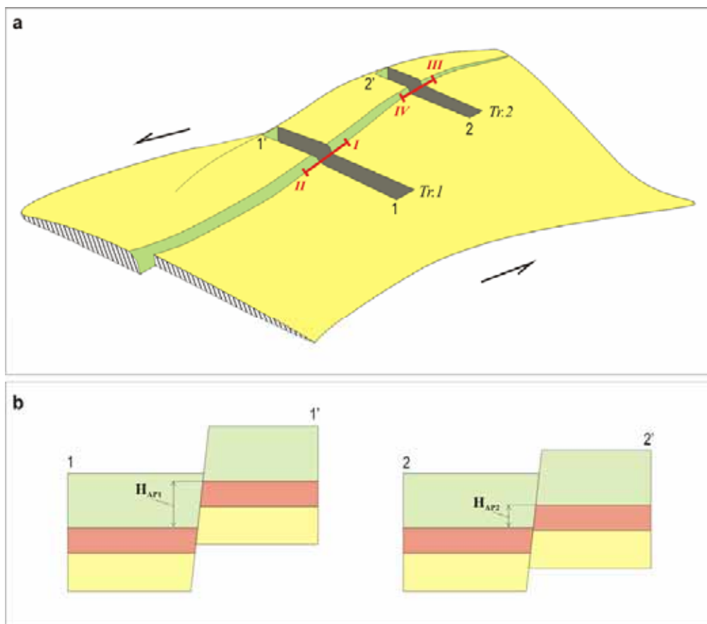
Figure III - 39 : a –modèle 3D de la colline déplacé par une faille et disposition des tranchées Tr.1 et Tr.2; b – logues des tranchées Tr.1 et Tr.2.
