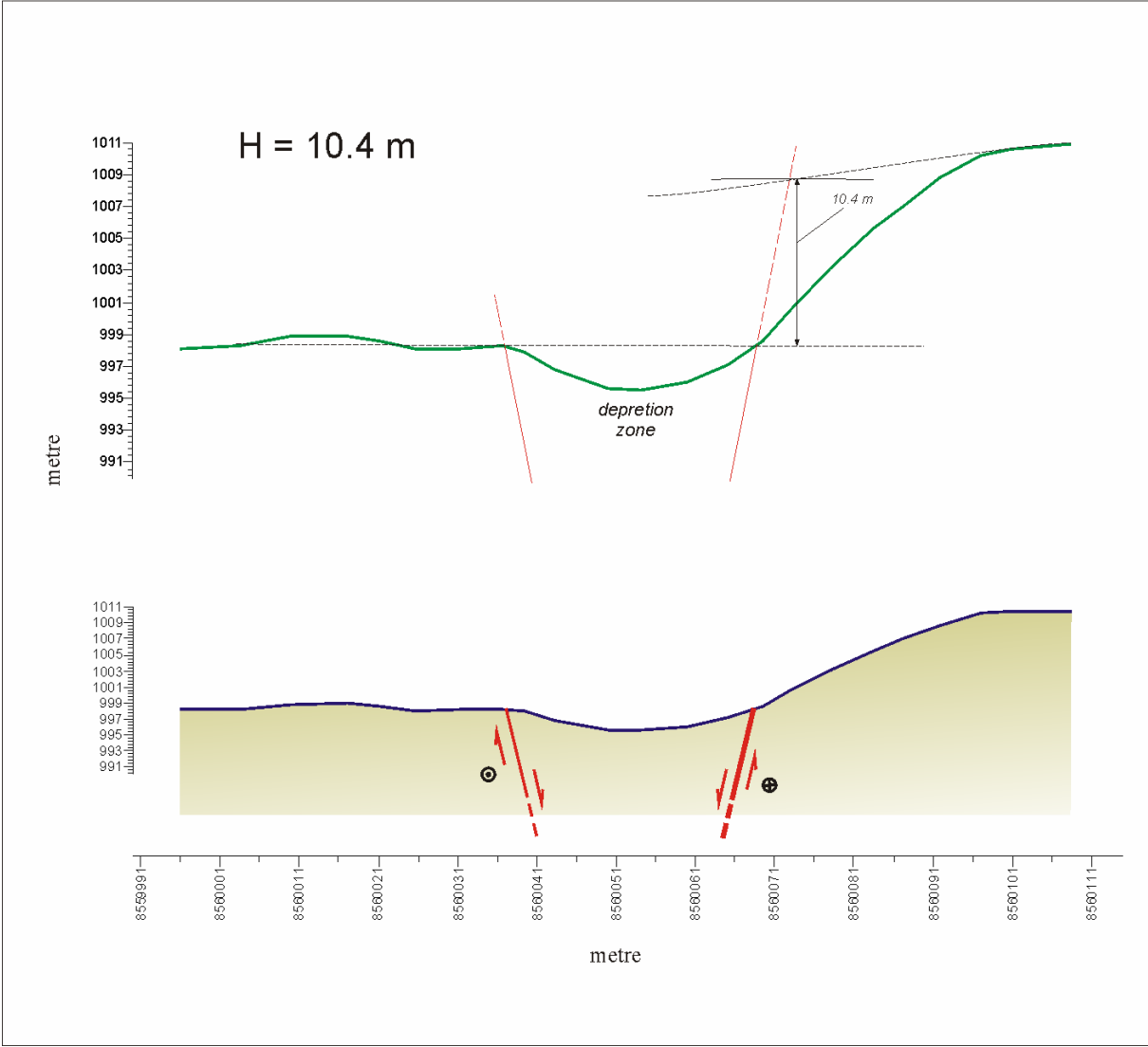
Profil 26-26'
