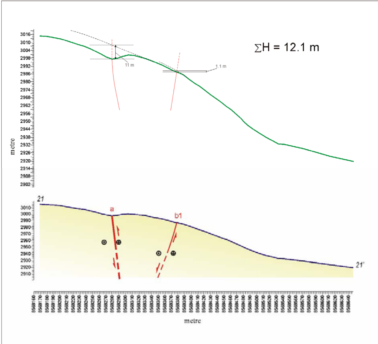
Profil 21-21'
