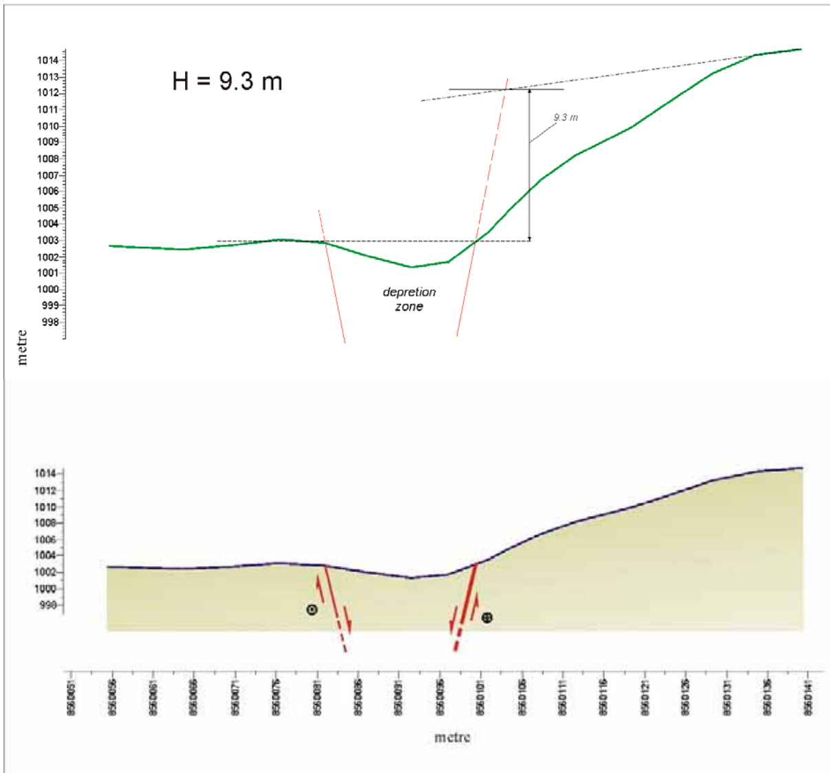
Profil 27-27'
