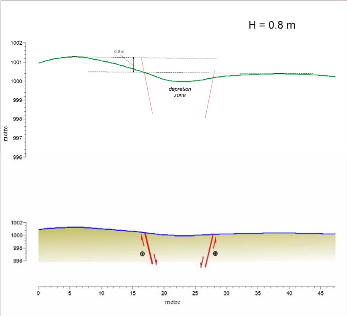
Profil 30-30'
