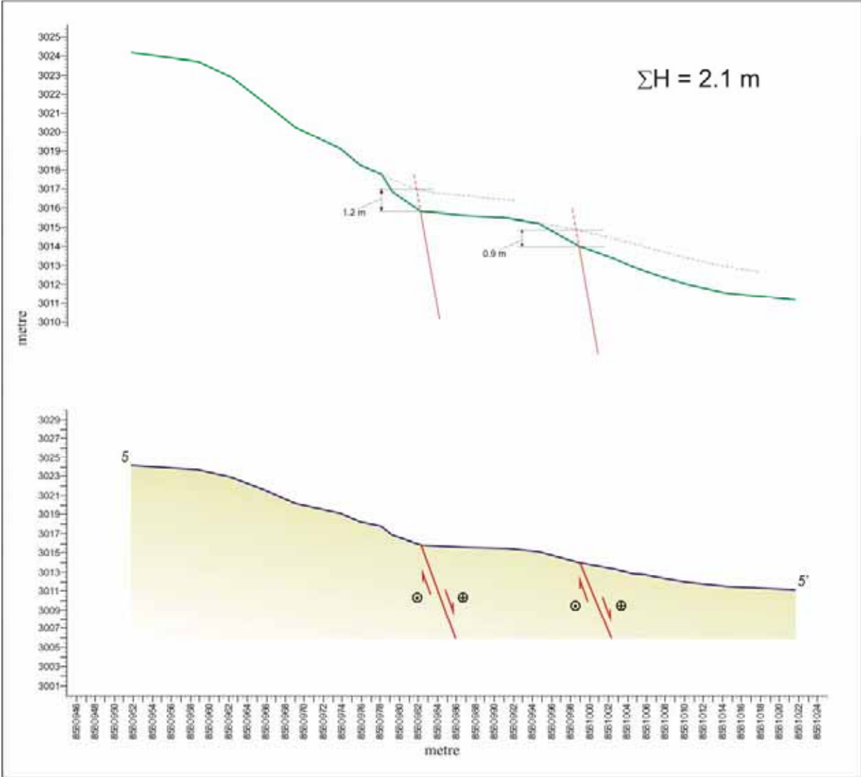
Profil 5-5'
