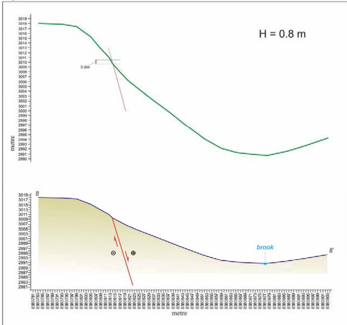
Profil 8-8'
