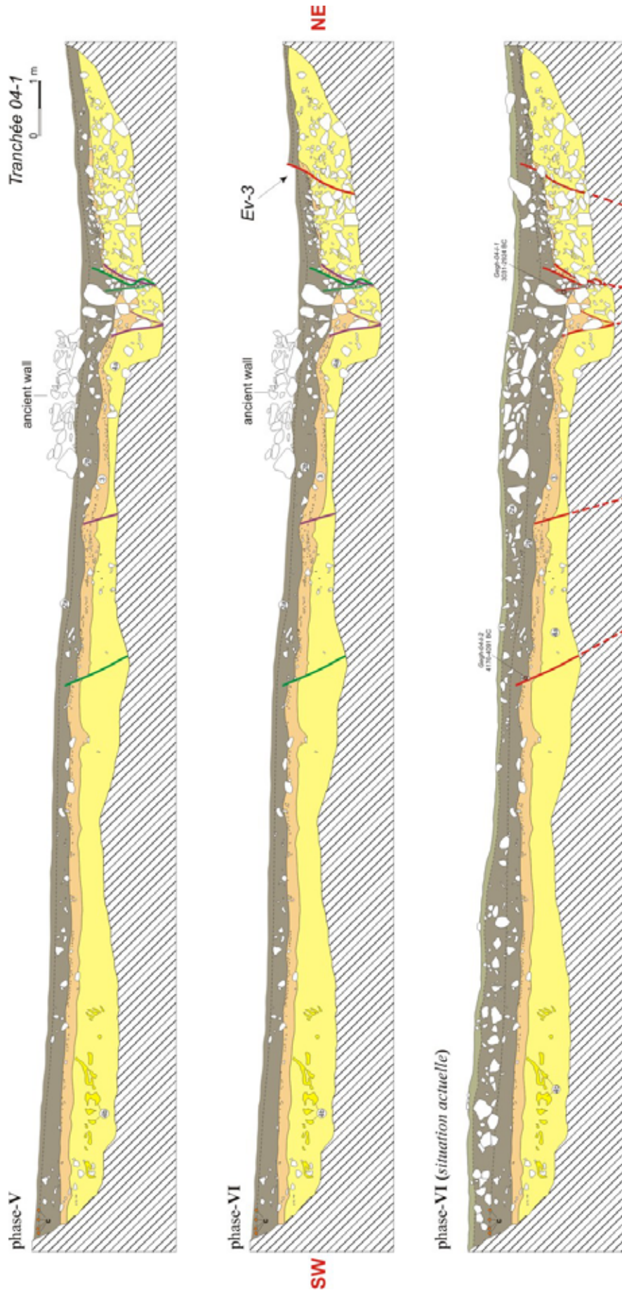
Figure III - 34 : Log de la tranchée paléosismologique 04-1. Scénario de l'interprétation des paléo séismes enregistrés sur le segment d'Artanish-Tskhuk de la faille de Pambak-Sevan-Suyunik.
