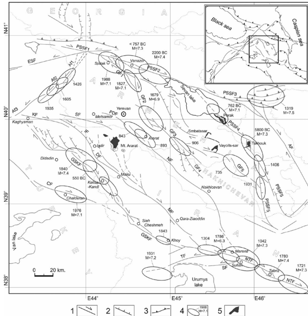
Figure I - 4 : Failles actives de l'Arménie, de l'Est de Turquie, du Nord-ouest de l'Iran. 1- failles décrochantes; 2- failles normales; 3- failles chevauchantes 4- épacentres des séismes principales; 5- éruptions volcaniques d'âge holocène. (d'après Karakhanian, et al., 2004).
