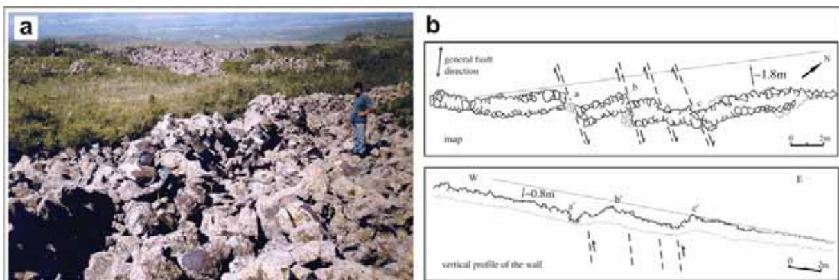
Figure III - 9 : a- le mur de fortification déplacé en dextre par la faille. b- la carte et profile vertical réalisés par A. Avagyan (2001).
