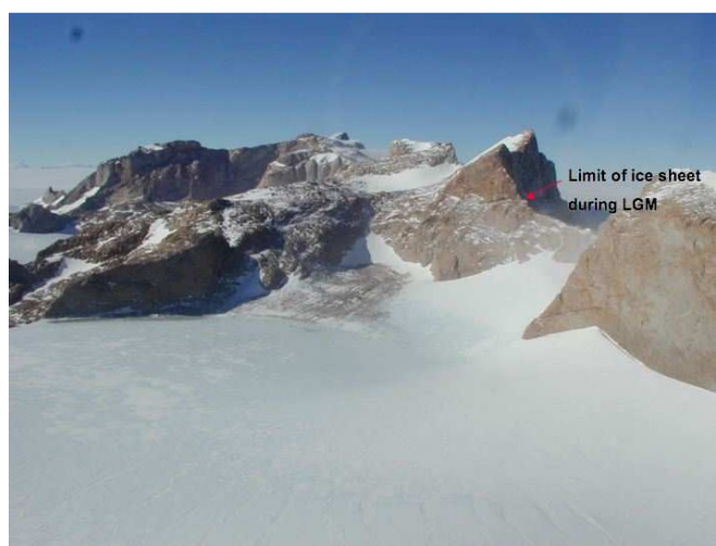
Figure 10 : empreintes géologiques relevées dans la zone des Frontier Moutains de l'altitude de la calotte glaciaire antarctique durant le DMG
