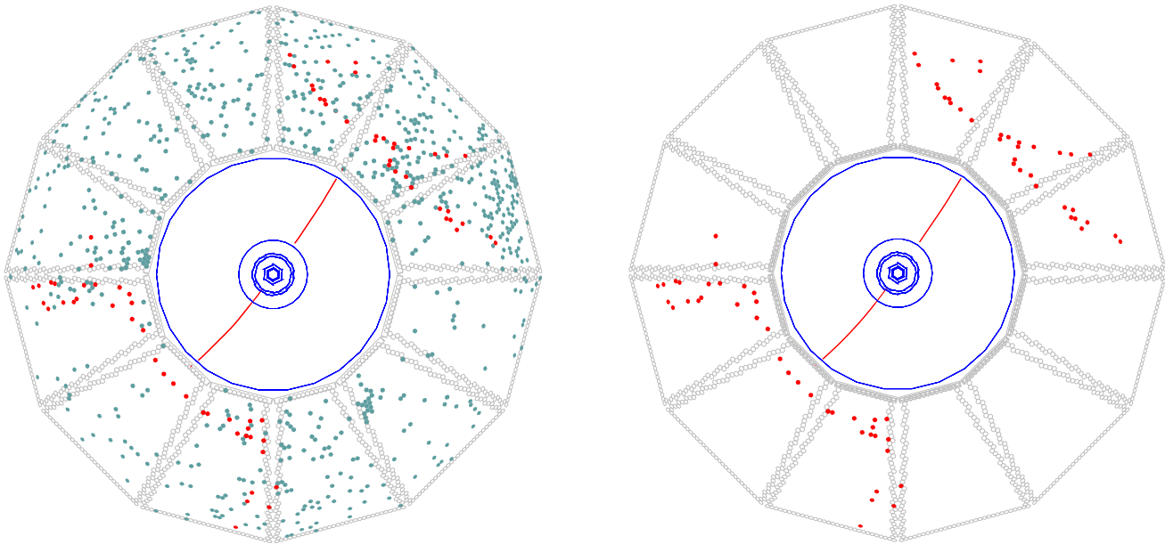
FIG. 1.6 – Un événement e^+e^- \rightarrow \mu^+\mu^- dans le plan transverse (x,y) . Les trajectoires sont reconstruites par le système SVT-DCH. Les points correspondent aux photo-multipliateurs touchés dans une fenêtre en temps de \pm 300 ns par rapport au temps de déclenchement de l'acquisition. A gauche : l'ensemble des photo-multipliateurs touchés est représenté. A droite : sélection des photo-multipliateurs avec un signal à \pm 8 ns du temps d'arrivée attendu. On voit clairement les arcs, intersection du cône Cherenkov avec la surface de détection. La réflexion des photons sur les surfaces des barres, les miroirs et les prismes crée plusieurs images symétriques.
