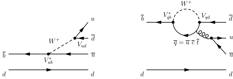
FIG. 2.6 – Diagrammes de la désintégration B^0 \rightarrow \pi^+ \pi^- . Droite : en arbre ; gauche : pingouin gluonique. Le diagramme pingouin électrofaible est obtenu en remplaçant le gluon émettant la paire u\bar{u} par un photon ou un Z^0 .
