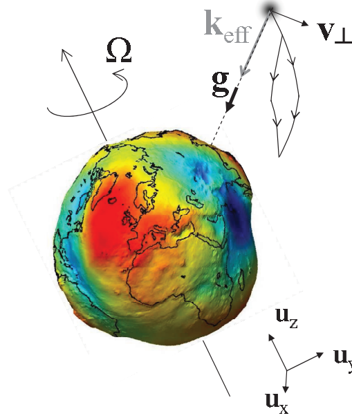
FIG. 3.10 – Principe de l'altération de la mesure de g par l'accélération de Coriolis subie par un atome de vitesse transverse non nulle sur l'axe Est - Ouest.
