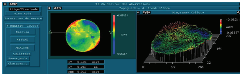
FIG. 6.6 – Front d'onde du miroir de rétro-réflexion mesuré au ZYGO.
