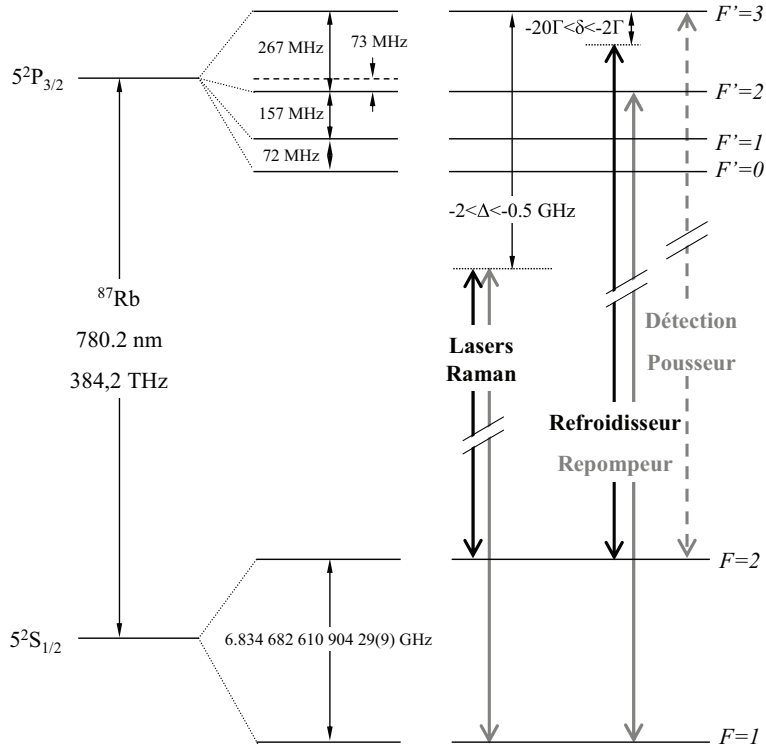
FIG. 3.4 – Structure atomique de l’atome de ^{87}\text{Rb} et fréquences optiques choisies pour le refroidissement et les Raman.
