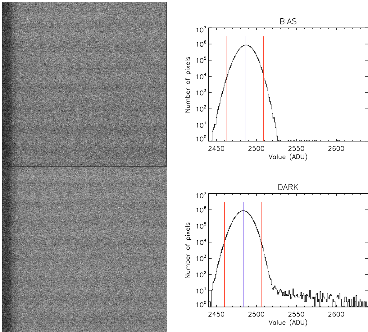
FIG. 5.4 – Exemple de bias (haut) et de dark (bas) accompagnés de leur histogramme. La médiane est indiquée en bleu et les limites contenant 99 % des pixels en rouge. Les pixels chauds constituent la queue de l’histogramme du dark.
