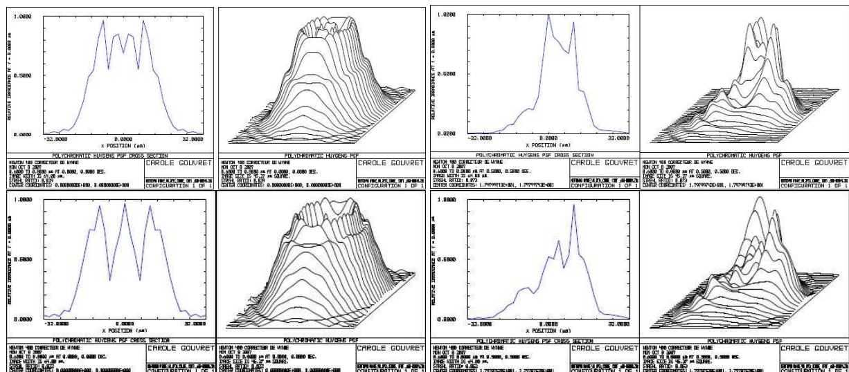
FIG. 6.12 – Vue en coupe et en 3 dimensions des PSF défocalisées à 3 px (haut) et 4 px (bas), au centre (gauche) et en bord de champ (droite).
