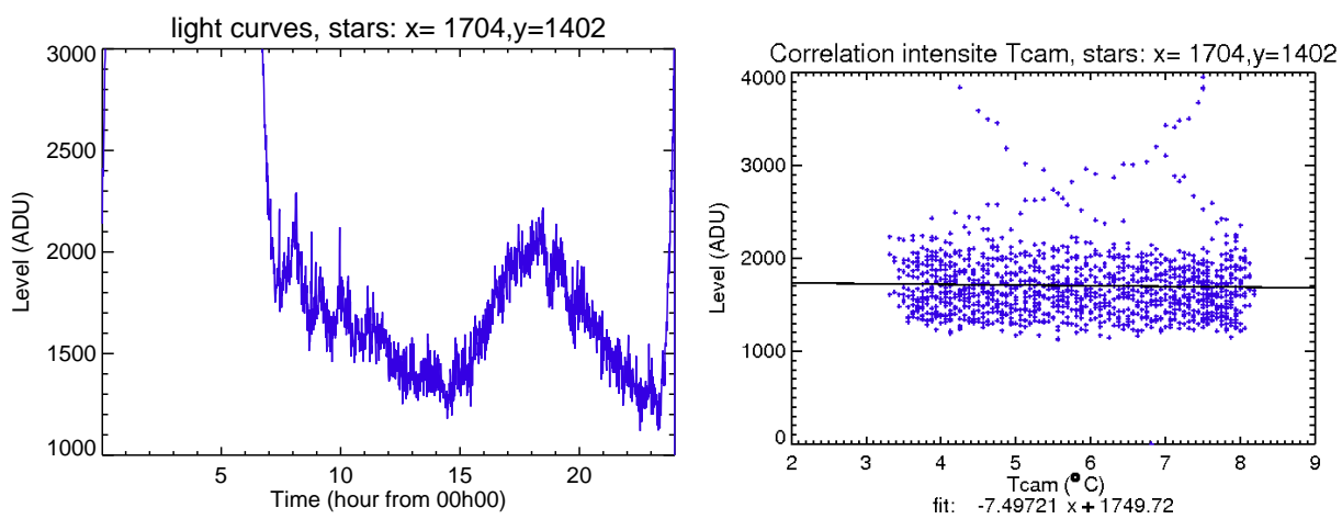
FIG. 5.10 – Courbes de lumière sur une zone de 6 \times 6 px sans étoiles (gauche), et corrélation avec la température de l’électronique de la caméra (droite), après correction de l’effet des variations de cette température. On diminue largement les oscillations, avec un résidu de -7.5 \text{ ADU}/^{\circ}\text{C} (soit 0.2 \text{ ADU}/^{\circ}\text{C}/\text{px} ).
