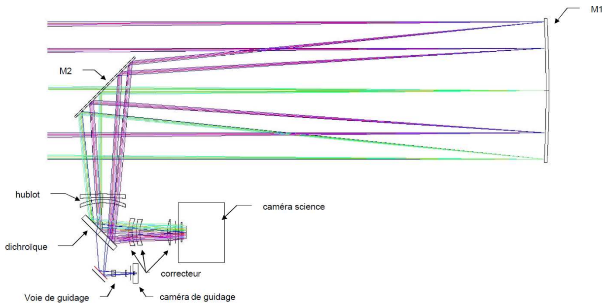
FIG. 6.1 – Schéma optique du télescope ASTEP400.
