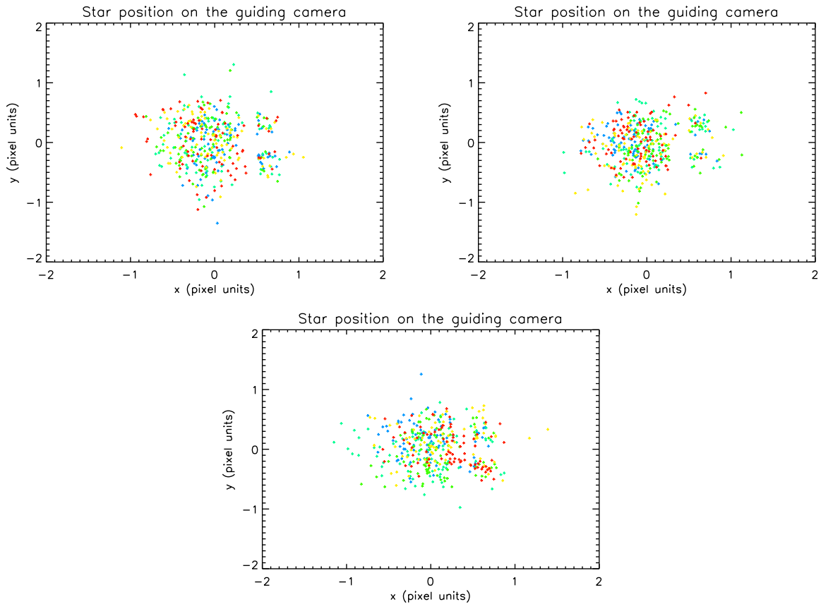
FIG. 6.22 – Position du centre de l'étoile guide sur des images simulées par SimPhot pour des PSF de différentes focalisations : -100 (bleu), -50 (turquoise), 0 (vert), +50 (jaune) et +100 (rouge) \mu\text{m} , pour une étoile de magnitude 8 (haut gauche), 10 (haut droite) et 12 (bas), et pour des déplacements standard du télescope.
