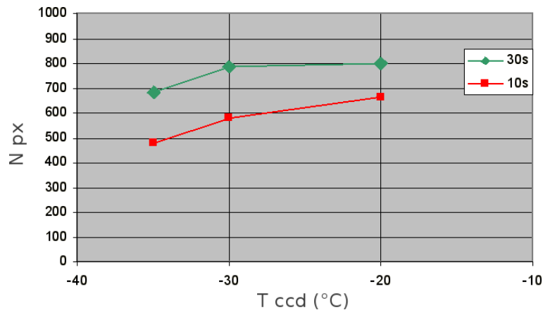
FIG. 3.15 – Nombre de pixels chauds dans le CCD ASTEP Sud pour des températures de -35 , -30 et -20^{\circ}\text{C} , et des temps de pose de 10 s (rouge) et 30 s (vert).
