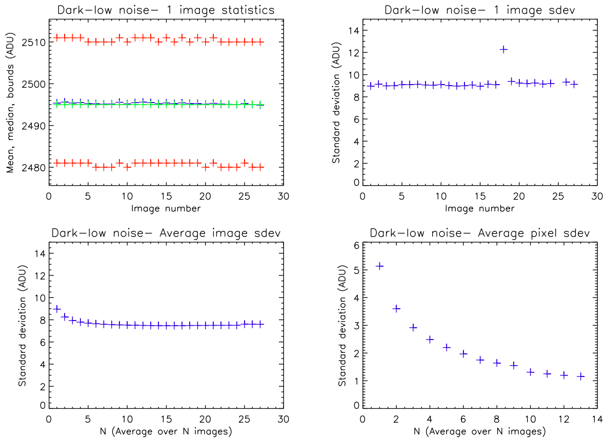
FIG. 3.9 – Statistiques sur les images de dark de 30 s prises en lecture lente pour la caméra ASTEP 400. Moyenne (bleu), médiane (vert), et intervalle contenant 99 % des pixels (rouge), pour chacune des \sim 30 images (haut gauche), déviation standard pour chacune des \sim 30 images (haut droite), déviation standard d’une image moyenne faite à partir de N images (bas gauche), et déviation standard par pixel sur plusieurs images moyennes de N images (bas droite).
