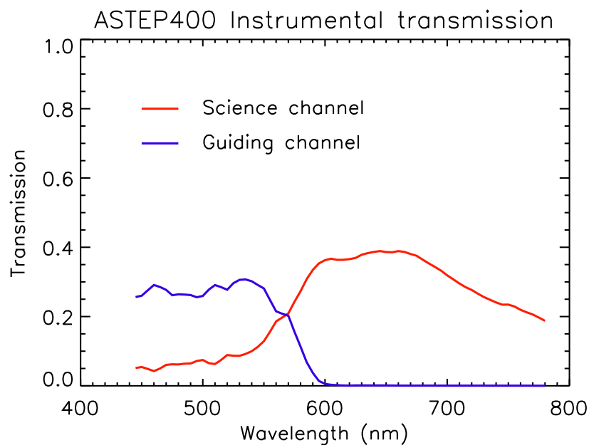
FIG. 6.29 – Transmission instrumentale totale du télescope ASTEP400, sur les voies science (rouge) et guidage (bleu).
