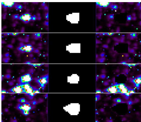
FIG. 2.7 – Exemples d'ouvertures photométriques pour 4 étoiles observées par CoRoT. Gauche : imagerie centrées sur la cible. Les PSF CoRoT sont volontairement asymétriques. Milieu : Masque utilisé pour chacune des cibles, qui prend en compte la forme de la PSF et l'environnement stellaire (en excluant ou incluant des étoiles voisines). Droite : champ en dehors du masque. Image tirée de Auvergne et al. [2009].
