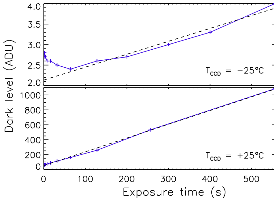
FIG. 3.12 – Valeur moyenne du dark en fonction du temps de pose pour différentes températures du CCD, après soustraction de la valeur du bias, pour la caméra ASTEP400.
