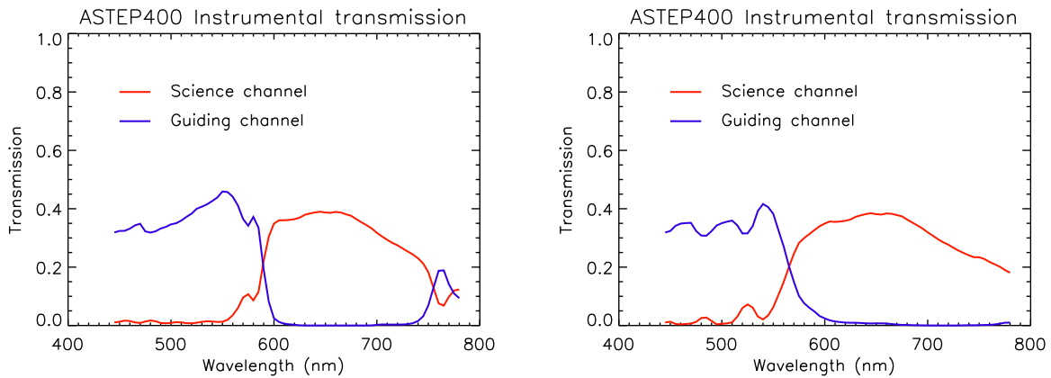
FIG. 6.28 – Transmission instrumentale totale du télescope, avec la lame dichroïque pas chère proposée par l'entreprise SEOP (gauche), et avec la lame dichroïque chère proposée par l'entreprise Fichou (droite), sur les voies science (rouge) et guidage (bleu).
