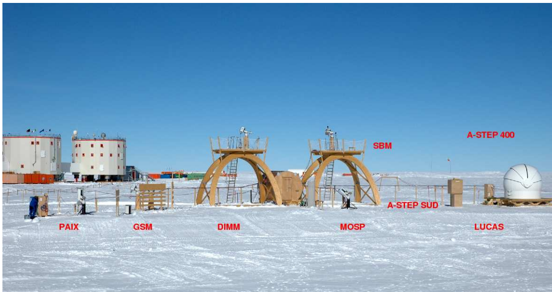
FIG. 1.12 – La station Concordia et la plateforme Astroconcordia, espace dédié aux instruments d'astronomie. Les instruments sont soit au niveau du sol, soit sur une structure en bois de 8 m de haut. Un abri en bois relié à la station contient les ordinateurs et les appareils permettant de faire fonctionner les instruments.
