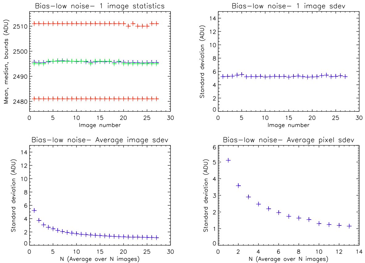
FIG. 3.8 – Statistiques sur les images de bias prises en lecture lente pour la caméra ASTEP 400. Moyenne (bleu), médiane (vert), et intervalle contenant 99 % des pixels (rouge), pour chacune des \sim 30 images (haut gauche), déviation standard pour chacune des \sim 30 images (haut droite), déviation standard d’une image moyenne faite à partir de N images (bas gauche), et déviation standard par pixel sur plusieurs images moyennes de N images (bas droite).
