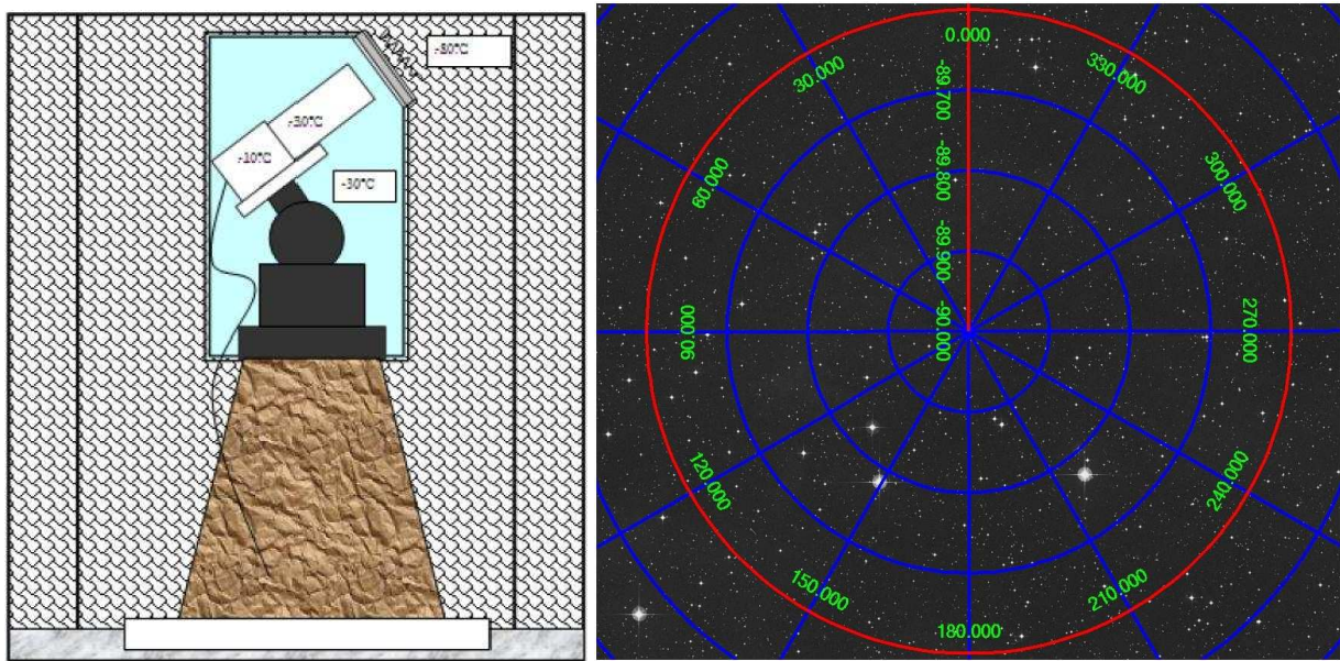
FIG. 4.1 – Principe d'ASTEP Sud : une lunette de 10 cm équipée d'une caméra CCD dans une enceinte thermalisée (gauche) observe en continu le champ centré sur le pôle sud céleste (droite).
