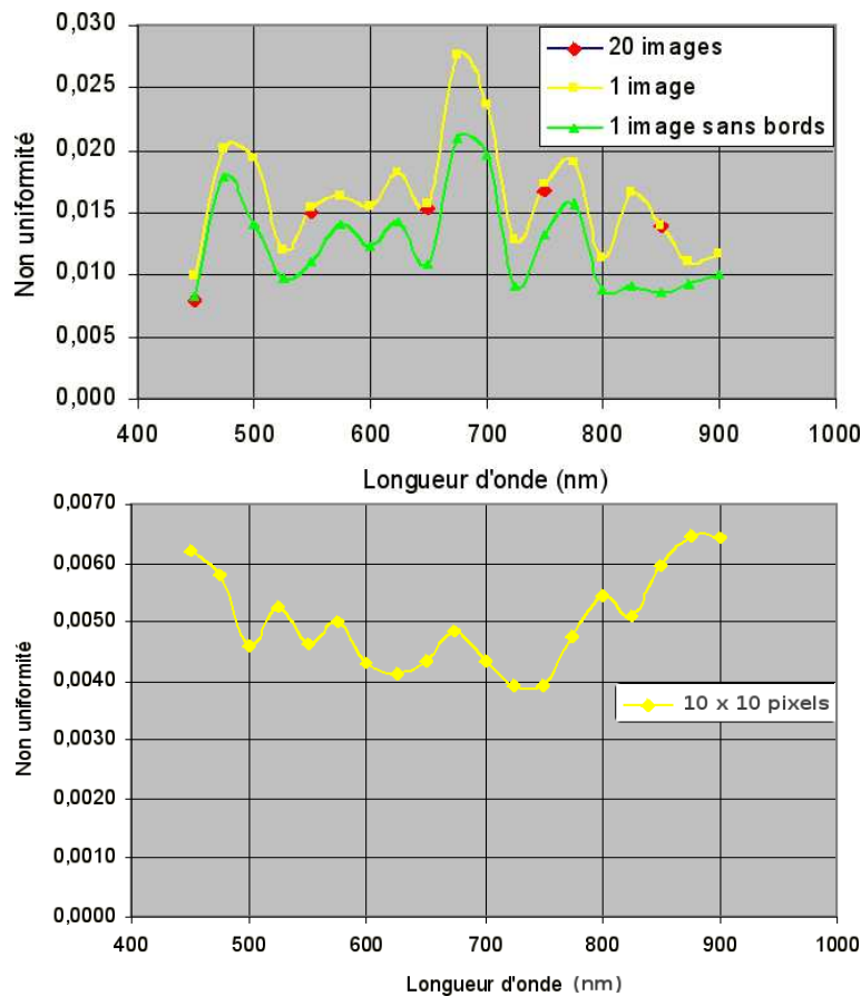
FIG. 3.16 – Non-uniformités globales (haut), sur une image (bas), sur une moyenne de 20 images (rouge) et sur 1 image en excluant les bords (vert), puis locales (droite), sur une région de 10 \times 10 pixels au centre du CCD, pour le CCD ASTEP Sud.
