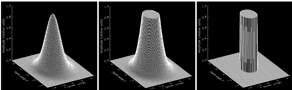
FIG. 2.17 – L'influence de la forme des PSF est étudiée à l'aide de 3 cas extrêmes : une PSF gaussienne (gauche), une PSF top-hat (centre) et une PSF cylindrique (droite).
