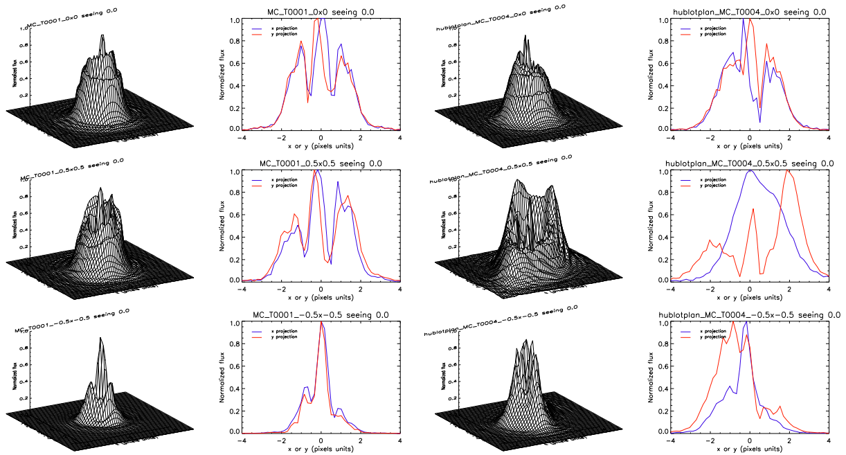
FIG. 6.14 – PSF issues des simulations de tolérancements classiques avec un hublot ménisque (gauche) et plan (droite), en 3 dimensions et en coupe selon x (bleu) et y (rouge), au centre du champ (haut), dans la diagonale à 0.5^\circ \times 0.5^\circ (milieu) et à -0.5^\circ \times -0.5^\circ (bas).
