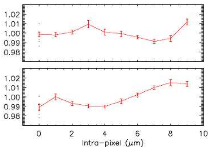
FIG. 2.5 – Variations de transmission au sein d'un pixel, mesurées par Karoff et al. [2006] sur un CCD E2V 47-20. Les variations sont de l'ordre de 1 %.
