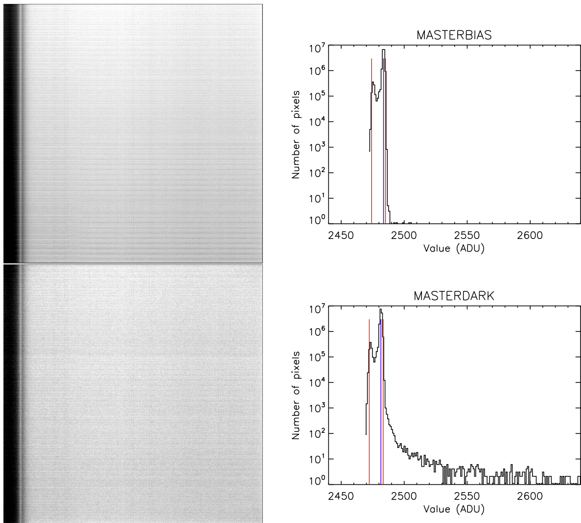
FIG. 5.5 – Masterbias (haut) et masterdark (bas) de la journée du 12 juillet 2008, accompagnés de leur histogramme. La médiane est indiquée en bleu et les limites contenant 99 % des pixels en rouge.
