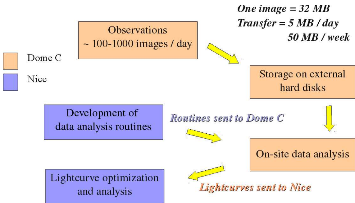
FIG. 7.17 – Schéma simplifié de la gestion des données et de leur traitement pour la campagne 2010.
