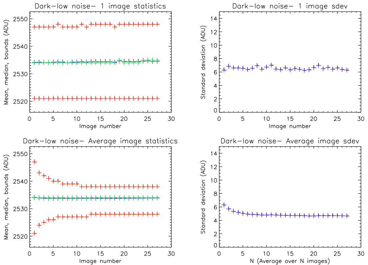
FIG. 3.13 – Statistiques sur les images de dark de 30 s prises en lecture rapide pour la caméra ASTEP Sud. Moyenne (bleu), médiane (vert), et intervalle contenant 99 % des pixels (rouge), pour chacune des \sim 30 images (haut gauche), déviation standard pour chacune des \sim 30 images (haut droite), déviation standard d’une image moyenne faite à partir de N images (bas gauche), et déviation standard par pixel sur plusieurs images moyennes de N images (bas droite).
