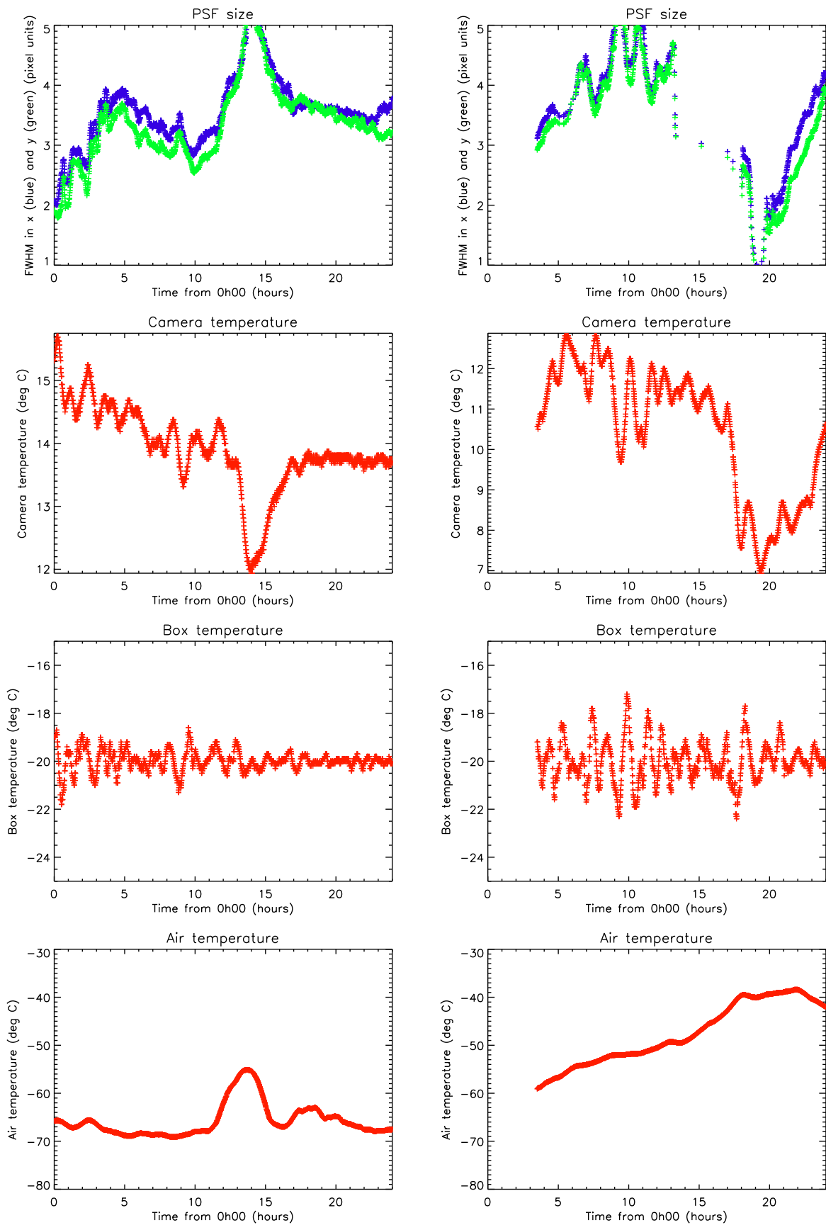
FIG. 4.29 – Comparaison de la taille des PSF selon les directions x (bleu) et y (vert) sur le CCD, avec les températures de l'électronique de la caméra, de l'enceinte et extérieure (rouge), pour les journées du 2 juin 2009 (gauche) et du 1 er juillet 2009 (droite). La taille des PSF est soit corrélée, soit anti-corrélée avec les températures de la caméra et extérieure. Les petites oscillations sont corrélées avec la température de l'enceinte.
