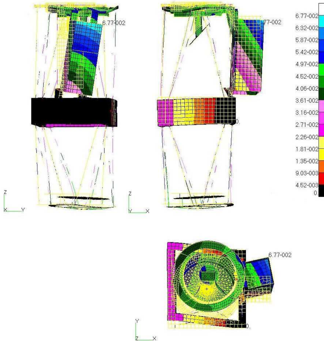
FIG. 6.5 – Déformations mécaniques dues au poids pour une orientation du télescope à 45° Nord, vues de côté (haut) et de dessus (bas).
