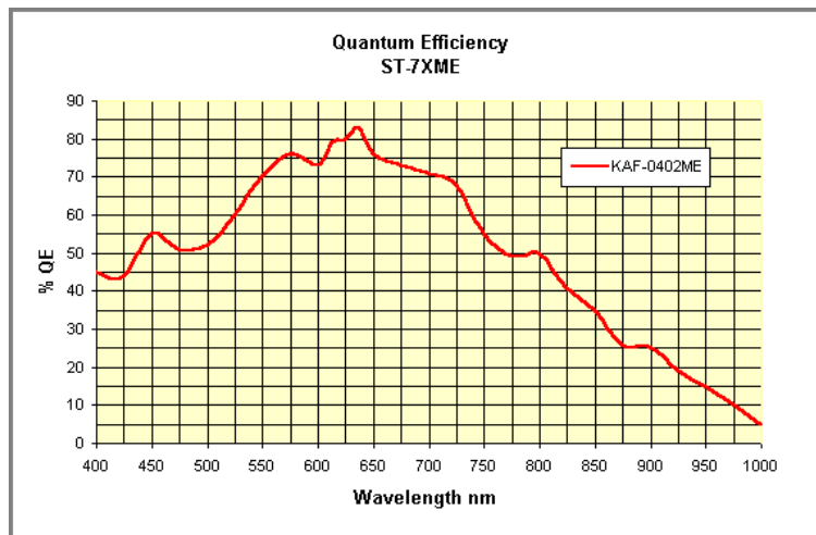
FIG. 6.16 – Courbe d'efficacité quantique de la caméra de guidage SBIG ST402. Le CCD est sensible dans tout le domaine visible ; on n'utilisera que la partie bleue.
