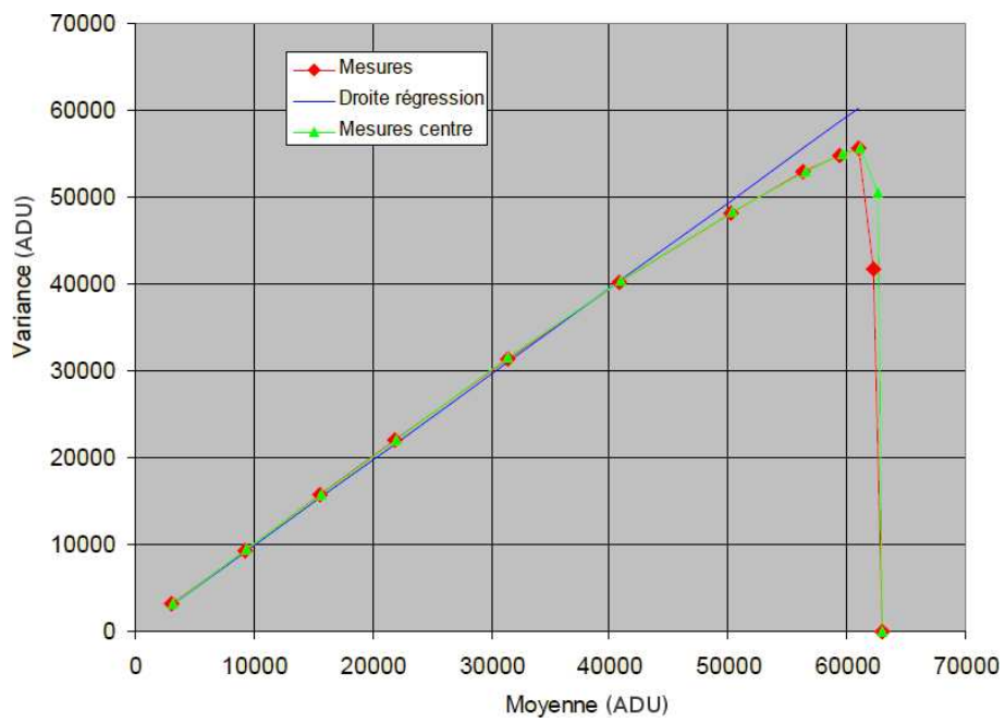
FIG. 3.6 – Mesure du gain pour la caméra ASTEP Sud, à partir de l’image complète (rouge), et de la partie de 1000 \times 1000 px au centre (vert). Les résultats sont identiques. Un ajustement linéaire (bleu) permet de mesurer le gain et la limite de linéarité.
