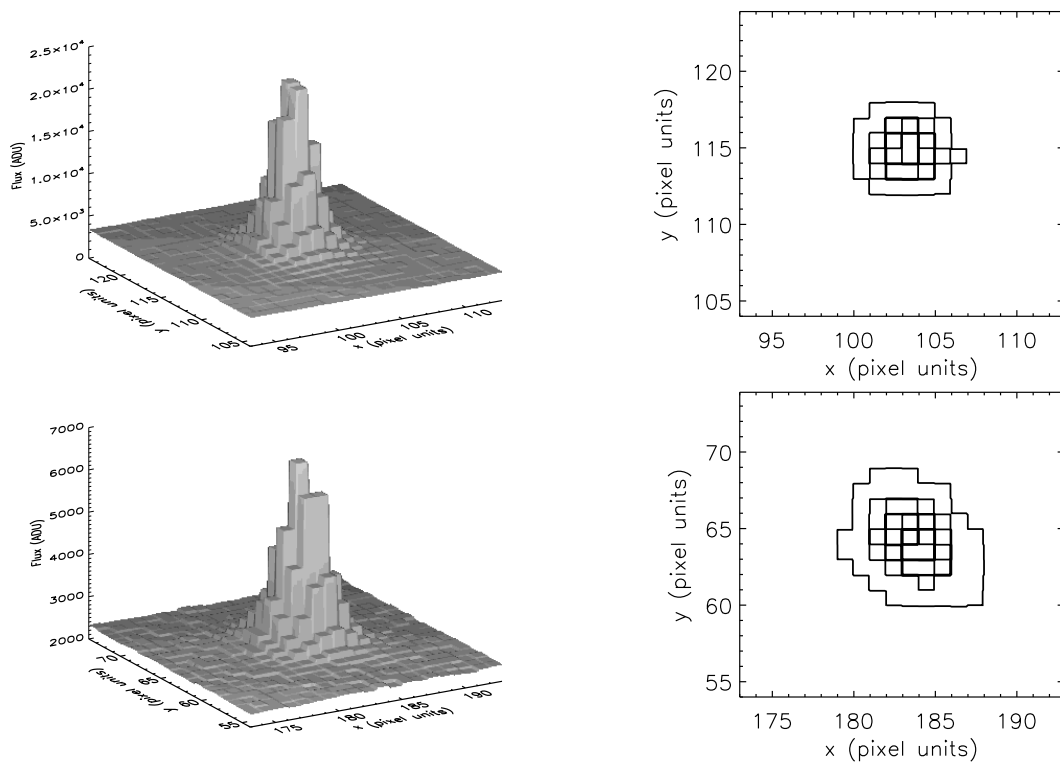
FIG. 7.11 – Exemples de PSF obtenues à l’issue des premiers réglages optiques d’ASTEP400 à Concordia, le 28 novembre 2009, au centre du champ (haut) et dans le coin en bas à gauche du champ (bas), en 3D (gauche) et en contours (droite).
