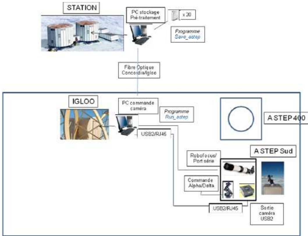
FIG. 4.17 – Schéma de principe de l’installation ASTEP Sud à Concordia. La zone rectangulaire symbolise la plateforme Astroconcordia.
