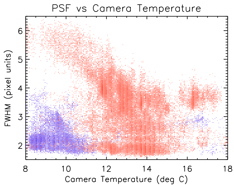
FIG. 4.30 – Corrélation entre la taille des PSF et la température de la caméra pour l'ensemble des données acquises entre le début de la campagne et le 1 er juillet 2009, avant (bleu) et après (rouge) le 21 mai. Après le 21 mai, la PSF est dégradée et la corrélation apparaît clairement.
