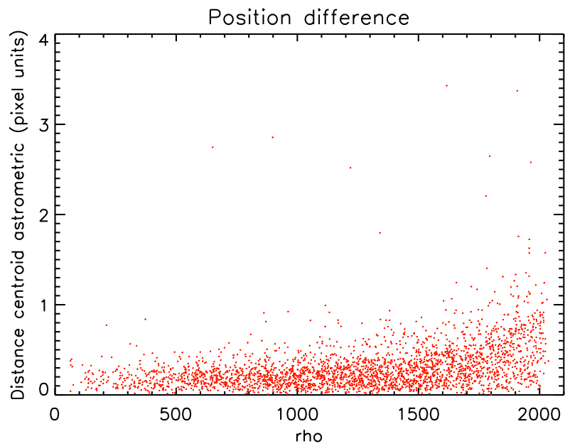
FIG. 5.18 – Différence entre les positions calculées par l’algorithme de reconnaissance de champ après amélioration, et par détermination du centroïde, en fonction de la distance radiale \rho .
