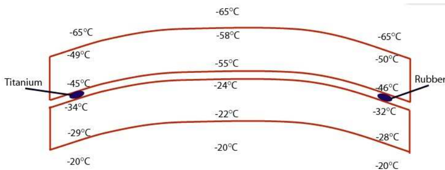
FIG. 6.8 – Température des différentes couches et interfaces du hublot double vitrage, dans la configuration thermique envisagée à Concordia (température extérieure : -65°C, température de l’enceinte : -20°C).
