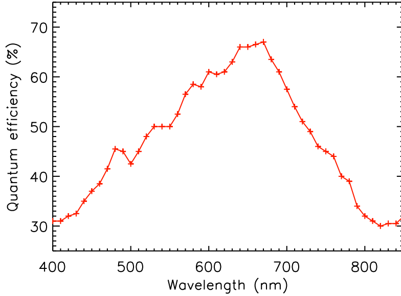
FIG. 3.3 – Courbe d’efficacité quantique du CCD Kodak KAF-16801E. La transmission est équivalente à une bande R élargie. Figure obtenue d’après les données constructeur.
