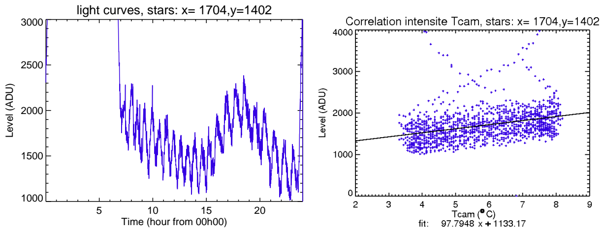
FIG. 5.8 – Courbes de lumière sur une zone de 6 \times 6 px sans étoiles (gauche), et corrélation avec la température de l'électronique de la caméra (droite). On observe des oscillations de 500 ADU, soit \sim 100 \text{ ADU}/^\circ\text{C} , sur une période d'une heure.
