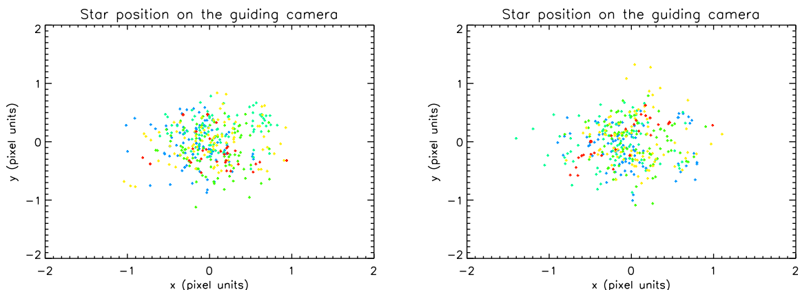
FIG. 6.23 – Position du centre de l'étoile guide sur des images simulées par SimPhot pour des PSF de différentes focalisations : -500 (bleu), -300 (turquoise), 0 (vert), +300 (jaune) et +500 (rouge) \mu\text{m} , pour une étoile de magnitude 8 (gauche) et 10 (droite), et pour des déplacements standard du télescope.
