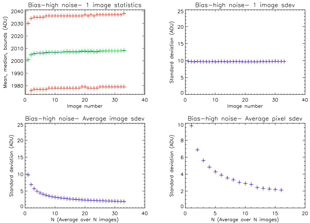
FIG. 3.10 – Statistiques sur les images de bias prises en lecture rapide pour la caméra ASTEP 400. Moyenne (bleu), médiane (vert), et intervalle contenant 99 % des pixels (rouge), pour chacune des \sim 30 images (haut gauche), déviation standard pour chacune des \sim 30 images (haut droite), déviation standard d’une image moyenne faite à partir de N images (bas gauche), et déviation standard par pixel sur plusieurs images moyennes de N images (bas droite).
