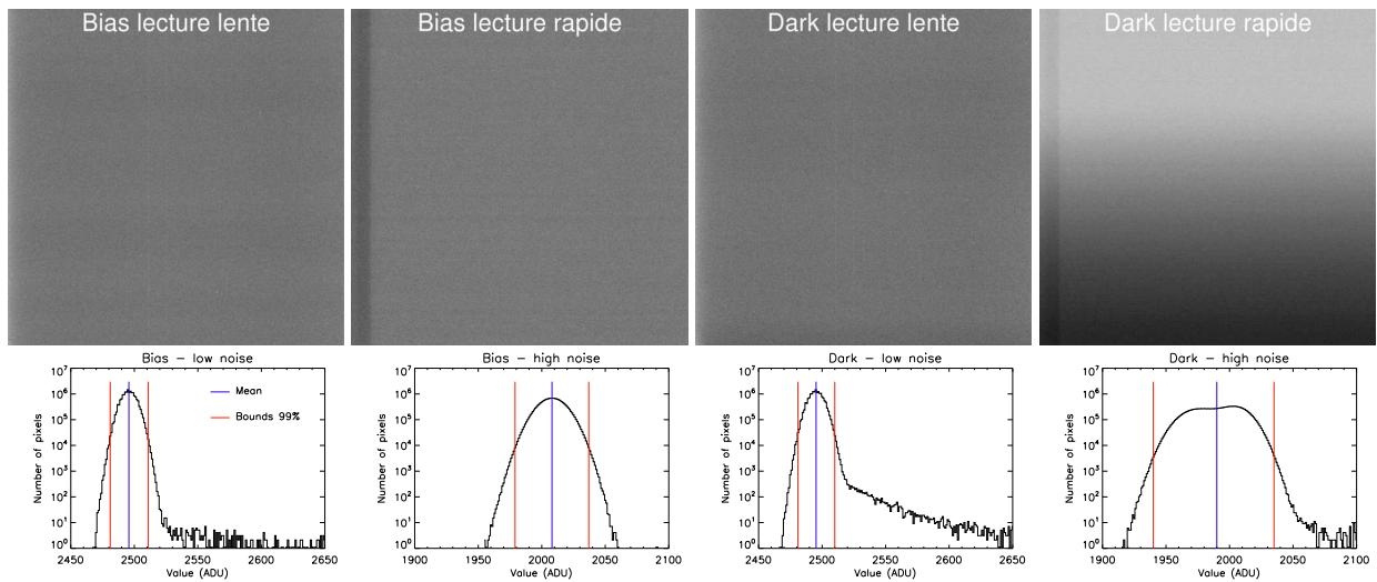
FIG. 3.7 – Exemple d’images de calibration : bias et dark en lecture lente et rapide, accompagnés de leurs histogrammes, pour la caméra ASTEP400 (classe A).
