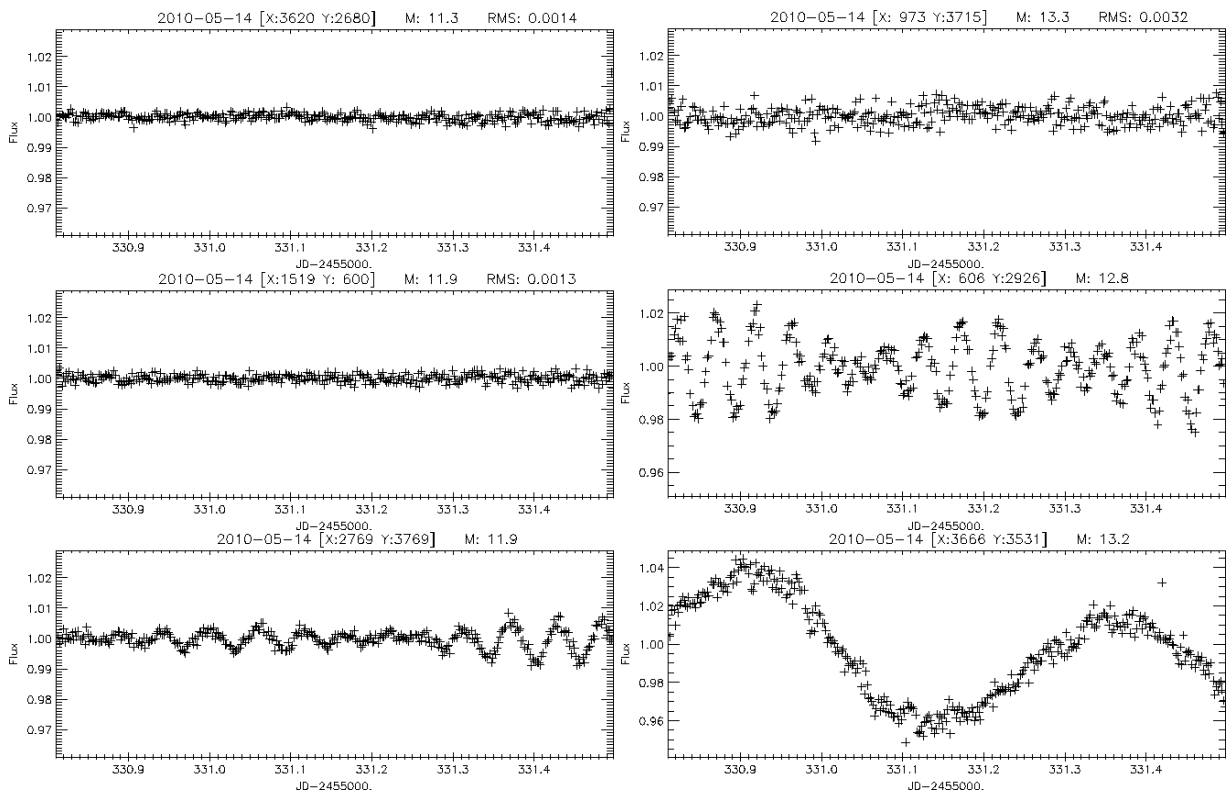
FIG. 7.31 – Courbes de lumière du 14 mai 2010. La précision est de 1.3 mmag pour une étoile de magnitude 11.9 ; on peut alors détecter des variations de l'ordre de 5 mmag (gauche). Pour une étoile de magnitude 13.3, la précision est de 3.2 mmag. On voit clairement des variations de l'ordre de 1% pour une magnitude 12.8 (droite).
