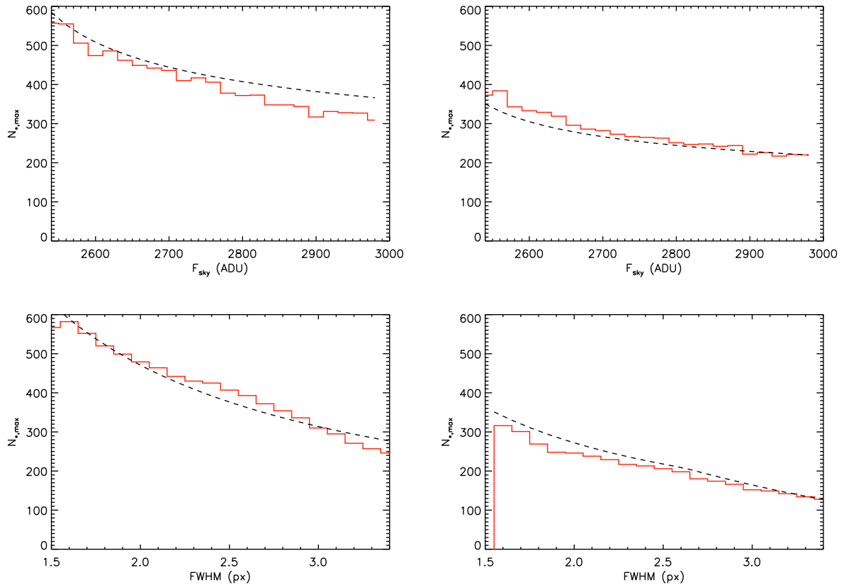
FIG. 4.33 – Validation du modèle pour les observations de 2009. La relation théorique N_{*,th} = f(F_{sky}, \omega) (ligne pointillée) est comparée au nombre d'étoiles détectées sur les meilleures images, d'abord en faisant varier le fond de ciel F_{sky} de 20 à 500 ADU (à partir de l'offset de 2490 ADU), pour un FWHM \omega fixé à 1.5 px (haut gauche) puis à 2.5 px (haut droite); ensuite en faisant varier le FWHM de 1.5 à 3.5 px, pour F_{sky} fixé à 20 ADU (bas gauche) puis à 500 ADU (bas droite). Ce test valide le modèle.
