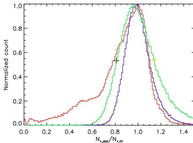
FIG. 4.34 – Rapport du nombre d'étoiles mesuré sur le nombre d'étoiles théorique pour l'hiver 2009, en rouge. Les histogrammes théoriques prenant en compte une erreur de mesure basse (de 0.25 px) et haute (de 0.38 px) sont représentés respectivement en bleu et vert. Les points noir et jaune permettent de calculer la largeur à mi-hauteur pour définir l'erreur haute.
