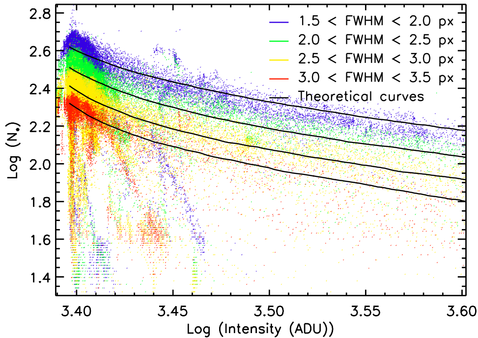
FIG. 4.21 – Nombre d'étoiles détectées en fonction de l'intensité du fond de ciel, pour différentes plages de FWHM, dans la 2 nd e approche. Les courbes théoriques sont indiquées en noir. On tient compte d'un offset de 2470 ADU sur l'intensité.
