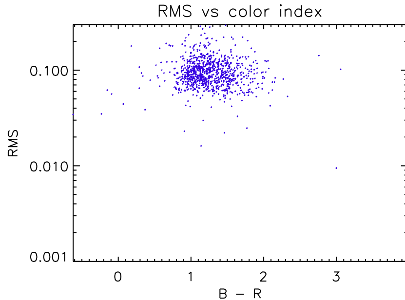
FIG. 5.20 – Bruit RMS en fonction l'indice de couleur B–R pour les étoiles dans la plage 13 < m_R < 13.5 .
