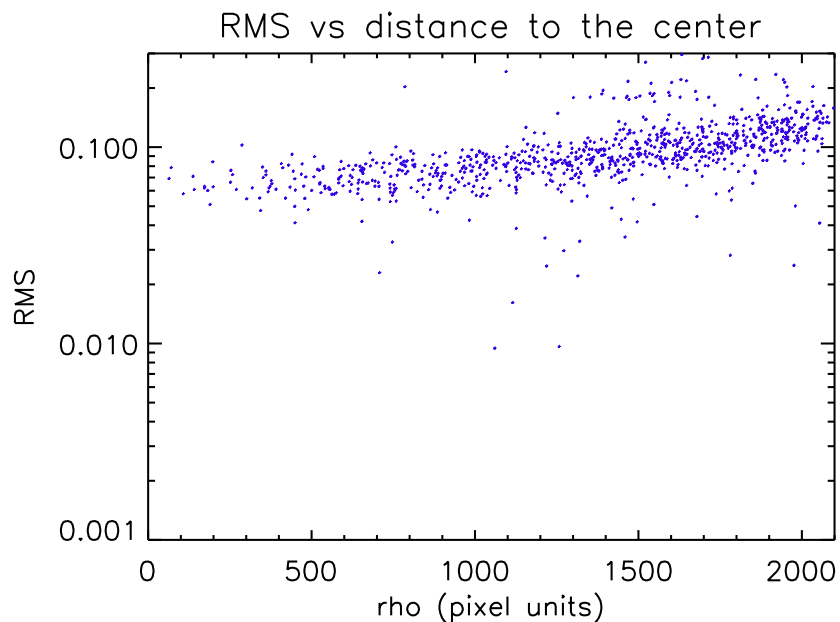
FIG. 5.19 – Bruit RMS en fonction de la distance radiale \rho pour les étoiles dans la plage 13 < m_R < 13.5 après amélioration de l’algorithme de reconnaissance de champ. On gagne un facteur 2 en bord de champ (voir figure 5.16), et on a un facteur 2 entre le centre et le bord du champ. Le bruit reste élevé.
