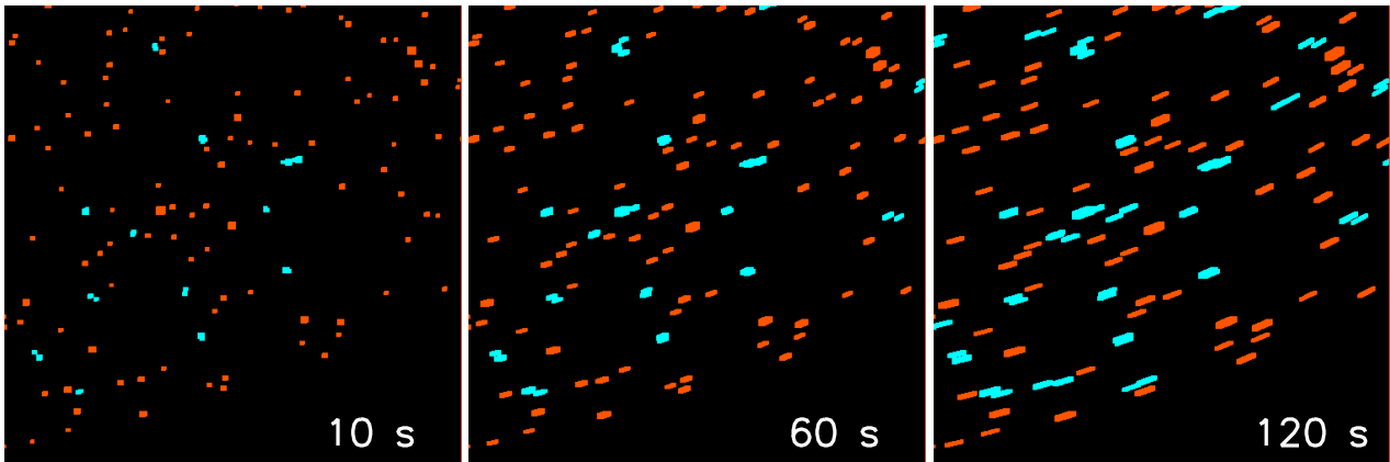
FIG. 4.9 – Simulation de la contamination dans le champ ASTEP Sud pour des temps de pose de 10 s, 60 s et 120 s, et une ouverture photométrique variable en fonction de la magnitude. On représente ici une zone de 500 \times 500 px prise dans un coin du CCD. Les étoiles non contaminées sont en orange et les étoiles contaminées en bleu. La contamination augmente avec le temps de pose.
