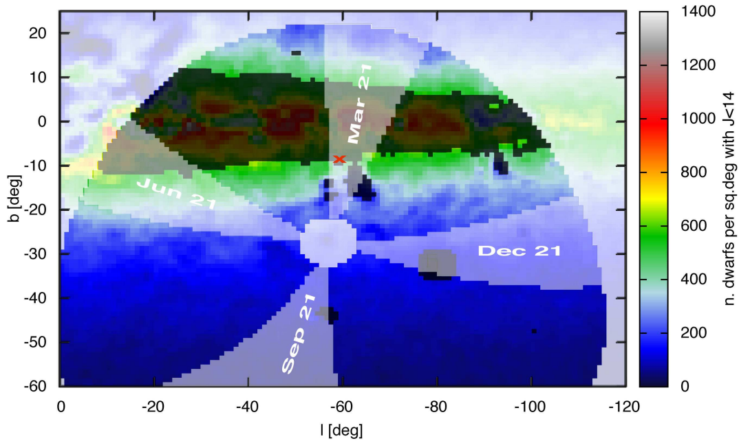
FIG. 7.14 – Densité de naines ( M_J < 14 ) par degré carré en coordonnées galactiques. La zone en couleurs pleines (non transparentes) correspond à la meilleure observabilité à la fois depuis Concordia et depuis le Chili (carte fournie par Mauro Barbieri). La zone noire correspond à une contamination élevée. On indique de plus les champs observables par BEST II en fonction de la période : les zones plus claires correspondent aux coordonnées des étoiles qui passent au méridien au Cerro Armazones entre 23h et 1h du matin à la date indiquée. La croix rouge montre la région de La Mouche, intéressante pour la recherche de transits.
