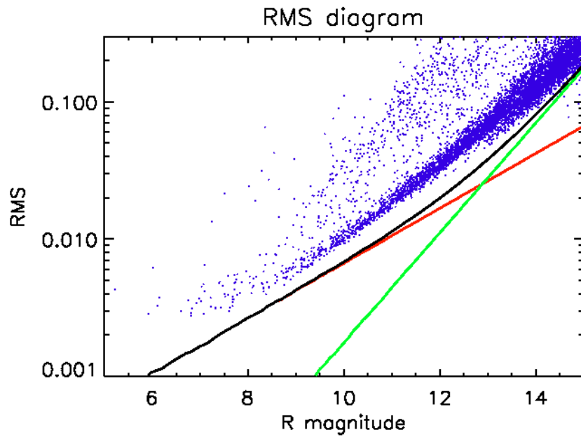
FIG. 5.23 – Diagramme RMS-magnitude obtenu avec ASTEP Sud (10 cm) après amélioration du traitement : les magnitudes sont les magnitudes instrumentales calibrées, l’algorithme de reconnaissance de champ a été amélioré, et les étoiles de référence sont mieux choisies. Le temps de pose est de 30 s. Le bruit de photons est indiqué en rouge, le bruit de fond de ciel en vert (en prenant une valeur de 40 ADU, la valeur exacte sera à préciser), et la somme des deux en noir.
