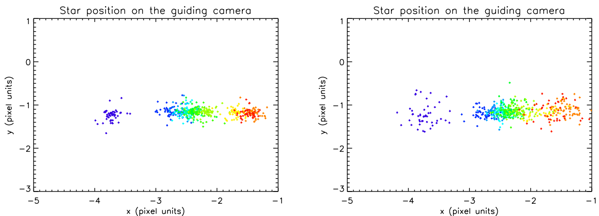
FIG. 6.20 – Position du centre de l'étoile guide sur des images simulées par SimPhot dans le cas d'une étoile fixe, pour des PSF de différentes focalisations : -500 (indigo), -300 (bleu roi), -100 (bleu), -50 (turquoise), 0 (vert), +50 (vert clair), +100 (jaune), +300 (orange) et +500 (rouge) \mu\text{m} , pour une étoile guide de magnitude 8 (gauche) et 10 (droite). Chaque point représente la position de l'étoile guide sur une image.
