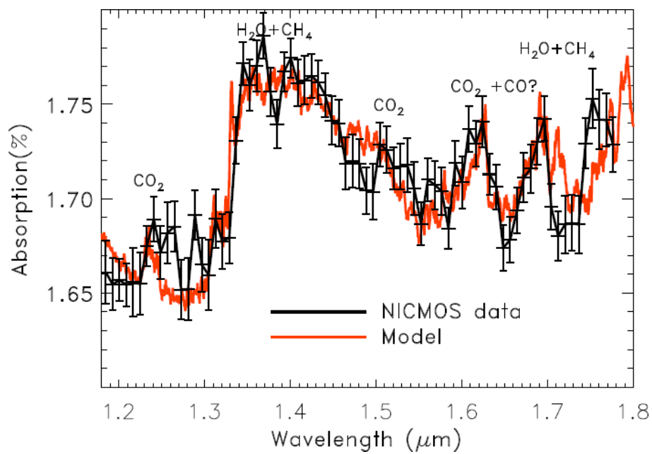
FIG. 1.10 – Spectre de l’atmosphère de la planète XO-1b, obtenu par Tinetti et al. [2010] avec l’instrument NICMOS du télescope spatial Hubble. On identifie la présence d’eau, de dioxyde de carbone, de méthane, et peut-être de monoxyde de carbone.
