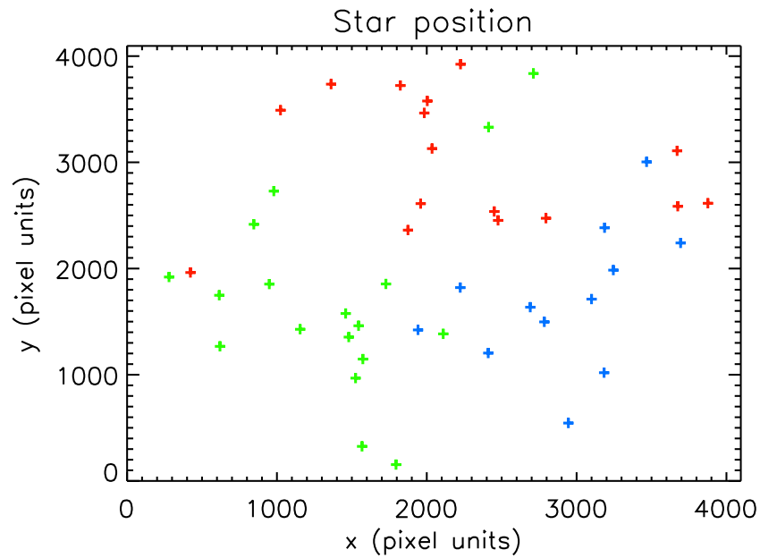
FIG. 5.26 – Position sur le CCD à un instant donné de plusieurs étoiles dont la courbe de lumière correspond à une des formes identifiées figure 5.25, repérées par les couleurs bleu, vert et rouge.
