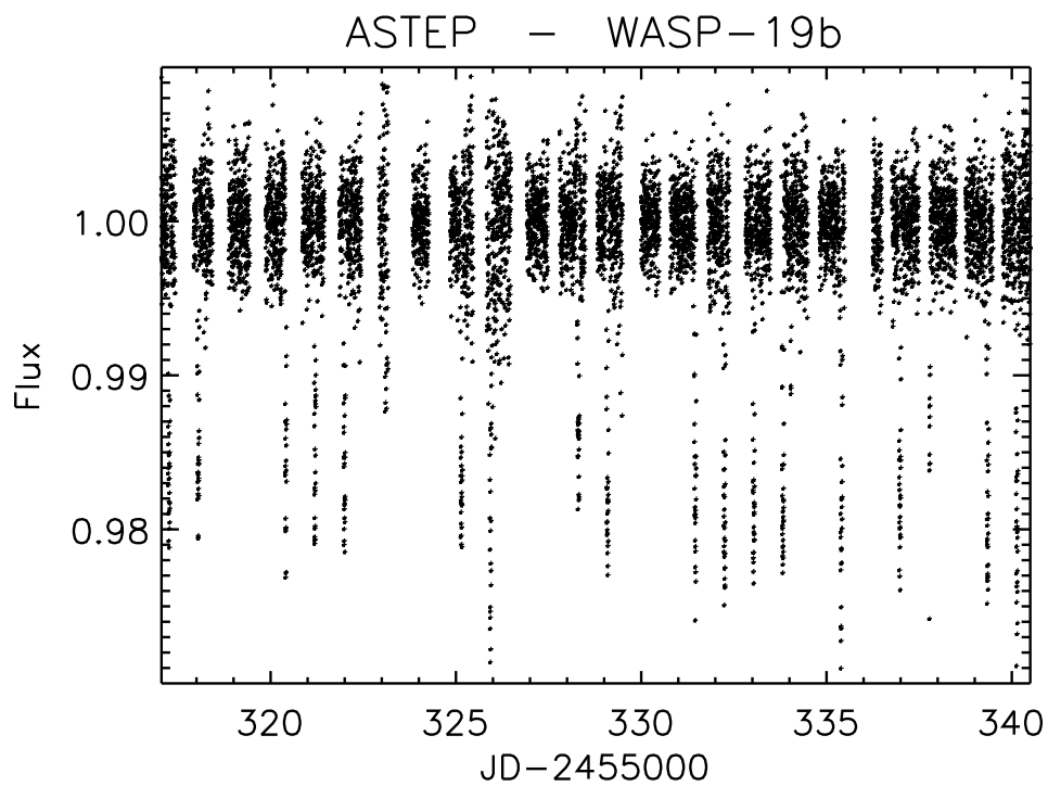
FIG. 7.19 – Courbe de lumière de WASP-19 sur toute la durée des observations, soit entre le 30 avril et le 23 mai 2010.
