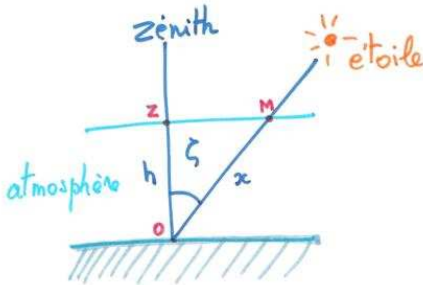
FIG. 2.4 – Atmosphère plan-parallèle et distance angulaire zénithale \zeta . Dans ce cadre, la masse d'air peut s'exprimer de manière simple.
