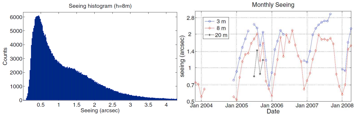
FIG. 1.15 – Histogramme des mesures de seeing à 8 m d’altitude sur 3.5 années (gauche), et statistiques par mois (droite). Le seeing à l’intérieur de la couche limite est bien moins bon en hiver qu’en été. Figure tirée de Aristidi et al. [2009].
