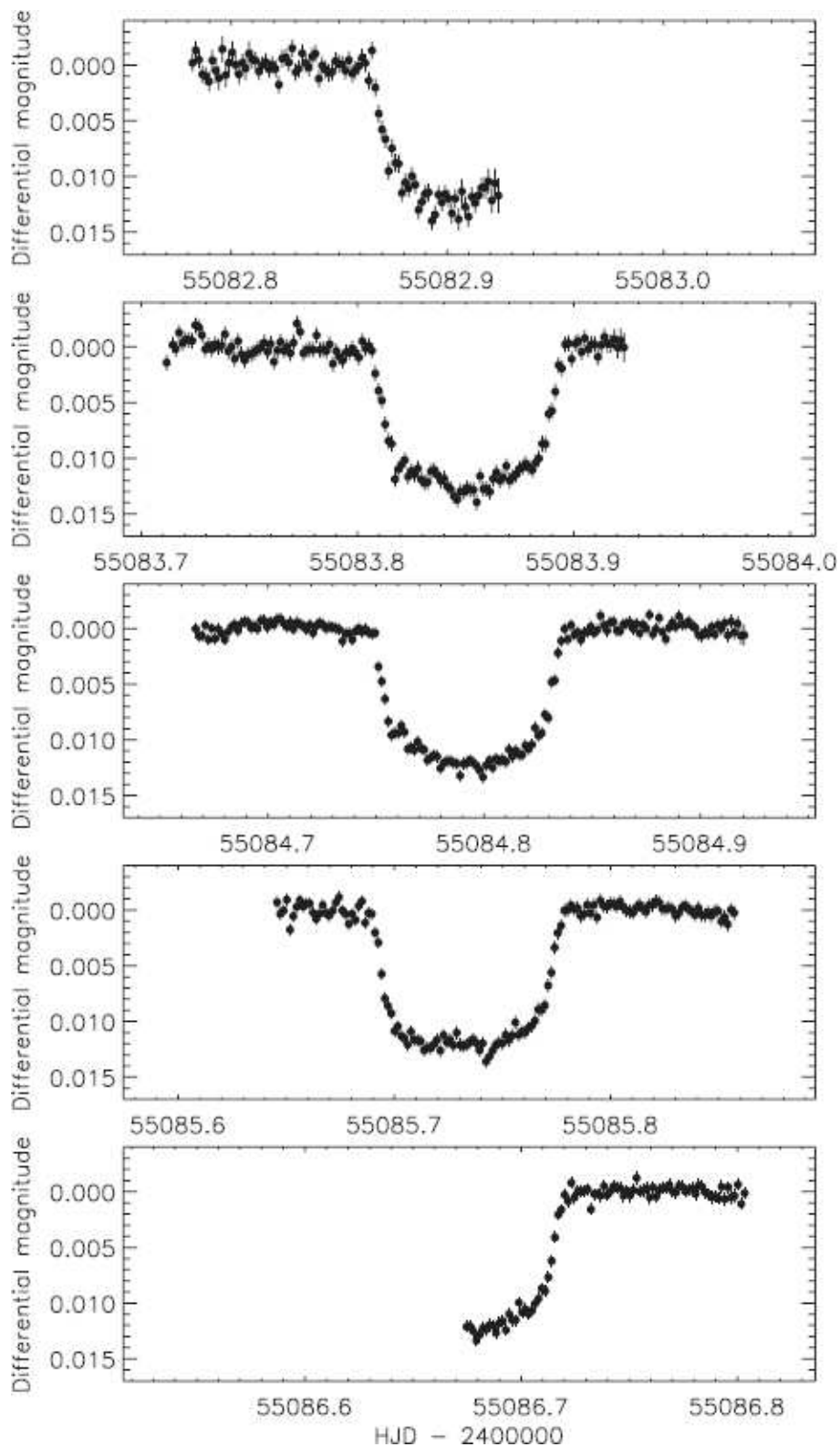
FIG. 7.24 – Courbes de lumière de WASP-18 obtenue par Southworth et al. [2009] avec le télescope Danois de l'ESO, de 1.54 m de diamètre. Les poses sont de 80 s, les observations sont faites en bande V de Johnson. La précision obtenue varie de 470 à 830 ppm.
