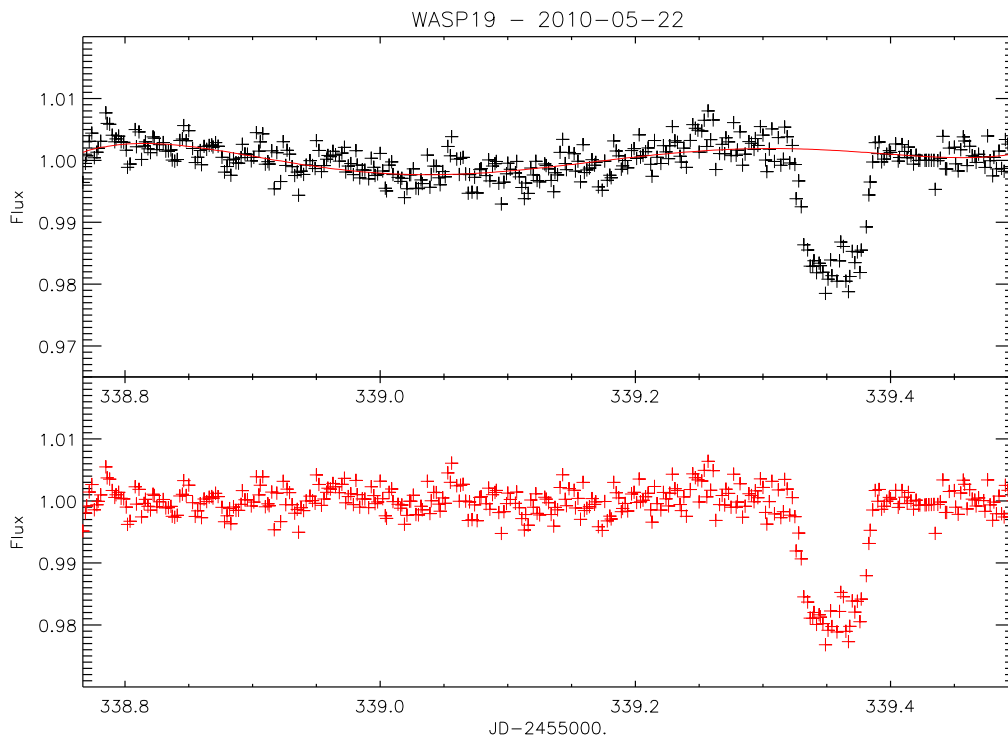
FIG. 7.18 – Courbe de lumière de WASP-19 pour la journée du 22 mai 2010, avec l’ajustement d’un polynôme (haut) et après soustraction de celui-ci (bas).
