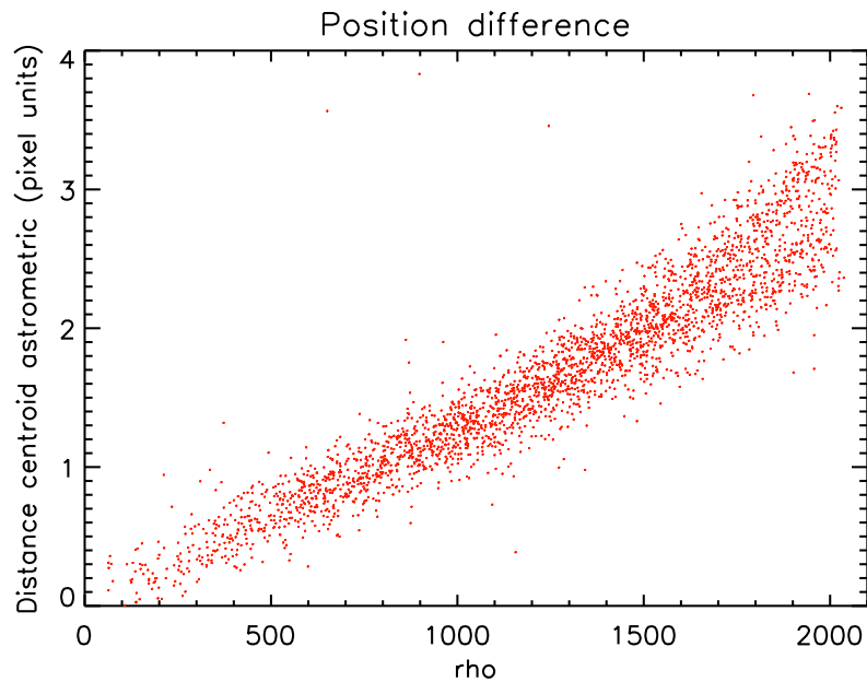
FIG. 5.17 – Différence entre les positions calculées par l'algorithme de reconnaissance de champ et par détermination du centroïde, en fonction de la distance radiale \rho . On a une corrélation nette.
