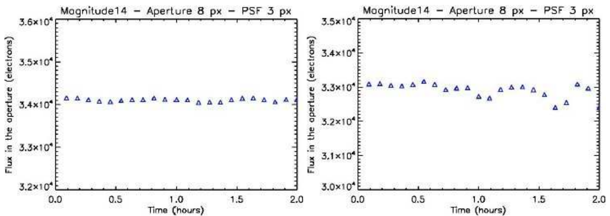
FIG. 6.11 – Courbes de lumière obtenues dans le cas d’un seeing optimiste (gauche), et pessimiste (droite), moyennées sur 20 minutes. Dans le cas pessimiste, on retrouve les variations de seeing, qui constituent le bruit dominant.
