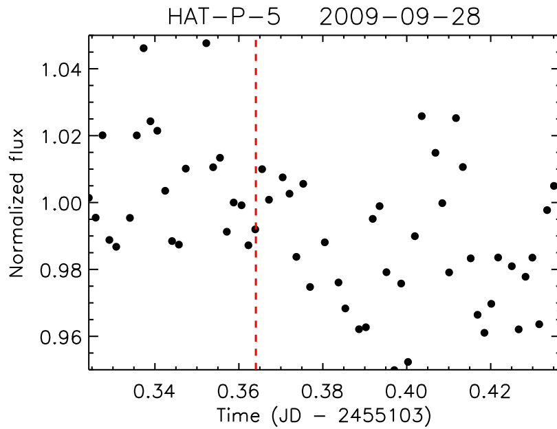
FIG. 7.4 – Courbe de lumière obtenue lors du transit de HAT-P-5b, par photométrie de soustraction. Le début du transit est représenté par la ligne pointillée rouge. La dispersion hors-transit est de 2.2%.
