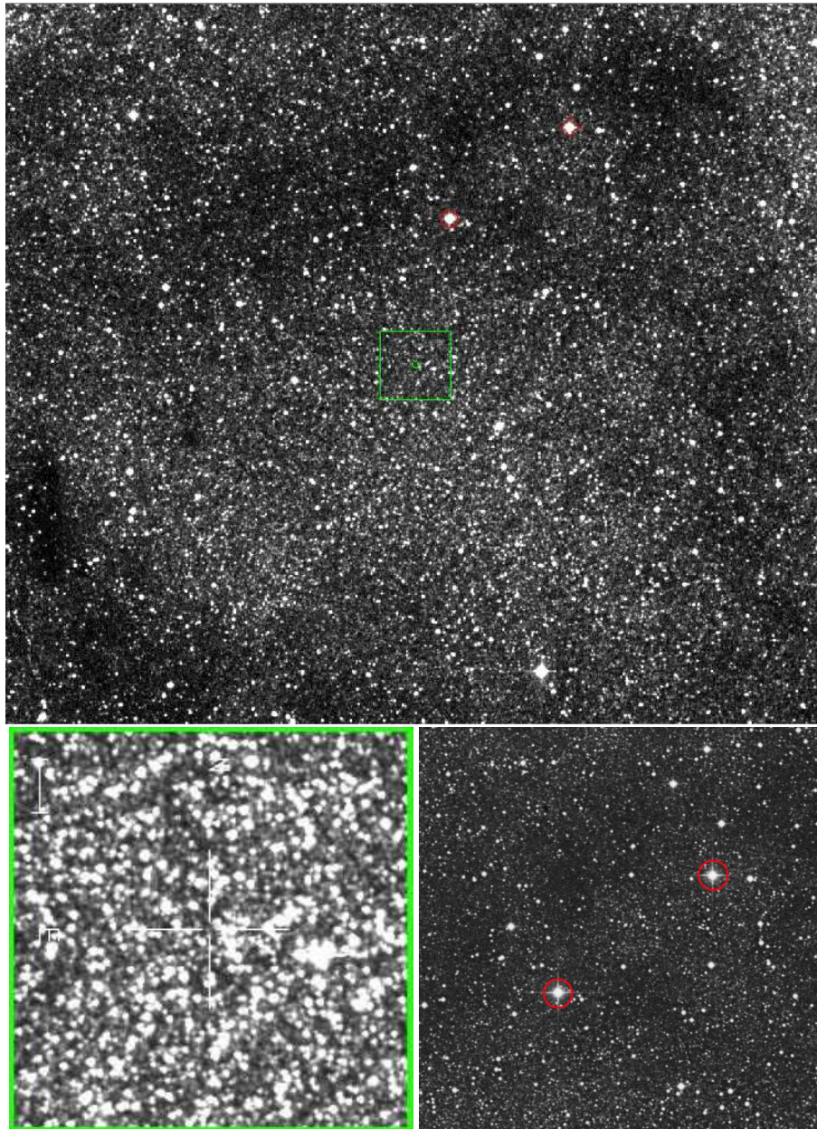
FIG. 7.26 – Cartes de champ envoyées à Concordia pour l'identification de la microlentille MOA 2010-BLG-285. Haut : carte de 0.5 \times 0.5^{\circ 2} . La cible doit apparaître dans le cercle vert au centre de l'image. Deux étoiles brillantes entourées en rouge peuvent servir d'étoile guide, la plus proche de la cible est HD 163301. Bas gauche : carte de la zone centrale de \sim 3' \times 3' . Bas droite : carte de 0.2 \times 0.2^{\circ 2} autour des deux étoiles-guide potentielles.
