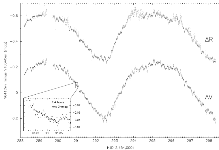
FIG. 1.20 – Courbes de lumière de V841 Cen et V1034 Cen, de magnitude 8.5, obtenues par l’instrument Small IRAIT sur 10 jours d’observations lors de l’hiver 2007. La précision sur un sous-ensemble de 2.4 heures est de 3 mmag en bande V et 4.2 mmag en bande R. Figure tirée de Strassmeier et al. [2008].
