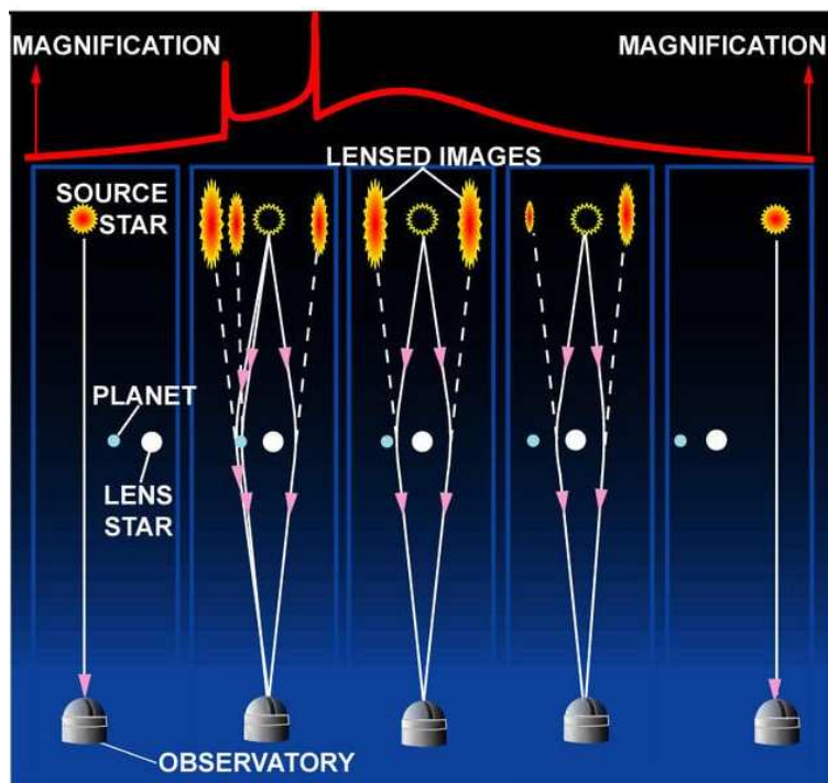
FIG. 1.2 – Détection d’une exoplanète par lentille gravitationnelle. Une étoile située entre la source et l’observateur va dévier la lumière et entraîner la formation de plusieurs images, et donc une magnification de l’éclat de la source. La courbe de magnification peut alors contenir des pics révélant la présence d’une planète.
