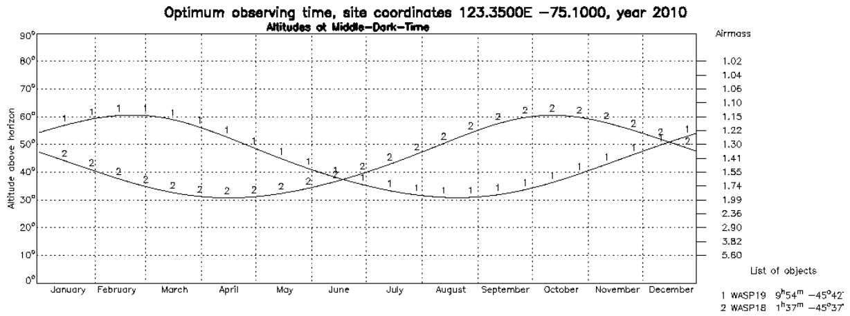
FIG. 7.15 – Altitude de WASP-19 (objet 1) et WASP-18 (objet 2) au cours de l’année 2010 depuis le Dôme C. WASP-19 est au-dessus de 40° du début de l’hiver jusqu’à début juin, et WASP-18 de fin juin jusqu’à la fin de l’hiver. Figure réalisée à partir de http://catserver.ing.iac.es/staralt/ .
