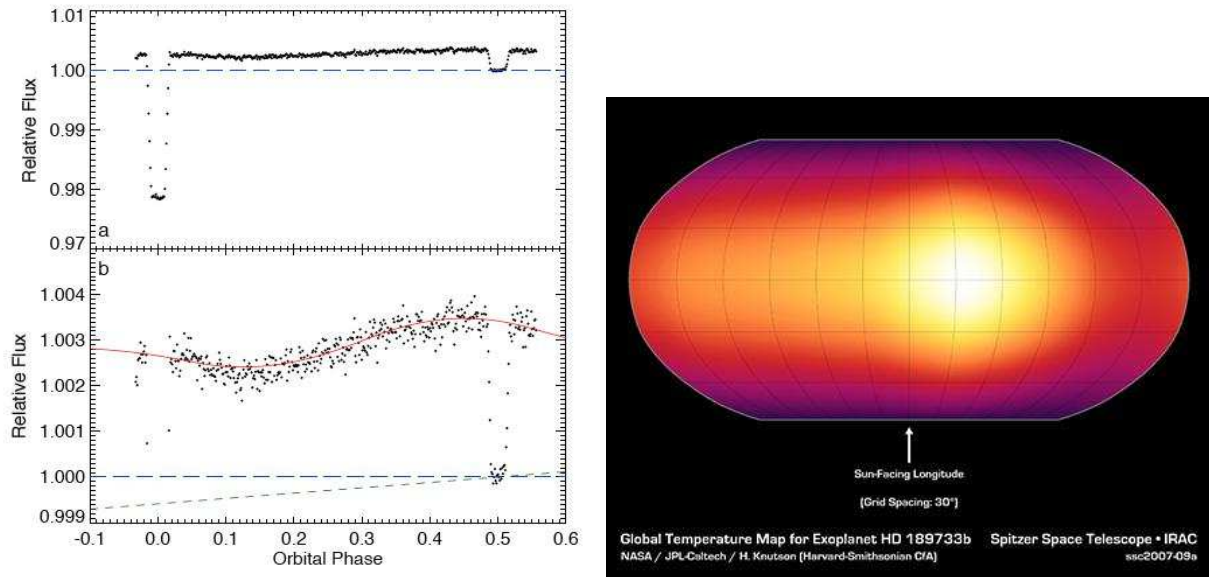
FIG. 1.9 – La courbe de lumière de HD189733 par le satellite Spitzer en infrarouge (gauche) fait apparaître les transits primaires et secondaires (haut) ainsi que des variations sur toute la période de rotation de la planète (bas) qui permettent d'obtenir la carte de température de la planète (droite). Figure tirée de Knutson et al. [2007].
