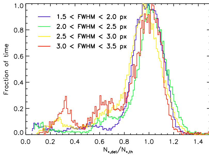
FIG. 4.24 – Histogramme du rapport du nombre d'étoiles détectées sur le nombre d'étoiles théorique pour les différentes plages de FWHM, dans la 2 nd e approche. Un critère ad hoc serait là encore nécessaire pour déduire la fraction de temps photométrique, et une incertitude serait engendrée par les résultats différents pour chaque plage de FWHM.
