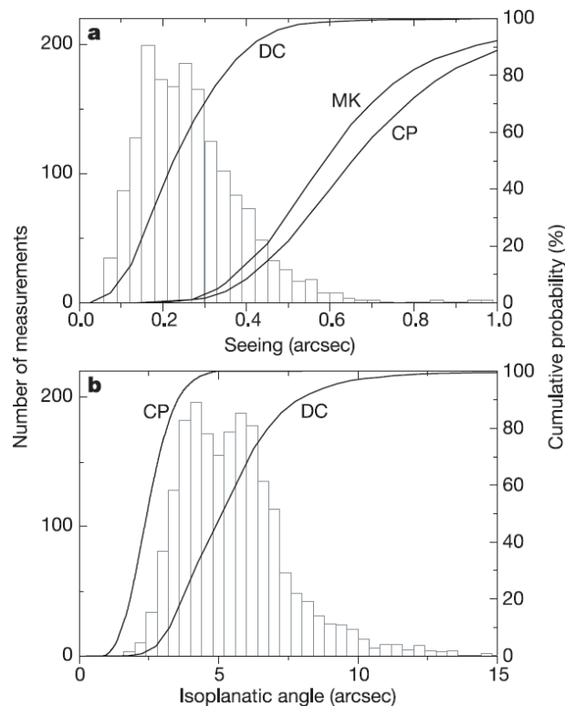
FIG. 1.14 – Histogrammes des mesures de seeing (haut) et d'angle isoplanétique (bas) obtenues au Dôme C entre avril et mai 2004. Le seeing médian est de 0.27 arcsec, et l'angle isoplanétique médian de \sim 5 arcsec. Ces valeurs sont meilleures d'un facteur 2 à 3 que dans les observatoires classiques, et sont valables au-dessus de 30 m. Figure tirée de Lawrence et al. [2004].
