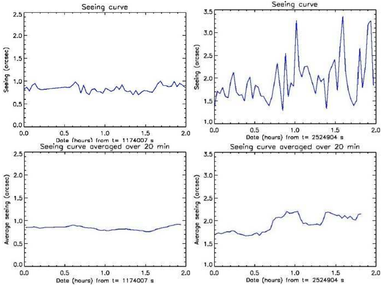
FIG. 6.10 – Deux cas de seeing tirés des mesures de l’hiver 2005 au Dôme C (haut) sont systématiquement utilisés pour les simulations : un cas de bon seeing (gauche) et un cas de mauvais seeing (droite). Une moyenne glissante sur 20 minutes (bas) permettra une comparaison avec les courbes de lumière simulées.
