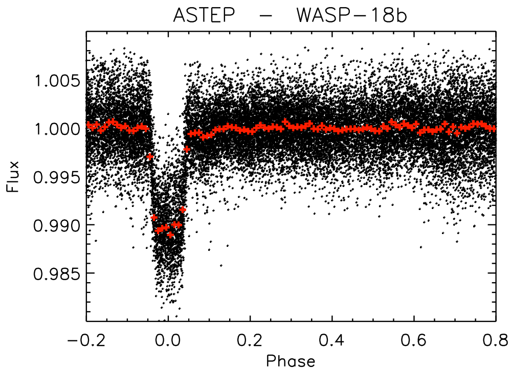
FIG. 7.25 – Courbe de lumière de WASP-18 en phase, à partir des 23 jours d’observations (~24 périodes). Une moyenne par intervalle de 1/100^{\text{ème}} de période, soit 14 mn, est représentée en rouge.
