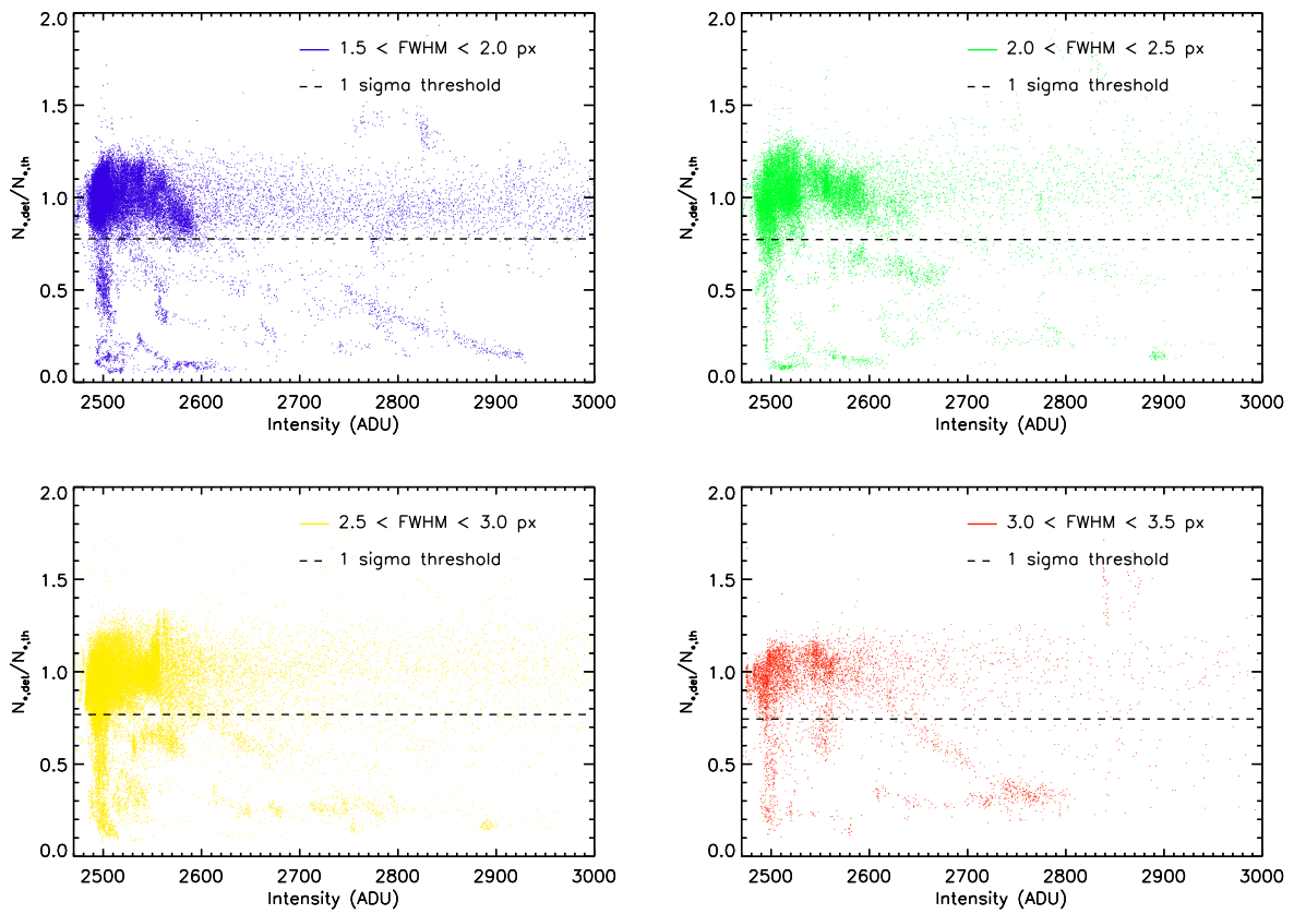
FIG. 4.22 – Rapport du nombre d'étoiles détectées sur le nombre d'étoiles théorique en fonction de l'intensité pour les différentes plages de FWHM, dans la 2 nde approche. La limite à 1 \sigma est indiquée en pointillés.
