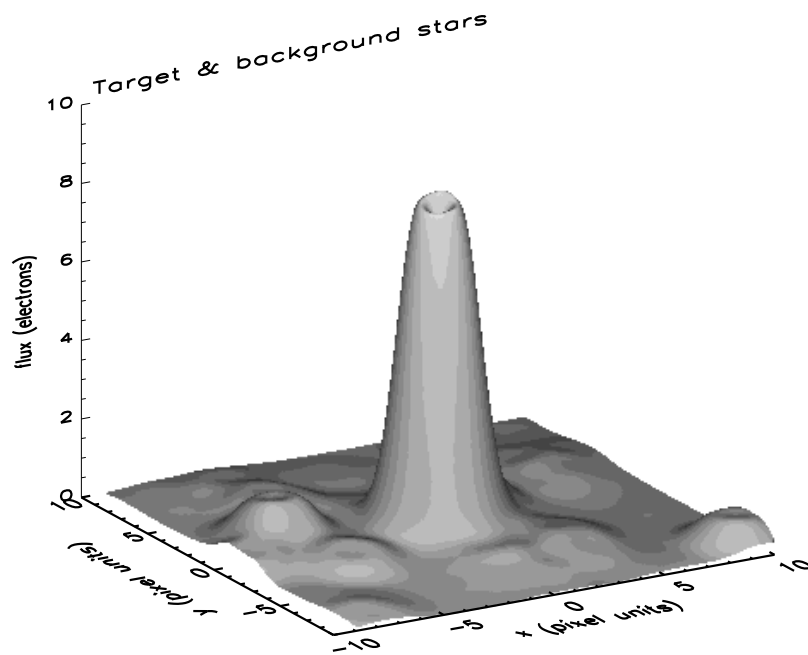
FIG. 2.14 – Portion de champ simulée par SimPhot, pour une étoile cible de magnitude 14, un temps de pose de 30 s et un télescope de diamètre 40 cm. L'étoile cible est placée à peu près au centre de la grille, et des étoiles de fond sont réparties aléatoirement.
