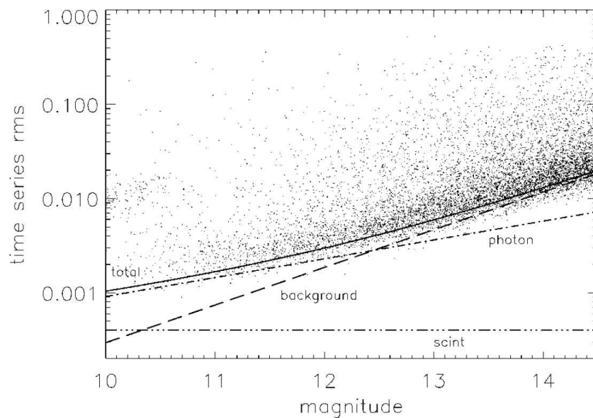
FIG. 5.24 – Diagramme RMS-magnitude obtenu avec le télescope de 20 cm BEST, sur des poses de 240 s pendant 3 heures d’observations [Rauer et al., 2004]. La précision est de \sim 1 mmag pour les magnitudes 10. Les bruits de photon, de fond de ciel et de scintillation sont indiqués.
