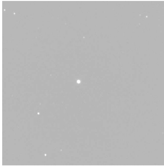
FIG. 7.12 – Exemple d’image de 512 \times 512 px obtenue lors des premières observations de nuit à Concordia, le 28 février 2010, au centre du champ.
