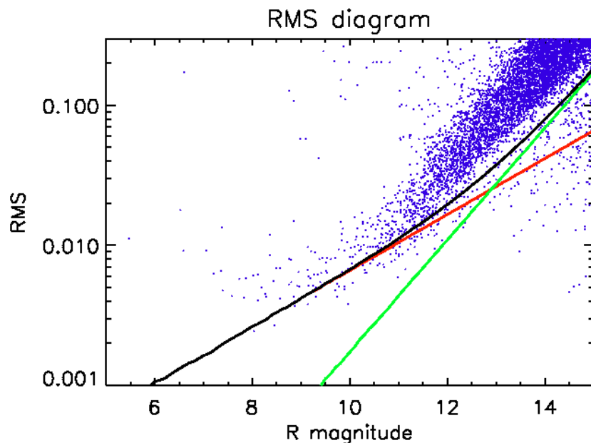
FIG. 5.13 – Diagramme RMS-magnitude obtenu avec ASTEP Sud sur la journée de 12 juillet 2008. Le temps de pose est de 30 s. Les magnitudes sont celles du catalogue GSC2.2. Le bruit de photons est indiqué en rouge, le bruit de fond de ciel en vert (en prenant une valeur de 40 ADU, la valeur exacte sera à préciser), et la somme des deux en noir. Une dispersion de quelques mmag est atteinte pour les étoiles les plus brillantes, mais la grande majorité des étoiles a une dispersion de plusieurs %, trop grande pour détecter un transit.
