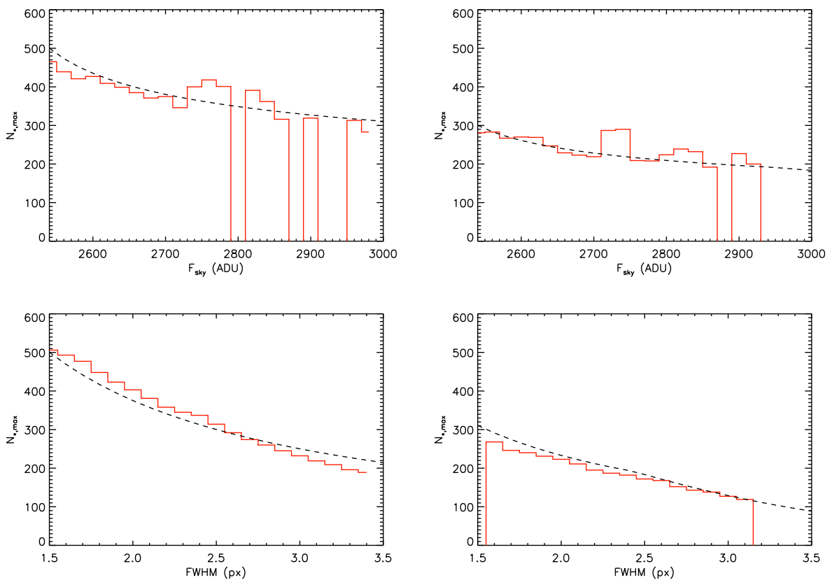
FIG. 4.26 – Validation du modèle de la 3 ème approche, pour les observations de 2008. La relation théorique N_{*,th} = f(F_{sky}, \omega) (ligne pointillée) est comparée au nombre d'étoiles détectées sur les meilleures images, d'abord en faisant varier le fond de ciel F_{sky} de 40 à 500 ADU (à partir de l'offset de 2470 ADU), pour un FWHM \omega fixé à 1.5 px (haut gauche) puis à 2.5 px (haut droite); ensuite en faisant varier le FWHM de 1.5 à 3.5 px, pour F_{sky} fixé à 40 ADU (bas gauche) puis à 500 ADU (bas droite). Ce test valide le modèle.
