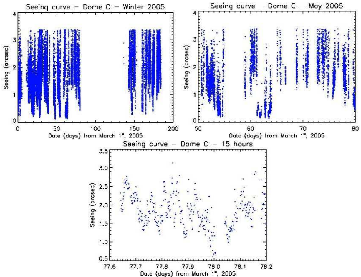
FIG. 6.9 – Valeurs de seeing mesurées durant l’hiver 2005, de mars à août (haut gauche), pour le mois de mai (haut droite), et durant une quinzaine d’heures (bas).
