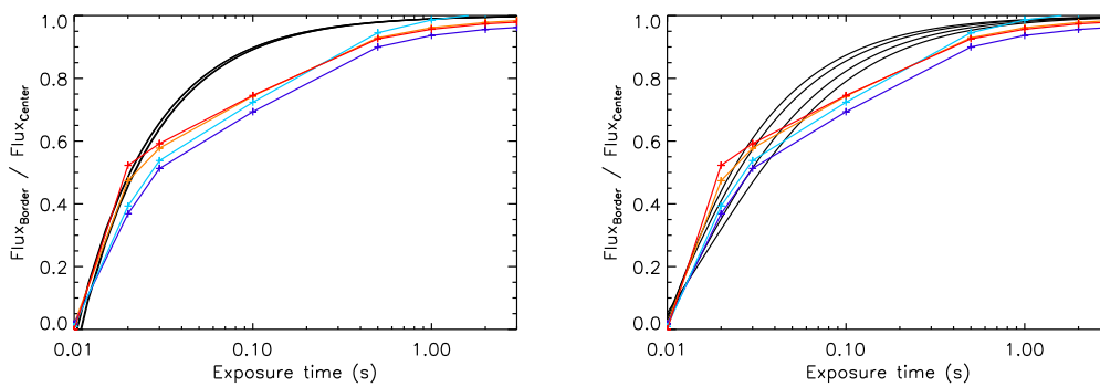
FIG. 3.19 – Tentative d’ajustement (en noir) du rapport des flux entre le bord et le centre de l’image en fonction du temps de pose (mêmes couleurs que figure 3.18), par une fonction r = 1 - t_s/t pour t > t_s et r = 0 sinon (gauche), et r = 1 - t_s/(t - t_0) pour t > t_s et r = 0 sinon (droite).
