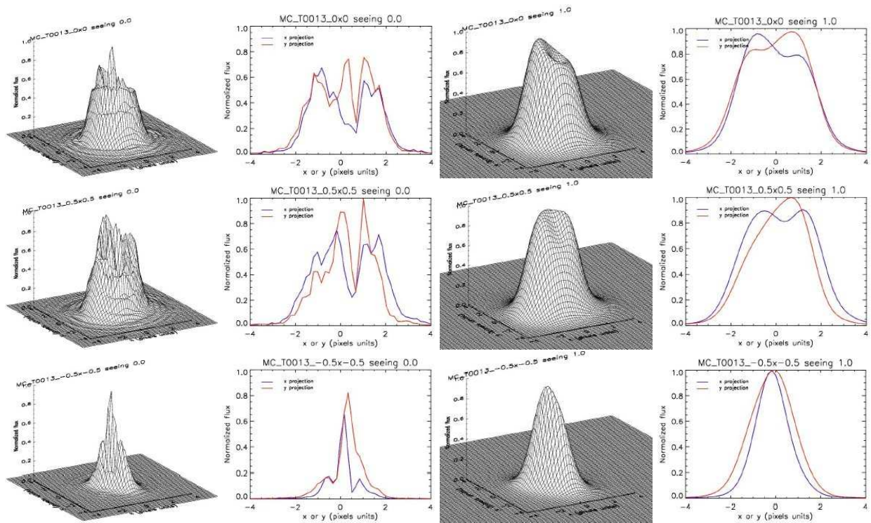
FIG. 6.13 – PSF issue des simulations de tolérancements et utilisée pour les simulations photométriques, en 3 dimensions et en coupe selon x (bleu) et y (rouge), avant (gauche) et après (droite) convolution avec une gaussienne de 1 arcseconde, au centre du champ (haut), dans la diagonale à 0.5^\circ \times 0.5^\circ (milieu) et à -0.5^\circ \times -0.5^\circ (bas).
