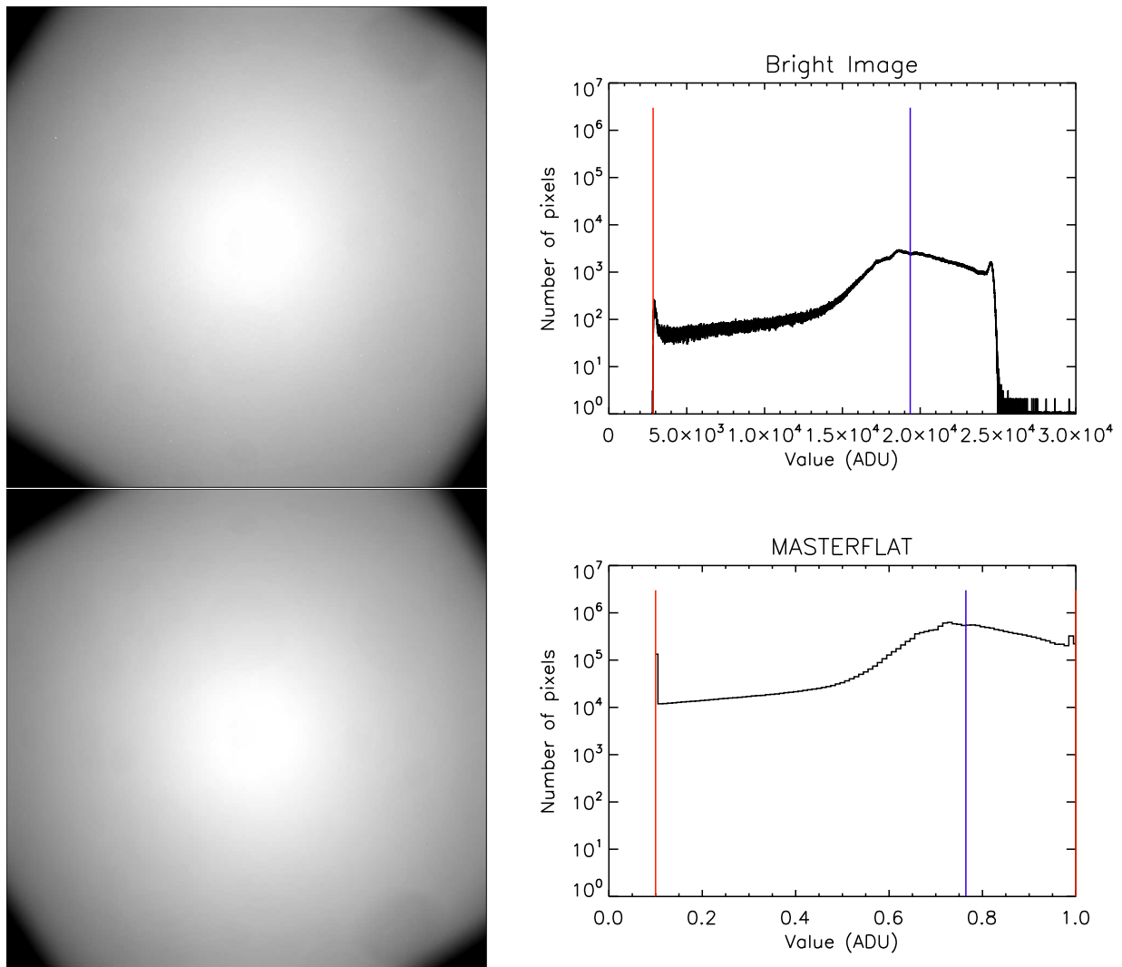
FIG. 5.6 – Exemple d’image brillante utilisée comme flat (haut), et masterflat de la journée du 12 juillet 2008 (bas), accompagnés de leur histogramme. La médiane est indiquée en bleu et les limites contenant 99 % des pixels en rouge.
