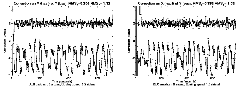
FIG. 7.1 – Correction appliquée en X et Y, équivalente à la distance au point de fonctionnement, pour une étoile à 45^\circ de déclinaison, avec différents paramètres pour la vitesse de guidage : 0.5 s (gauche) et 1 s (droite). Le backlash n'est pas compensé. Les courbes sont centrées sur \pm 2 px pour une bonne lisibilité.
