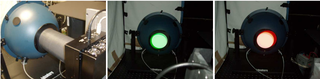
FIG. 3.4 – Sphère intégrante utilisée pour les tests des caméras ASTEP. Un monochromateur placé en amont permet de choisir la longueur d'onde.
