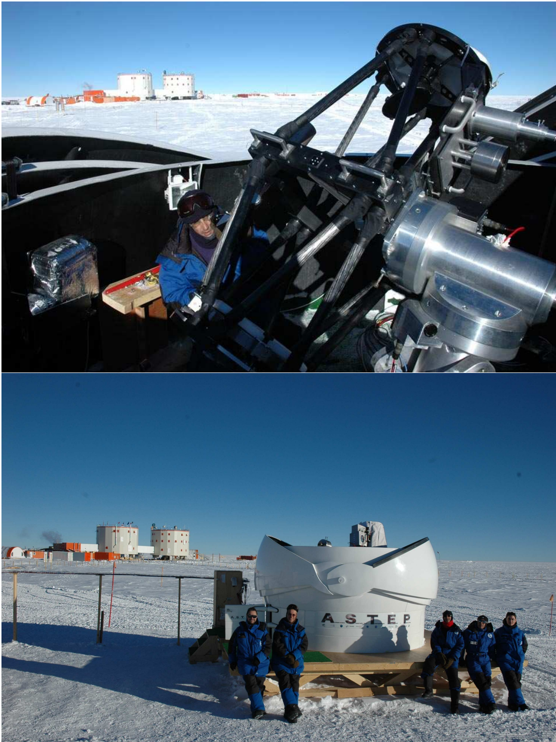
FIG. 7.9 – Installation d'ASTEP400 dans sa coupole, à Concordia, durant la campagne d'été 2010.
