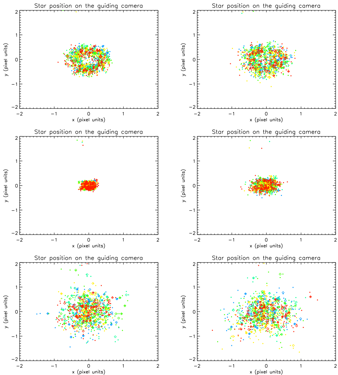
FIG. 6.21 – Position du centre de l'étoile guide sur des images simulées par SimPhot dans le cas d'une étoile mobile, pour des PSF de différentes focalisations : -100 (bleu), -50 (turquoise), 0 (vert), +50 (jaune) et +100 (rouge) \mu\text{m} , et pour une étoile de magnitude 8 (gauche) et 10 (droite). Divers mouvements sont appliqués au télescope : une dérive de 0.6 px/s sans jitter (haut), de 0.1 px/s sans jitter (milieu), et de 0.1 px/s avec un jitter de 0.2 px/s (bas). Les croix représentent la position de l'étoile guide sur chaque image, et les losanges la position médiane sur 5 poses successives à partir desquelles une correction de guidage est appliquée.
