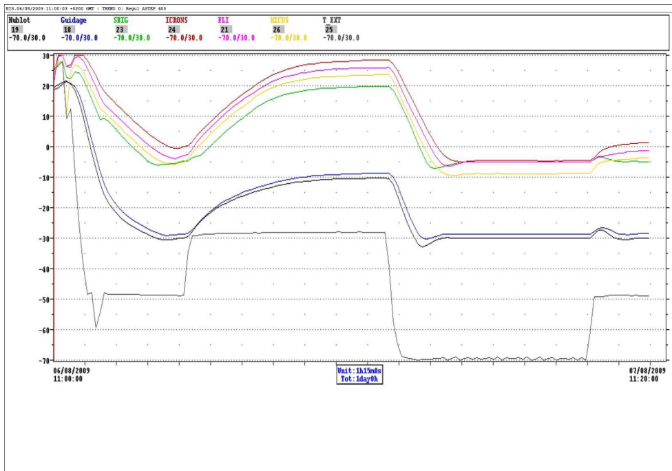
FIG. 6.32 – Exemple de courbes de température de la boîte caméra d’ASTEP 400 obtenues dans l’enceinte climatique au Mont Gros, sur 24 heures. Les courbes correspondent aux données de différents capteurs de température placés respectivement : (en noir) à l’intérieur du double hublot d’entrée de la boîte ; (en bleu) au niveau du miroir M3 ; (en vert) au niveau de la caméra de guidage ; (en rouge) au niveau du transformateur ICRON ; (en rose) au niveau de la caméra de science ; (en jaune) au niveau de la platine de focalisation MICOS. La courbe la plus basse (en noir) correspond à la température extérieure, imposée, dans l’enceinte climatique.
