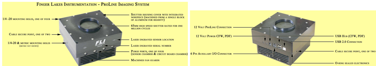
FIG. 3.1 – Caméra ProLines de Finger Lake Instrumentation utilisée pour les instruments ASTEP.
