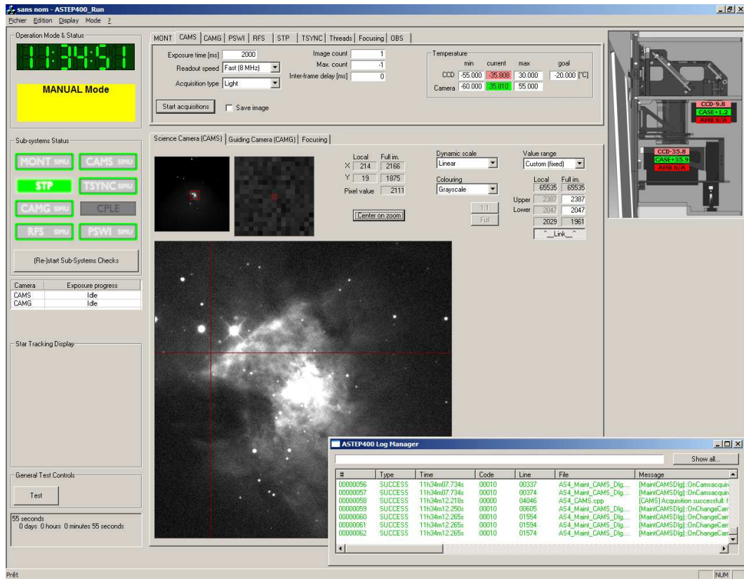
FIG. 6.30 – Interface graphique du logiciel de commande d’ASTEP400. Ce logiciel gère le fonctionnement de tous les éléments d’ASTEP400. Il effectue les étapes préliminaires aux observations, les acquisitions et la sauvegarde des données.
