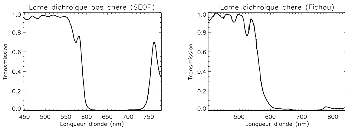
FIG. 6.27 – Transmission des lames dichroïques. Modèle pas cher proposé par l'entreprise SEOP (gauche), et modèle cher proposé par l'entreprise Fichou (droite). Les courbes sont simulées et fournies par le constructeur.
