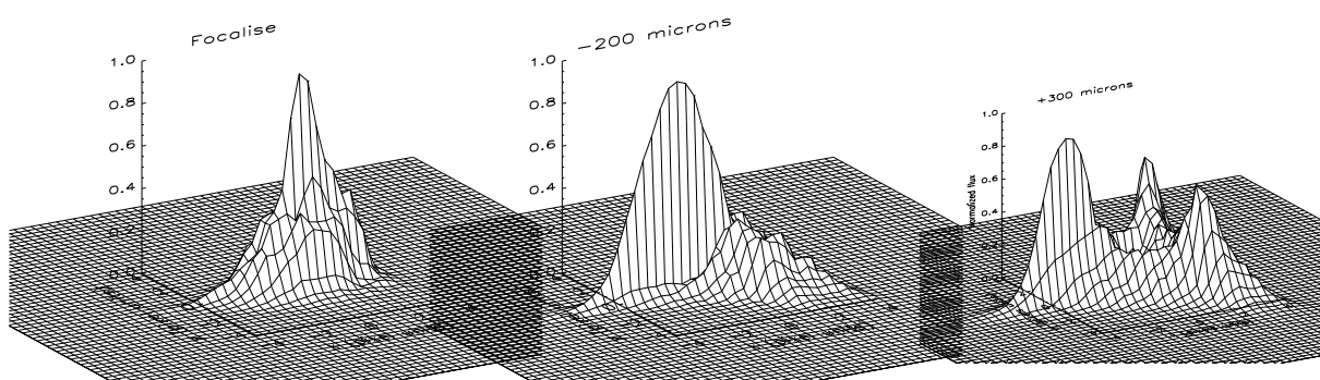
Fig. 6.26 – Exemples de PSF de la voie de guidage avec une lame dichroïque prismatique : PSF focalisée (gauche), défocalisée à -200 \mu\text{m} (centre) et à +300 \mu\text{m} (droite).
