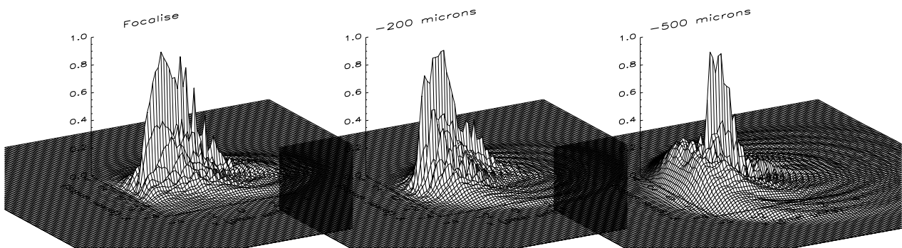
FIG. 6.18 – Exemples de PSF de la voie de guidage : PSF focalisée (gauche) et défocalisée à -200 \mu\text{m} (centre) et -500 \mu\text{m} (droite).
