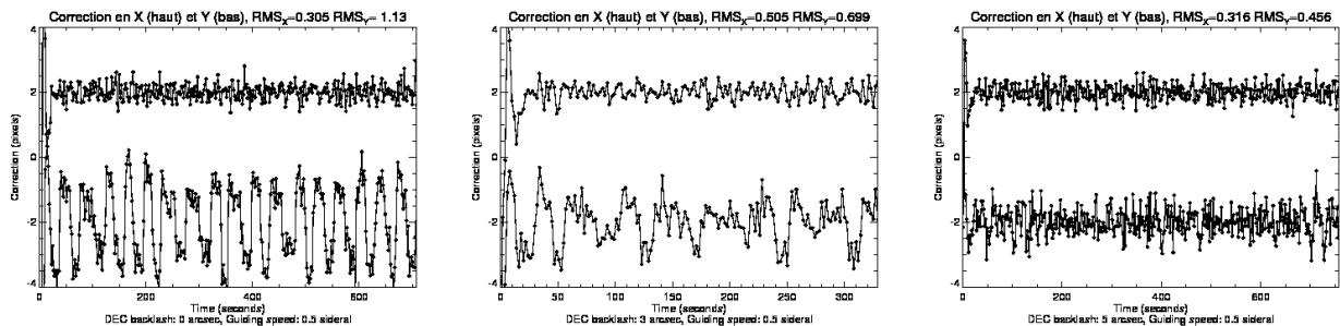
FIG. 7.2 – Correction appliquée en X et Y, équivalente à la distance au point de fonctionnement, pour une étoile à 45^\circ de déclinaison, avec différents paramètres pour la compensation du backlash en déclinaison : 0 arcsec (gauche), 3 arcsec (milieu) et 5 arcsec (droite). La vitesse de guidage est de 0.5 s. Les courbes sont centrées sur \pm 2 px pour une bonne lisibilité.
