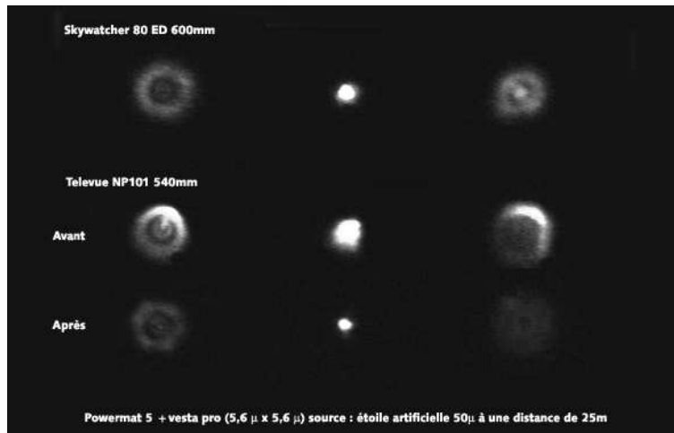
FIG. 4.19 – PSF pour une lunette Skywatcher bien collimatée (haut), et pour la lunette Télévue d'ASTEP Sud avant (milieu) et après (bas) la recollimation, pour une position intra-focale (gauche), focalisée (milieu) et extra-focale (droite). La lunette ASTEP Sud, soumise à la température extérieure entre son installation et le début de la campagne, a subi une décollimation importante. Une recollimation a dû être effectuée par les hivernants. Image : Erick Bondoux.
