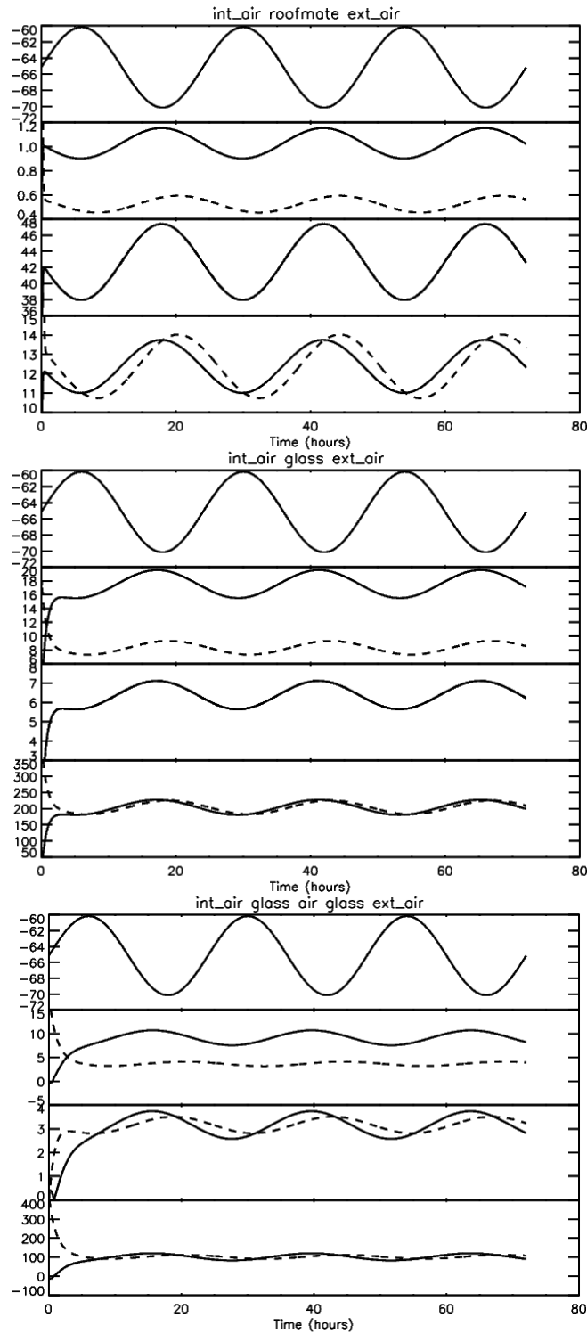
FIG. 6.6 – Résultats des simulations thermiques pour le roofmate (haut), la vitre simple (milieu), et le double vitrage avec une couche réfléchissante dans l'infrarouge (bas). On fait osciller la température extérieure entre -60 et -70^{\circ}\text{C} (1 er graphe). La température intérieure est contrôlée pour être à -20^{\circ}\text{C} . Le 2 ème graphe montre la différence de température entre l'air extérieur et la surface extérieure de la couche isolante (ligne pleine), et entre l'air intérieur et la surface intérieure de la couche isolante (ligne pointillée). Le 3 ème graphe montre la différence de température entre les deux surfaces de la couche isolante. Le 4 ème graphe montre le flux sortant (ligne pleine) et le flux à l'intérieur de l'enceinte (ligne pointillée), en \text{W}/\text{m}^2 .
