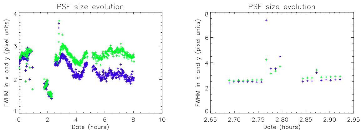
FIG. 4.15 – Taille des PSF lors des observations de test réalisées le 1 er octobre 2007 à l'Observatoire de Calern, au cours de la nuit (gauche), et zoom lors des tests du hublot (droite). Le temps est compté à partir du début des observations. La meilleure focalisation obtenue est 1.5 px de FWHM. Les variations au cours de la nuit seront a priori éliminées grâce à la thermalisation. Lorsqu'une lame est placée manuellement devant la lunette, soit entre 2.76h et 2.81h puis à 2.87h, la PSF passe de 2.5 à environ 3.5 px de FWHM.
