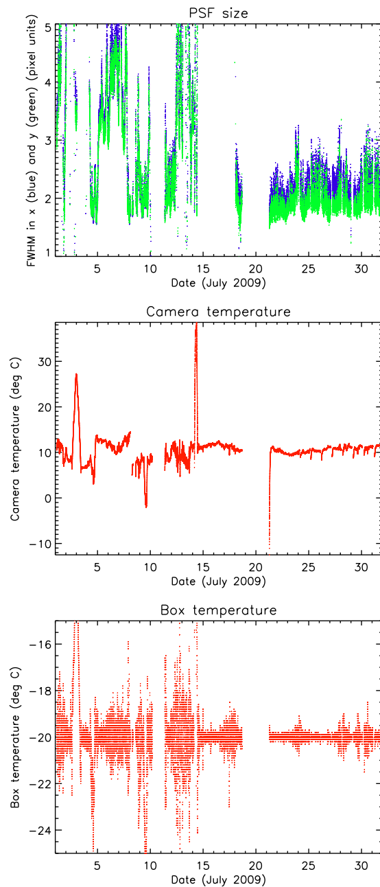
FIG. 4.31 – Taille des PSF et températures de la caméra et de l'enceinte pour le mois de juillet 2009. Les ventilateurs ont été branchés directement sur le secteur le 15, permettant une ventilation continue. La refocalisation a été effectuée le 21. Les fluctuations long terme des PSF disparaissent alors, et les températures deviennent stables.
