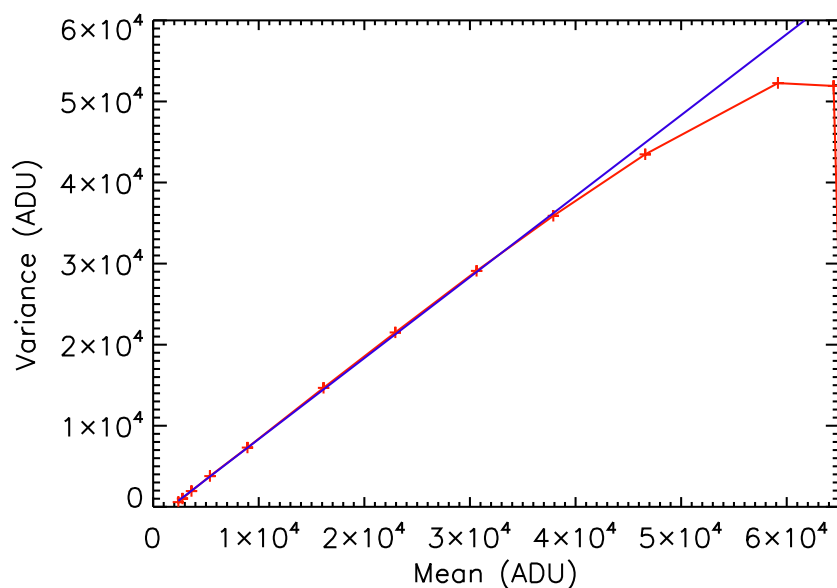
FIG. 3.5 – Mesure du gain pour la caméra ASTEP 400, ici à 600 nm et à -30^{\circ}\text{C} (rouge). Un ajustement linéaire (bleu) permet d'obtenir la valeur du gain dans la zone de linéarité et la limite de linéarité. On remarque un léger offset ; l'offset présent dans les images est étudié section 3.4.
