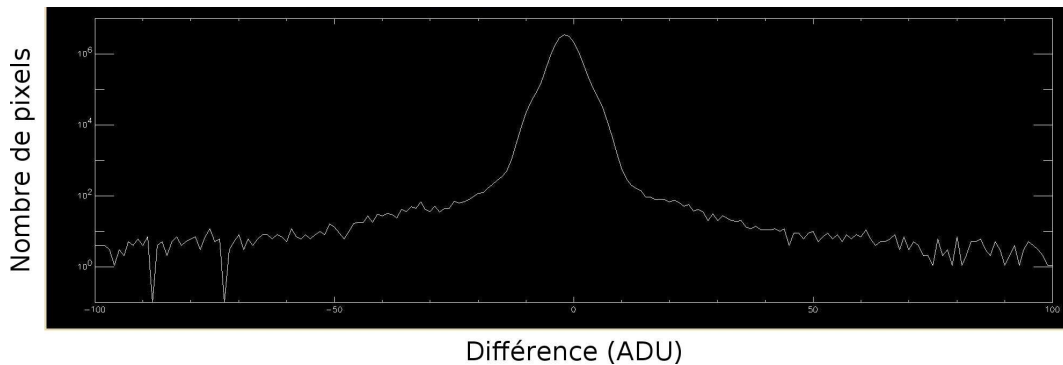
FIG. 3.14 – Histogramme de la différence de deux darks moyens réalisés à 1 mois d’intervalle, pour la caméra ASTEP Sud.
