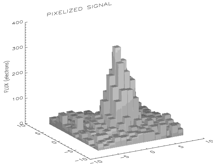
FIG. 2.15 – Signal pixélisé pour une étoile de magnitude 14, un temps de pose de 30 s et un télescope de diamètre 40 cm, accompagné des différentes sources de bruit. Cette image est sauvegardée au format FITS.
