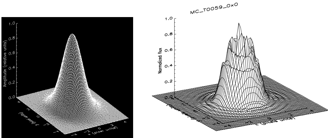
FIG. 2.11 – Exemples de PSF disponibles dans SimPhot : une PSF analytique gaussienne (gauche), et une PSF simulée par Carole Gouvret à l’aide du logiciel Zeemax (droite).
