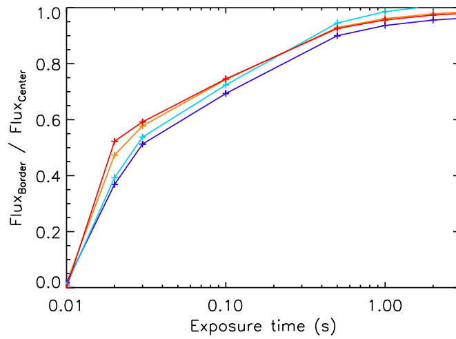
FIG. 3.18 – Rapport des flux entre le bord et le centre de l’image en fonction du temps de pose, permettant d’évaluer le temps d’ouverture du shutter sur la caméra ASTEP Sud. Les bords sont pris aux 4 coins de l’image : en haut à droite (rouge), en bas à gauche (orange), en haut à gauche (bleu foncé), en bas à droite (bleu clair).
