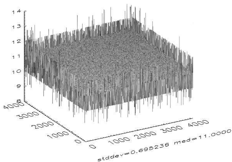
FIG. 5.9 – Soustraction de deux bias pris avec une différence de température de \sim 4^{\circ}\text{C} . La déviation standard de 0.7 ADU montre qu’il n’y a pas de dépendance spatiale de la variation du bias avec la température de l’électronique de la caméra.
