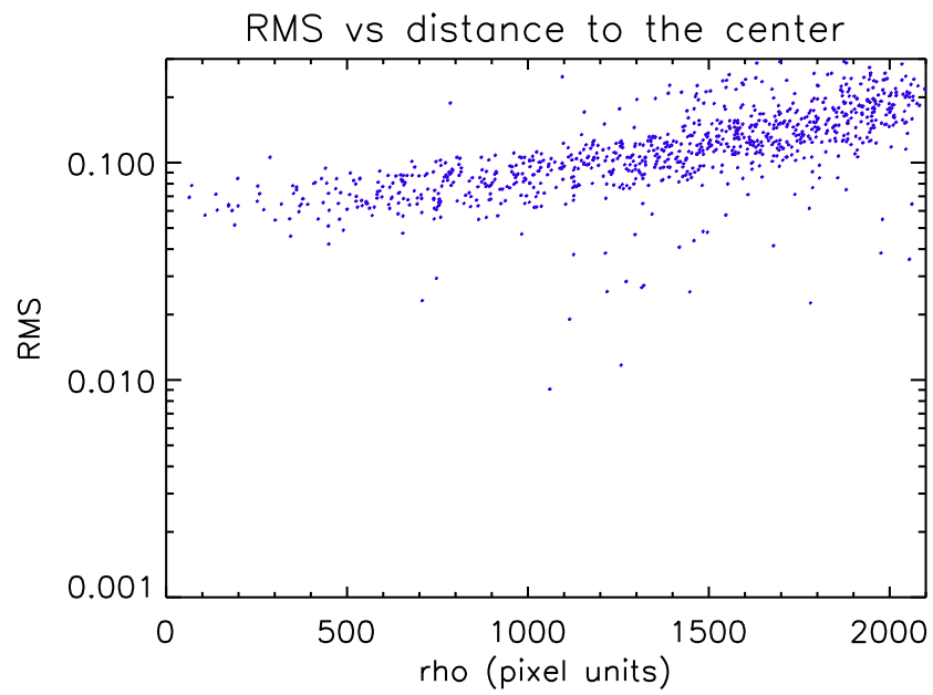
FIG. 5.16 – Niveau de bruit pour les étoiles de magnitude 13 < m_R < 13.5 en fonction de la distance radiale \rho . La dispersion augmente avec \rho , d'un facteur 4 entre le centre et le bord du champ.
