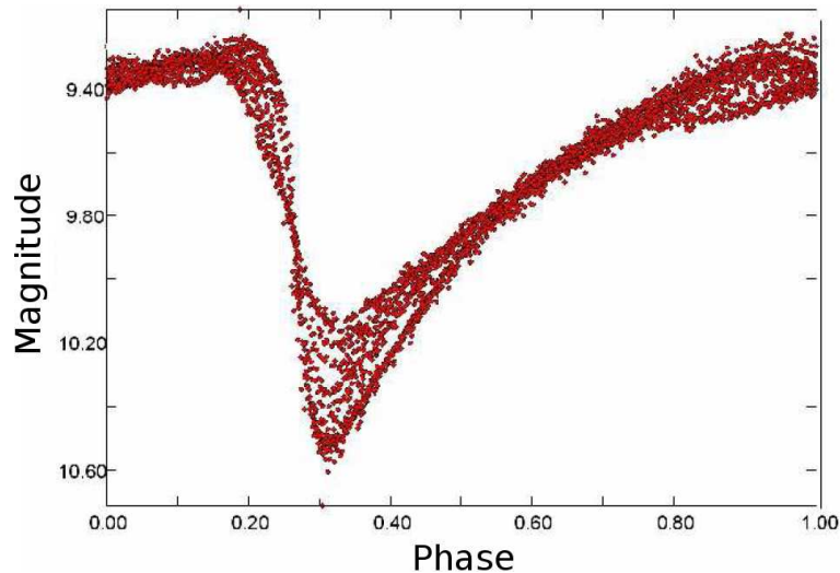
FIG. 1.19 – Courbe en phase de l'étoile pulsante S Ara obtenue par Chadid et al. [2009], à partir de 80 jours d'observations avec l'instrument PAIX durant l'hiver 2007, mettant en évidence l'effet Blazhko.
