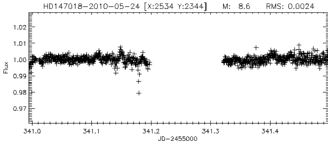
FIG. 7.30 – Courbe de lumière de HD147018 le 24 mai 2010 entre 12h et 24h UTC, avec une interruption de ~3 heures. Les observations ne montrent pas de transit.
