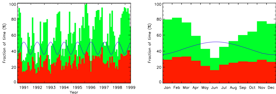
FIG. 4.28 – Statistiques mensuelles pour La Silla entre janvier 1990 et mai 1999 (gauche), et moyenne par mois sur ces 9 années, donnée à titre informatif (droite). Vert : fraction de temps photométrique f_{phot,LaSilla} ; bleu : fraction de nuit f_{nuit,LaSilla} ; rouge : fraction de temps utilisable pour les observations f_{obs,LaSilla} . On note que la fraction de temps photométrique est plus élevée d'un facteur \sim 2 pour les mois d'été que pour les mois d'hiver, les nuits sont donc beaucoup plus claires. Cependant, elles sont aussi plus courtes, et ce facteur est réduit à \sim 1.5 pour la fraction de temps utilisable. Figure réalisées à partir des données fournies par l'ESO (voir texte).
