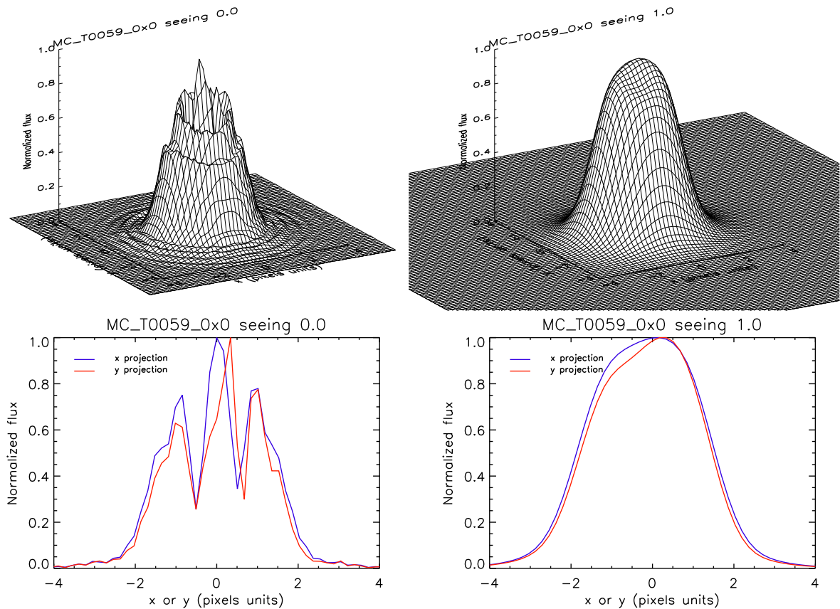
FIG. 2.13 – Exemple de PSF avant (gauche) et après (droite) convolution par un seeing de 1 arcsec, vue en 3 dimensions (haut) et en coupe (bas) selon x (bleu) et y (rouge). Le seeing est modélisé par une gaussienne de 1 arcsec de largeur à mi-hauteur.
