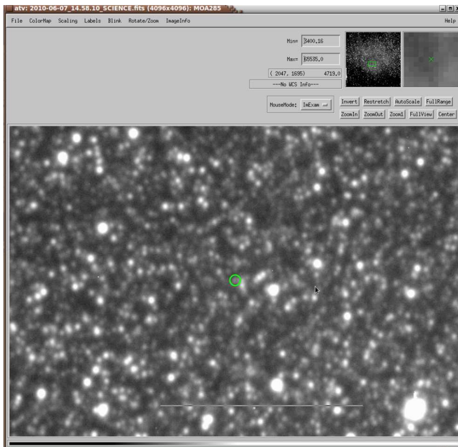
FIG. 7.27 – Image ASTEP de MOA285. La présence de la microlentille (en vert au centre de l’image) est bien mise en évidence par comparaison avec les cartes de champ.
