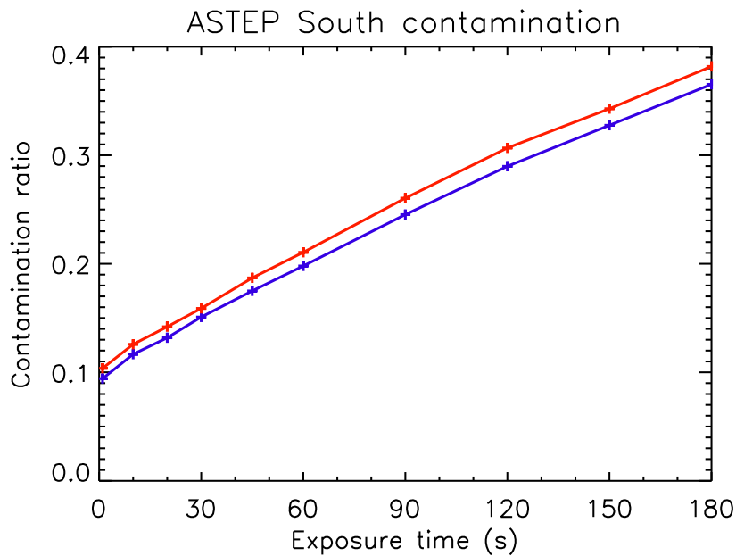
FIG. 4.10 – Facteur de contamination dans le champ ASTEP Sud en fonction du temps de pose, pour une ouverture photométrique fixe (bleu) ou variable en fonction de la magnitude (rouge). Le champ est de 3.88 \times 3.88^{\circ 2} et on considère toutes les étoiles jusqu'à magnitude 15.
