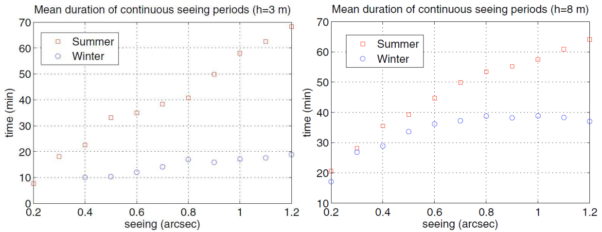
FIG. 1.17 – Durée moyenne des périodes de stabilité du seeing à 3 m (gauche) et à 8 m d'altitude (droite), en été (rouge) et en hiver (bleu). Cette durée est inférieure à la durée typique d'un transit. La photométrie pour les instruments situés dans la couche limite sera donc affectée par les variations de seeing. Figure tirée de Aristidi et al. [2009].
