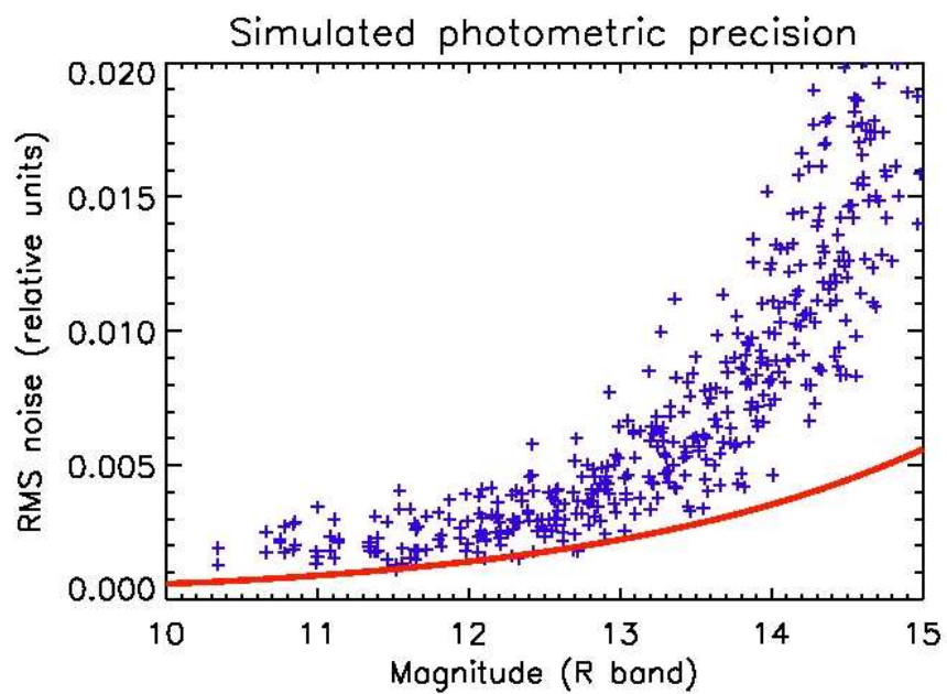
FIG. 4.5 – Bruit RMS des courbes de lumière simulées en fonction de la magnitude. Chaque étoile dans une zone de 1^{\circ 2} autour du pôle sud céleste est représentée par une croix. La courbe rouge indique le bruit de photons.
