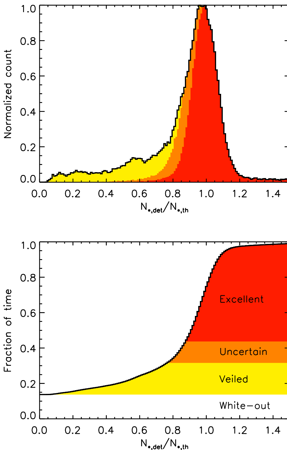
FIG. 4.27 – Haut : rapport du nombre d'étoiles mesuré sur le nombre d'étoiles théorique (ligne noire) pour l'hiver 2008, dans la 3 ème approche. Les histogrammes théoriques prenant en compte les erreurs de mesure permettent d'identifier 3 zones, correspondant au temps excellent (rouge), incertain (orange) et voilé (jaune). Bas : même histogramme représenté de manière cumulative. La zone blanche est la fraction de temps durant laquelle les acquisitions sont stoppées à cause du mauvais temps (white-out).
