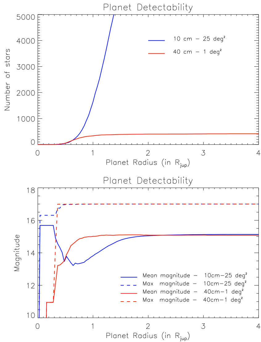
FIG. 4.3 – Haut : Nombre d'étoiles pour lesquelles une planète de rayon R_p serait détectée. Bas : Magnitudes moyenne (ligne pleine) et maximale (ligne pointillée) de ces étoiles. Les courbes rouges et bleues correspondent respectivement aux configurations 40 cm / 1° 2 et 10 cm / 25° 2 .
