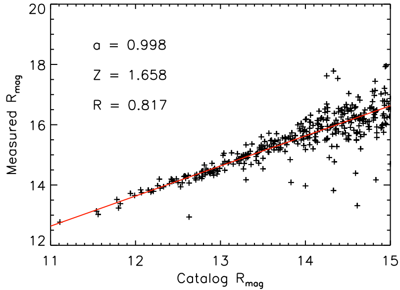
FIG. 5.21 – Comparaison entre magnitudes instrumentales et magnitudes du catalogue GSC2.2. L'ordonnée à l'origine Z de la régression linéaire permet de calibrer les magnitudes instrumentales.
