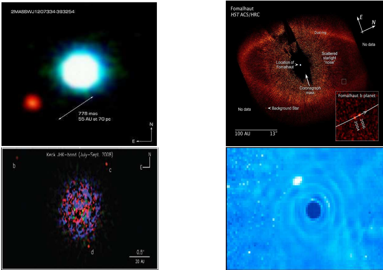
FIG. 1.4 – Coin supérieur gauche : image infrarouge de l'étoile 2M1207 (en bleu) et de son compagnon planétaire 2M1207b (en rouge), prise par Chauvin et al. [2004] avec le télescope Yepun de 8.2 m de l'ESO. Coin supérieur droit : Première photographie optique d'une planète extrasolaire, Fomalhaut b, prise par Kalas et al. [2008] avec le coronographe du télescope spatial Hubble. Coin inférieur droit : Combinaison de trois images du système planétaire autour de HR8799, prises en bande J, H et K par Marois et al. [2008] avec le télescope KECK. Coin inférieur gauche : Image infrarouge de \beta Pictoris prise par Lagrange et al. [2009] avec l'instrument NaCo du télescope Yepun de 8.2 m de l'ESO ; après traitement, on distingue un compagnon très probablement planétaire dans le coin supérieur gauche du disque entourant l'étoile.
