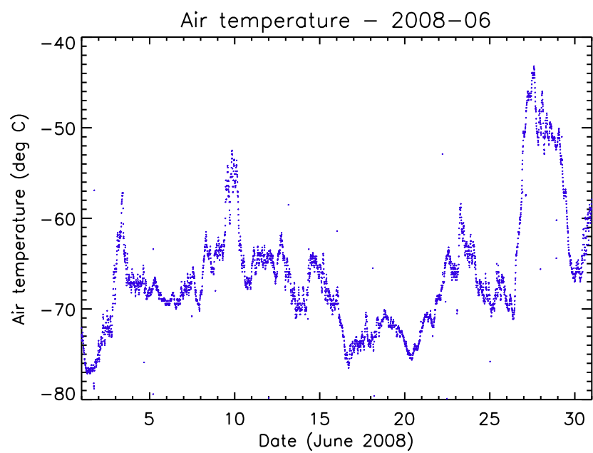
FIG. 1.18 – Mesures de température au niveau du sol au Dôme C, obtenues par la station météorologique AWS (Automatic Weather Station), pour le mois de juin 2008. On note une montée rapide de la température avec une augmentation de plus de 25°C en une journée, autour du 27 juin. Ce type de courbe est caractéristique des mesures obtenues durant la période hivernale.
