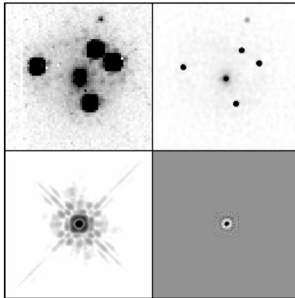
FIG. 2.10 – Exemple de traitement par déconvolution d'une image de la lentille gravitationnelle WFI2033-4723 (en haut à gauche). L'algorithme de déconvolution calcule le noyau de la PSF (en bas à gauche), et permet d'obtenir une image déconvoluée (en haut à droite). Une composante numérique (en bas à droite) est ici ajoutée à la PSF. Figure tirée de Magain et al. [2007].
