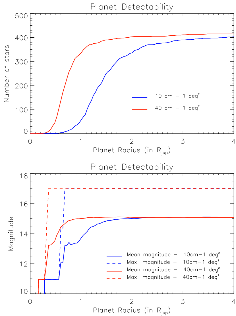
FIG. 4.4 – Haut : Nombre d'étoiles pour lesquelles une planète de rayon R_p serait détectée. Bas : Magnitudes moyenne (ligne pleine) et maximale (ligne pointillée) de ces étoiles. Les courbes rouges et bleues correspondent respectivement aux 40 cm et 10 cm, avec un champ identique de 1^{\circ 2} .
