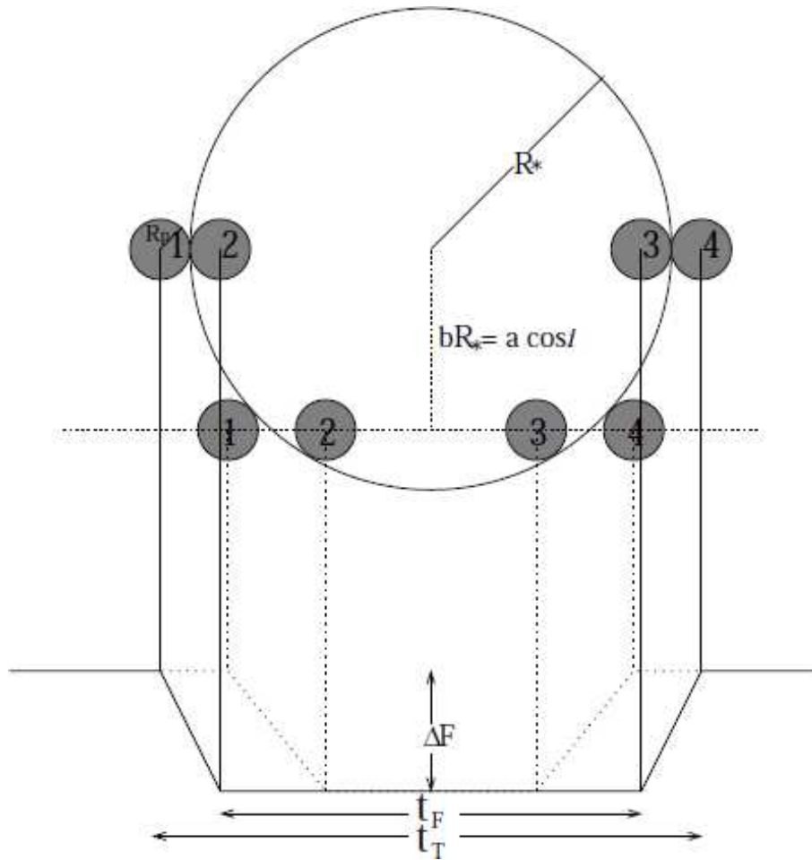
FIG. 1.8 – Définition des observables d’une courbe de transit. Deux géométries possibles du système étoile-planète sont illustrées, et les courbes de lumière correspondantes (shématiques) sont représentées en-dessous. On indique pour la courbe en ligne pleine : la profondeur du transit \Delta F , la durée totale du transit t_T , et la durée entre la fin de l’entrée et le début de la sortie du transit (la partie “plate” de la courbe, lorsque la planète est totalement superposée à l’étoile). Les chiffres représentent les différents contacts pour une planète se déplaçant de gauche à droite. On indique également R_* , R_p , le paramètre d’impact b , et l’inclinaison correspondante i . Différents paramètres d’impact (ou inclinaisons) vont donner différentes courbes, comme le montrent les lignes pleine ( b = 0 ) et pointillée ( b quelconque). Figure tirée de Seager & Mallén-Ornelas [2003].
