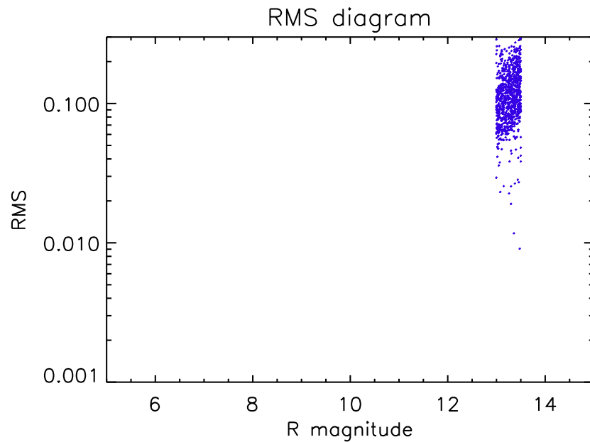
FIG. 5.15 – Diagramme RMS-magnitude restreint à la plage 13 < m_R < 13.5 .
