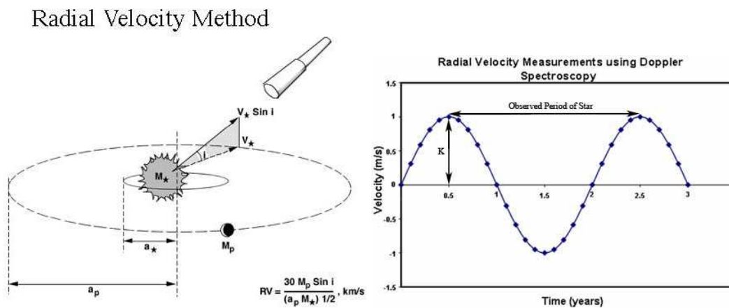
FIG. 1.1 – Détection d'une planète extrasolaire par vitesses radiales. L'étoile et la planète sont en mouvement autour du barycentre du système (gauche), et l'amplitude K de la courbe de vitesses radiales (droite) permet de connaître la masse de la planète à un facteur \sin i près.
