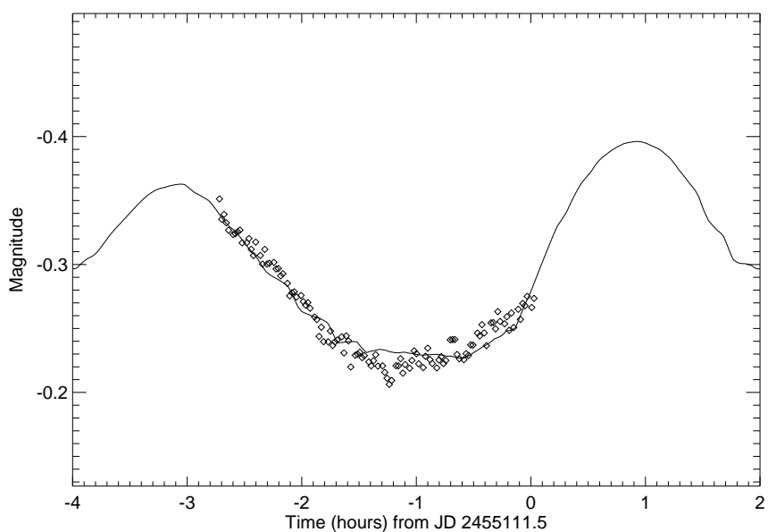
FIG. 7.7 – Courbe de lumière de l’astéroïde (41) Daphne (losanges), obtenue durant 3 heures d’observations dans la nuit du 6 au 7 octobre 2009, avec le télescope ASTEP400. Un ajustement (ligne continue) permet de déduire la phase rotationnelle.
