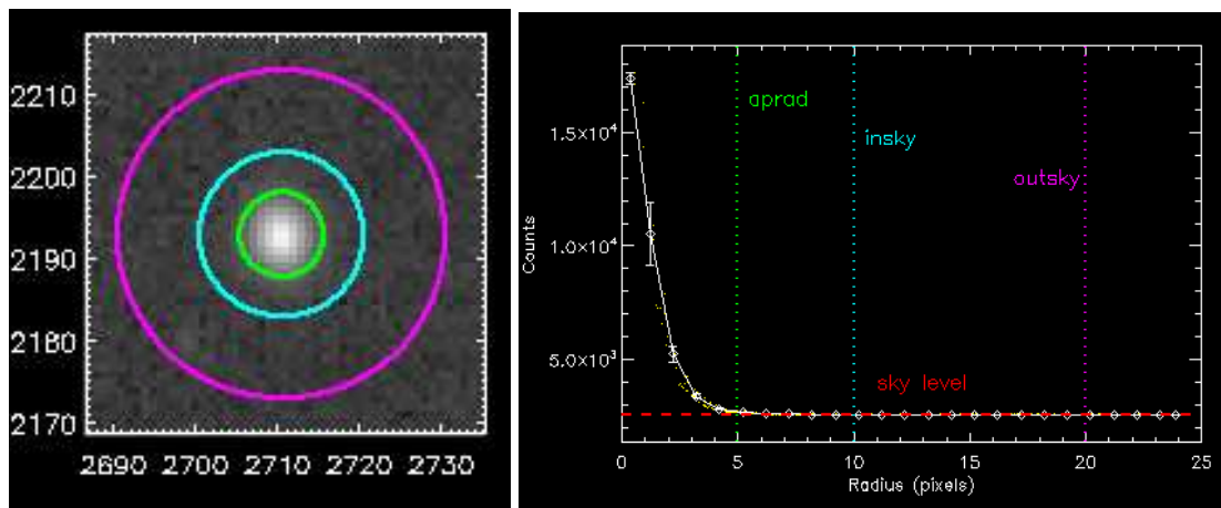
FIG. 2.8 – Principe de la photométrie d’ouverture effectuée par la routine APER, sur l’image (gauche), et en coupe (droite). L’étoile est ici au pixel (2712,2193) du CCD. Le niveau de fond de ciel (ligne pointillée rouge) est calculé dans une couronne autour de la cible (délimitée par les cercles bleu et violet), puis soustrait. Le flux est alors mesuré dans une ouverture circulaire (cercle vert). Images réalisées à partir du logiciel ATV 1 [Barth, 2001].
