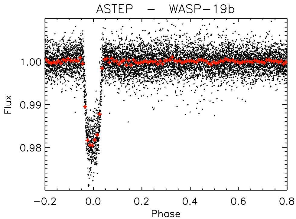
FIG. 7.21 – Courbe de lumière de WASP-19 en phase, à partir des 24 jours d’observations (~30 périodes). Une moyenne par intervalle de 1/100^{\text{ème}} de période, soit 11 mn, est représentée en rouge.
