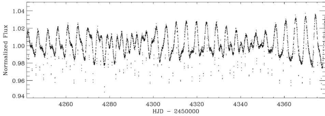
FIG. 2.1 – Courbe de lumière de CoRoT-2 sur \sim 150 jours, montrant une forte activité stellaire et 78 transits d’un compagnon planétaire. Figure tirée de Alonso et al. [2008].
