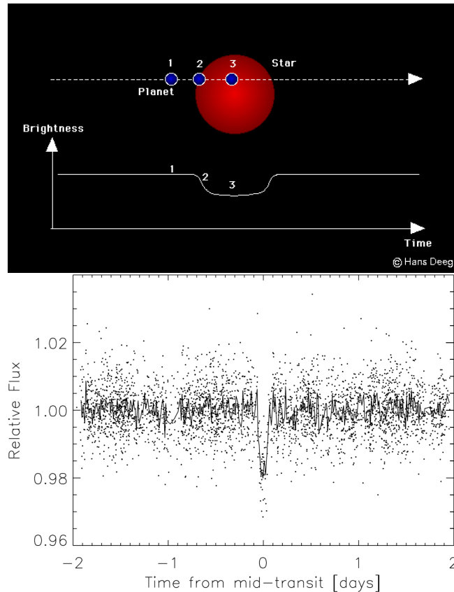
FIG. 1.7 – Haut : principe de la photométrie des transits. Le flux reçu diminue lorsque la planète passe devant son étoile. Bas : courbe de lumière de l'étoile XO-1, qui montre la présence de la planète XO-1b [McCullough et al., 2006]. Plus de 3000 points ont été obtenus au cours des années 2004 et 2005, puis sont mis en phase. La période de la planète est de 3.94 jours. La courbe continue est une moyenne glissante sur 15 mn.
