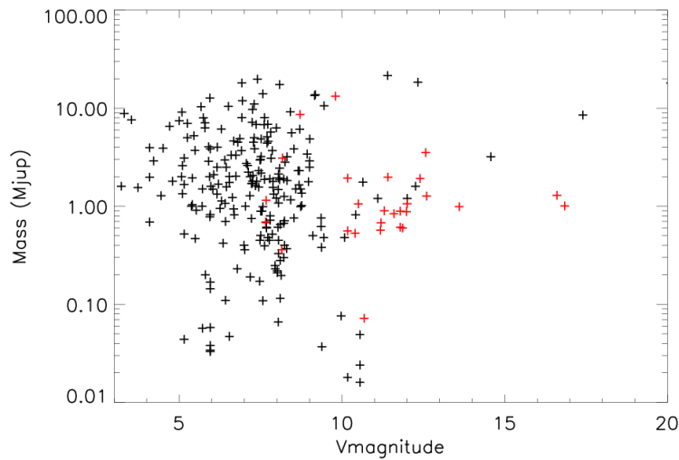
FIG. 6.17 – Distribution en magnitude des exoplanètes connues au moment de l'étude du guidage. Les planètes en transit sont représentées en rouge et celle découvertes par vitesses radiales en noir.
