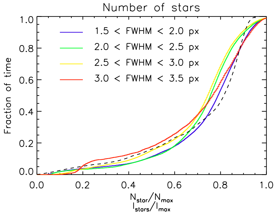
FIG. 4.20 – Histogramme cumulé du nombre d'étoiles détectées sur les images ASTEP Sud pour un FWHM compris entre 1.5 et 2 px (bleu), 2 et 2.5 px (vert), 2.5 et 3 px (jaune), et 3 et 3.5 px (rouge), et de l'intensité des 10 étoiles les plus brillantes (noir). Les histogrammes sont en bon accord. Cette 1 ère approche permet de déduire la fraction de temps photométrique pour l'hiver 2008 au Dôme C à l'aide d'un critère ad hoc .
