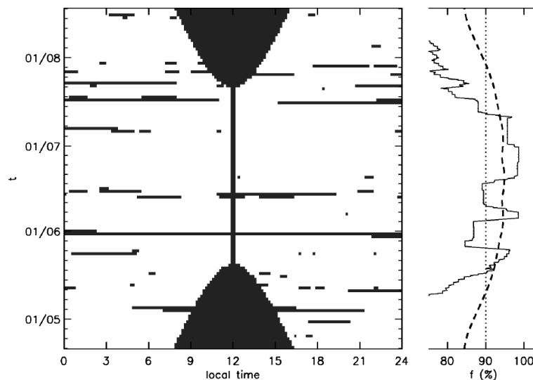
FIG. 1.13 – Fenêtres d'observation pour l'hiver 2006, prenant en compte la présence de nuages et l'illumination du fond de ciel par le Soleil autour de midi, obtenues par Mosser & Aristidi [2007]. Pour une hauteur du Soleil inférieure à 4^\circ sous l'horizon, la fraction de temps utilisable est de 88.5 %.
