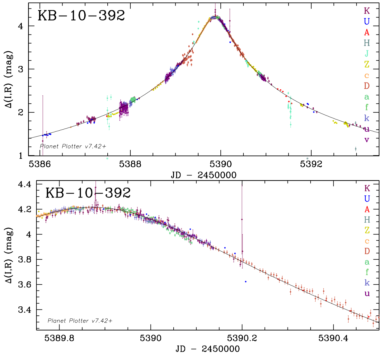
FIG. 7.29 – Courbe d’amplification de MOA392 obtenue en combinant les données de différents télescopes, représentés par différentes couleurs. Les données ASTEP sont en marron (lettre “D”). Haut : courbe globale. Bas : zoom après le maximum d’amplification. Les données ASTEP complètent bien celles des autres télescopes. Courbes fournies par Christian Coutures.
