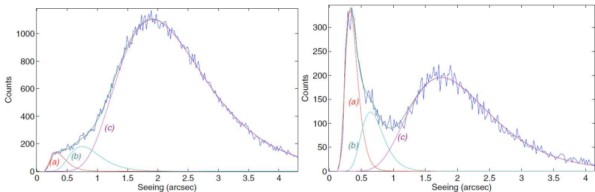
FIG. 1.16 – Histogrammes des mesures de seeing obtenues lors de l’hiver 2006 à 3 m (gauche) et à 8 m d’altitude (droite). Les mesures sur 3 hivers donnent une médiane de 2.37 arcsec à 3 m et de 1.65 arcsec à 8 m. A 8 m, on observe un comportement bimodal. Figure tirée de Aristidi et al. [2009].
