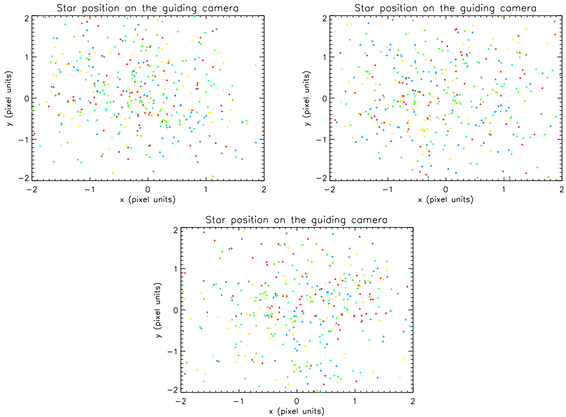
FIG. 6.25 – Position du centre de l'étoile guide sur des images simulées par SimPhot pour des PSF de différentes focalisations : -100 (bleu), -50 (turquoise), 0 (vert), +50 (jaune) et +100 (rouge) \mu\text{m} , pour une étoile de magnitude 8 (haut gauche), 10 (haut droite) et 12 (bas), et pour des déplacements du télescope 3 fois plus grands que les déplacements standard.
