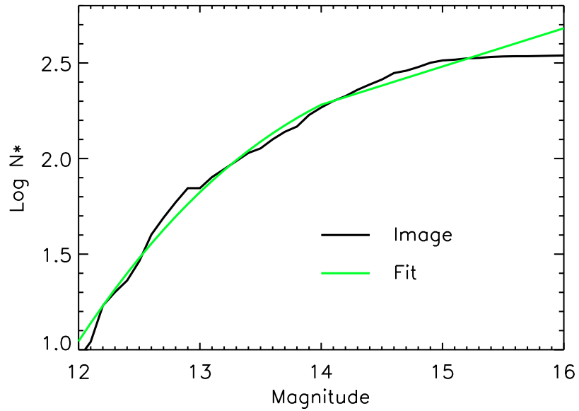
FIG. 4.25 – Diagramme cumulatif du nombre d'étoiles en fonction de magnitude instrumentale sur une image prise lorsque le temps est excellent (noir), et ajustement par un polynôme d'ordre 3 (vert), utilisé dans la 3 ème approche, pour l'hiver 2008.
