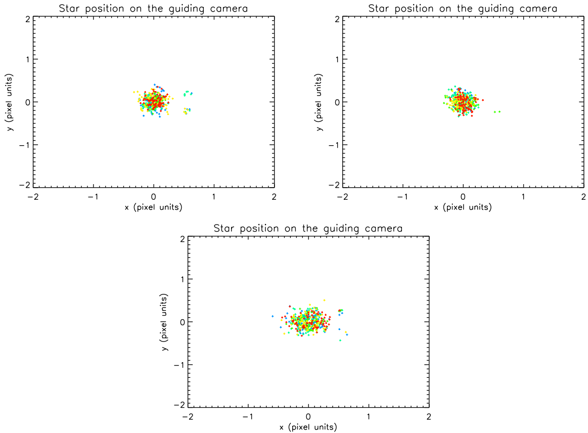
FIG. 6.24 – Position du centre de l'étoile guide sur des images simulées par SimPhot pour des PSF de différentes focalisations : -100 (bleu), -50 (turquoise), 0 (vert), +50 (jaune) et +100 (rouge) \mu\text{m} , pour une étoile de magnitude 8 (haut gauche), 10 (haut droite) et 12 (bas), et pour des déplacements du télescope 3 fois plus petits que les déplacements standard.
