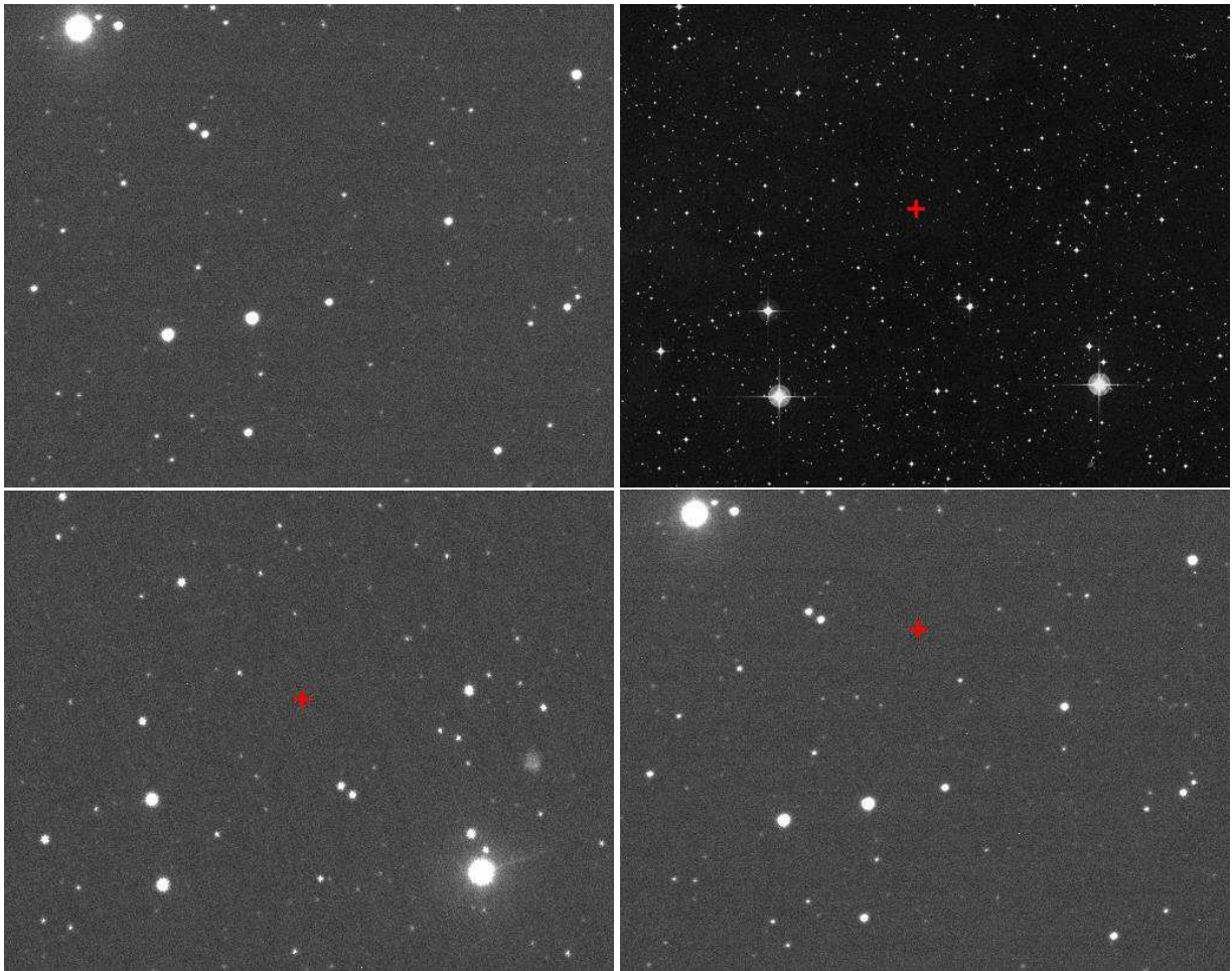
FIG. 4.13 – Principe de la reconnaissance de champ. On cherche la transformation qui permet de faire correspondre l’image ASTEP Sud (haut gauche) à un catalogue standard (haut droite, ici représenté par une image du Digitized Sky Survey). Une fois la transformation trouvée (bas gauche), on détermine la position du pôle sur l’image initiale par l’inverse de cette transformation appliquée au pixel (2048,2048) (bas droite). Le pôle sud est représenté par une croix rouge.
