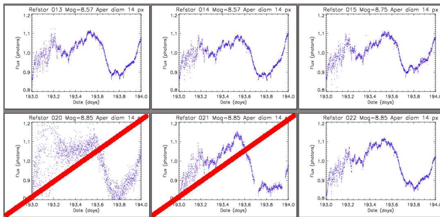
FIG. 5.22 – Sélection des étoiles de référence. On élimine celles dont la courbe de lumière n'est pas satisfaisante (dispersion anormalement élevée ou forme différente des autres).
