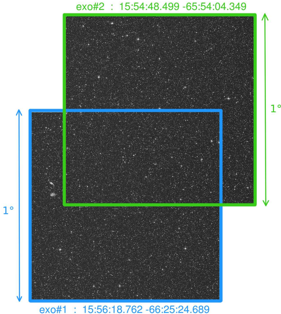
FIG. 7.16 – Champs exo#1 et exo#2 observés par ASTEP400, dédiés à la recherche de nouvelles planètes en transits.
