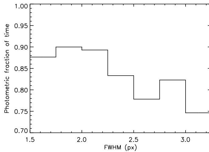
FIG. 4.23 – Fraction de temps photométrique en fonction du FWHM, dans la 2 nde approche. On voit clairement une dépendance. (Les périodes de white-out ne sont ici pas prises en compte.)
