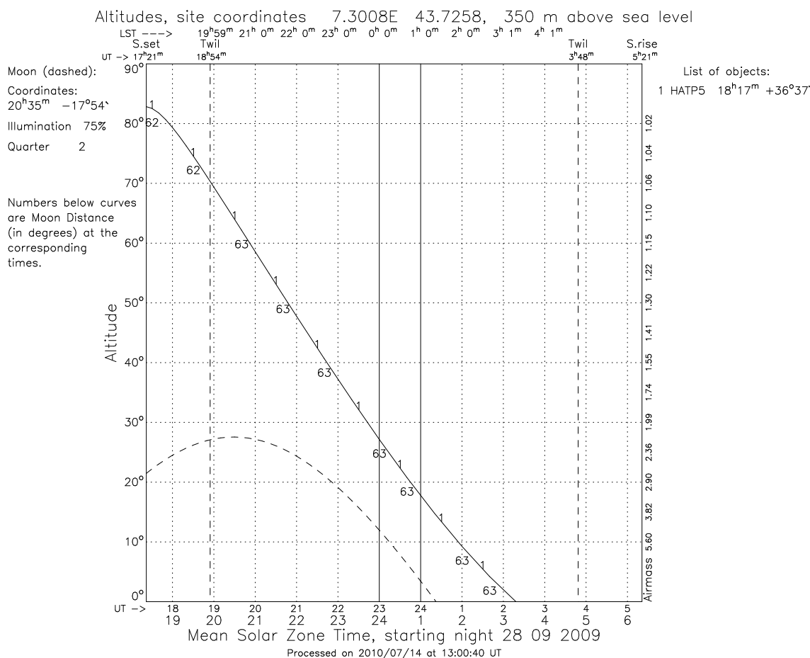
FIG. 7.3 – Altitude de HAT-P-5 au cours de la nuit du 28 septembre 2009, observée depuis l’observatoire de Nice (ligne pleine). La cible est au-dessus de 30° jusqu’à 22h30 UT, soit 0h30 heure de Nice. Figure réalisée à partir de http://catserver.ing.iac.es/staralt/ .
