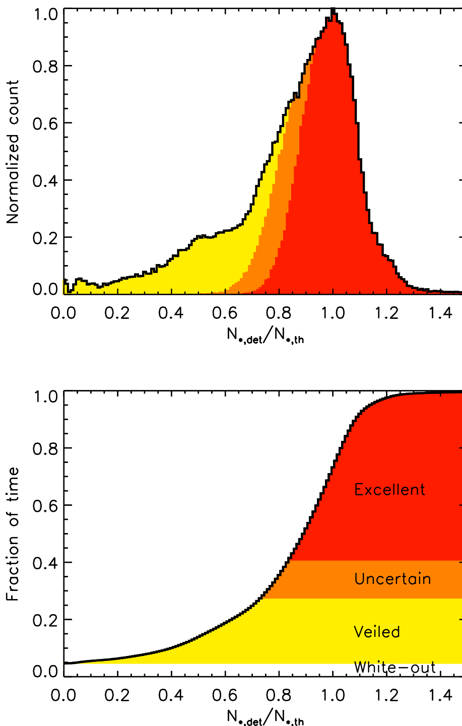
FIG. 4.35 – Haut : rapport du nombre d'étoiles mesuré sur le nombre d'étoiles théorique (ligne noire) pour l'hiver 2009. Les histogrammes théoriques prenant en compte les erreurs de mesure permettent d'identifier 3 zones, correspondant au temps excellent (rouge), incertain (orange) et voilé (jaune). Bas : même histogramme représenté de manière cumulative. La zone blanche est la fraction de temps durant laquelle les acquisitions ont été stoppées à cause du mauvais temps (white-out).
