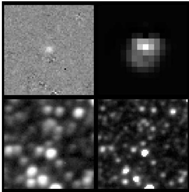
FIG. 2.9 – Principe de la photométrie de soustraction. L'image originale est en bas à gauche, et l'image de référence en bas à droite. Un ajustement permet de déterminer le noyau de convolution entre les deux images, représenté en haut à gauche. La différence entre l'image ainsi reconstruite et l'image originale permet alors d'identifier les variations de flux, en haut à droite (zoom sur l'étoile centrale). Figure tirée de Alard & Lupton [1998].
