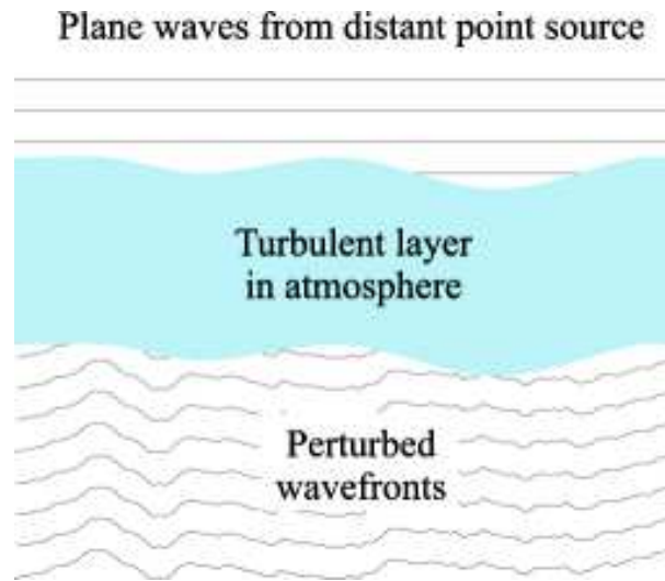
FIG. 2.2 – Déformation du front d’onde par une atmosphère turbulente.
