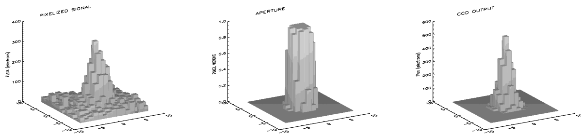
FIG. 2.16 – Photométrie d’ouverture effectuée par SimPhot, dans le cas d’une ouverture circulaire, pour une étoile de magnitude 14, un temps de pose de 30 s et un télescope de diamètre 40 cm. L’image initiale (a) est multipliée par une ouverture, par exemple circulaire avec un poids pour les pixels de bord (b), pour extraire le signal de l’étoile cible (c).
