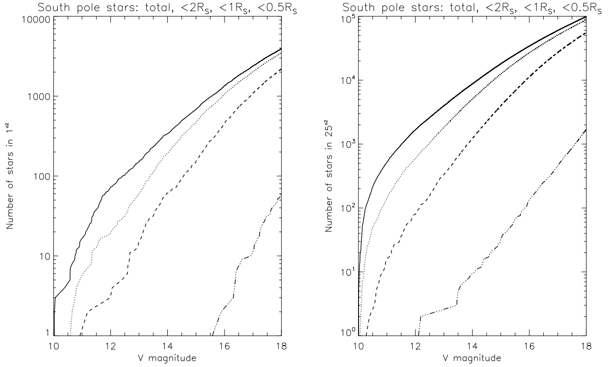
FIG. 4.2 – Distribution en magnitude des étoiles dans un champ centré sur le pôle sud, à partir du modèle de Besançon. Gauche : champ de 1^{\circ 2} , droite : champ de 22^{\circ 2} (dû à un effet de projection, ce champ est légèrement plus petit que 25^{\circ 2} ). Les courbes indiquent le nombre total d'étoiles dans le champ (ligne pleine), ainsi que le nombre d'étoiles de rayon R \leq 2R_{\odot} (points), R \leq R_{\odot} (traits), et R \leq 0.5R_{\odot} (traits-points)
