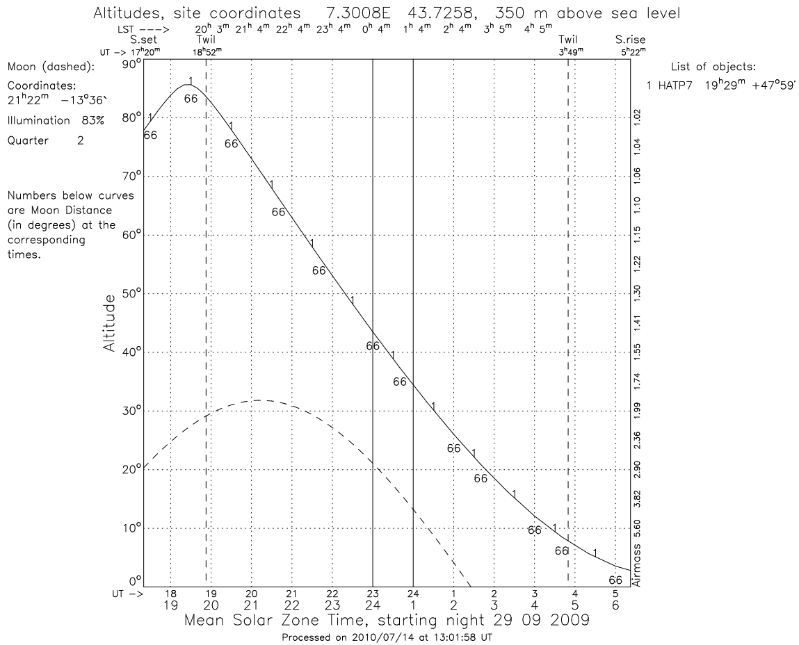
FIG. 7.5 – Altitude de HAT-P-7 au cours de la nuit du 29 septembre 2009, observée depuis l’observatoire de Nice (ligne pleine). La cible est au-dessus de 30° jusqu’à 0h30 UT, soit 2h30 heure de Nice. Figure réalisée à partir de http://catserver.ing.iac.es/staralt/ .
