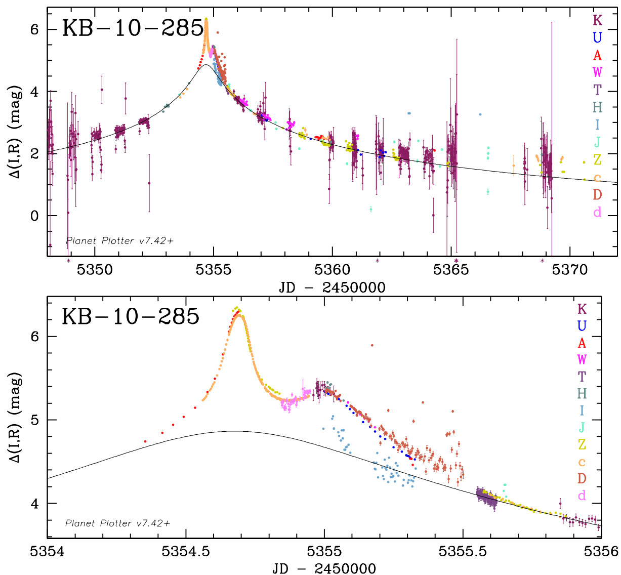
FIG. 7.28 – Courbe d’amplification de MOA285 obtenue en combinant les données de différents télescopes, représentés par différentes couleurs. Les données ASTEP sont en marron (lettre “D”). Haut : courbe globale, sur laquelle on observe une déformation. Bas : zoom sur la partie déformée. Les données ASTEP complètent bien celles des autres télescopes. Les modèles d’ajustement de la courbe permettent d’identifier un compagnon de type naine brune. Courbes fournies par Christian Coutures.
