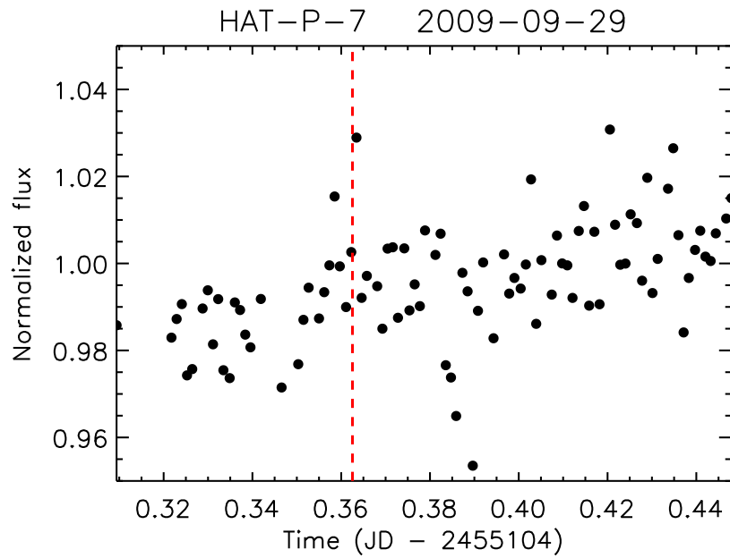
FIG. 7.6 – Courbe de lumière obtenue lors du transit de HAT-P-7b, par photométrie de soustraction. La fin du transit est représentée par la ligne pointillée rouge. La dispersion hors-transit est de 1.3%.
