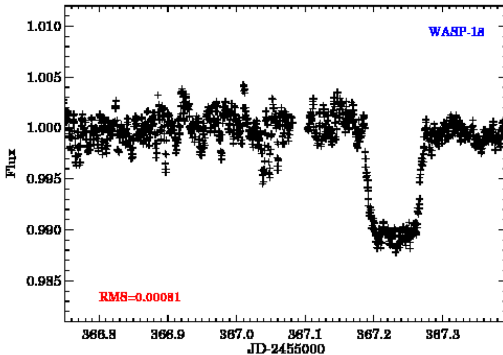
FIG. 7.22 – Courbe de lumière de WASP-18 pour la journée du 19 juin 2010. Les poses sont de 15 s. La précision est de 810 ppm.
