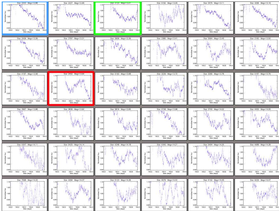
FIG. 5.25 – Exemples de courbes de lumière obtenues après une moyenne glissante sur 30 mn, sur la journée du 12 juillet 2008. On met en évidence des variations à long terme sur la journée. Plusieurs formes apparaissent fréquemment, encadrées en bleu, vert et rouge.
