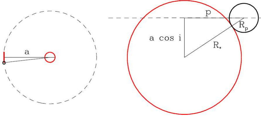
FIG. 1.6 – La durée d'un transit est obtenue à partir de la fraction de l'orbite durant laquelle la planète cache une partie du disque stellaire, projeté en rouge (gauche). La projection de l'arc orbital parcouru durant le transit peut alors être calculée (droite). Figure adaptée de Sackett [1999].
