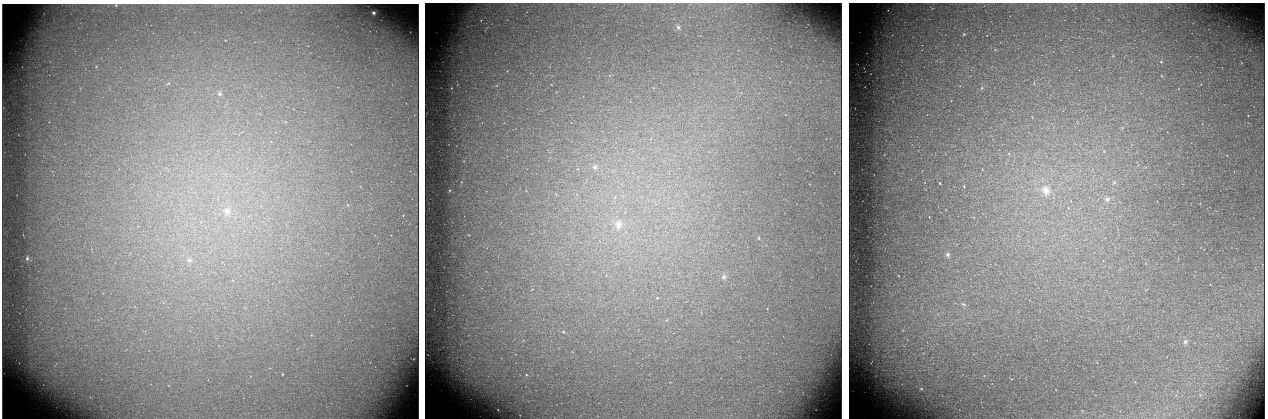
FIG. 5.1 – Images ASTEP Sud du 12 juillet 2008, à 0h (gauche), 8h (milieu) et 16h (droite) UTC. Les étoiles effectuent une rotation sur le CCD en \sim 24 h.
