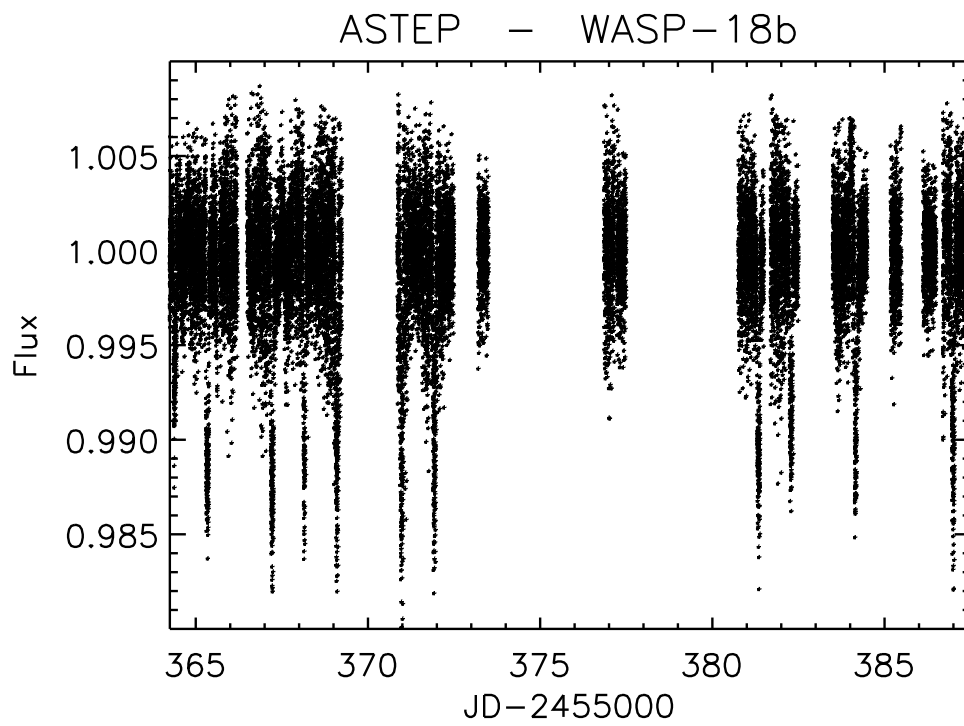
FIG. 7.23 – Courbe de lumière de WASP-18 sur toute la durée des observations, soit entre le 16 juin et le 9 juillet 2010.
