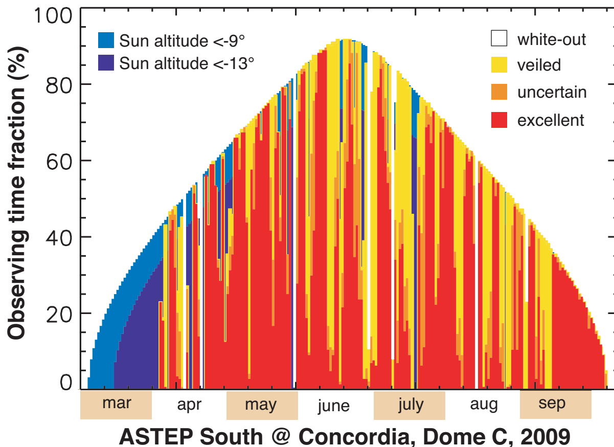
FIG. 4.36 – Fraction de temps d'observation par jour avec ASTEP Sud pour l'hiver 2009. Les zones bleu clair et bleu foncé indiquent la fraction du temps pour laquelle le Soleil est plus bas que -9 et -13^\circ sous l'horizon, respectivement. Les périodes de temps excellent, incertain et voilé déterminées par ASTEP Sud sont en rouge, orange et jaune, respectivement. Les zones blanches correspondent aux périodes durant lesquelles les observations sont stoppées à cause du mauvais temps (white-out). Les données acquises entre le 4 et le 27 avril ne sont pas encore récupérées.
