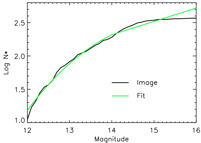
FIG. 4.32 – Diagramme cumulatif du nombre d'étoiles en fonction de magnitude instrumentale sur une image prise lorsque le temps est excellent (noir), et ajustement par un polynôme d'ordre 3 (vert), pour l'hiver 2009.
