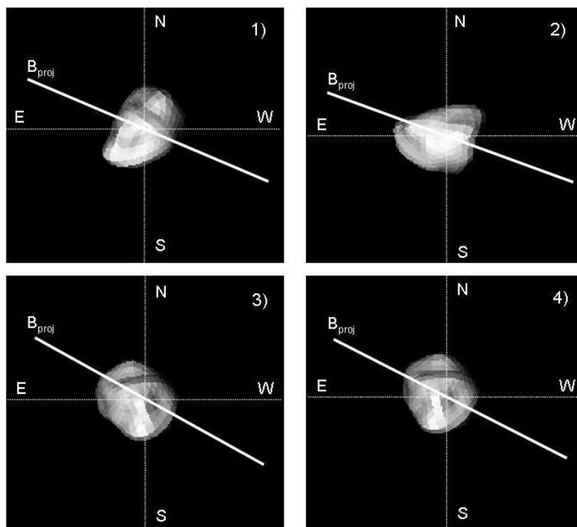
FIG. 7.8 – Images de l’astéroïde (41) Daphne synthétisées par le modèle thermophysique, avec un modèle de forme concave. L’orientation de la ligne de base projetée sur le plan du ciel pour différentes observations VLTI est représentée par une ligne blanche.
