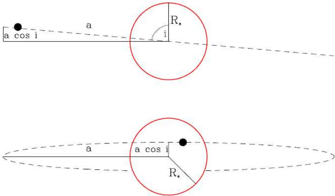
FIG. 1.5 – Géométrie d'un transit, avec a le demi-grand axe orbital, i l'inclinaison, et R_* le rayon de l'étoile, vu de côté (haut) et vu par l'observateur (bas). La planète est en noir et l'étoile en rouge. Figure adaptée de Sackett [1999].
