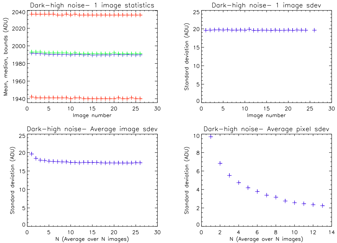
FIG. 3.11 – Statistiques sur les images de dark de 30 s prises en lecture rapide pour la caméra ASTEP 400. Moyenne (bleu), médiane (vert), et intervalle contenant 99 % des pixels (rouge), pour chacune des ~30 images (haut gauche), déviation standard pour chacune des ~30 images (haut droite), déviation standard d’une image moyenne faite à partir de N images (bas gauche), et déviation standard par pixel sur plusieurs images moyennes de N images (bas droite).
