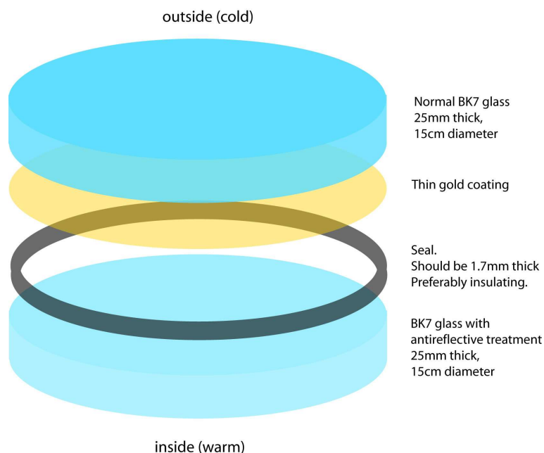
FIG. 6.7 – Schéma du hublot utilisé pour les enceintes thermalisées d’ASTEP Sud et ASTEP 400 (dans le cas d’un hublot plan). Le double vitrage avec une couche réfléchissante sur une des faces permet une très bonne isolation thermique.
