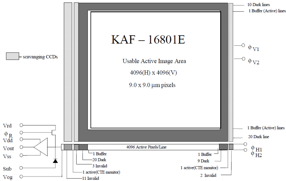
FIG. 3.2 – Schéma de principe du CCD Kodak KAF-16801E de la caméra de classe C1. La caméra de classe C2 ne possède pas de colonnes et de lignes en dehors de la zone sensible.
