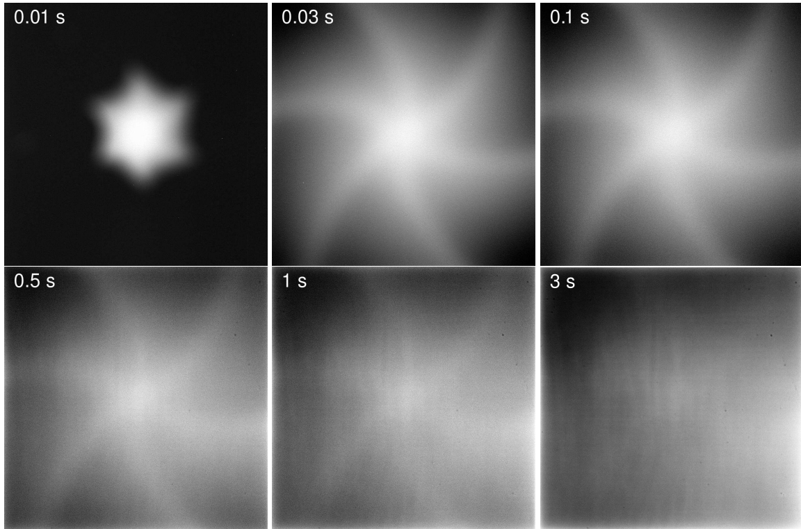
FIG. 3.17 – Images avec des temps de pose courts montrant l'ouverture du shutter. Pour cette visualisation, l'échelle est étalée entre le minimum et le maximum de l'image.
