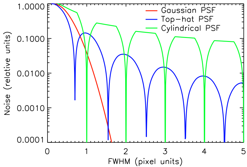
FIG. 2.18 – Bruit de jitter lié aux électrodes pour différentes formes de PSF : gaussienne (rouge), top-hat (bleu) et cylindrique (vert). Le bruit devient négligeable pour une PSF gaussienne de FWHM > 1.7 px, et reste élevé pour les deux autres PSF (sauf pour certaines valeurs singulières de FWHM).
