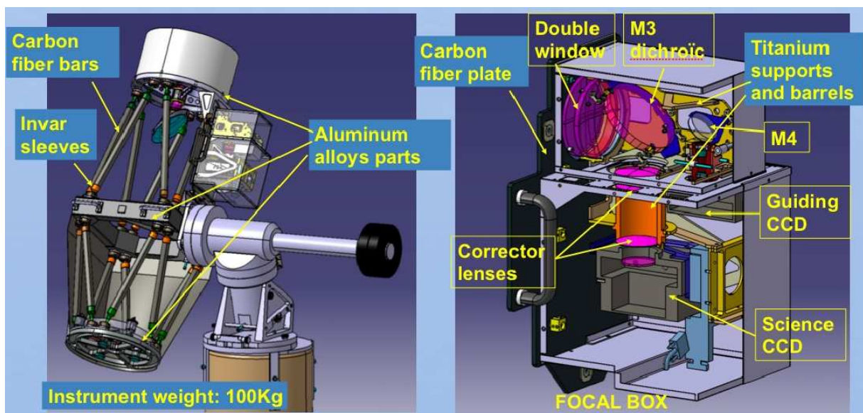
FIG. 6.4 – Vue d'ensemble de la structure mécanique du télescope ASTEP400 (gauche) et de la boîte caméra (droite).
