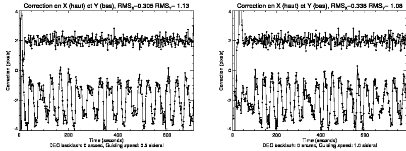
FIG. 7.1 – Correction appliquée en X et Y, équivalente à la distance au point de fonctionnement, pour une étoile à 45° de déclinaison, avec différents paramètres pour la vitesse de guidage : 0.5 s (gauche) et 1 s (droite). Le backlash n'est pas compensé. Les courbes sont centrées sur \pm 2 px pour une bonne lisibilité.
