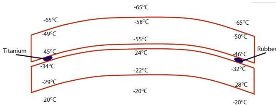
FIG. 6.8 – Température des différentes couches et interfaces du hublot double vitrage, dans la configuration thermique envisagée à Concordia (température extérieure : -65^{\circ}\text{C} , température de l’enceinte : -20^{\circ}\text{C} ).
