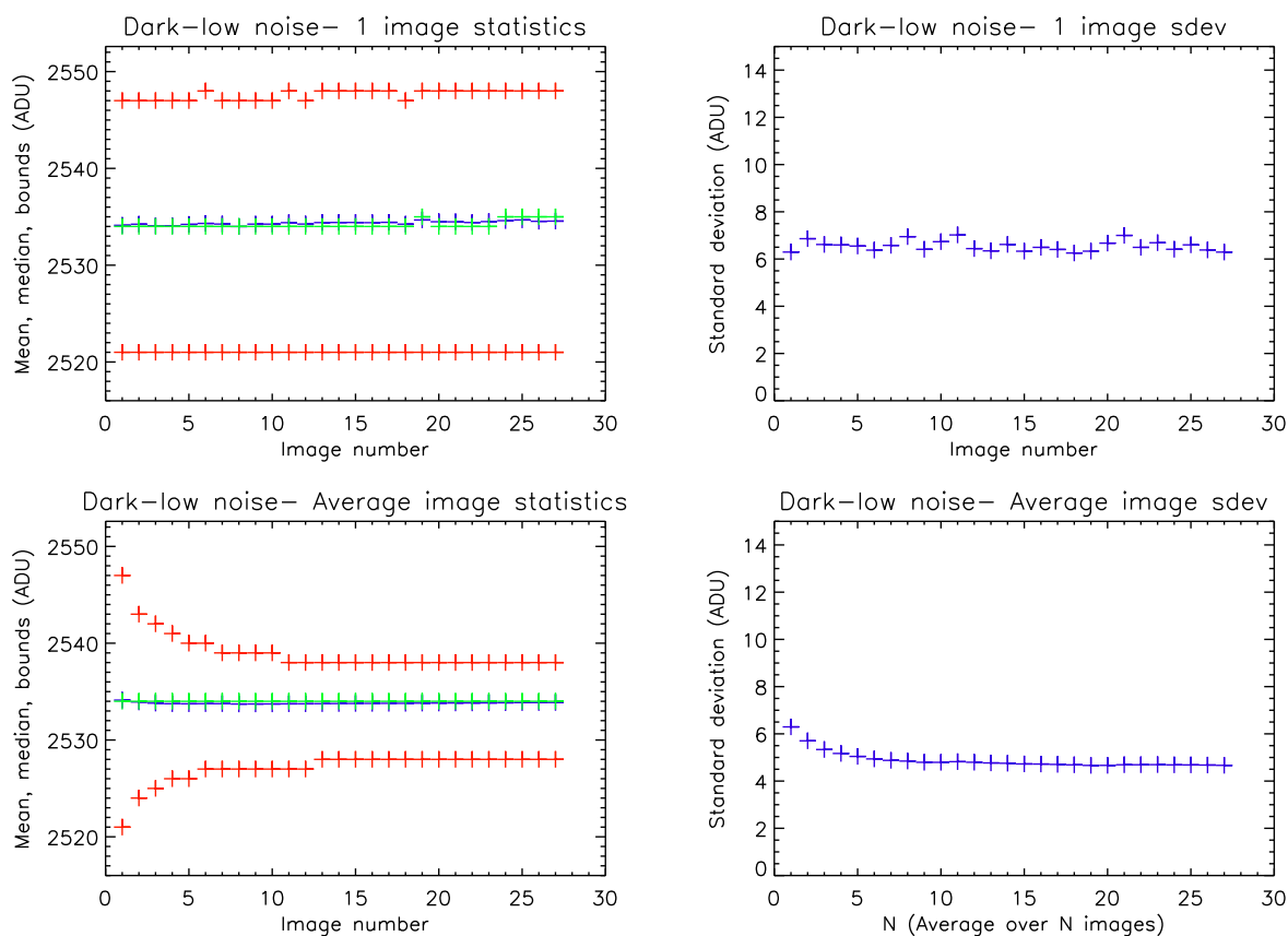
FIG. 3.13 – Statistiques sur les images de dark de 30 s prises en lecture rapide pour la caméra ASTEP Sud. Moyenne (bleu), médiane (vert), et intervalle contenant 99 % des pixels (rouge), pour chacune des \sim 30 images (haut gauche), déviation standard pour chacune des \sim 30 images (haut droite), déviation standard d’une image moyenne faite à partir de N images (bas gauche), et déviation standard par pixel sur plusieurs images moyennes de N images (bas droite).
