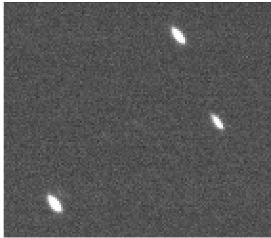
FIG. 5.2 – Portion d’image de 150 \times 150 px centrée sur le pixel (3655,3610) montrant l’étalement des PSF en bord de champ.
