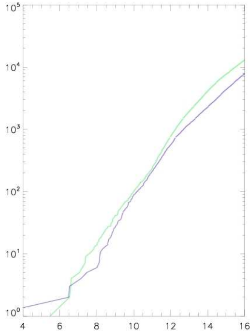
FIG. 4.14 – Distribution d'étoiles dans les champs centrés sur les pôles nord (bleu) et sud (vert). Le nombre d'étoiles par magnitude est du même ordre de grandeur dans les deux champs.
