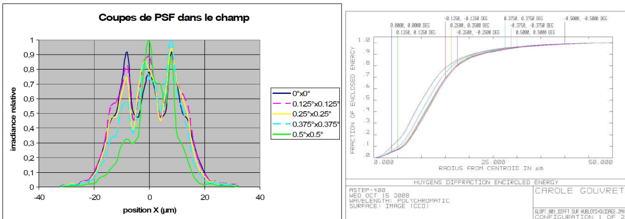
FIG. 6.2 – PSF finale vue en coupe selon la direction x (gauche), et énergie intégrée en fonction du rayon d'intégration (droite), en différents points de la diagonale du champ : 0^\circ (bleu foncé), 0.125^\circ (rose), 0.25^\circ (jaune), 0.375^\circ (bleu clair), 0.5^\circ (vert).
