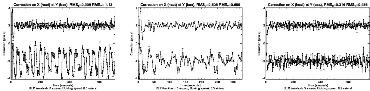
FIG. 7.2 – Correction appliquée en X et Y, équivalente à la distance au point de fonctionnement, pour une étoile à 45° de déclinaison, avec différents paramètres pour la compensation du backlash en déclinaison : 0 arcsec (gauche), 3 arcsec (milieu) et 5 arcsec (droite). La vitesse de guidage est de 0.5 s. Les courbes sont centrées sur \pm 2 px pour une bonne lisibilité.
