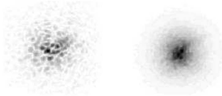
FIG. 2.3 – Effet de la turbulence atmosphérique au foyer d’un télescope. Gauche : temps de pose court (~100 ms), droite : temps de pose long (> 1 s).
