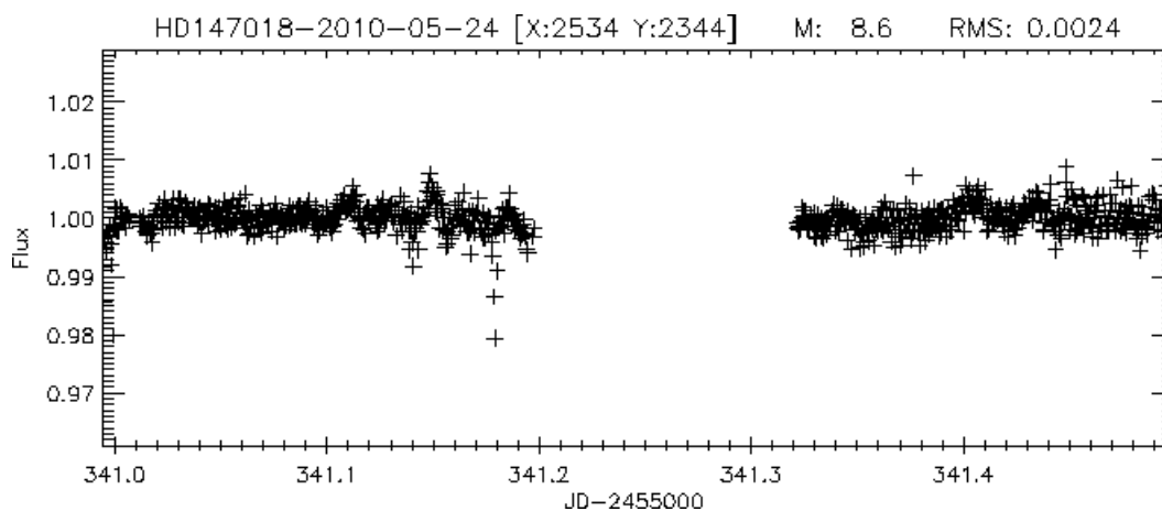
FIG. 7.30 – Courbe de lumière de HD147018 le 24 mai 2010 entre 12h et 24h UTC, avec une interruption de ~3 heures. Les observations ne montrent pas de transit.
