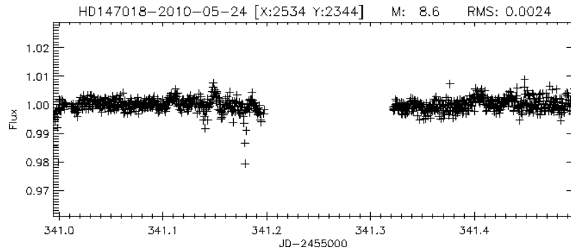
FIGURE 8.30 – Courbe de lumière de HD147018 le 24 mai 2010 entre 12h et 24h UTC, avec une interruption de \sim 3 heures. Les observations ne montrent pas de transit.
