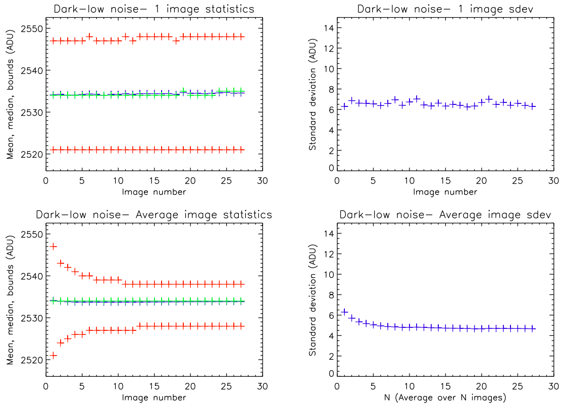
FIGURE 3.13 – Statistiques sur les images de dark de 30 s prises en lecture rapide pour la caméra ASTEP Sud. Moyenne (bleu), médiane (vert), et intervalle contenant 99 % des pixels (rouge), pour chacune des \sim 30 images (haut gauche), déviation standard pour chacune des \sim 30 images (haut droite), déviation standard d'une image moyenne faite à partir de N images (bas gauche), et déviation standard par pixel sur plusieurs images moyennes de N images (bas droite).
