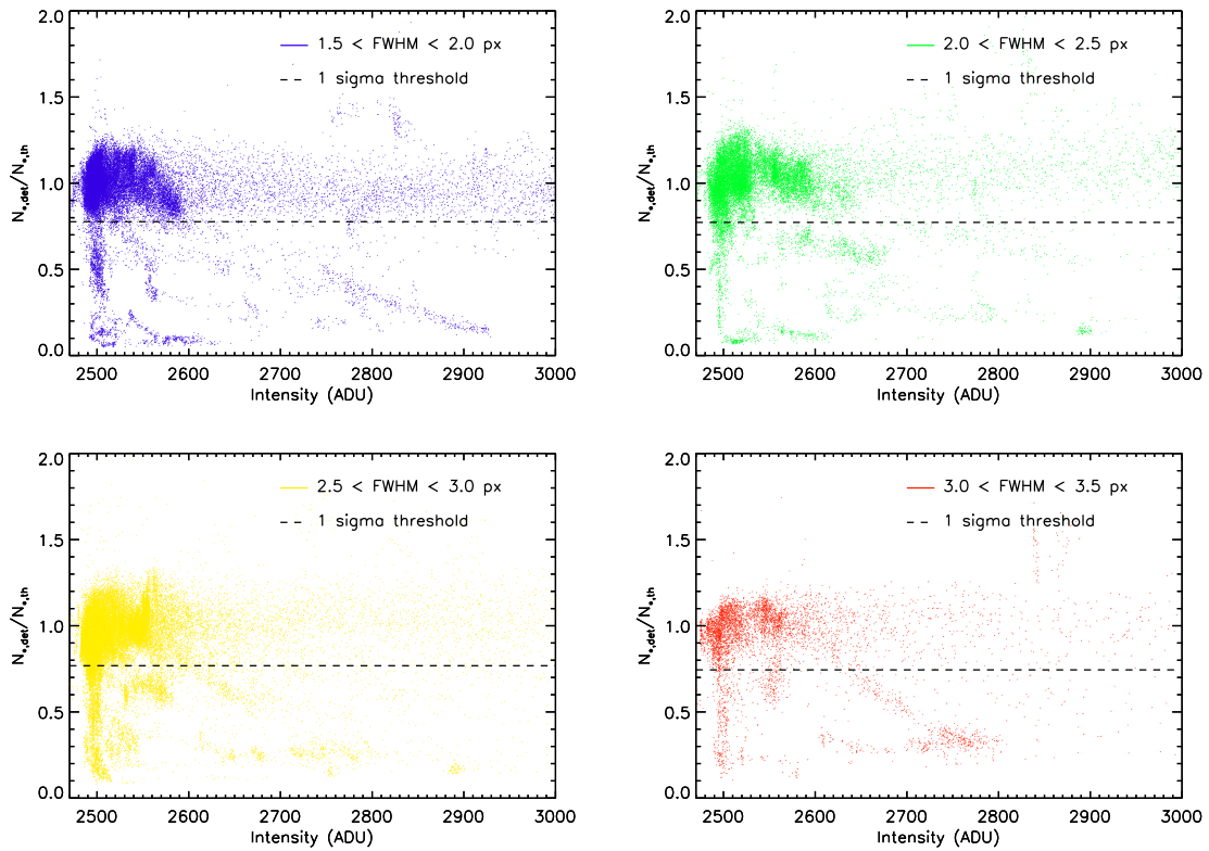
FIGURE 5.4 – Rapport du nombre d'étoiles détectées sur le nombre d'étoiles théorique en fonction de l'intensité pour les différentes pages de FWHM, dans la 2 nde approche. La limite à 1\sigma est indiquée en pointillés.
