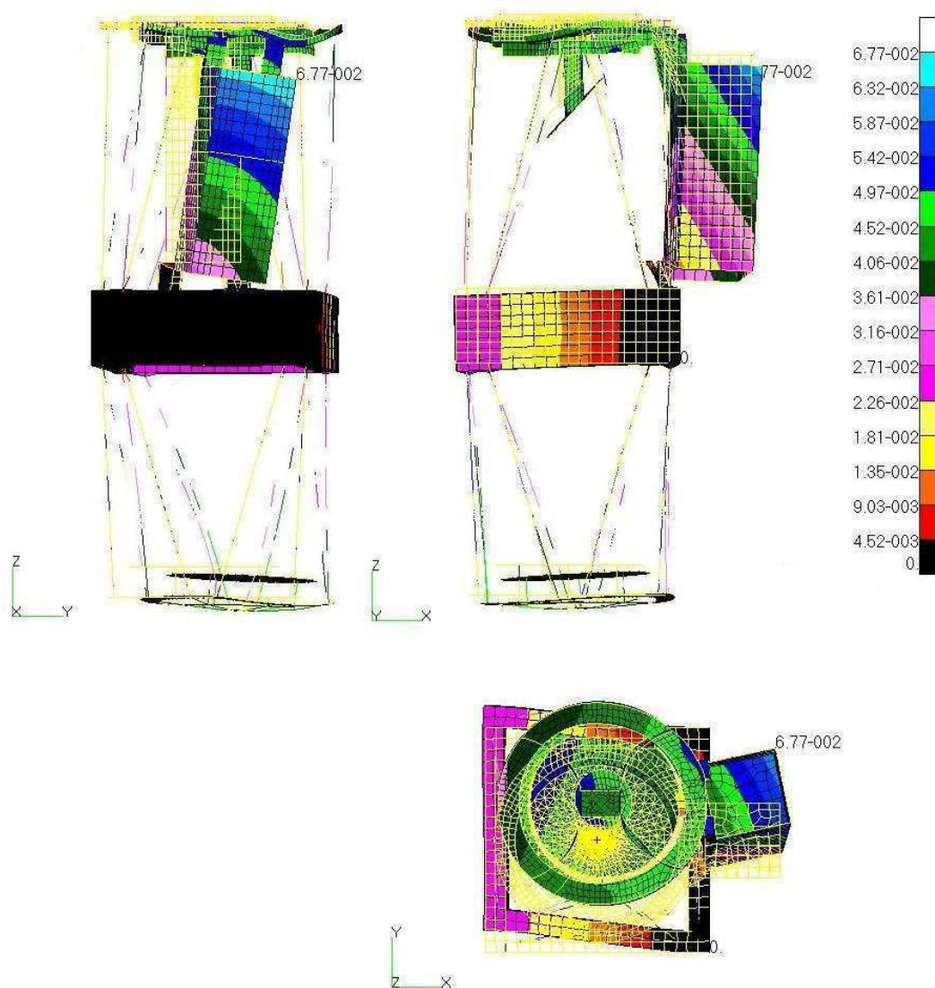
FIGURE 7.6 – Déformations mécaniques dues au poids pour une orientation du télescope à 45° Nord, vues de côté (haut) et de dessus (bas).
