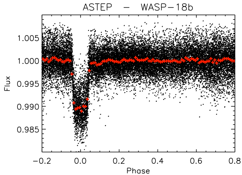
FIGURE 8.25 – Courbe de lumière de WASP-18 en phase, à partir des 23 jours d'observations ( \sim 24 périodes). Une moyenne par intervalle de 1/100^{\text{me}} de période, soit 14 mn, est représentée en rouge.
