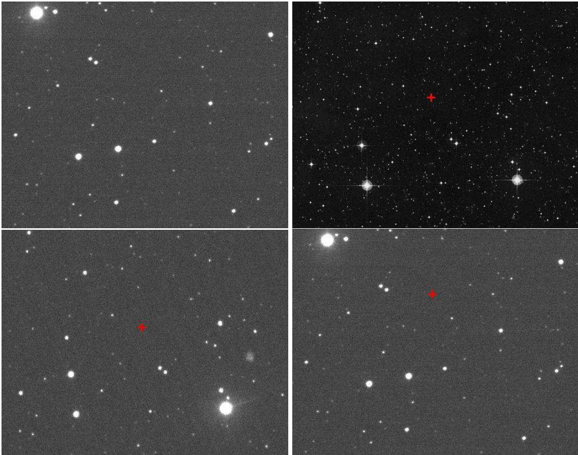
FIGURE 4.13 – Principe de la reconnaissance de champ. On cherche la transformation qui permet de faire correspondre l'image ASTEP Sud (haut gauche) à un catalogue standard (haut droite, ici représenté par une image du Digitized Sky Survey). Une fois la transformation trouvée (bas gauche), on détermine la position du pôle sur l'image initiale par l'inverse de cette transformation appliquée au pixel (2048, 2048) (bas droite). Le pôle sud est représenté par une croix rouge.
