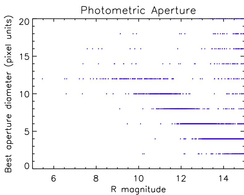
FIGURE 6.12 – Meilleure ouverture photométrique en fonction de la magnitude des étoiles. La sélection automatique donne le résultat attendu : la taille de l'ouverture diminue vers les étoiles plus faibles.
