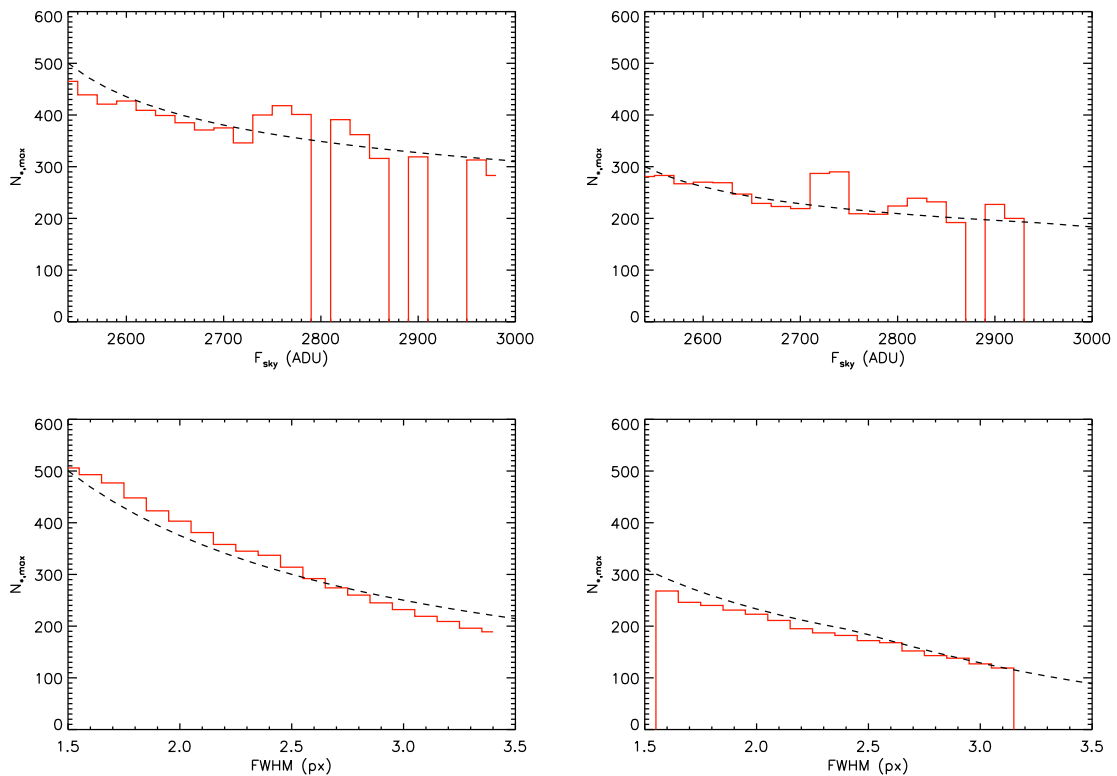
FIGURE 5.8 – Validation du modèle de la 3 0 me approche, pour les observations de 2008. La relation théorique N_{*,th} = f(F_{sky}, \omega) (ligne pointillée) est comparée au nombre d'étoiles détectées sur les meilleures images, d'abord en faisant varier le fond de ciel F_{sky} de 40 à 500 ADU (à partir de l'offset de 2470 ADU), pour un FWHM \omega fixé à 1.5 px (haut gauche) puis à 2.5 px (haut droite); ensuite en faisant varier le FWHM de 1.5 à 3.5 px, pour F_{sky} fixé à 40 ADU (bas gauche) puis à 500 ADU (bas droite). Ce test valide le modèle.
