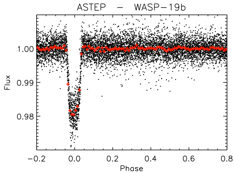
FIGURE 8.21 – Courbe de lumière de WASP-19 en phase, à partir des 24 jours d’observations ( \sim 30 périodes). Une moyenne par intervalle de 1/100^{\text{me}} de période, soit 11 mn, est représentée en rouge.
