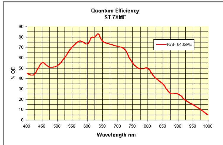
FIGURE 7.16 – Courbe d’efficacité quantique de la caméra de guidage SBIG ST402. Le CCD est sensible dans tout le domaine visible ; on n’utilisera que la partie bleue.
