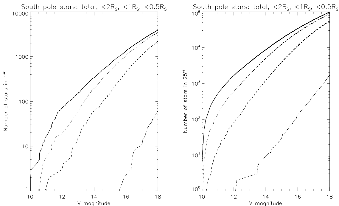
FIGURE 4.2 – Distribution en magnitude des étoiles dans un champ centré sur le pôle sud, à partir du modèle de Besançon. Gauche : champ de 1^\circ , droite : champ de 22^\circ (dû à un effet de projection, ce champ est légèrement plus petit que 25^\circ ). Les courbes indiquent le nombre total d'étoiles dans le champ (ligne pleine), ainsi que le nombre d'étoiles de rayon R \leq 2R_\odot (points), R \leq R_\odot (traits), et R \leq 0.5R_\odot (traits-points)
