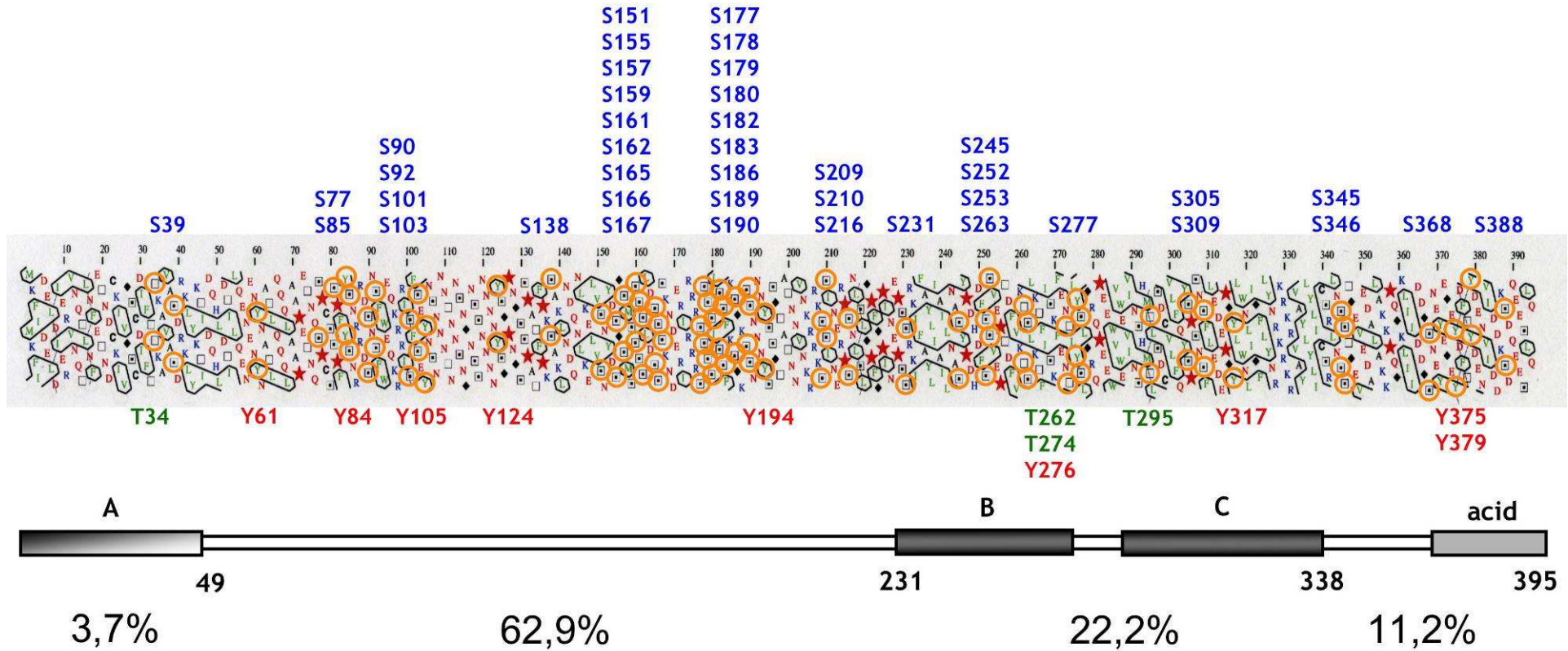
Figure 11. Localisation des résidus potentiellement phosphorylables dans la protéine Maf1 chez S. cerevisiae . La figure présente les localisations des sérines (bleu), thréonine (vert) et tyrosine (rouge) prédites pour être phosphorylées. Les résidus potentiellement phosphorylables (entourés par un cercle orange) sont représentés sur une représentation obtenue par analyse des clusters hydrophobes (HCA) (Callebaut et al. , 1997). Une représentation schématisée des domaines de Maf1 est présentée en bas. Les pourcentages de résidus potentiellement phosphorylables dans chaque domaine A, « linker », BC et région acide sont indiqués.
