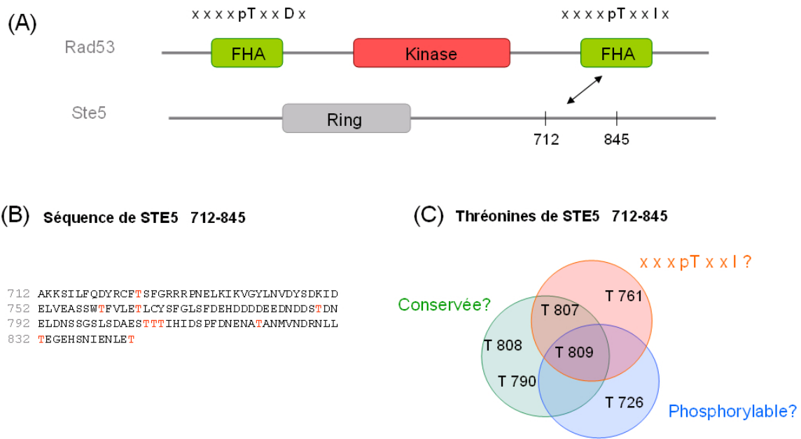
figure 50 : Etude de l'interaction entre le domaine FHA2 de Rad53 et Ste5. En haut : Interaction entre le domaine FHA2 de Rad53 et le fragment 712-845 de Ste5 mise en évidence lors du criblé double hybride. A gauche : séquence du fragment 712-845 de la protéine Ste5. Les thréonines sont indiquées en rouge. A droite : analyse des différentes thréonines de la séquence de Ste5 712-845 par les 3 critères de respect du motif de plus forte affinité du domaine FHA2 de Rad53, pTxxI (ensemble rouge), de phosphorylabilité (ensemble bleu), de conservation de la thréonine et de l'acide aminé en position +3 relativement à la thréonine (ensemble vert). Seule la thréonine T809 respecte ces trois critères simultanément, avec les seuils abaissés (intersection des trois ensembles).
