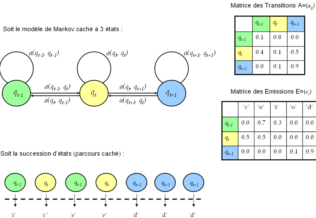
figure 14 : Modèle de Markov caché contenant 3 états : q_{t-1} , q_t , q_{t+1} . La matrice de transition A=(a_{ij}) indique les probabilités de transition de chaque état i vers chaque état j . La somme des probabilités de transition sortantes de chaque état (somme des éléments d'une ligne) est égale à 1. La matrice des émissions stocke, pour chaque état, la probabilité d'émettre chacune des 5 lettres 'c', 'e', 'i', 'o', 'd', dont la somme est égale à 1. Pour une succession d'états (q_{t-1}, q_t, q_{t-1}, q_t, q_{t+1}, q_{t+1}, q_{t+1}) , on peut observer une séquence ('i', 'c', 'e', 'e', 'd', 'd', 'd').
