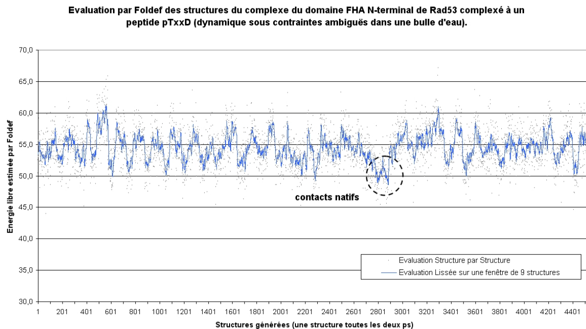
figure 70 : Evaluation des structures générées au cours de la dynamique par la fonction d'énergie Foldef. Pour plus de clarté, la courbe est lissée avec une fenêtre de 9 structures (4 structures en amont et 4 en aval).
