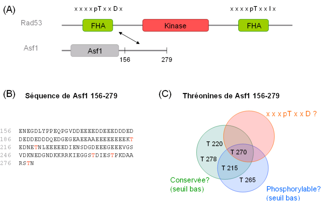
figure 43 : Etude de l'interaction entre le domaine FHA1 de Rad53 et Asf1. (A) Interaction entre le domaine FHA1 de Rad53 et le fragment 156-279 de Asf1. (B) Séquence du fragment 156-279 de la protéine Asf1. Les thréonines sont indiquées en rouge. (C) Analyse des différentes thréonines de Asf1 156-279 par les 3 critères de respect du motif de plus forte affinité du domaine FHA1 de Rad53, pTxxD (ensemble rouge), de phosphorylabilité (ensemble bleu), de conservation de la thréonine et de l'acide aminé en position +3 relativement à la thréonine (ensemble vert). Seule la thréonine T270 respecte ces trois critères simultanément avec les seuils abaissés (intersection des trois ensembles).
