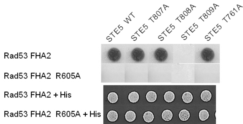
figure 51 : Etude par double hybride de l'interaction entre le domaine FHA2 de Rad53 et différents mutants de Ste5 : Ste5 wild-type (WT), Ste5 T807A, Ste5 T808A, Ste5 T809A et Ste5 T761A. Le mutant Ste5 T809A est affecté dans sa liaison au domaine FHA2 de Rad53. La substitution R605A du domaine FHA2 de Rad53 abroge l'interaction avec Ste5 à la fois dans le wild-type et dans tous les mutants, ce qui suggère que l'interaction est bien phospho-dépendante.
