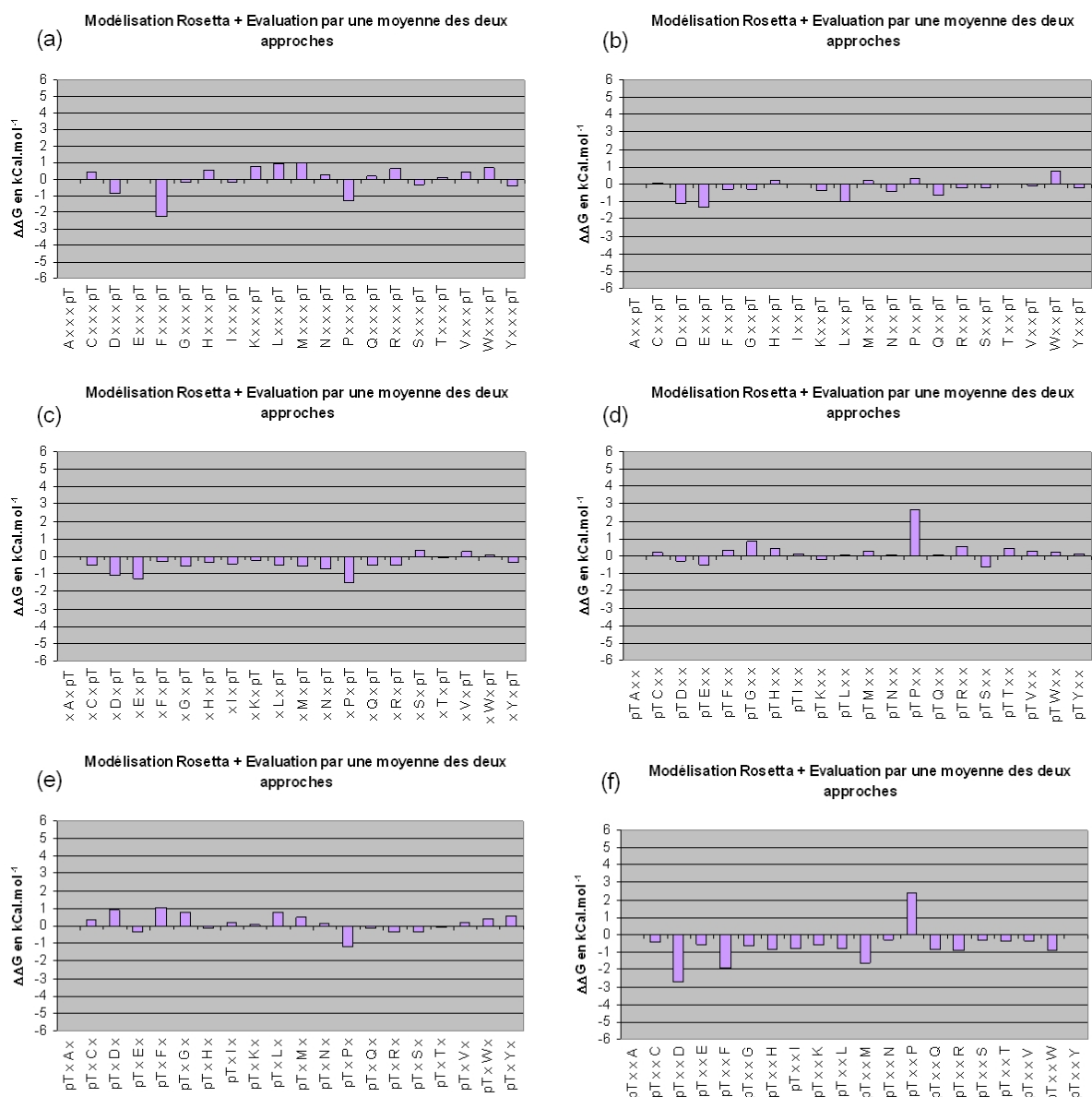
figure 75 : Criblage in silico du peptide en contact avec le domaine FHA N-terminal de la protéine Rad53. Les variations d'énergie libre sont estimées par ROSETTA et FOLDEF en kcal.mol -1 . Les positions criblées sont (a) pT-4, (b) pT-3, (c) pT-2, (d) pT+1, (e) pT+2, (f) pT+3. La position pT-1, complètement exposée au solvant, n'est pas criblée.
