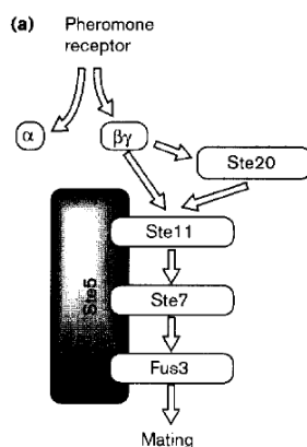
figure 49 : Représentation schématique du rôle de scaffolding protein de Ste5. Chez la levure, la voie de signalisation menant à la conjugaison utilise Ste5 comme scaffolding protein permettant de lier les membres du module formé de Ste11, Ste7 et Fus3. Figure extraite de (Garrington and Johnson, 1999).
