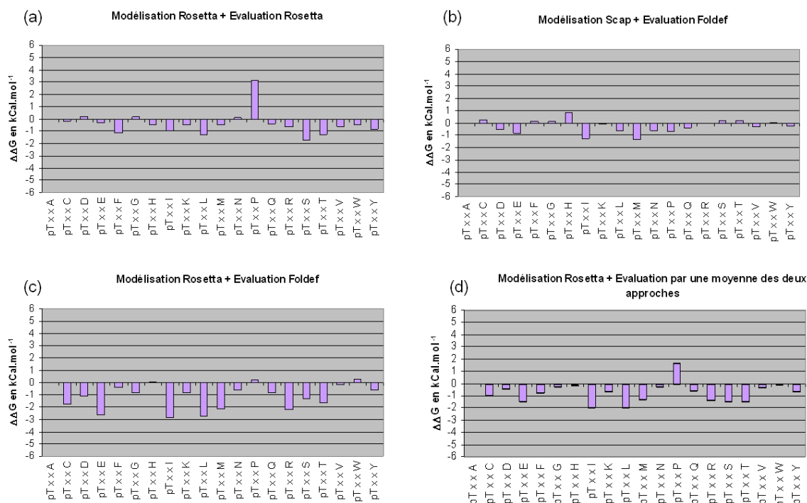
figure 71 : Criblage in silico du domaine FHA N-terminal de la protéine Chk2 sur la position pT+3. Le motif le plus affiné pour ce domaine FHA est pTxxL/L. Les graphes (a) (b) (c) et (d) sont construits de la même façon que dans la figure figure 63 .
