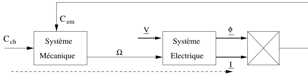
FIG. 3.11 – Schéma fonctionnel causal global d'un entraînement à base de machine électrique
