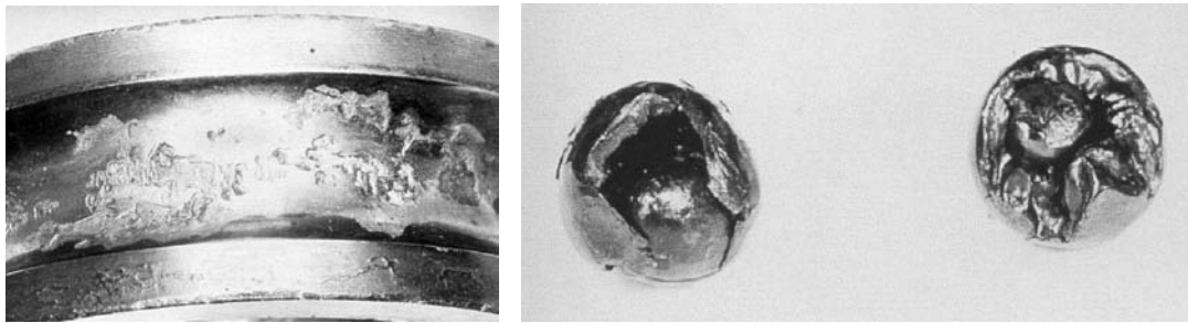
(a) Écaillage d'un chemin de roulement
