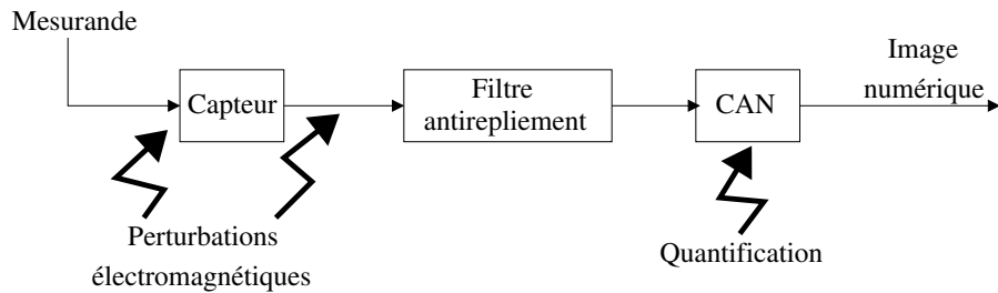
FIG. 4.5 – Schéma d'une chaîne de mesure avec les perturbations responsables des bruits
