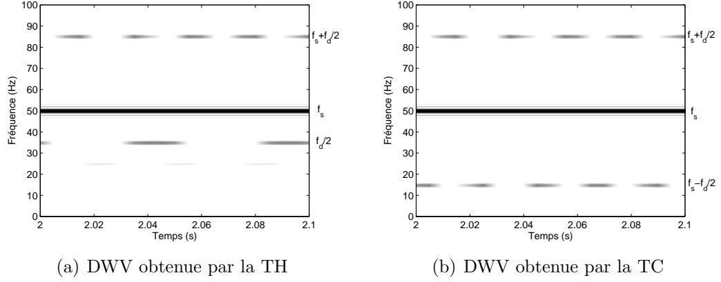
FIG. 6.22 – DWW de signaux de courants simulés en présence d’une modulation de phase rapide
