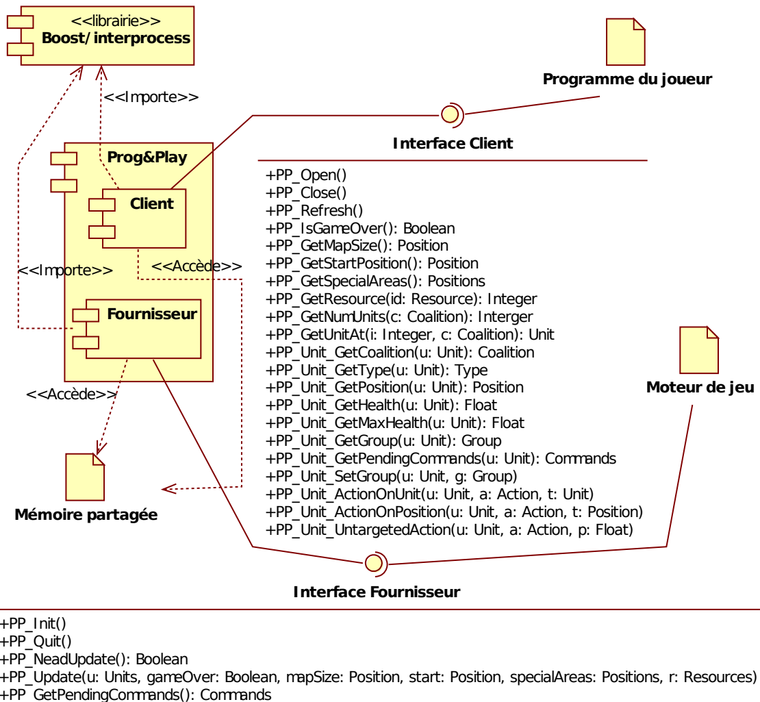
FIGURE 4.15 – Diagramme de composants du système Prog&Play.
