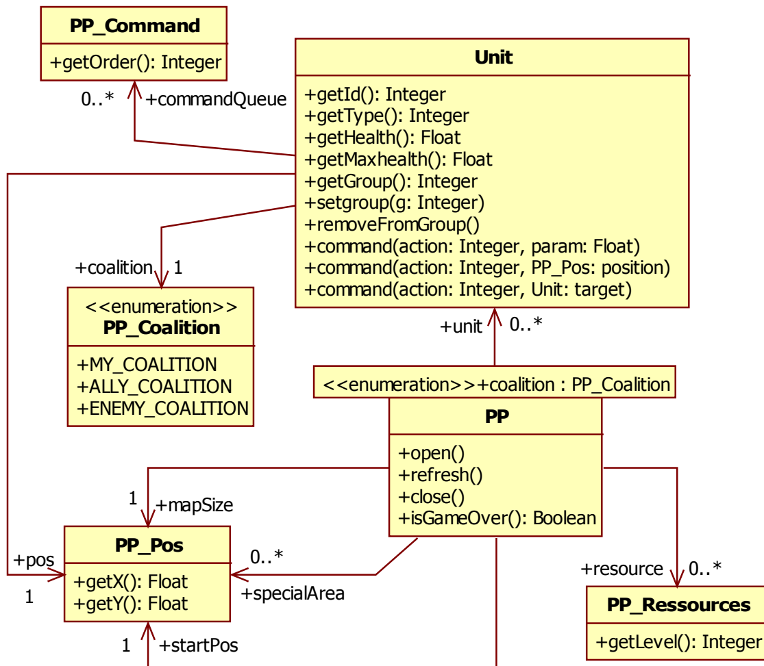
FIGURE 4.25 – Proposition d’une représentation de l’API Prog&Play sous une forme orientée objet.
