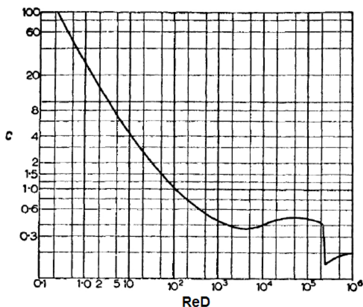
FIG. II.1 – Evolution du coefficient de traînée C d'une gouttelette sphérique en fonction de son nombre de Reynolds Re_D
