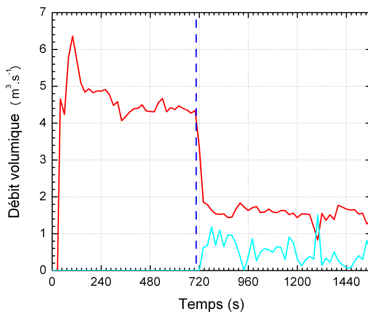
FIG. V.42 – Essai bûcher ETun21 - Evolution temporelle des débits volumiques \dot{V}_{\text{gaz}, \text{foy}} (—) et \dot{V}_{\text{vap}} (—)
