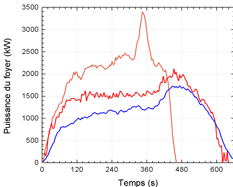
FIG. IV.4 – Essais ETun 01 et ETun 02 - Evolution temporelle de la puissance du foyer - (—) : ETun01 - Puissance par la mesure de perte de masse, (—) : ETun02 - Puissance par la mesure de consommation d'oxygène
