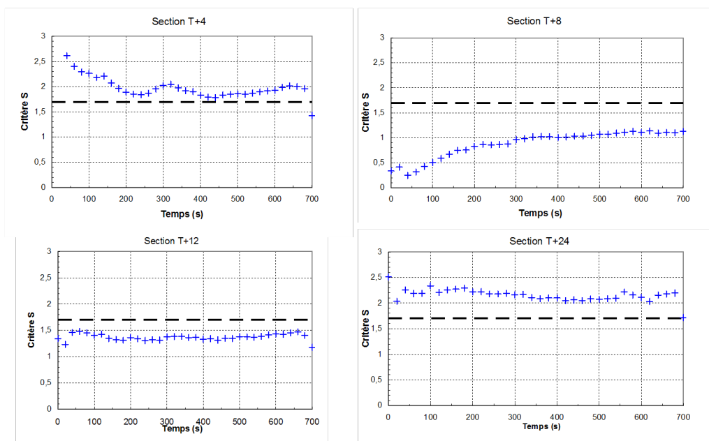
FIG. IV.67 – Essai ETun06 - Evolution temporelle du critère de stratification S
