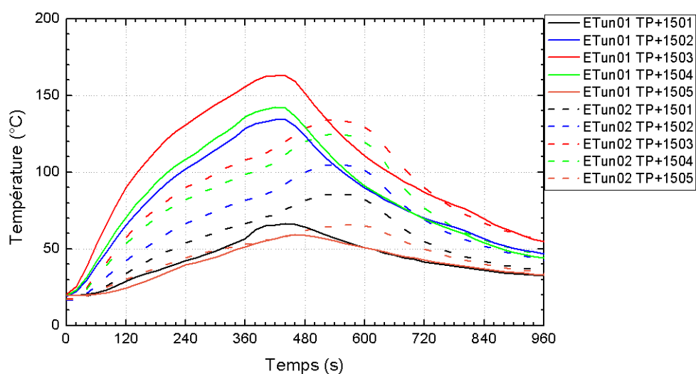
FIG. IV.5 – Essais ETun 01 et ETun 02 - Evolution temporelle des niveaux des températures de surface de la paroi du tunnel en section S+15
