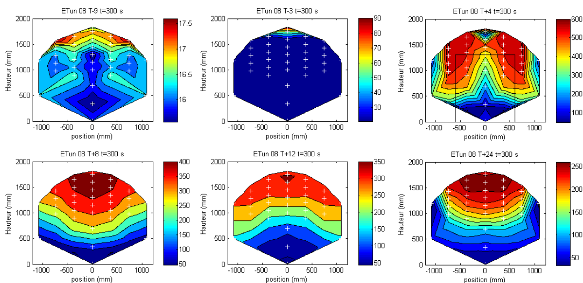
FIG. IV.25 – Essai ETun08 - Répartition de la température par section - t=300s
