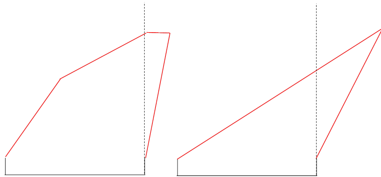
FIG. IV.8 – Variation de la projection du volume de flamme sur la nappe de combustible, cas d'un essai sans couverture
