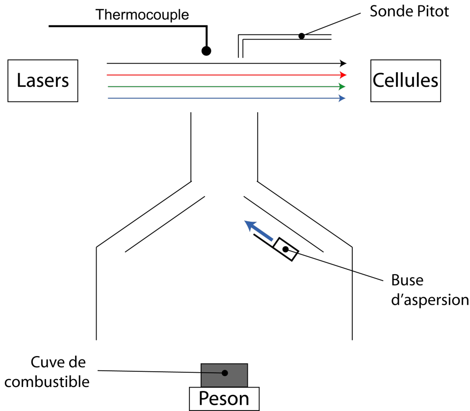
FIG. VI.10 – Schéma du dispositif de caractérisation des fumées
