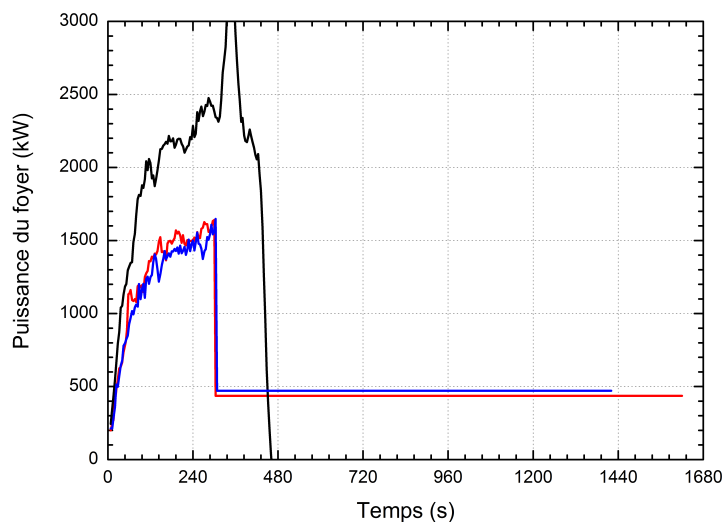
FIG. V.10 – Essai ETun09 et ETun10 - Evolution temporelle de la puissance du foyer par mesure de perte de masse - Essais ETun09 (—) et ETun10 (—) - Comparaison avec l'essai ETun01 (—)
