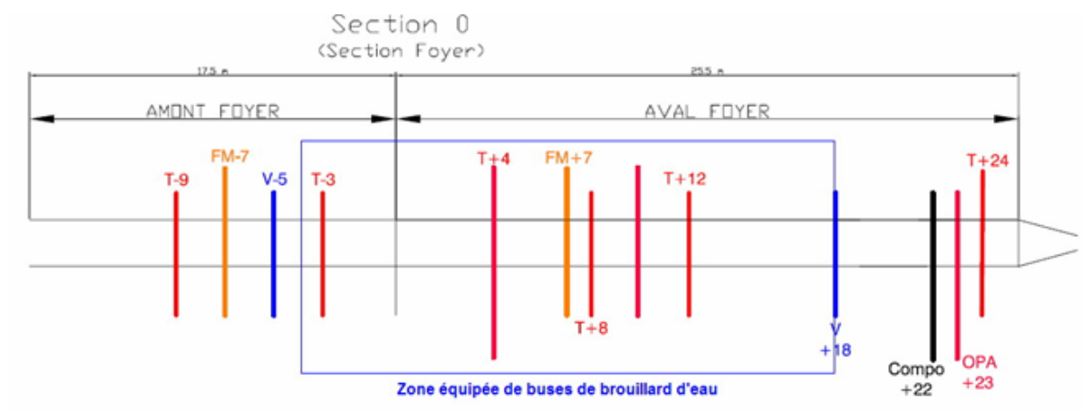
FIG. V.6 – Représentation de la zone du tunnel équipée de buses d'aspersion
