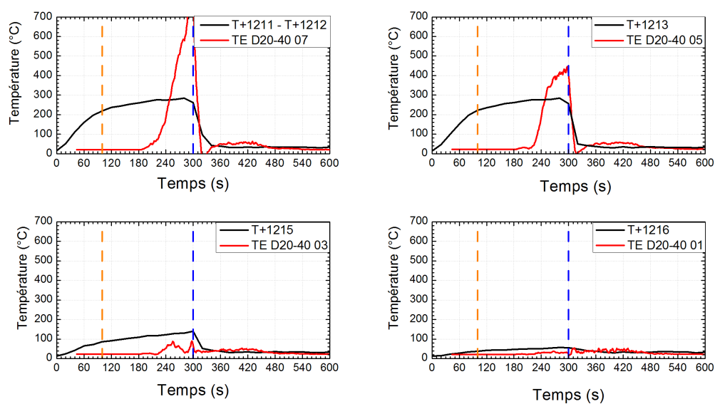
FIG. V.78 – Section ETunT+12 - Comparaison des évolutions temporelles de température de la campagne ETun (—) et SOLIT (—)
