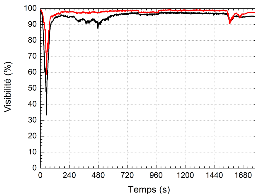
FIG. IV.59 – Essai Etun04 - Evolution de la visibilité en section S+23, à 50 cm du sol (—) et à 50cm du plafond (—)
