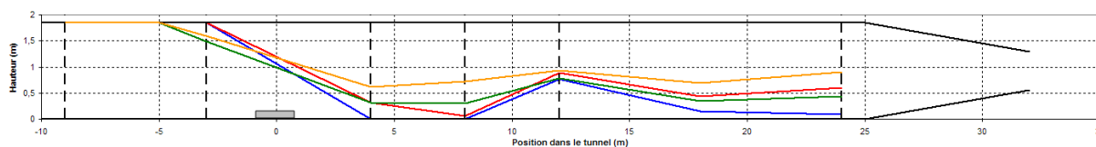
FIG. IV.80 – Essais ETun02 et ETun08 - Limite basse des zones de tenabilité : (—) : ETun02 - 50°C, (—) : ETun08 - 50°C, (—) : ETun02 - 100°C, (—) : ETun08 - 100°C
