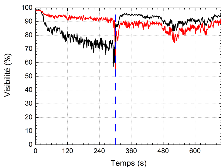
FIG. VI.3 – Essai Etun27 - Evolution de la visibilité en section S+23 : (—) : à 50 cm du sol et (—) : à 50cm du plafond
