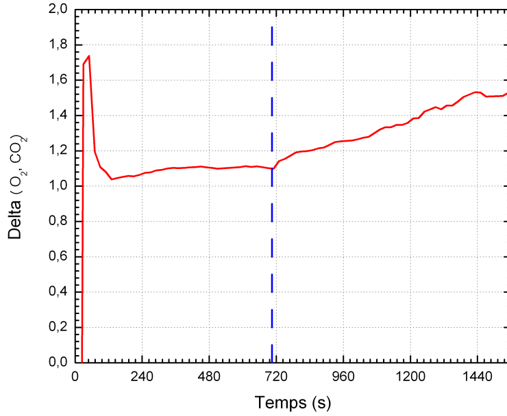
FIG. V.41 – Essai bûcher ETun21 - Evolution temporelle de l'écart \Delta(\text{O}_2, \text{CO}_2) entre les concentrations de \text{O}_2 et de \text{CO}_2
