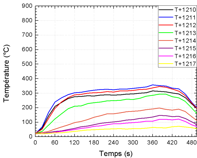
FIG. IV.15 – Essai ETun01 - Evolution temporelle des niveaux de température en section T+12
