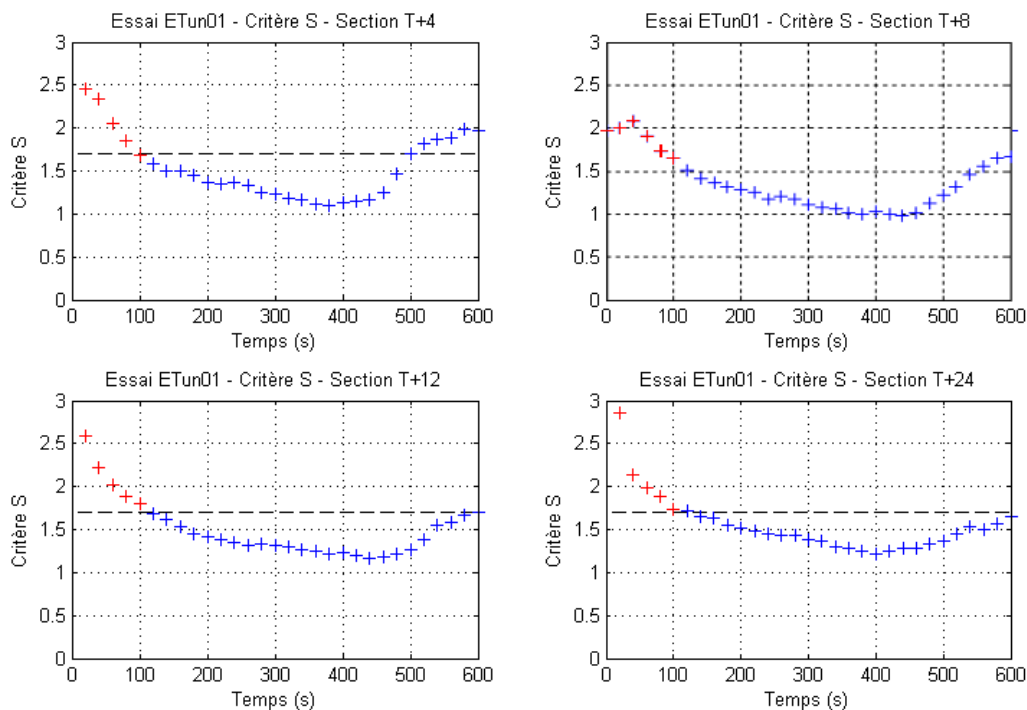
FIG. IV.28 – Essai ETun01 - Evolution temporelle du critère de stratification S
