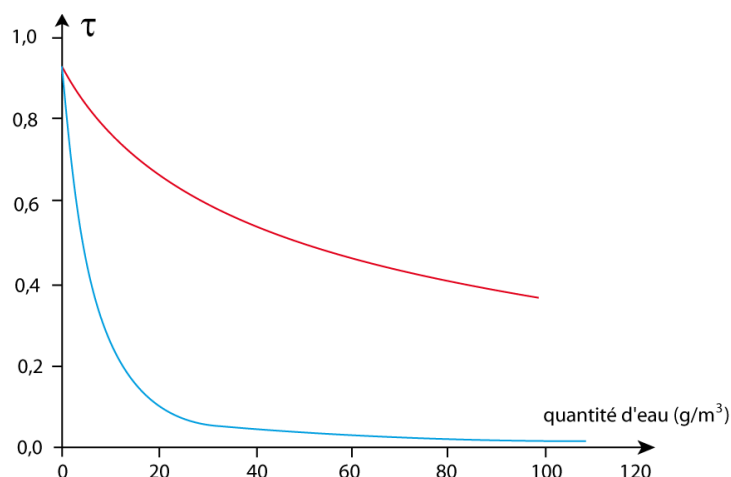
FIG. I.18 – Evolution du taux de transmission \tau en fonction de la quantité d'eau injectée lorsque l'on tient compte de la diffusion ou non ( L=0,5 m, T_s = 1300 K, R=0 , d=10 \mu\text{m} ) - (—) : taux de transmission \tau_{BL} , (—) : taux de transmission \tau [6]
