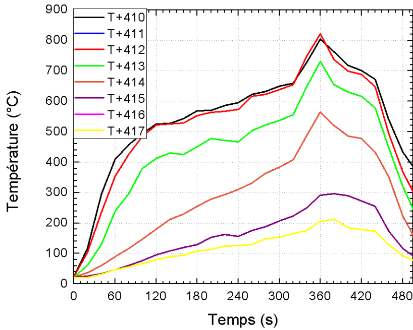
FIG. IV.11 – Essai ETun01 - Evolution temporelle des niveaux de température en section T+4
