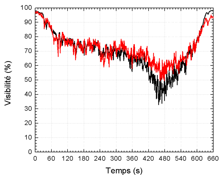
FIG. IV.40 – Essai ETun02 - Evolution de la visibilité en section S+23, à hauteur d'homme 50 cm dans le tunnel (—) et à 50cm du plafond (—)
