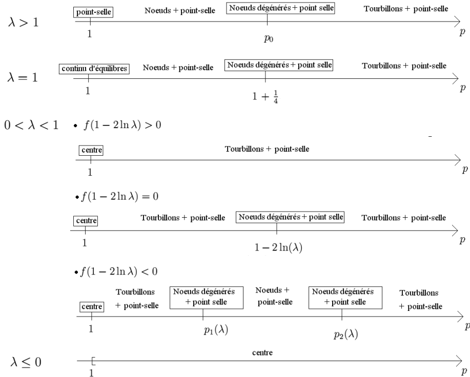
FIG. 2.16 – Bifurcation en fonction de p .
