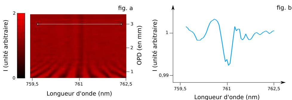
FIGURE 5.6 – Mise en évidence du phénomène de Bragg par un balayage en longueurs d'ondes
