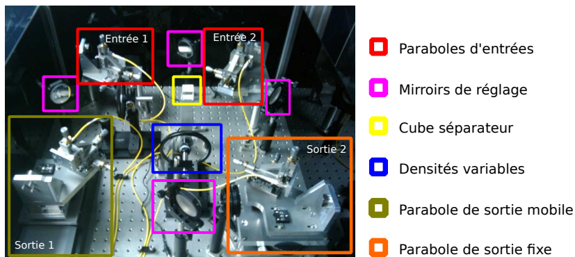
FIGURE 4.15 – Photographie du banc séparateur de flux/variable d'OPD
