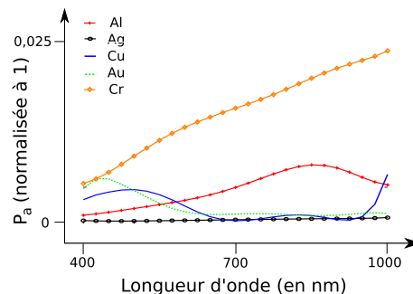
FIGURE 3.11 – Pouvoir d'absorption des matériaux
