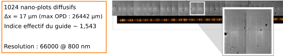
FIGURE 5.3 – Exemple d'un composant de la dernière série
