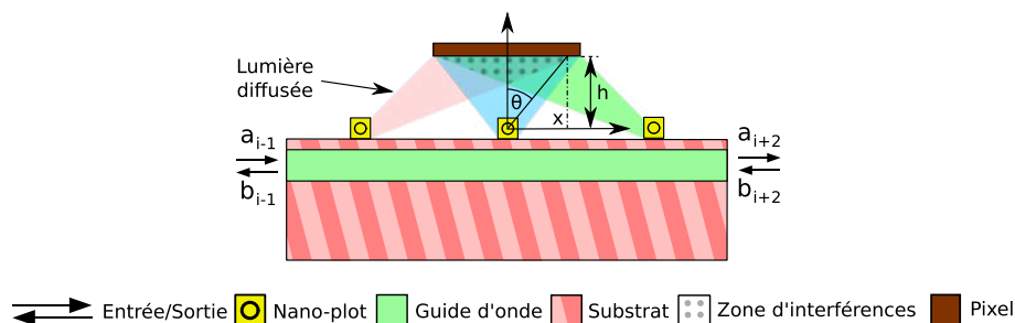
FIGURE 4.6 – Phénomène de diaphotie entre les nano-plots voisins
