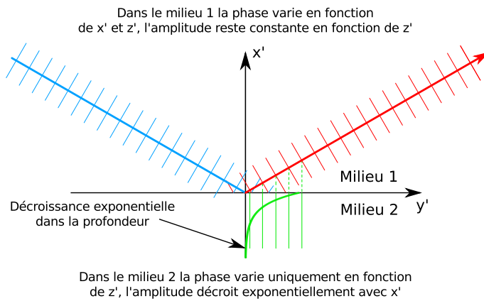
FIGURE 2.20 – Réflexion totale d'une onde à l'interface de deux milieux diélectriques
