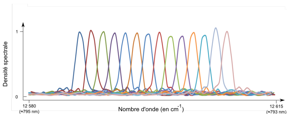
FIGURE 5.12 – Reconstruction du « spectre » d'une source monochromatique accordable en longueur d'onde pour différentes positions
