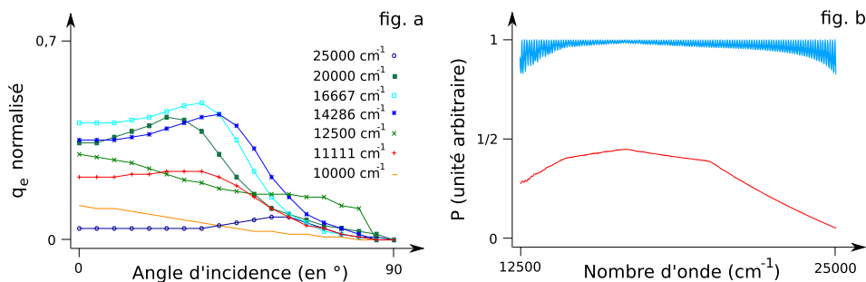
FIGURE 4.8 – Limitation du phénomène de diaphotie grâce au filtrage angulaire effectué par le pixel
