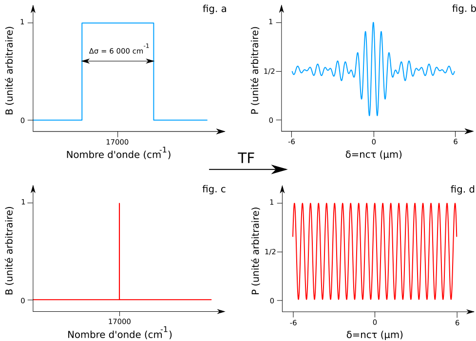
FIGURE 2.6 – Schémas de correspondance entre un spectre et son interférogamme
