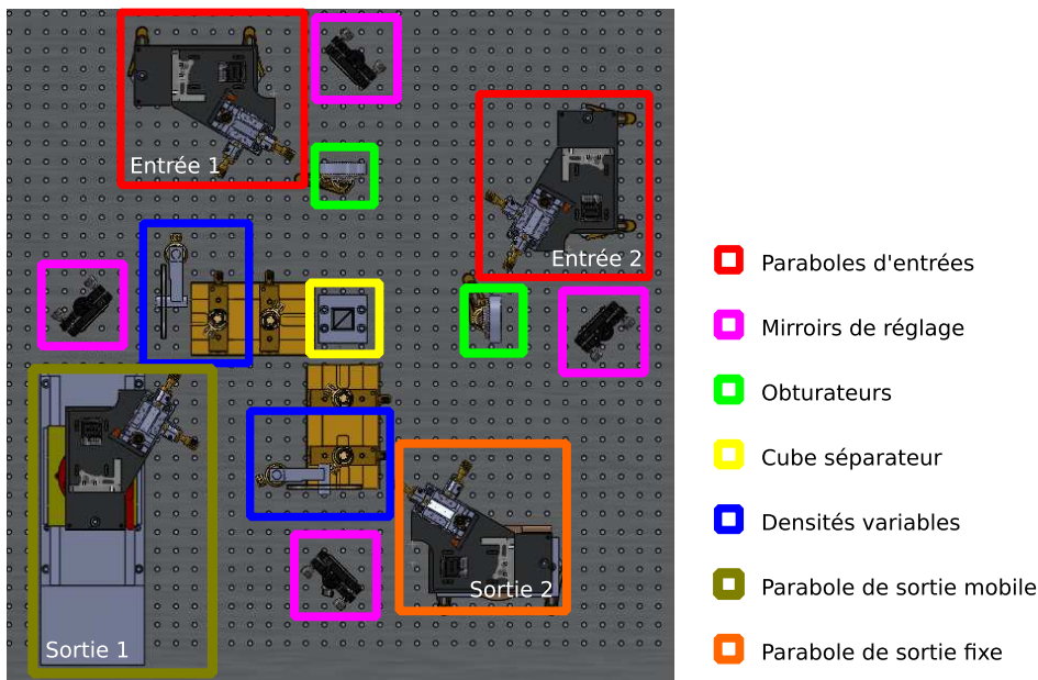
FIGURE 4.14 – Schéma mécanique global du banc séparateur de flux/variable d'OPD
