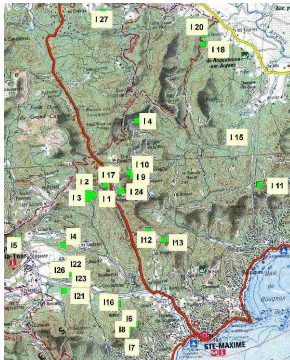
Figure 2.2 : Localisation des parcelles d'étude dans le massif des Maures (Venetier et al. , 2008).
