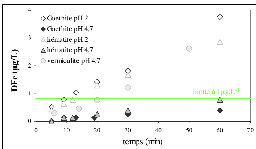
Figure 2.6 : Concentration en fer dissous mesuré en fonction du contact pour la vermiculite, l'hématite et de la goethite à pH 2 et 4,7 d'après les travaux de Sofitikis (2004). La ligne verte indique la concentration minimale nécessaire pour la mesure de Fe(II) dissous.
