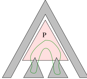
FIGURE 1.5 – Cycle dans un graphe de dépendances
