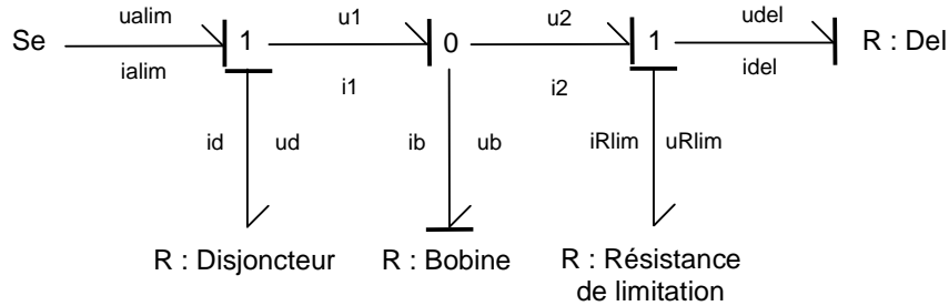
Figure 2.43 : Représentation sous forme de graphe de liaison de l'association d'un disjoncteur et d'un contacteur électromécanique constitué de 3 sous ensembles
