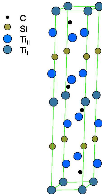
FIGURE 3.16 – Structure cristallographique de la phase MAX Ti_3SiC_2 .
