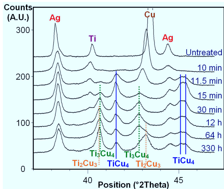
FIGURE 3.2 – Évolution du diffractogramme obtenu en DRX d'un mélange Ag 20 Cu 50 Ti 30 (en at.%) recuit pendant des durées croissantes à 790 °C.
