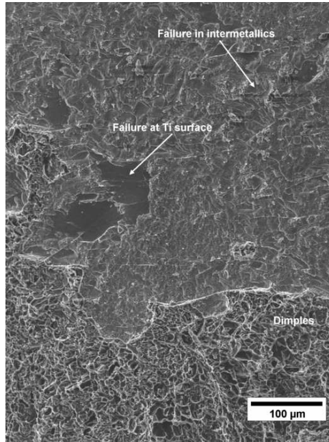
FIGURE 4.11 – Image MEB du faciès de rupture caractéristique d’une interface Ti/AS-7 après traitement thermique et essai mécanique en flexion circulaire.
