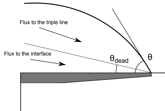
FIGURE 2.10 – Représentation schématique du sens physique que revêt l'existence de l'angle mort qui doit être soustrait à l'angle de contact instantané dans l'équation de Mortensen (Eq. 2.10). Le flux de soluté réactif qui pénètre dans l'angle solide délimité par l'angle mort ne parvient pas à la ligne triple et est consommé par l'épaississement de la couche de réaction en arrière de la ligne triple.
