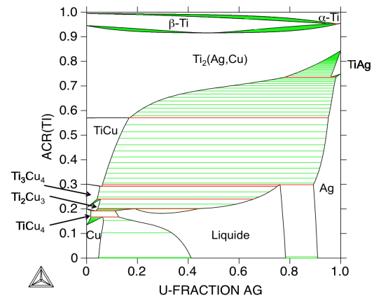
FIGURE 3.15 – Activité de Ti en fonction de u_{Ag} (= \frac{x_{Ag}}{x_{Ag} + x_{Cu}}) à 850 °C. Référence HCP à 850 °C.
