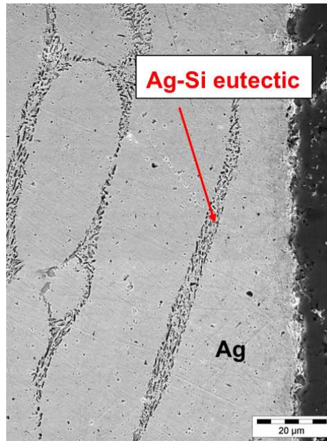
FIGURE 3.17 – Micrographie MEB en section d’une interface entre une goutte Ag pur et \text{Ti}_3\text{SiC}_2 après 4 h de contact à 980 °C.
