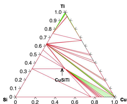
FIGURE 3.23 – Section isotherme à 800 °C du système Cu-Si-Ti
