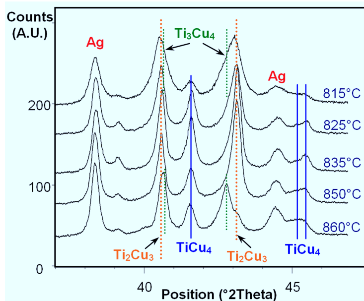
FIGURE 3.1 – Évolution du diffractogramme d’un mélange de composition \text{Ag}_{20}\text{Cu}_{50}\text{Ti}_{30} (en at.%) réagit 205 h à 815 °C puis recuit à plus haute température : 825, 835, 850, 854 et 860 °C
