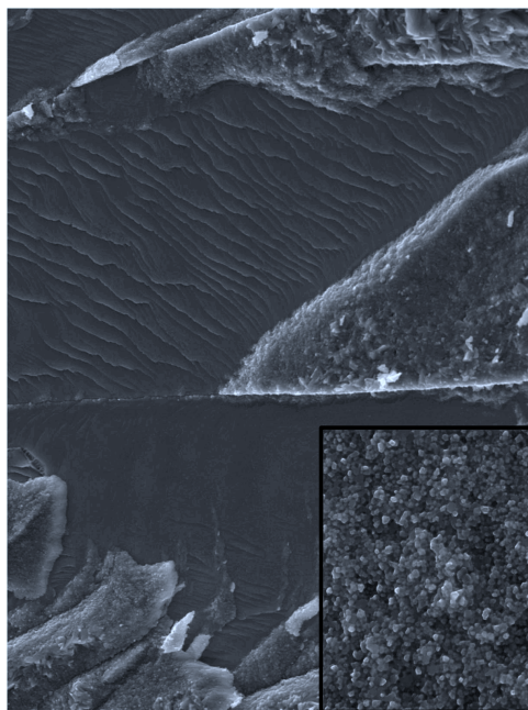
FIGURE 4.12 – Micrographie MEB du faciès de rupture sur un insert Ti après traitement thermique et test en flexion circulaire. Zones caractéristiques de la rupture fragile : apparence intragranulaire (surface avec vaguelette) et intergranulaire (agrandissement dans l’encart). L’analyse EDS indique Ti pur dans la première zone et un siliciure de titane pour la seconde.
