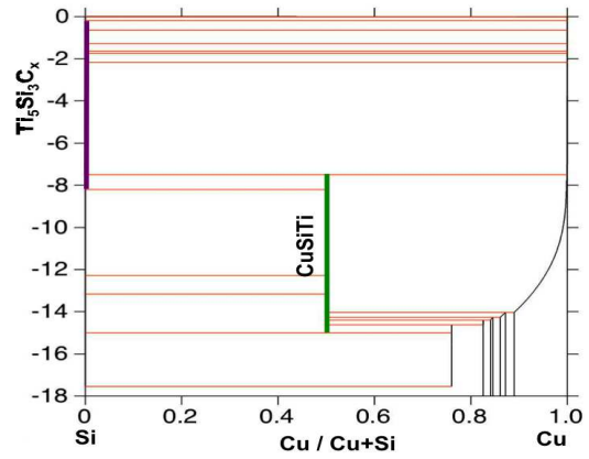
FIGURE 3.25 – Logarithme de l’activité de Ti en fonction de u_{Cu} (= \frac{x_{Cu}}{x_{Cu}+x_{Si}}) à 800 °C. Référence HCP à 800 °C.
