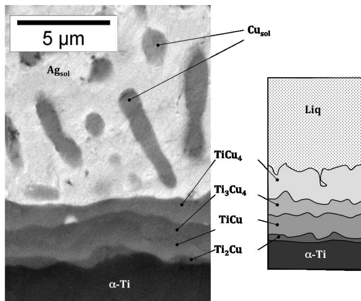
FIGURE 3.8 – Séquence réactionnelle à l'interface solide/liquide du couple Ti/Ag-40Cu après 50 min à 795 °C
