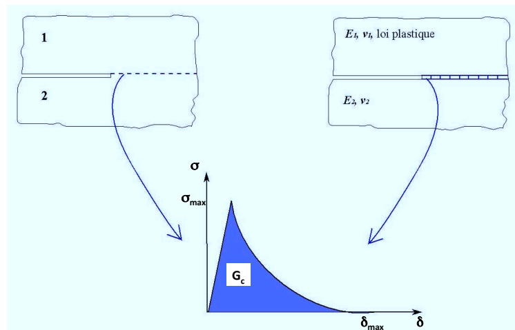
FIGURE 4.17 – Schéma de principe d'une loi de traction séparation utilisée pour une interface en mode I dans un modèle de zone cohésive [Bra09].
