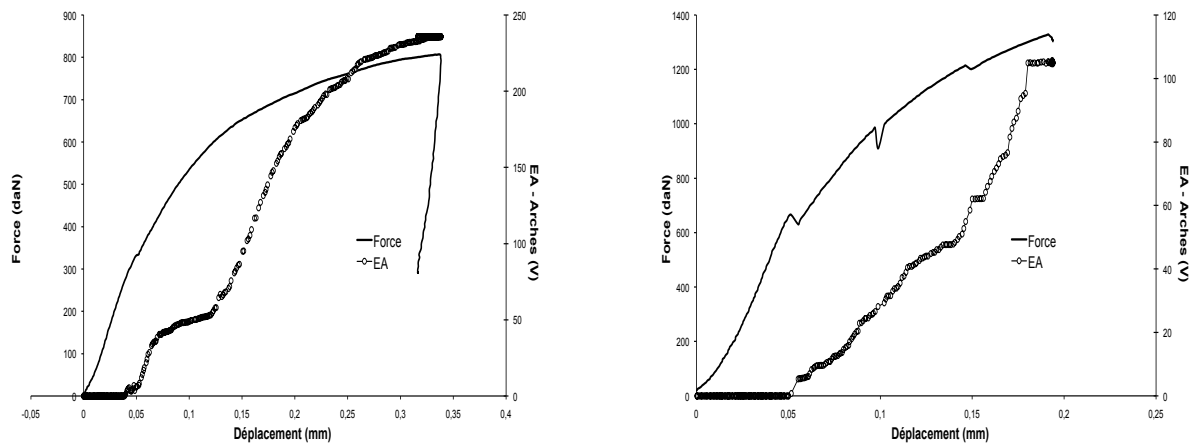
FIGURE 4.10 – Courbe charge-déplacement typiquement obtenue lors d'un essai de flexion circulaire d'une matrice AS-7 renforcée par un insert Ti pour une tranche de 5 mm d'épaisseur : sans traitement thermique (gauche) et après un traitement thermique de type T6 (droite).
