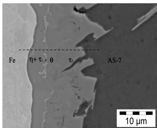
FIGURE 4.14 – Micrographie d’une interface type entre Fe et AS-7 obtenue après 2 min de contact à 800 °C (gauche). Profil de concentration des différents éléments au travers de cette zone obtenu en microsonde électronique (droite).
