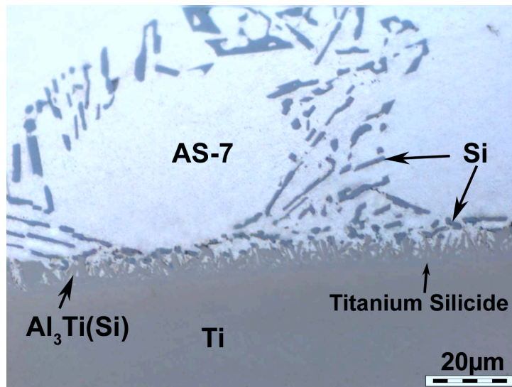
FIGURE 4.3 – Micrographie optique de la zone réactionnelle qui se forme entre un insert Ti et un liquide Al-7wt.%Si après 15 min à 700 °C. Section perpendiculaire à l’axe de l’insert.
