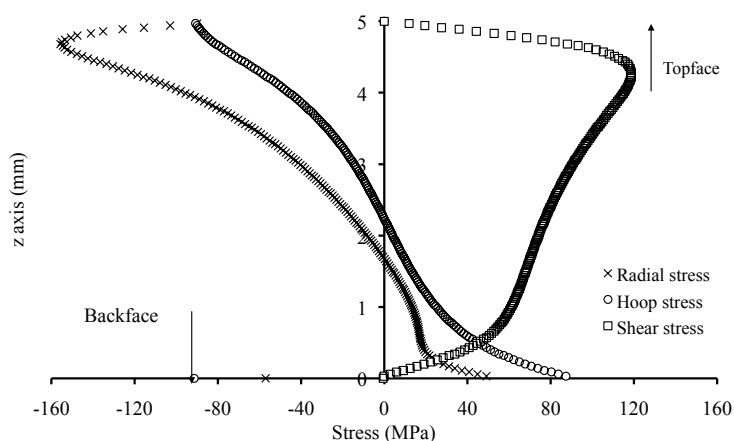
FIGURE 4.1 – Evolution des contraintes radiales \sigma_{rr} , tangentielles \sigma_{\theta\theta} et de cisaillement \sigma_{rz} le long d'une interface Ti/Al-7Si au cours d'un chargement en push-out à 600 daN (niveau de chargement correspondant au premier endommagement détecté par l'émission acoustique).
