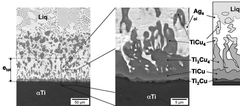
FIGURE 3.9 – Séquence réactionnelle à l'interface solide/liquide du couple Ti/Ag-40Cu saturé en Ti après 50 min à 795 °C
