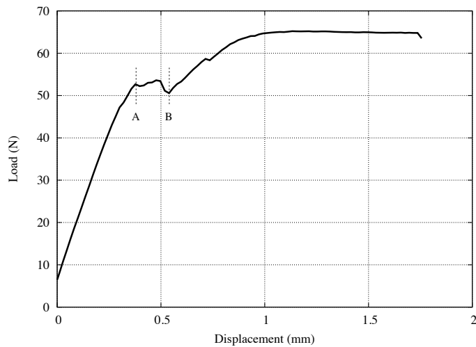
FIGURE 4.16 – Courbe Force-déplacement type obtenu lors d’un essai de flexion 4-points sur une lame Fe d’épaisseur 1 mm, aluminée dans un bain AS-7 pendant 2 min à 800 °C. La propagation de la fissure début au point A et s’achève au point B, lorsque les appuis intérieurs sont atteints.
