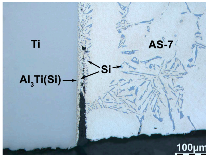
FIGURE 4.5 – Micrographie optique après un essai de push-out interrompu à 60% de la force maximale, c'est à dire pour un niveau de chargement proche du début de l'endommagement constaté par émission acoustique. Présence d'une fissure proche de la zone interfaciale au niveau de la face inférieure.
