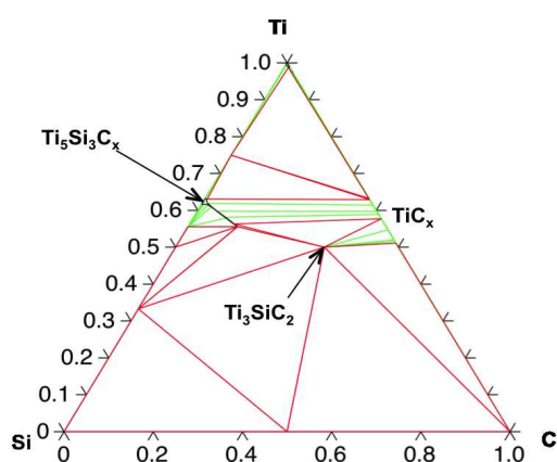
FIGURE 3.22 – Section isotherme à 800 °C du système C-Si-Ti
