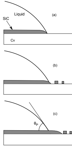
FIGURE 2.7 – Représentation schématique de la configuration à la ligne triple (a) pour \theta < \theta_N , contact direct entre le liquide et le substrat initial conduisant à un fort couplage entre réaction locale et cinétique d'étalement. (b) à \theta = \theta_N , le liquide n'est plus en contact direct avec le substrat, le couplage est faible, et l'extension du film se fait par germination et croissance de particules de P en avant de la ligne triple (c) quand \theta_P est atteint, la croissance du produit de réaction en avant de la ligne triple se poursuit mais est maintenant totalement découplée du processus d'étalement.
