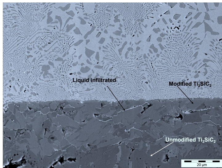
FIGURE 3.18 – Micrographie électronique de l'interface Ag-28wt.%Cu / \text{Ti}_3\text{SiC}_2 après 420 s de contact à 800 °C et un traitement de la surface de \text{Ti}_3\text{SiC}_2 de 15 min à 900 °C sous vide. La composition des phases résulte d'une analyse en microsonde de Castaing.
