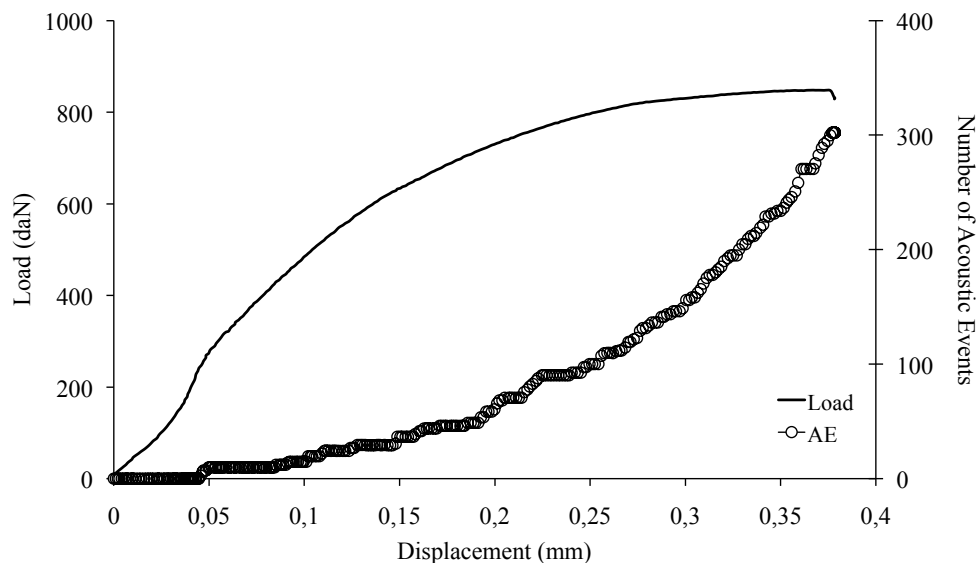
FIGURE 4.8 – Courbe Force-Déplacement typique obtenue lors d'un essai de flexion circulaire d'une matrice AS-7 renforcée par un insert Ti dans le cas d'une tranche d'épaisseur 5 mm.
