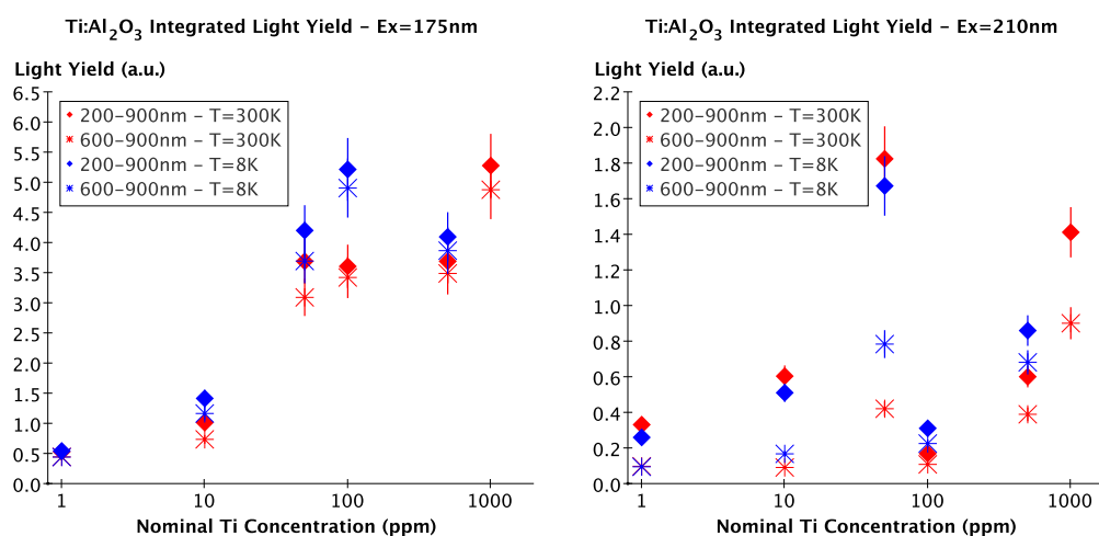
Figure 6.3 – Spectres d’émission intégrés pour les différentes concentrations en Ti, sur les plages 200-900 nm et 600-900 nm à 300 K et 8 K pour deux excitations : (gauche) 175 nm (7.1 eV) et (droite) 210 nm (5.9 eV). Les points à 1 ppm représentent le cristal F + , mais ne reflètent en rien sa concentration en Ti.
