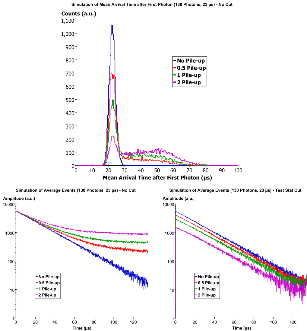
Figure 4.18 – Simulations Monte-Carlo montrant des événements de scintillation présentant une unique constante de 23 \mu\text{s} et une moyenne de 130 photons par événement primaire, correspondant aux mesures du BGO à 30 K (voir Chapitre 5), et présentant de l'empilement d'événements dont le nombre d'empilements est donné en valeur moyenne et suit des fluctuations de Poisson. Haut : distribution des temps moyens d'arrivée des photons dont la valeur moyenne permet d'appliquer la coupure sur le test statistique. Bas-gauche : avant coupures il y a apparition d'une constante de temps longue artéfact lorsqu'il y a de l'empilement. Bas-droite : la coupure sur le test statistique permet de supprimer les événements présentant de l'empilement. Toutefois la coupure perd en efficacité plus y a d'empilements.
