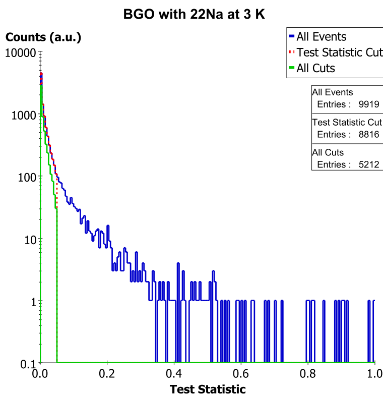
Figure 4.17 – Distribution du test statistique. La valeur de référence est obtenue à partir de l’ajustement de la Figure 4.15. Bleu : Histogramme des tous les évènements. Rouge pointillé : Histogramme des évènements après la coupure sur le test statistique. Vert : Histogramme des évènements après toutes les coupures.
