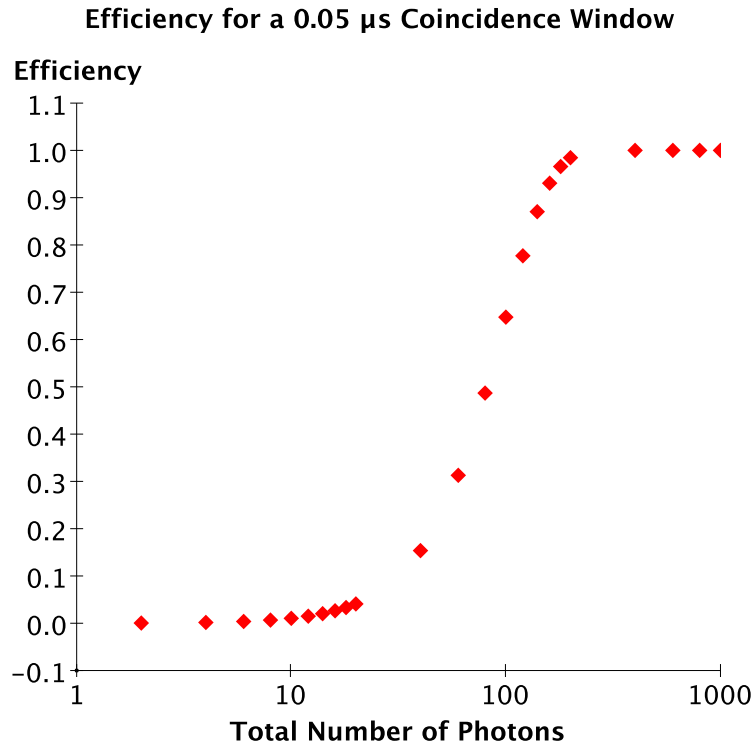
Figure 5.11 – Efficacité de déclenchement pour les mesures du BaF_2 à 3 K avec une fenêtre de coïncidence de 50 ns en fonction du nombre total de photons (sommés des photons dans les 2 PMTs) en considérant un nombre égal de photons dans chaque PMT (voir équation 4.2.10).
