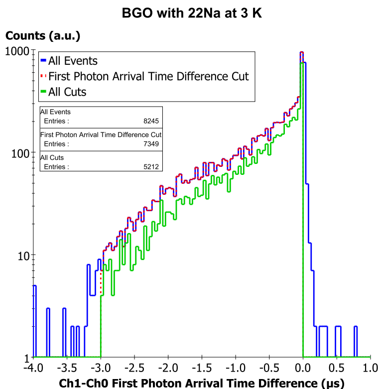
Figure 4.21 – Distribution de la différence des temps d'arrivée des premiers photons entre le cristal de référence (Ch1) et le cristal dans le cryostat (Ch0). Bleu : tous les événements. Rouge pointillé : après la coupure sur la différence des temps d'arrivée du premier photon. Vert : après toutes les coupures.
