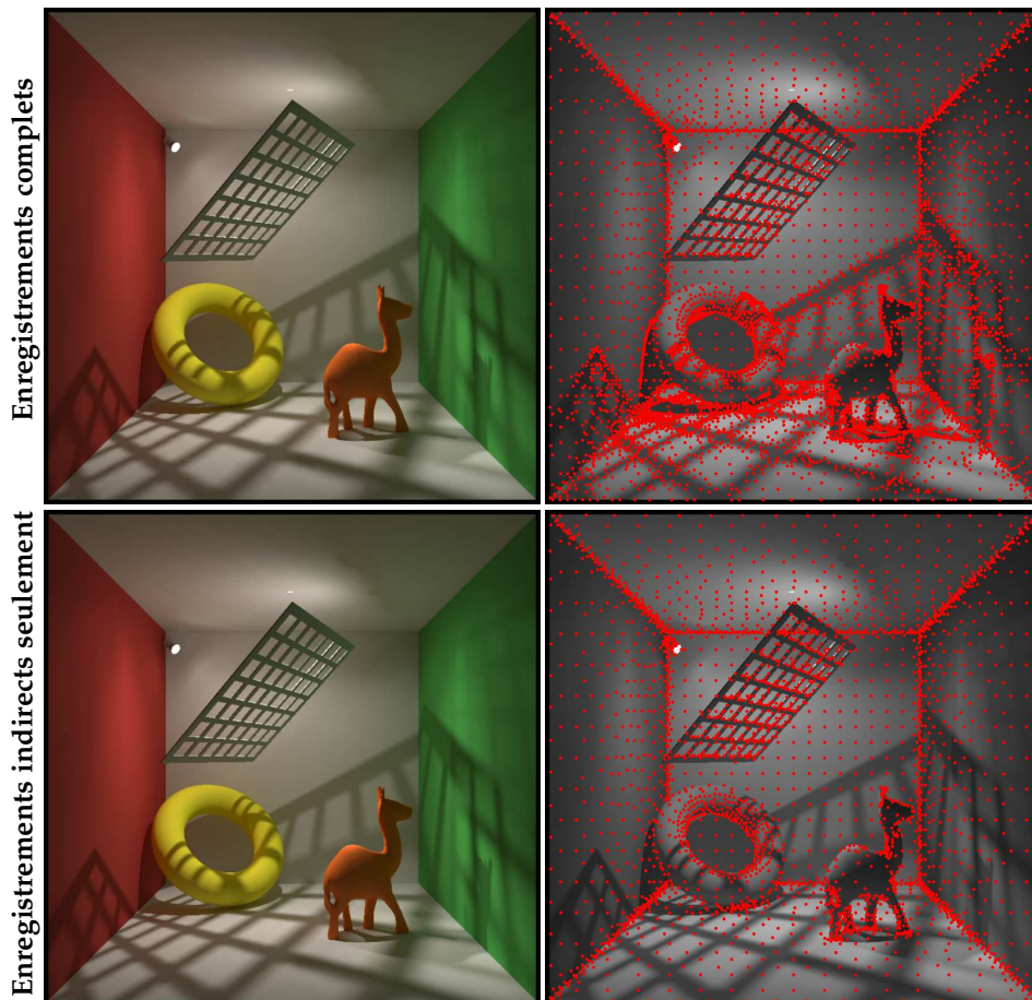
FIG. 2.12: Une scène composée de surfaces courbes (concaves et convexes) et présentant des changements d'éclairage hautes fréquences. La première ligne est calculée avec des enregistrements adaptatifs stockant les contributions directes et indirectes. La seconde ligne est quant à elle calculée avec des enregistrements adaptatifs ne stockant que les contributions indirectes (l'éclairage direct est recalculé durant la phase de rendu). Le résultat de la seconde ligne offre une meilleure qualité mais nécessite deux fois plus de temps de calcul.
