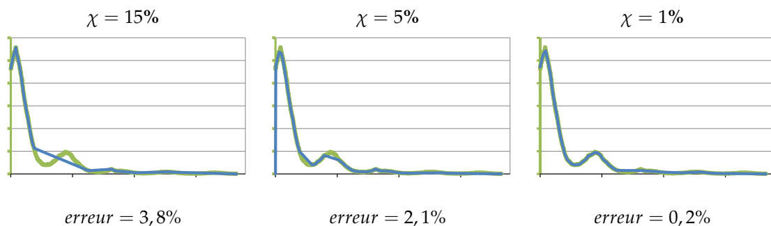
FIG. 2.12: Test de la précision de la méthode d'ajout pour la scène du couloir pour différentes valeurs de \chi . Les erreurs relatives entre la valeur réelle (la courbe verte) et l'estimation (la courbe bleue) de l'intégrale de la luminance incidente diffusée et atténuée \int_{x_e}^{x_s} \tau(x_e, x) \sigma(x) L_i(x, \vec{\omega}) dx sont données sous chaque graphe.
