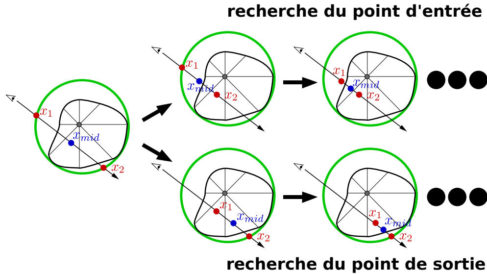
FIG. 2.4: Le processus de recherche approximative par dichotomie des intersections d'un rayon avec la zone d'influence d'un enregistrement : la sphère englobante est représentée en vert. La recherche est initialisée avec les points x_1 et x_2 (les intersections avec la sphère englobante) et le point x_{mid} (le point au milieu du segment |\overline{x_1x_2}| ). Pour le point d'entrée, la recherche est réalisée entre x_1 et x_{mid} et pour le point de sortie entre x_{mid} et x_2 . La recherche est faite entre un point à l'intérieur et un point à l'extérieur de la zone d'influence. Le processus recommence ensuite n fois. Le dernier point à l'intérieur de la zone d'influence est le point recherché.
