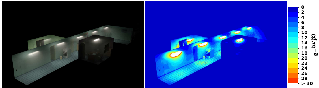
FIG. 2.18: Résultat obtenu avec la scène du couloir et l'image en fausse couleur représentant les niveaux de luminance. L'échelle, en \text{cd.m}^{-2} , est donnée à droite.
