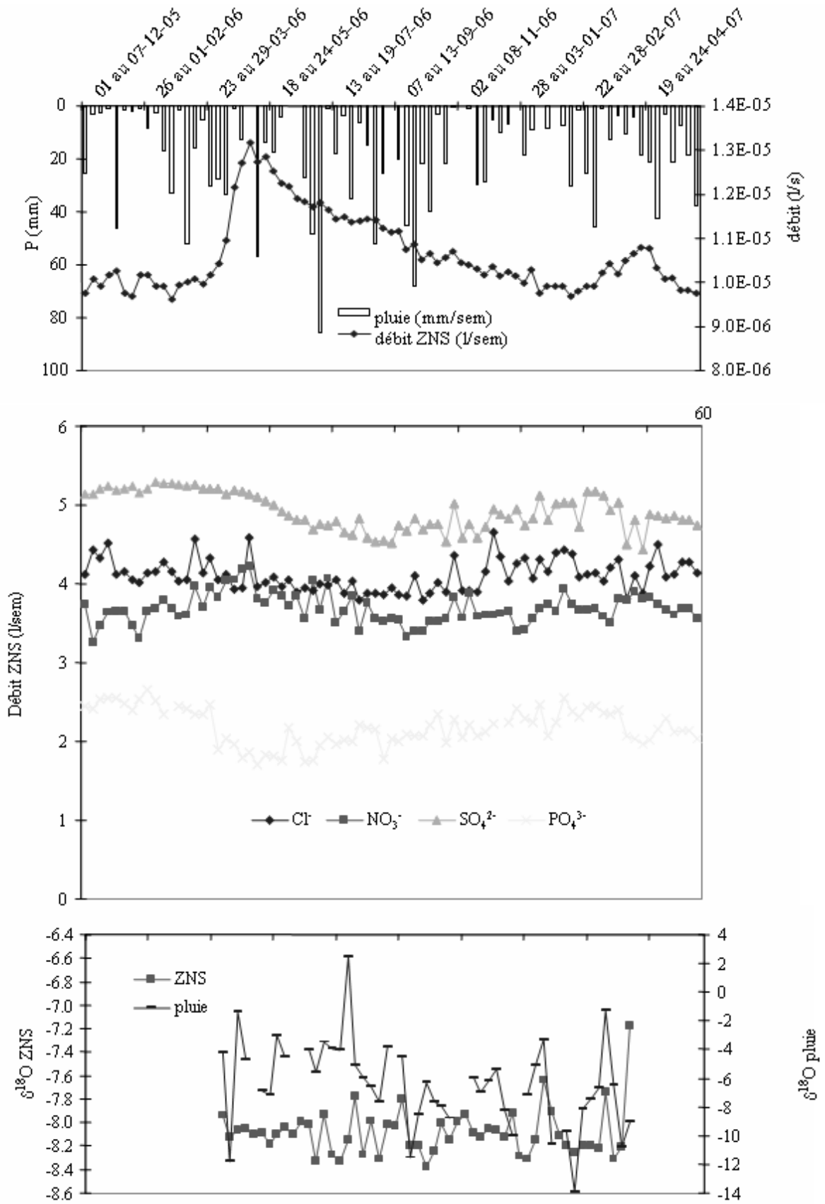
Figure III-13 : Evolution temporelle du NO 3 - , Cl - , SO 4 2- , PO 4 3- et δ 18 O dans la ZNS des Grosliers.
