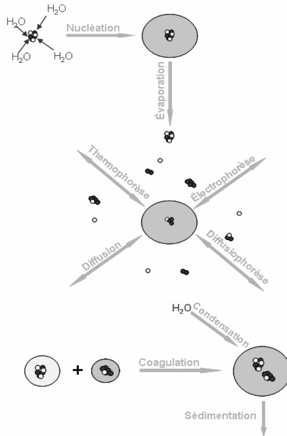
Figure II-1 : Processus se déroulant lors du rainout des aérosols particulaires (d'après Hales, 1995).
