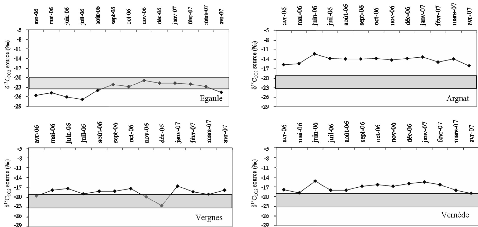
Figure IV-20 : Evolution temporelle du \delta^{13}C_{CO_2} des émergences du bassin d'Argnat.
