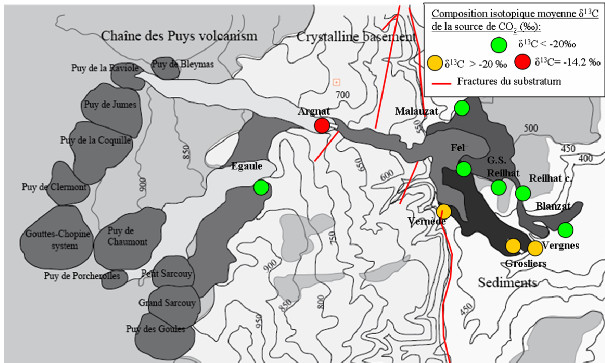
Figure IV-22 : Distribution spatiale du \delta^{13}C_{CO_2} source sur le bassin d'Argnat (avril 2006-avril 2007).
