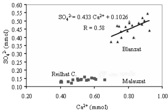
Figure IV-13 : Ca 2+ vs SO 4 2- à Blanzat, Malauzat et Reilhat captée.
