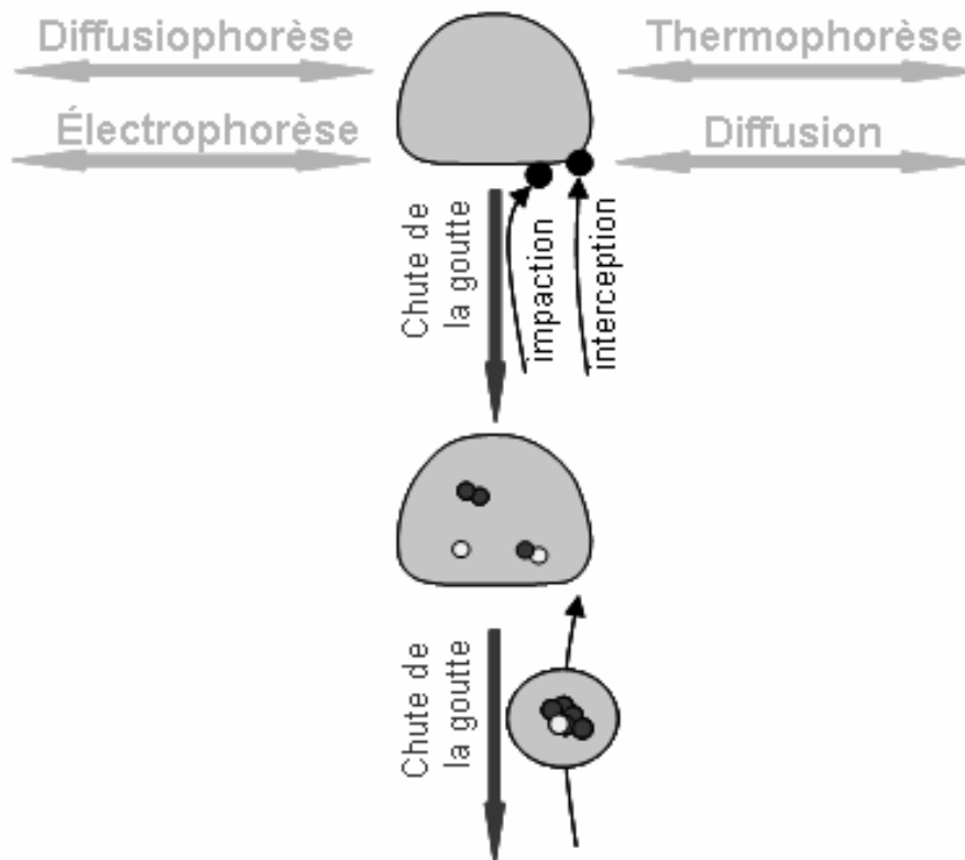
Figure II-2 : Processus se déroulant lors du washout des aérosols particulaires (d'après Hales, 1995).
