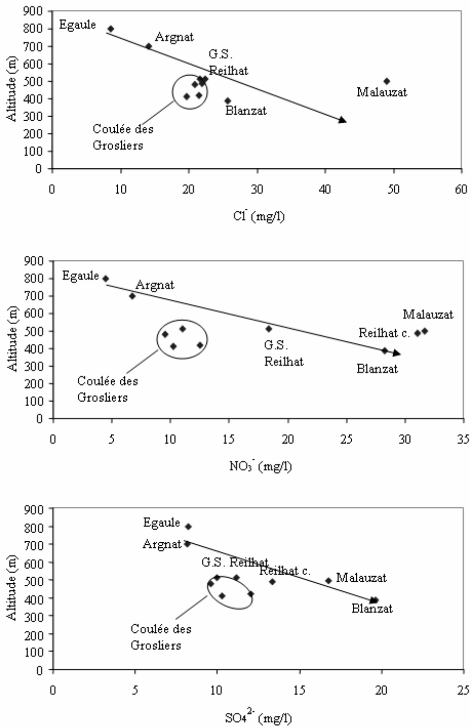
Figure IV-12 : Evolution amont-aval des teneurs moyennes en Cl - , NO 3 - , SO 4 2- .
