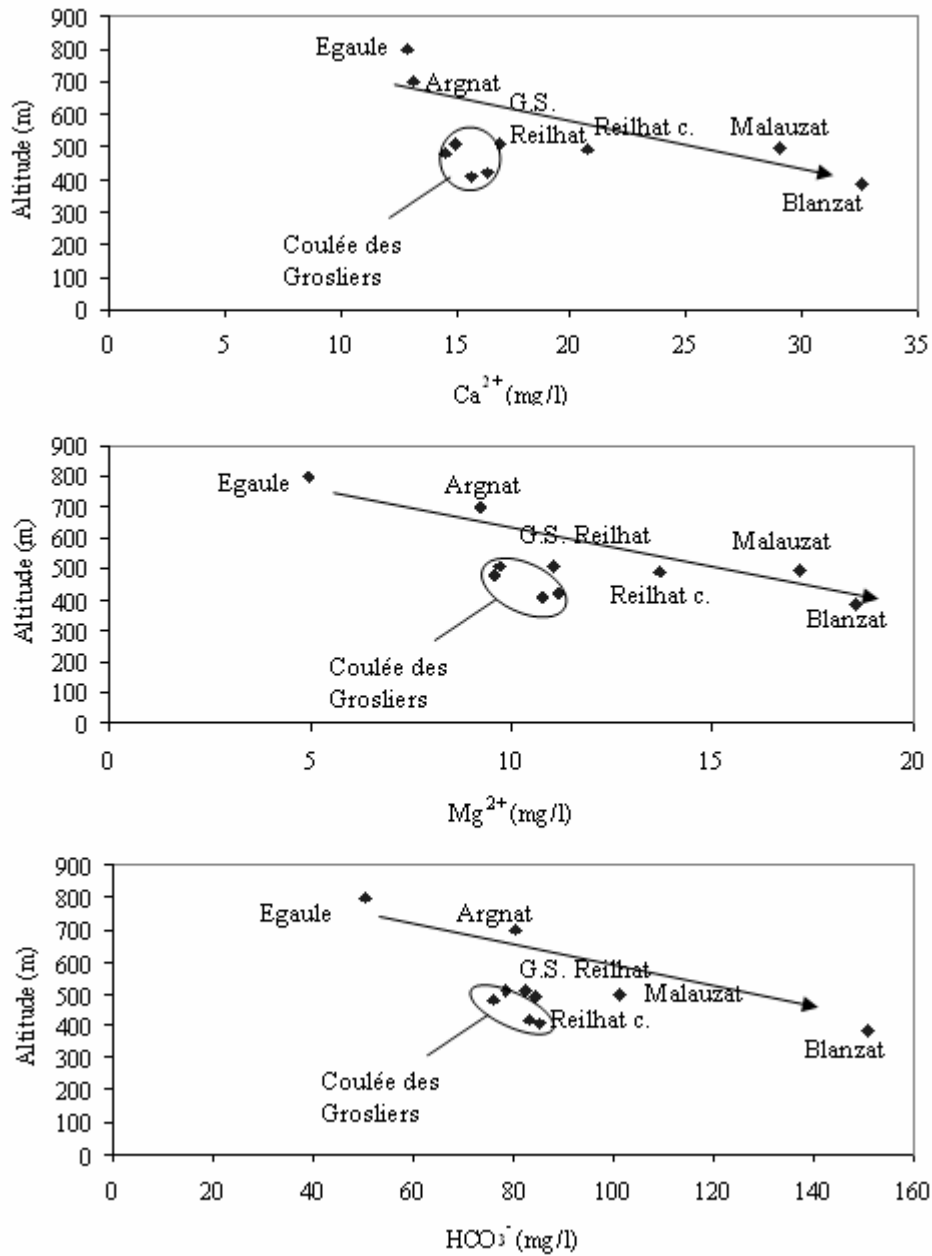
Figure IV-17 : Evolution amont-aval des teneurs moyennes en Ca 2+ , Mg 2+ et HCO 3 - .
