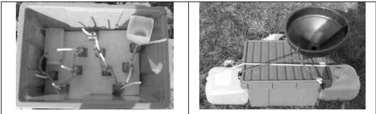
Figure I-13 : Pluviocollecteur séquentiel.
