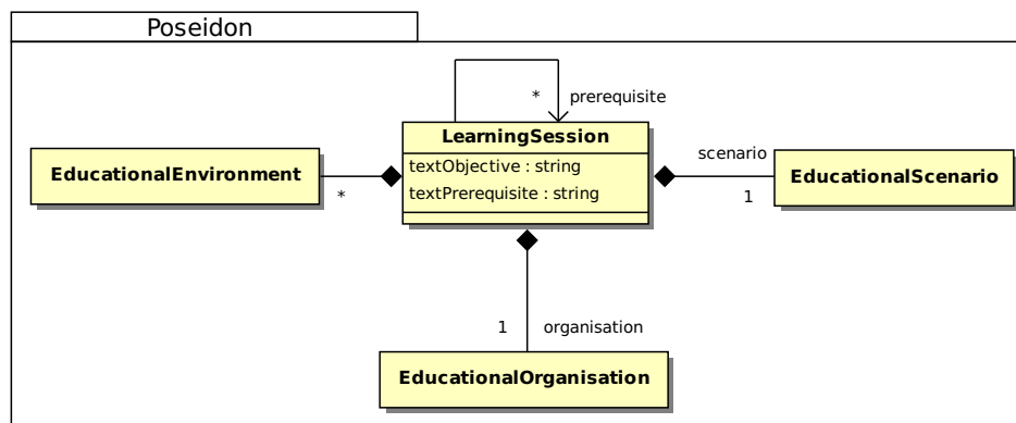
FIGURE 4.4 – Diagramme de classes synthétique des principaux éléments du modèle.
