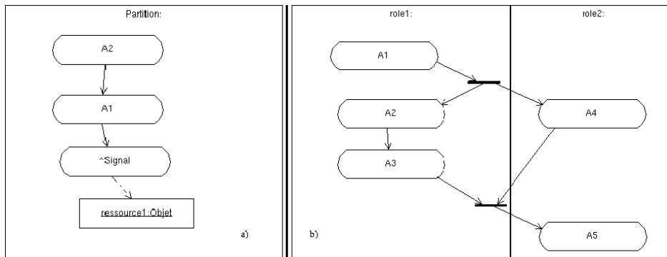
FIGURE 2.26 – Interprétation des ControlNode .
