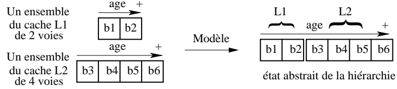
FIG. 2.11: Modélisation des hiérarchies de caches exclusives sous la forme d'un état abstrait de la hiérarchie (cas particulier où le nombre d'ensembles du L1 est égal à celui du L2).
