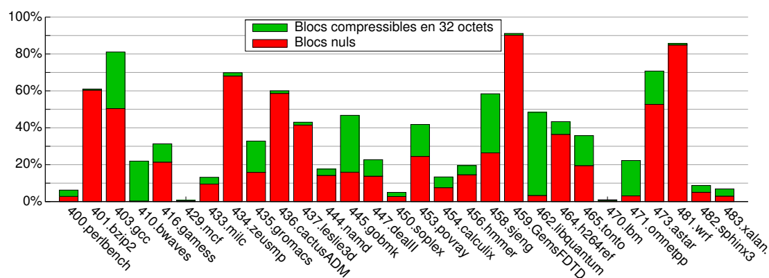
FIGURE 4.1 – Taux de blocs de 64 octets nuls ou compressibles en 32 octets avec FPC après 50.10^9 instructions présents en mémoire dans les pages accédées.
