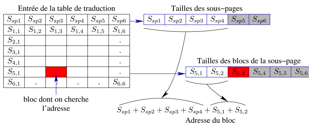
FIGURE 1.8 – Traduction d'adresse. S_{sp_i} est la taille de la sous-page i et S_{i,j} est la taille du j e bloc de la i e sous-page. Exemple avec le calcul de l'adresse du 3 e bloc de la 5 e sous-page obtenu grâce aux tailles des 4 sous-pages et des 2 blocs précédents.
