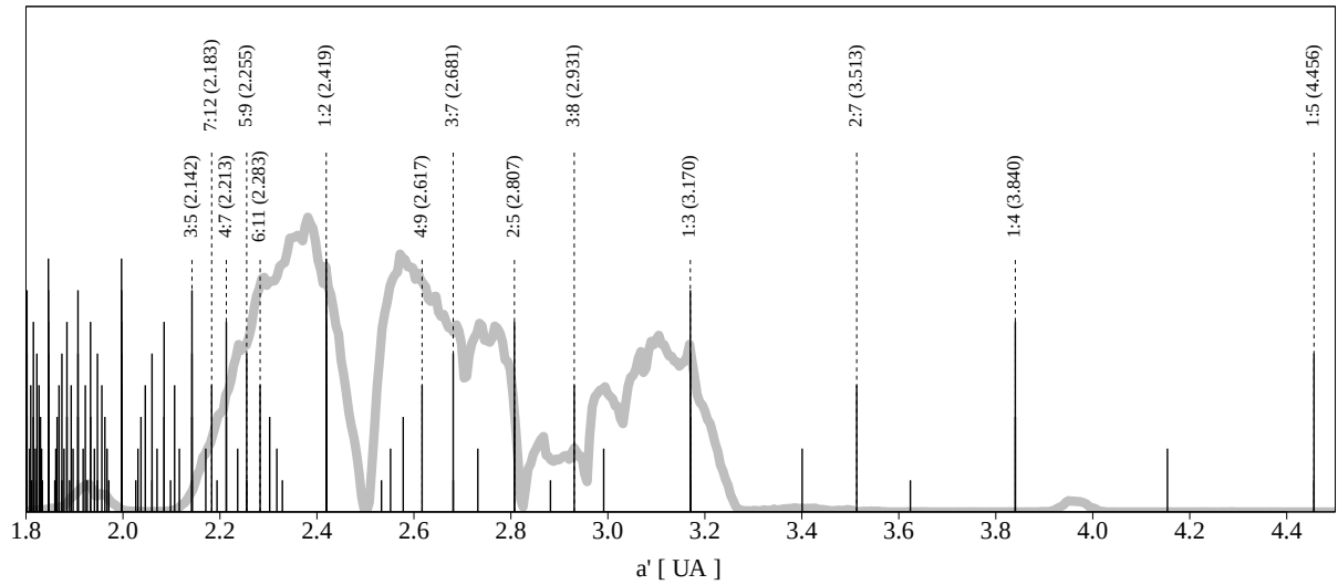
FIGURE 3.14 – Analogie de la figure 3.13, tracé pour Mars. Seulement les résonances pour lesquelles a' > 2.12 et d'ordre inférieur ou égale à 5 sont annotées.
