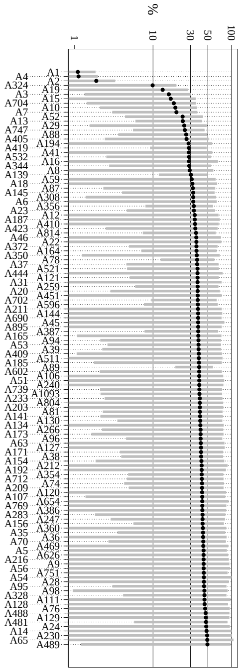
FIGURE 5.12 – Analogie de la figure 5.11 pour le modèle B. La figure représente uniquement les astéroïdes qui en moyenne s’ajustent à mieux que 50%.
