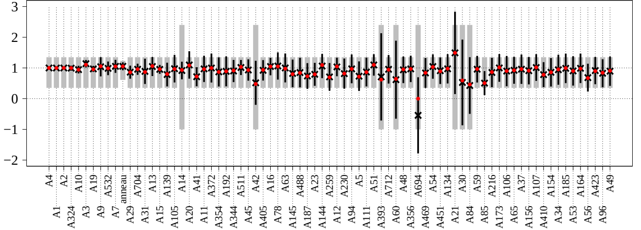
FIGURE 5.7 – Ajustement par régularisation de Tihonov simple (croix) et par régularisation avec contraintes (points rouges). Les traits verticaux représentent les incertitudes des à priori gaussiens (en gris) et les incertitude à posteriori de l’ajustement sans contraintes (en noir).
