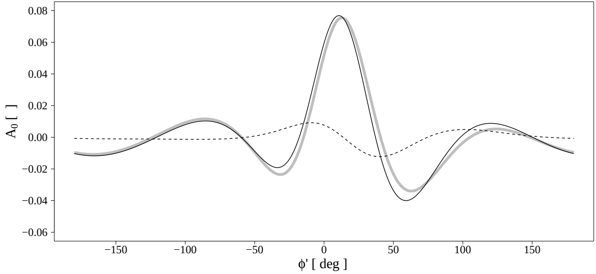
FIGURE 7.5 – En gris, évolution de A_0 calculée à l'ordre 0 en (q_2^0, q_3^0, p_2^0, p_3^0) . En noir, évolution de A_0 calculée à l'ordre 3. En pointillé, la différence entre les deux courbes.
