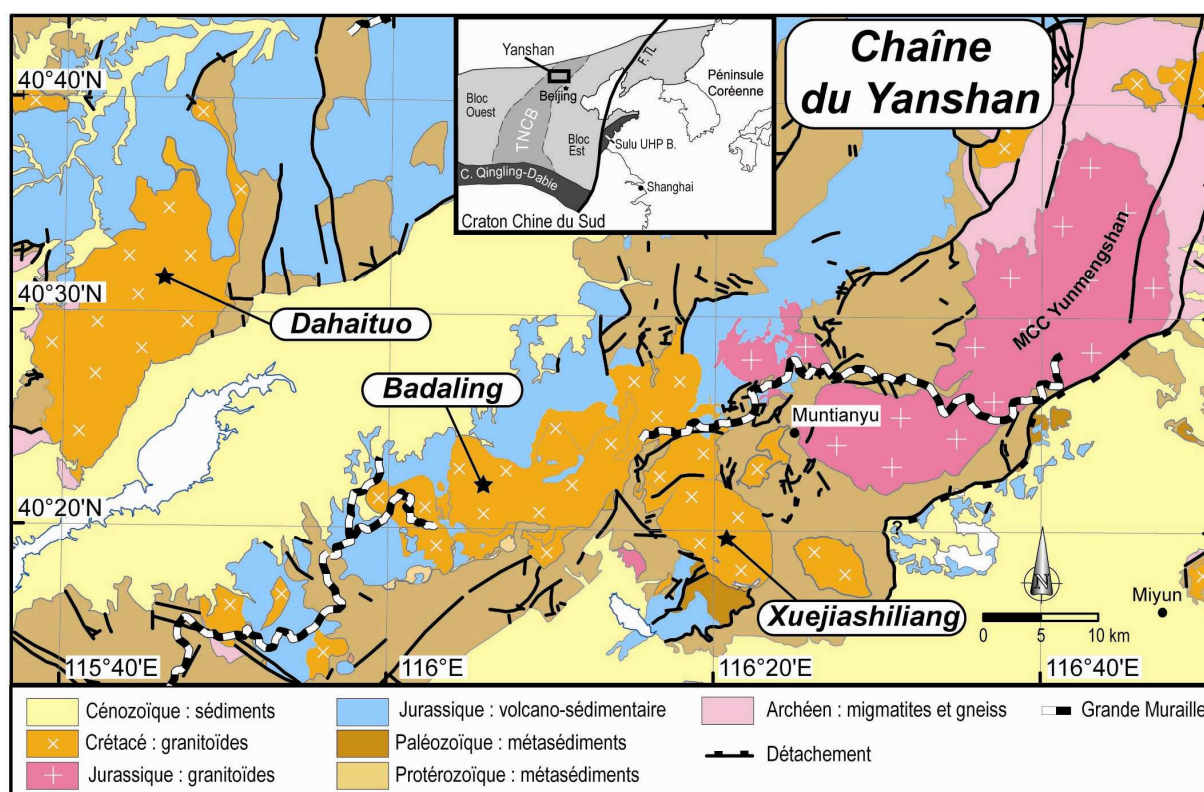
Figure 3.5 : Carte géologique simplifiée d'une partie de la chaîne du Yanshan. Les massifs faisant l'objet d'études dans la thèse sont identifiés sur la carte (Badaling, Dahaituo et Xuejiashiliang).
