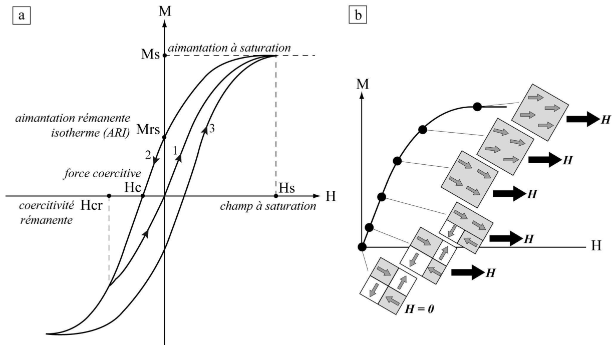
Figure A1.16 : Cycle d'hystérésis (modifié d'après Lanza et Meloni, 2006). (a) Cycle d'hystérésis avec les trois étapes (1, 2, 3) d'application du champ magnétique H et mesure de l'aimantation induite M . M_s : aimantation induite à saturation, M_{rs} : aimantation rémanente isotherme, H_s : champ magnétique appliqué à saturation, H_c : force coercitive, H_{cr} : coercitivité rémanente. (b) Evolution de la direction des moments magnétiques au cours de l'application du champ magnétique H (segment 1 du cycle d'hystérésis).
