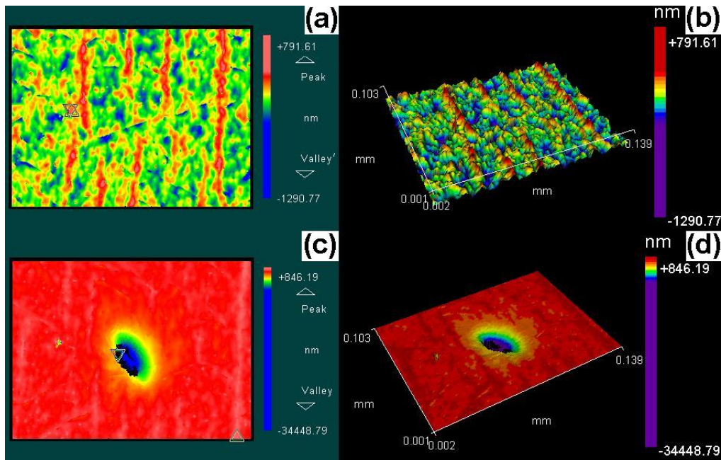
FIG. 5.22 – Images réalisées par profilométrie optique d'un dépôt d'AlN de 7 \mu\text{m} d'épaisseur sur substrat de SiC 4H (0001) 8°off montrant le phénomène de “step bunching” (a et b) et mise en évidence d'un défaut de type “micropipe” (c et d).
