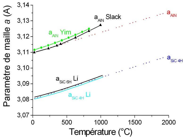
FIG. 4.6 – Variations des paramètres de maille a_{\text{AlN}} et a_{\text{SiC } 6\text{H}} en fonction de la température. Le paramètre a_{\text{AlN}} est calculé à partir du coefficient de dilatation thermique linéaire de AlN [42] (en rouge) et comparé aux valeurs expérimentales mesurées par Yim et Paff [40] (en vert) et par Slack et Bartram [41] (en noir). La valeur de a_{\text{SiC } 4\text{H}} est calculée à partir du coefficient de dilatation thermique linéaire de SiC 4H (en bleu) [217] et la valeur de a_{\text{SiC } 4\text{H}} [217] et a_{\text{SiC } 6\text{H}} [218] à partir des mesures expérimentales réalisées par Li et Bradt.
