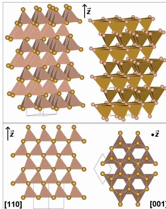
FIG. 1.4 – Structure d'AlN 2H : descriptions en termes de tétraèdres Al et N sur les images du haut ; projections des tétraèdres Al selon des axes de zone [110] et [001] sur les images du bas.
