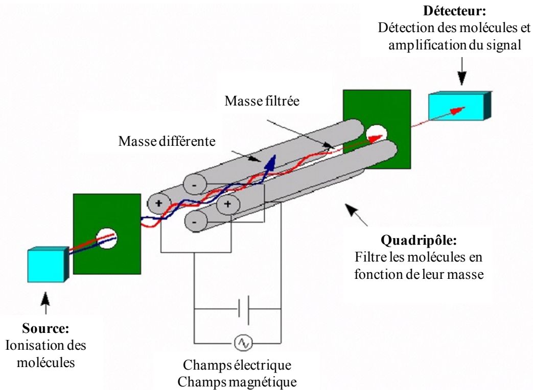
Figure 45 : Analyseur quadripôle.
