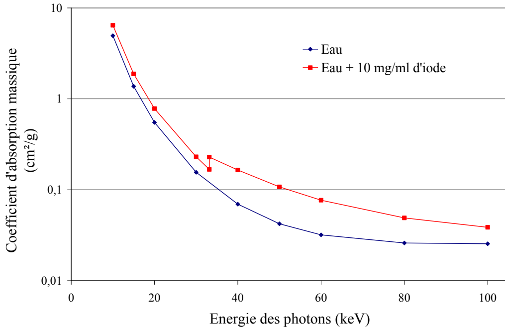
Figure 60 : Coefficients d'absorption massique de l'eau et d'un milieu iodé à 10 mg/ml (d'après le NIST) dans la gamme d'énergie utilisée pour la radiothérapie par rayonnement synchrotron.
