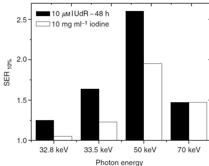
Figure 64 : Variation du SER 10% en fonction de l'énergie d'irradiation pour des cellules pré-incubées 48h avec de l'IUdR ou des cellules irradiées en présence d'ioméron (Corde et al. , 2004).
