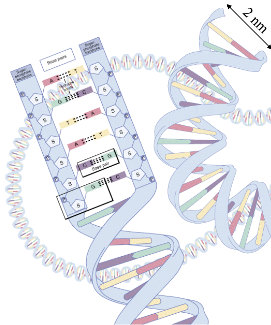
Figure 8 : Molécule d'ADN.
