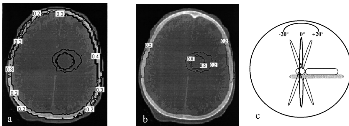
Figure 28 : Distribution de dose calculée pour une irradiation CT avec un arc (a) et avec 3 arcs (b) Vue de profil du CT scanner représentant les 3 axes coplanaires désaxés de 20 degrés (c) (Mesa et al. , 1999).
