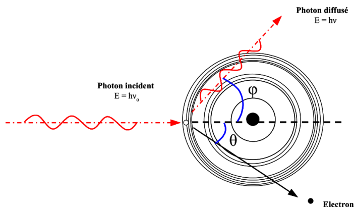
Figure 23 : Effet Compton.
