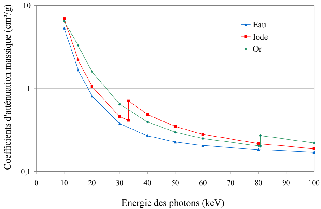
Figure 88 : Coefficients d'atténuation massique de l'eau et d'un milieu aqueux contenant 10 mg/ml en atomes lourds en fonction de l'énergie des photons (d'après le NIST).
