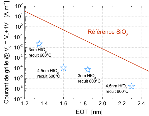
FIGURE 1.3 – Résultats électriques I_g(EOT) d'empilements HfO 2 présentant différentes épaisseurs et températures de recuit [13]. La réduction de courant par rapport au SiO 2 est indéniable mais apparaît fortement variable en fonction des conditions de procédé (les températures indiquées sont celles des recuits post-dépôt).
