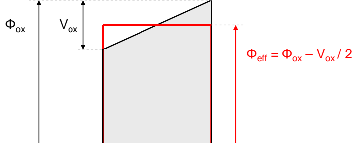
FIGURE 3.14 – Approximation d’une barrière trapézoïdale de hauteur \phi_{\text{ox}} sous potentiel V_{\text{ox}} en une barrière carrée de hauteur effective \phi_{\text{eff}} .
