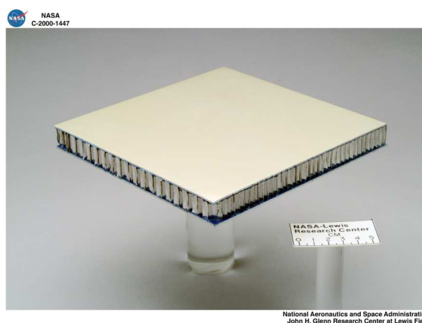
Figure 2.10 – Un panneau sandwich de très haute qualité structurale en nid d'abeilles aluminium et peaux en aluminium (Glenn, 2000)
