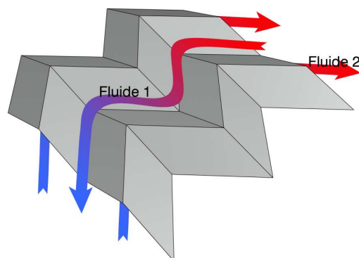
Figure 2.6 – Le fonctionnement en échangeur double flux du module à chevrons
