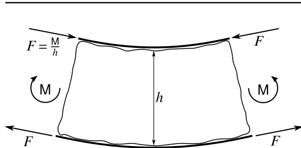
Figure 2.11 – Effet de la flexion sur les peaux
